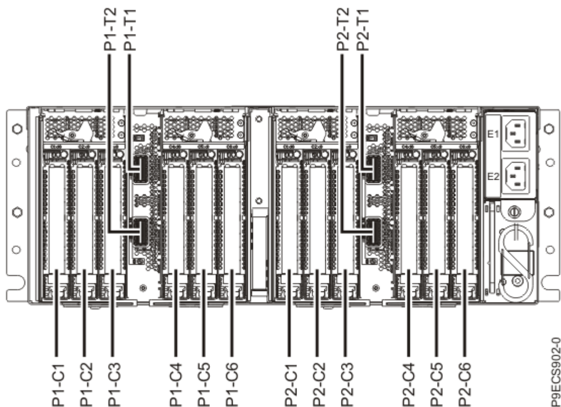
図 2. PCIe スロットのロケーション・コード付きの EMX0 PCIe3 拡張ドロワーの背面図
