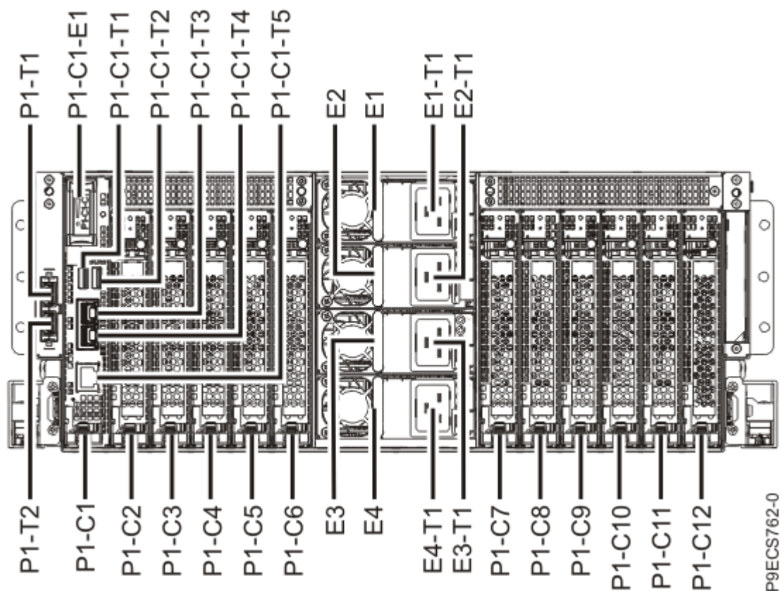
図 1. PCIe スロットのロケーション・コード付きのラック・マウント型 9040-MR9 システムの背面図
