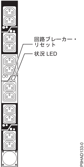
図 43. PDU コンセントの図
