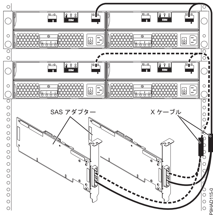
図 62. 2 つの SAS RAID アダプターと 2 つのディスク拡張ドロワー間 (マルチ・イニシエーター HA RAID 構成)
