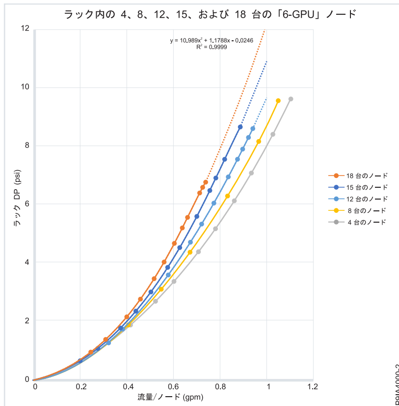
図 2. 水流量対圧力低下
