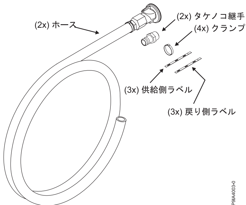
図 23. ホース・キット
