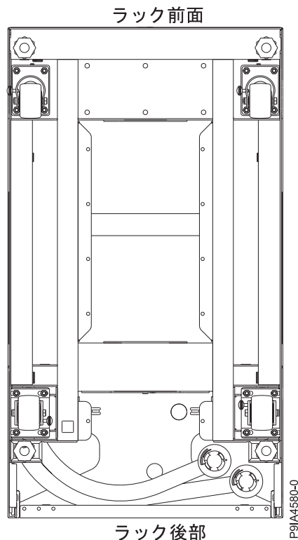
図 37. 下部ホース出口の位置 (下から見た場合)
