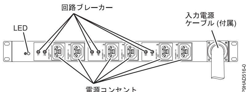
図 45. HVDC PDU
