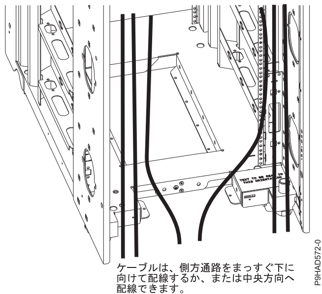
図 27. 床下ケーブル接続
