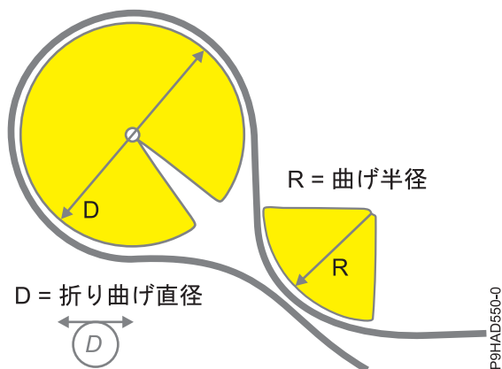
図 47. ケーブルの曲げ半径
