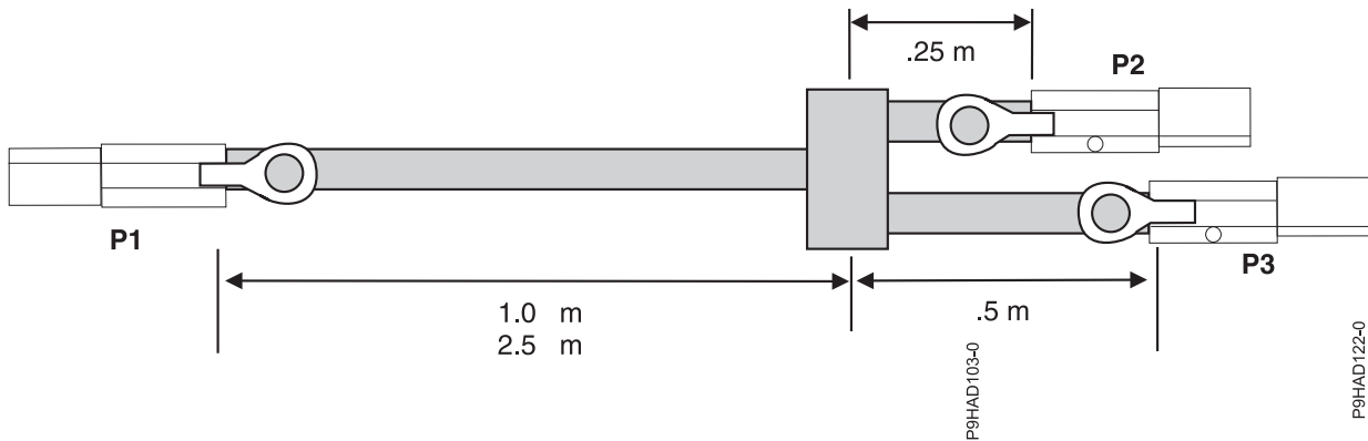
図 51. SAS 外付け YI ケーブル・アセンブリのケーブルの長さ
