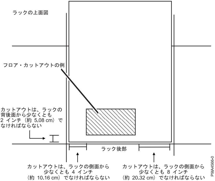
図 24. フロア・カットアウト
