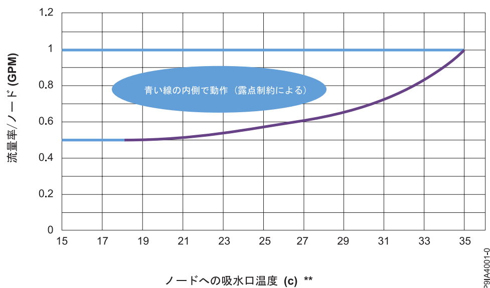
図 1. 水流量対温度
