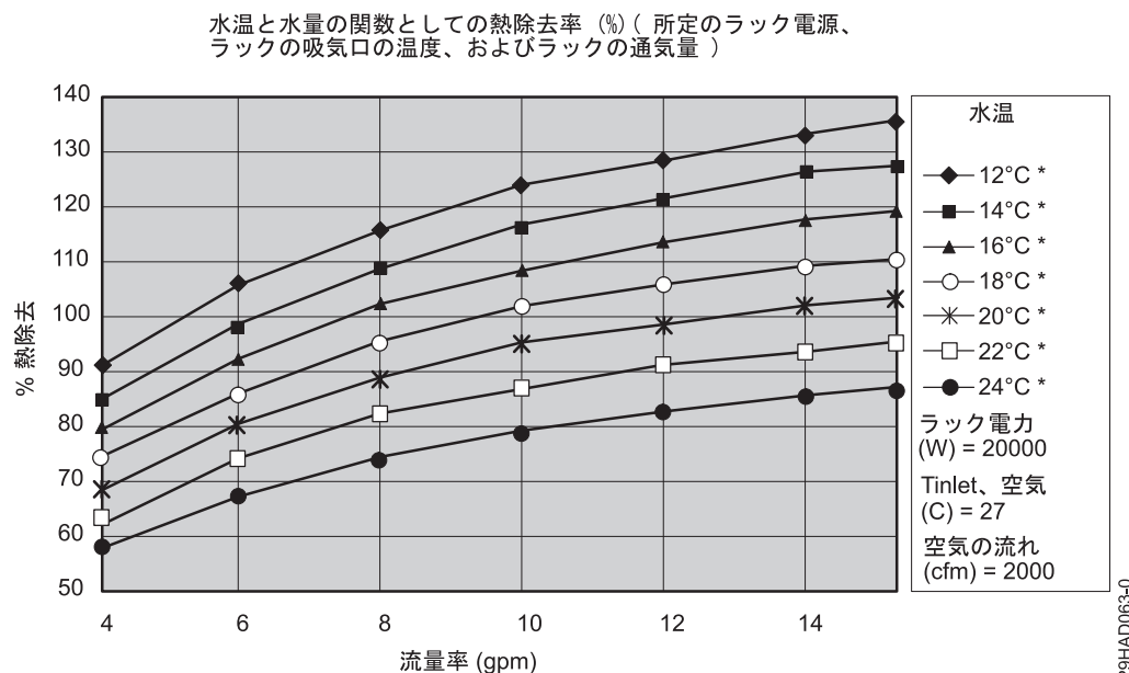
図 15. 熱負荷 20 kW のヒート・エクスチェンジャーの標準的な効率
