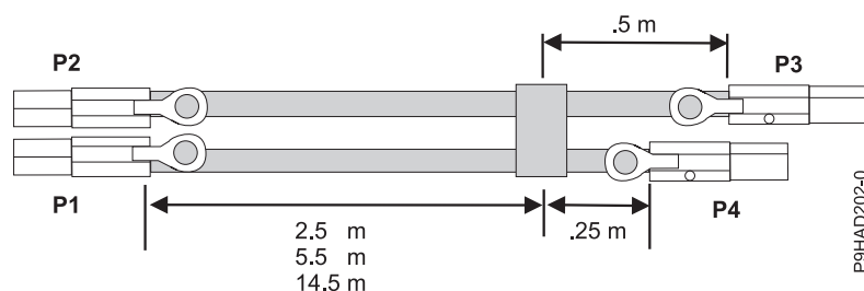
図 49. SAS 外付け X ケーブル・アセンブリのケーブルの長さ
