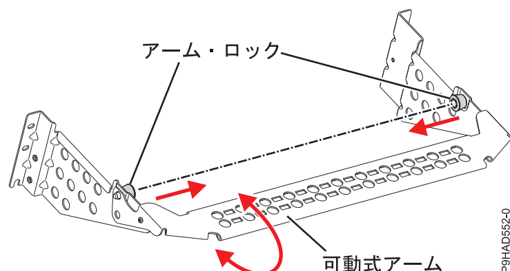
図 48. ケーブル管理ブラケット
