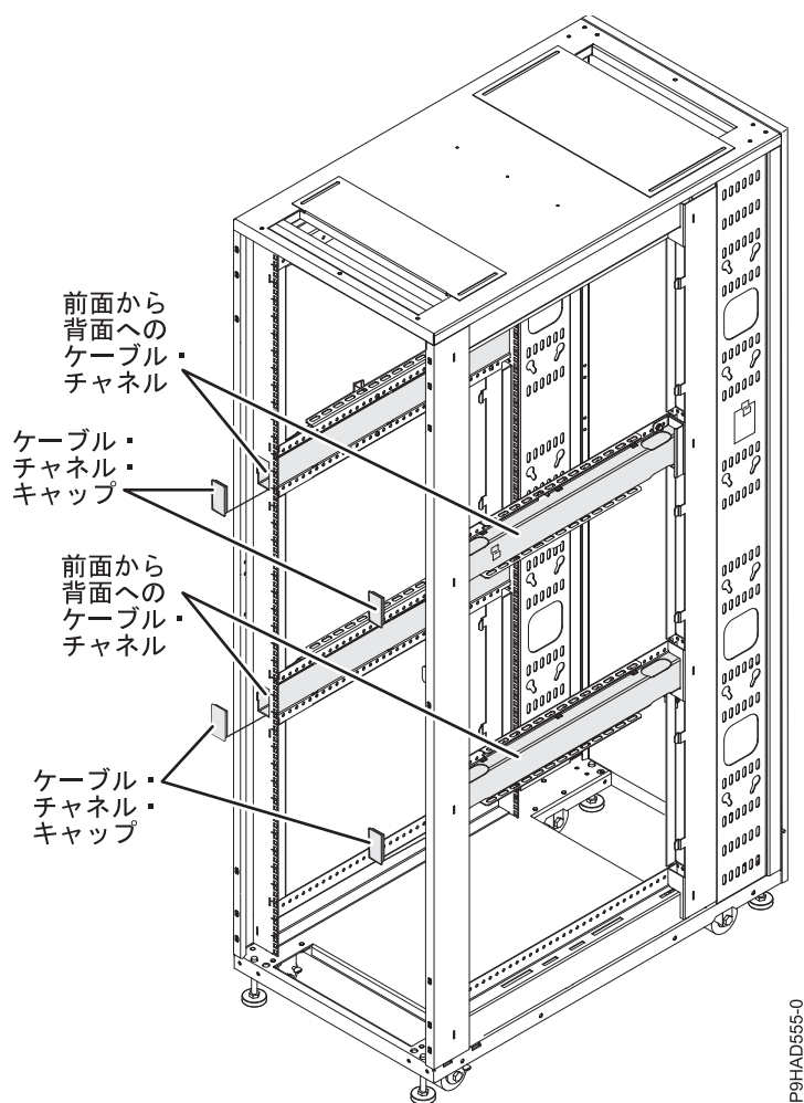
図 10. ラック内ケーブル接続
