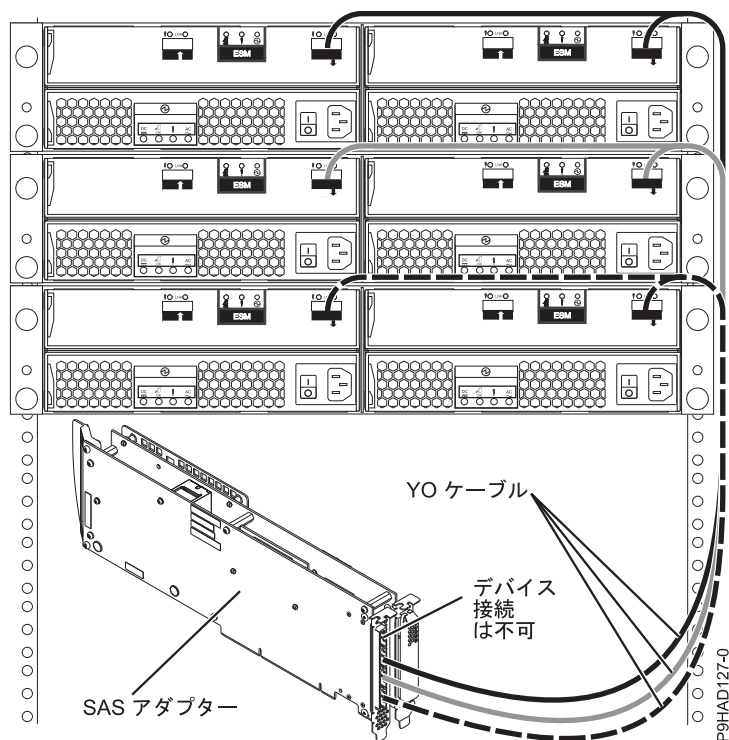
図 55. トライ・ポート SAS アダプターとディスク拡張ドロワー間
