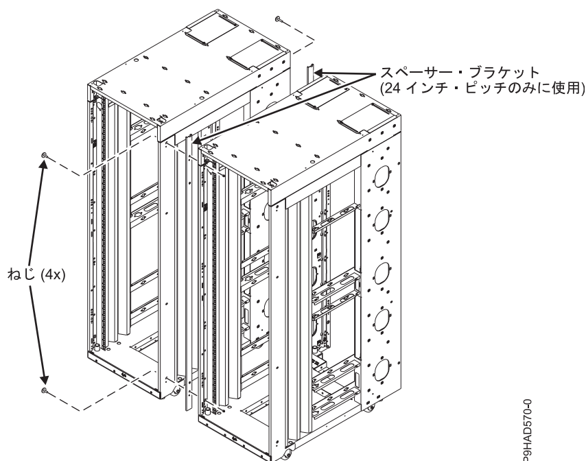
図 29. 複数のラックの接続
