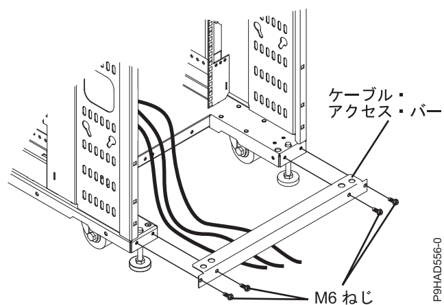
図 11. ケーブル・アクセス・バー
