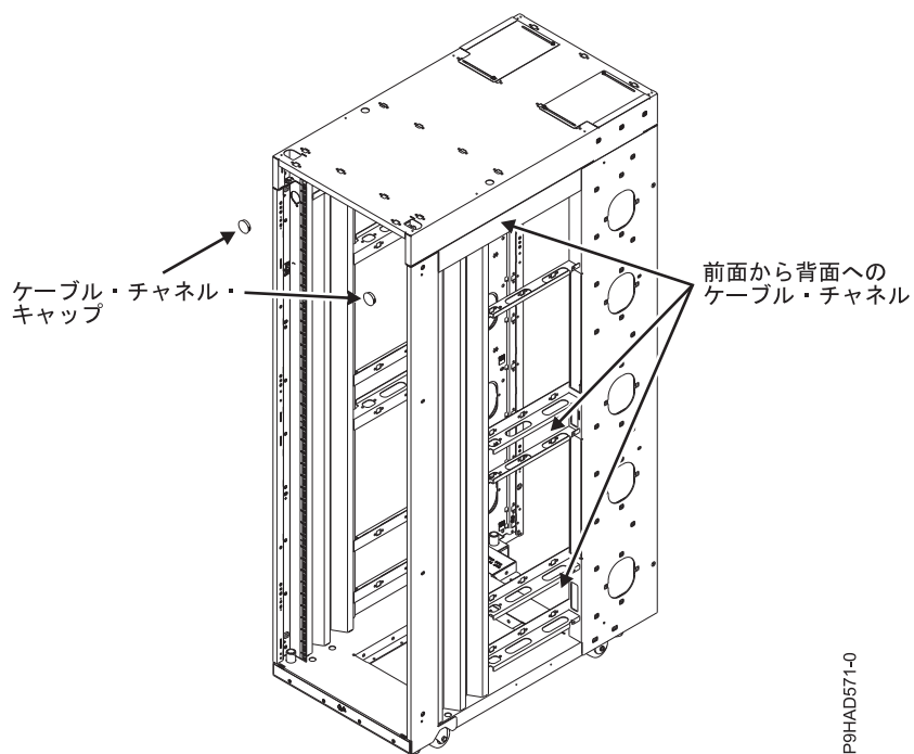
図 26. ラック内ケーブル接続
