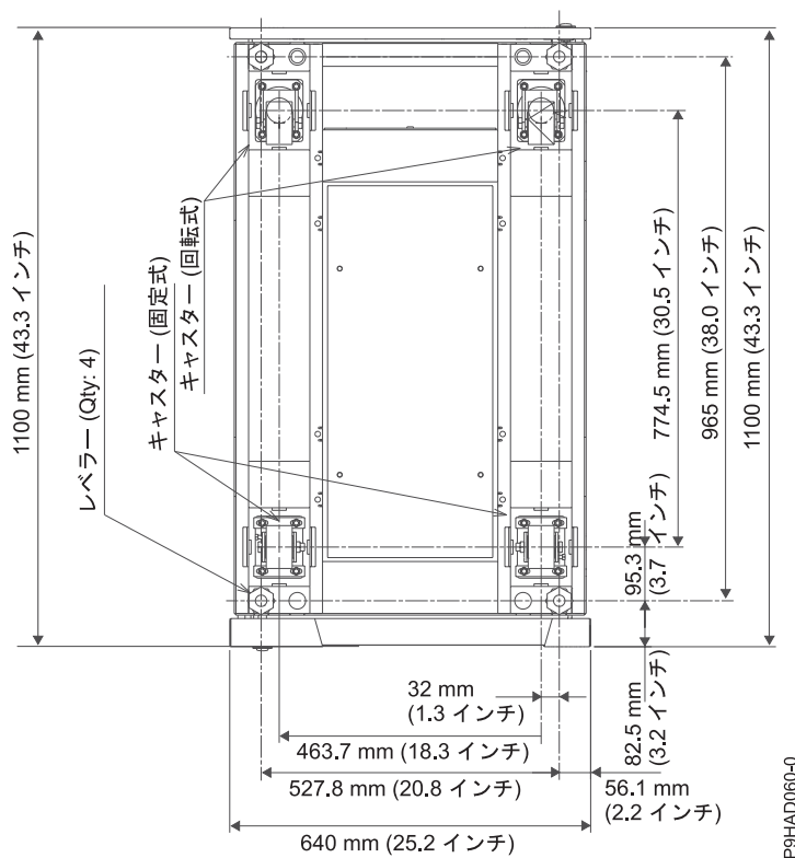
図 6. キャスターおよびレベラーの位置
