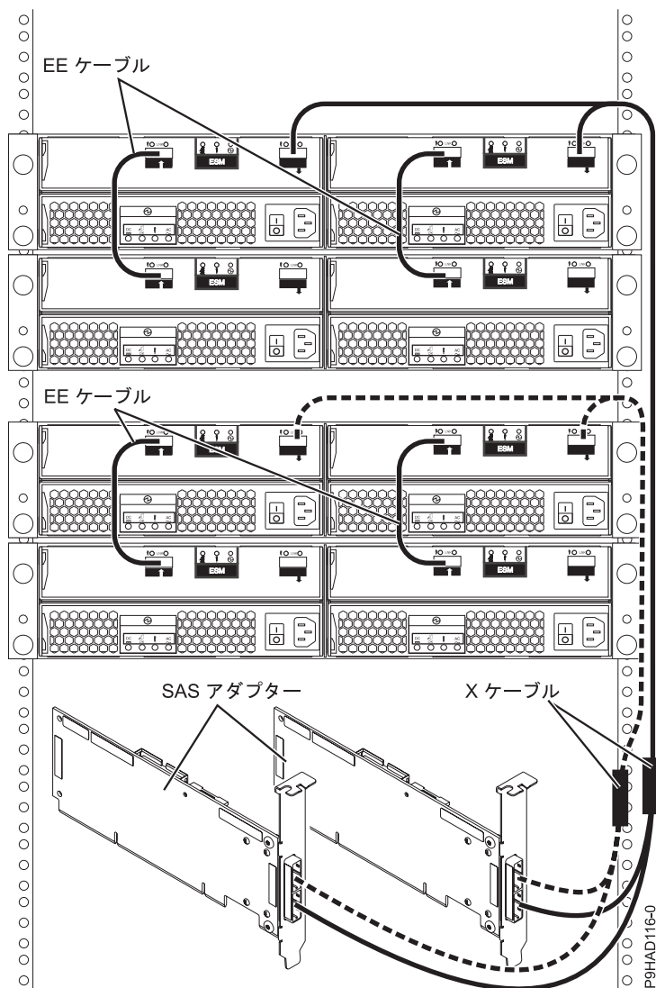
図 63. 2 つの SAS RAID アダプターと 4 つのディスク拡張ドロワー間 (マルチ・イニシエーター HA RAID 構成)
