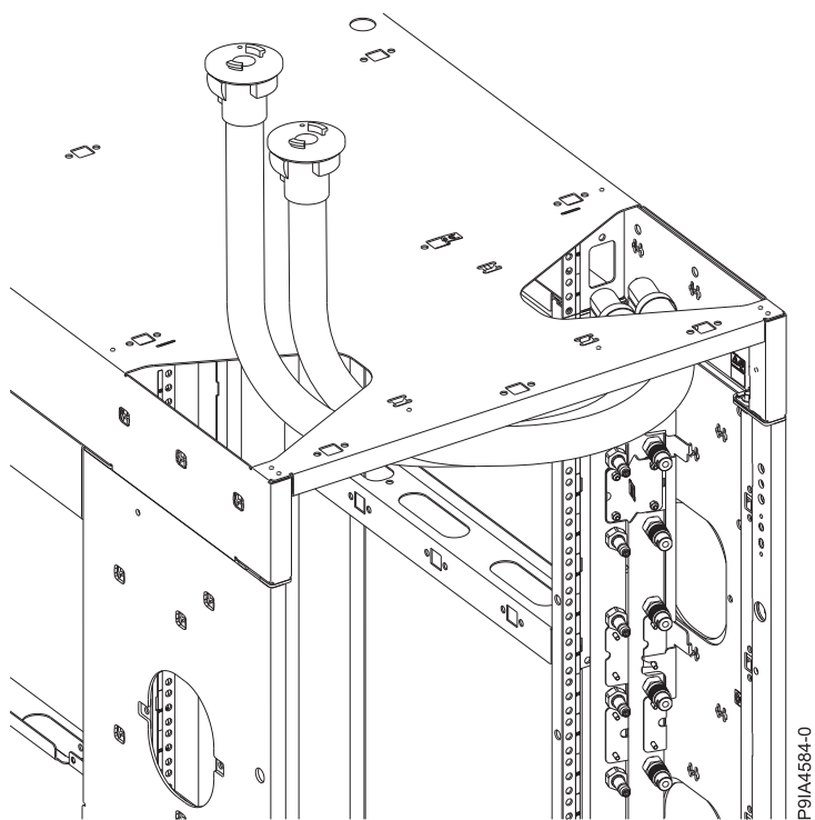
図 34. 上部ホース出口の位置
