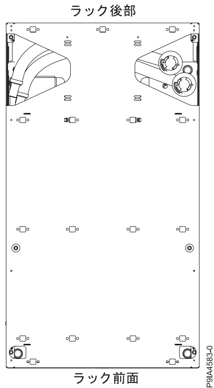
図 35. 上部ホース出口の位置 (上から見た場合)
