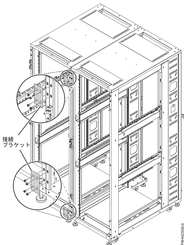
図 14. 接続ブラケット
