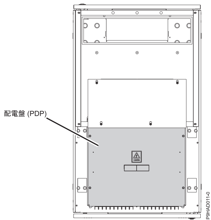
図 4. FC EPB8 - 配電盤 (上から見た図)
