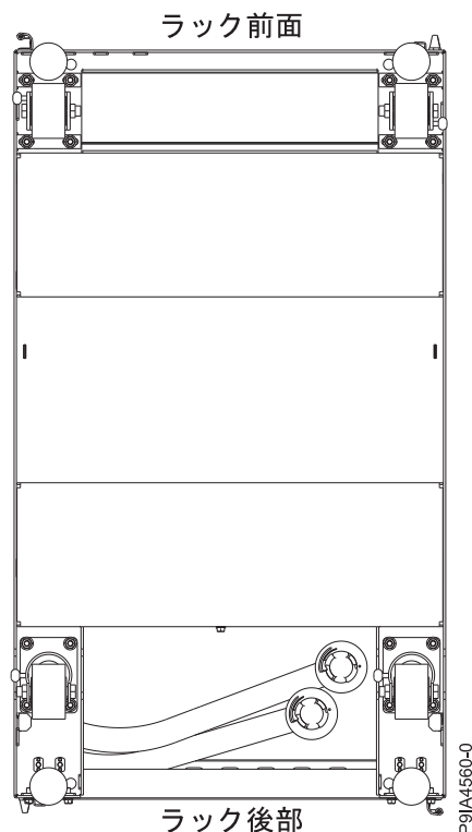
図 22. 下部ホース出口の位置 (下から見た場合)
