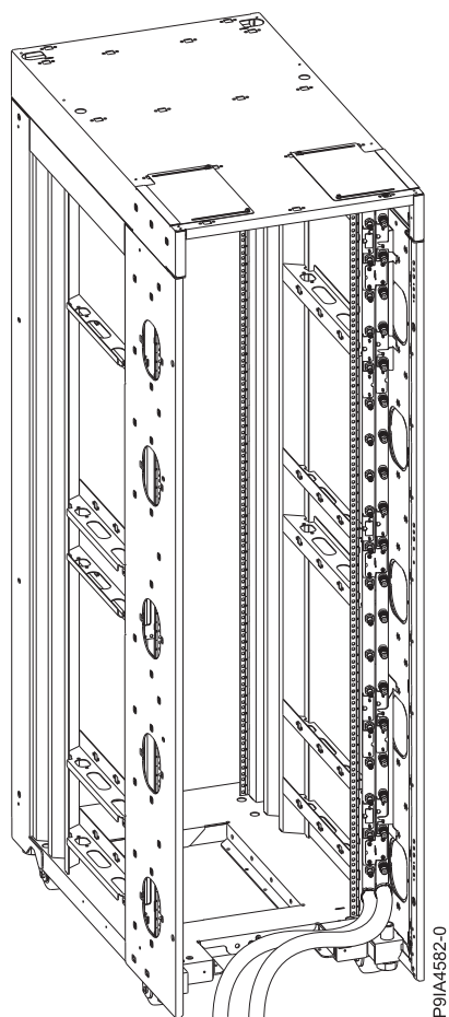
図 33. ラック、および供給ホースと返送ホースがラックの下部から出る連結管
