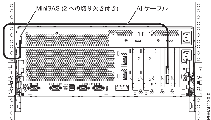
図 59. SAS アダプターと内部 SAS ディスク・スロット間 (システム外部 SAS ポートを使用)
