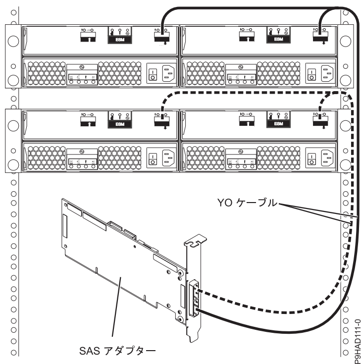
図 53. SAS アダプターと 2 つのディスク拡張ドロワー間
