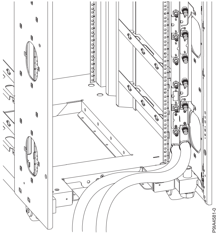
図 36. 下部ホース出口の位置
