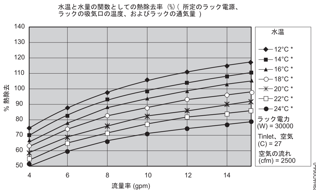
図 31. 熱負荷 30 kW のヒート・エクスチェンジャーの標準的な効率
