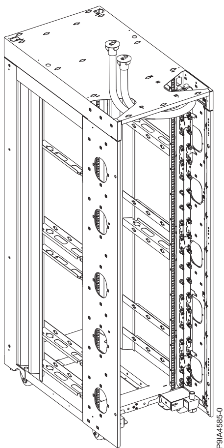
図 32. ラック、および供給ホースと返送ホースがラックの上部から出る連結管
