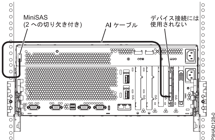
図 60. ディスク拡張ドロワーに接続された FC5904 または FC5908 アダプター
