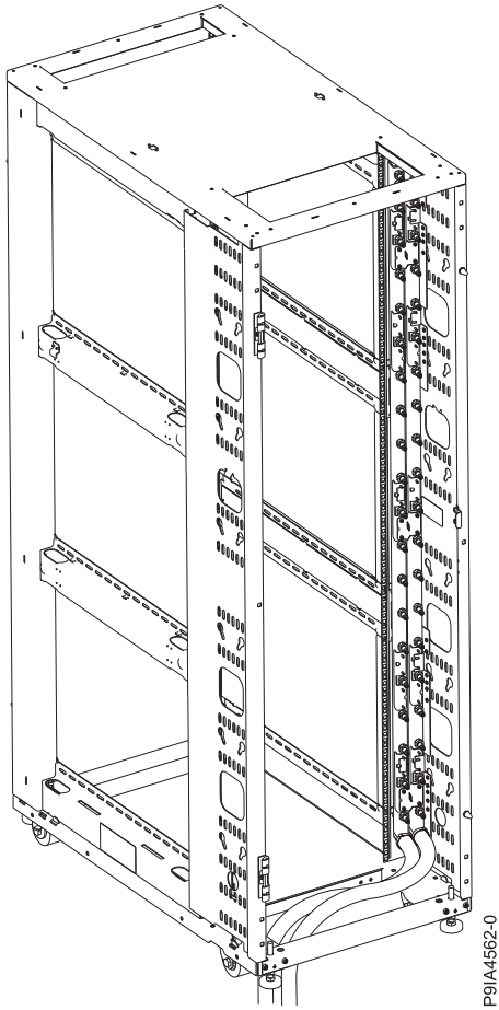
図 18. ラック、および供給ホースと返送ホースがラックの下部から出る連結管
