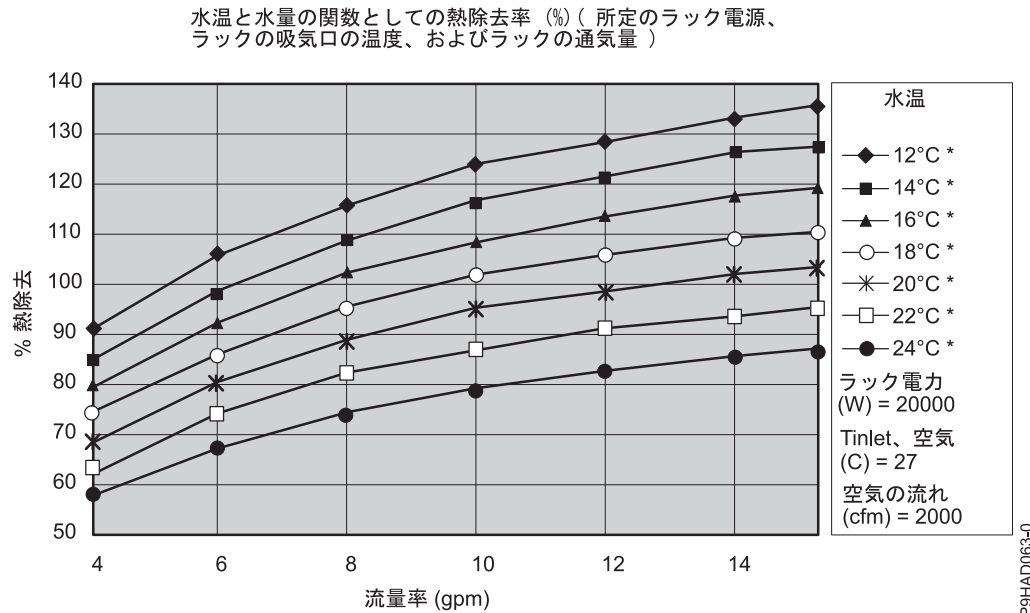
図 30. 熱負荷 20 kW のヒート・エクスチェンジャーの標準的な効率
