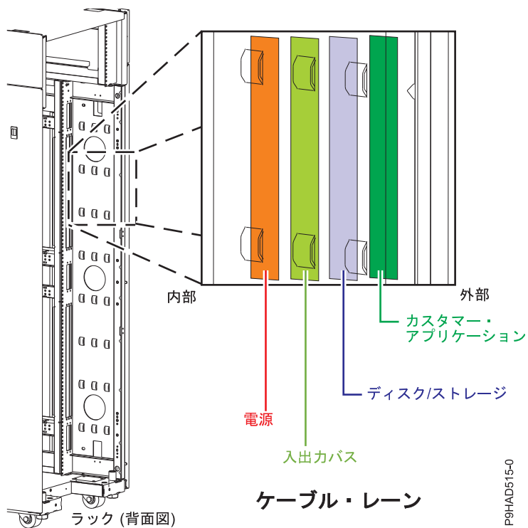
図 46. ケーブル管理ブリッジのレーン
