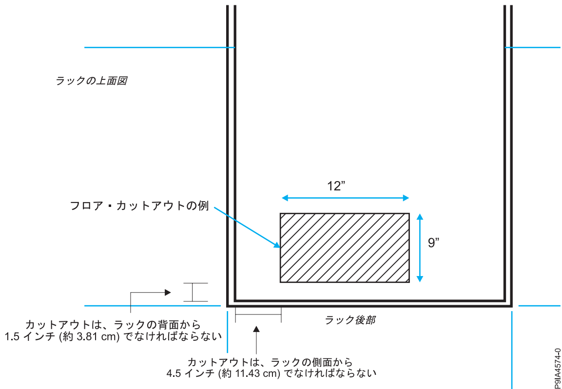
図 39. フロア・カットアウト
