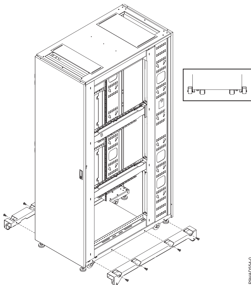
図 13. アウトリガーの位置
