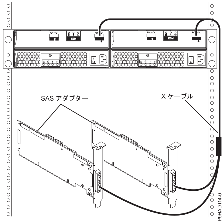
図 61. 2 つの SAS RAID アダプターと 1 つのディスク拡張ドロワー間 (マルチ・イニシエーター HA RAID 構成)
