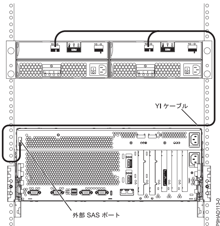
図 58. システム外部 SAS アダプター・ポートとディスク拡張ドロワー間
