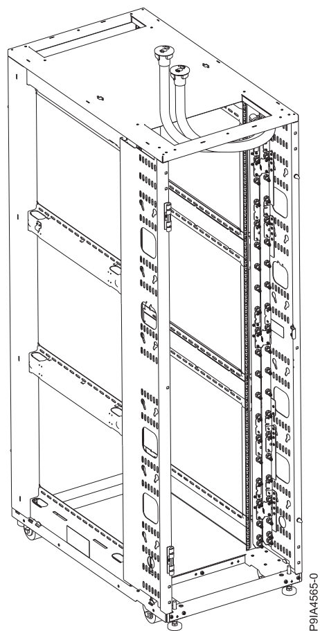
図 17. ラック、および供給ホースと返送ホースがラックの上部から出る連結管
