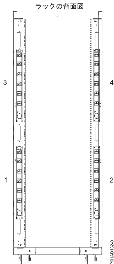
図 42. 電力配分装置の縦の位置
