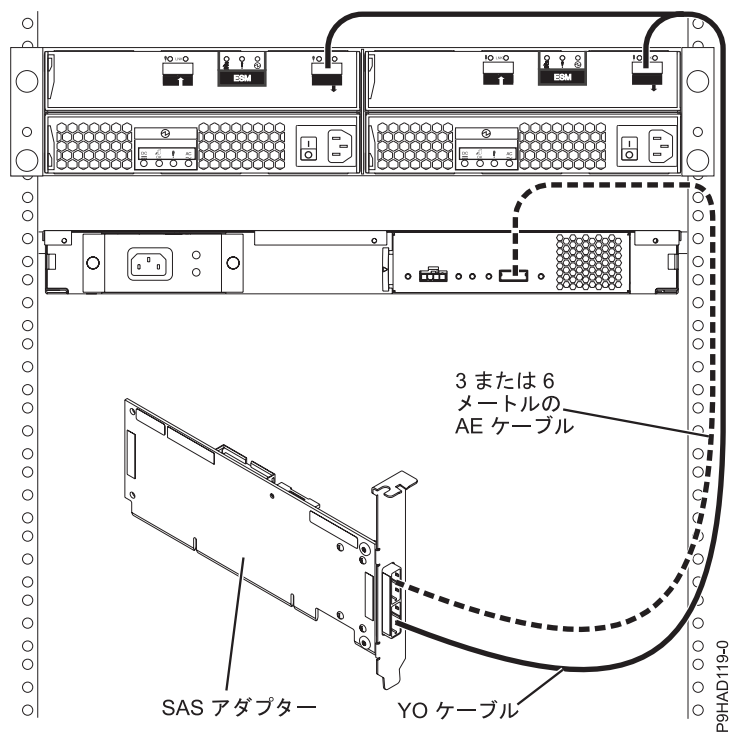
図 57. ディスク拡張ドロワーとメディア拡張ドロワーの両方と SAS アダプター間
