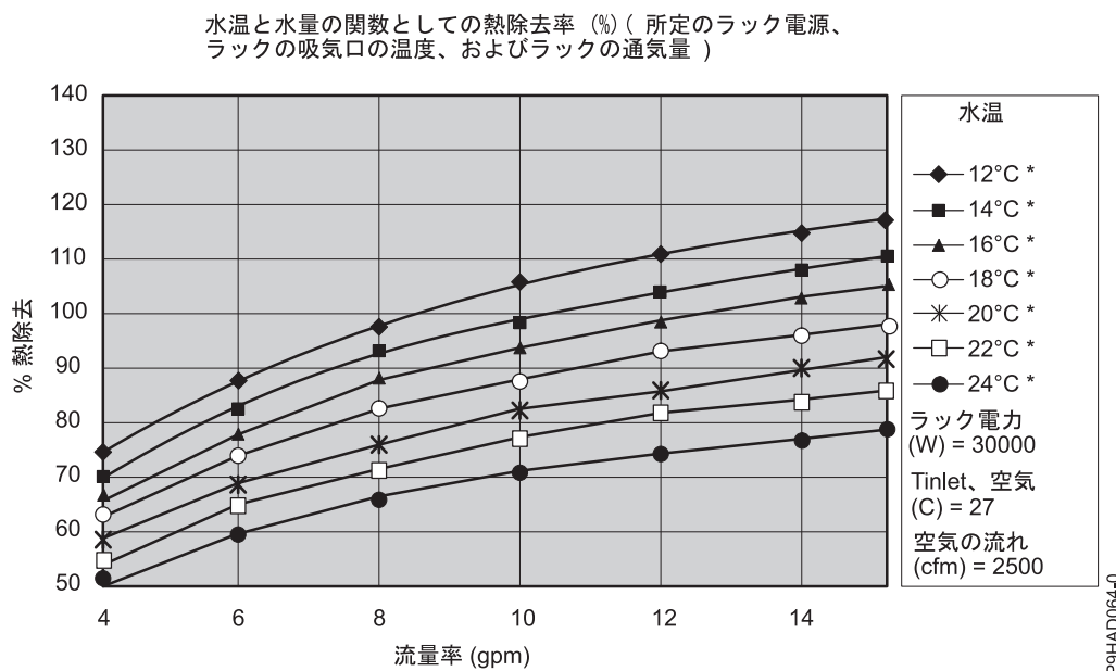
図 16. 熱負荷 30 kW のヒート・エクスチェンジャーの標準的な効率
