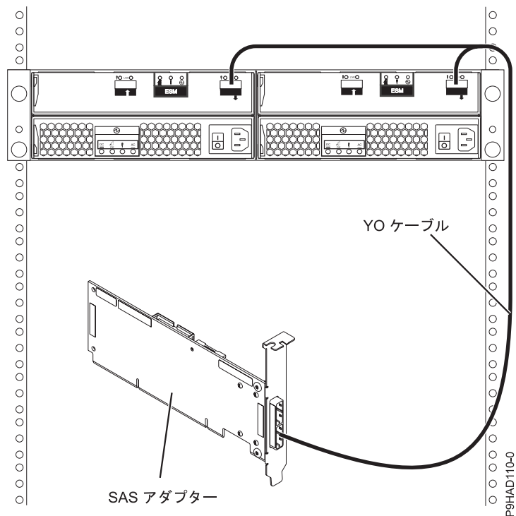
図 52. SAS アダプターとディスク拡張ドロワー間
