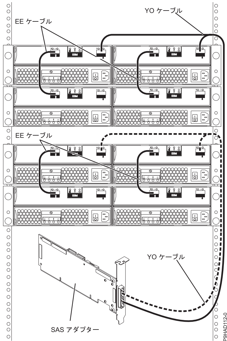
図 54. SAS アダプターと 4 つのディスク拡張ドロワー間
