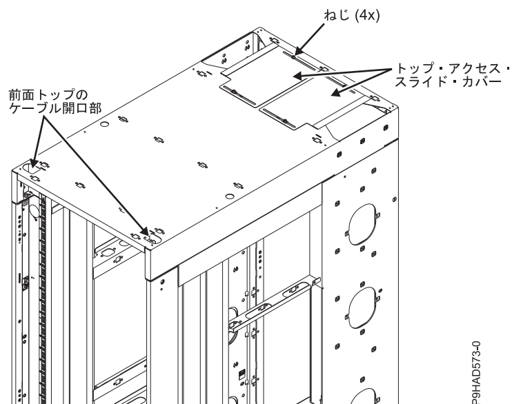
図 28. 上部でのケーブル接続
