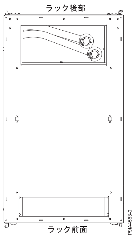
図 20. 上部ホース出口の位置 (上から見た場合)
