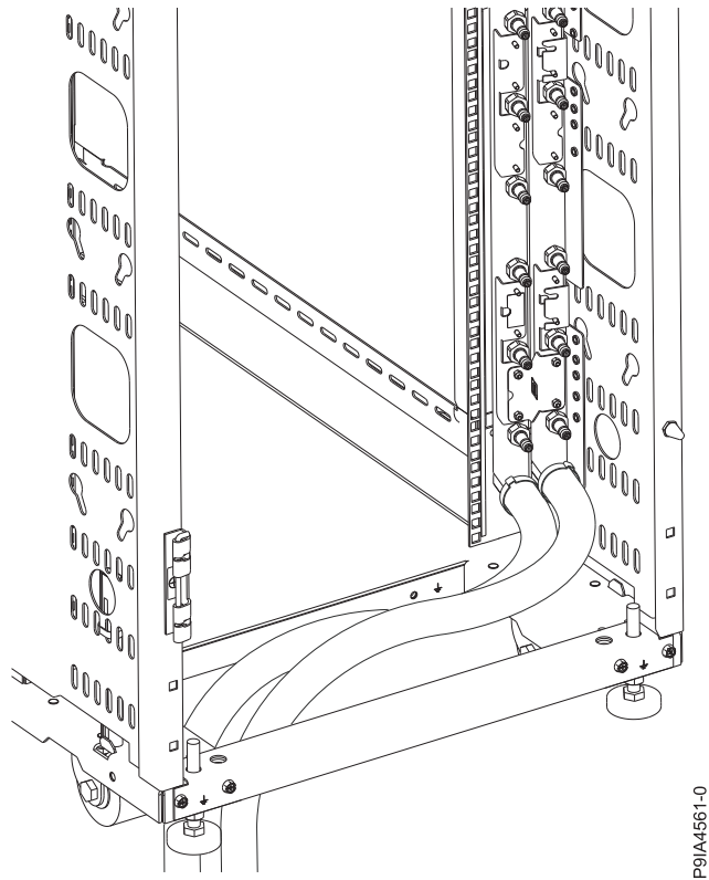
図 21. 下部ホース出口の位置
