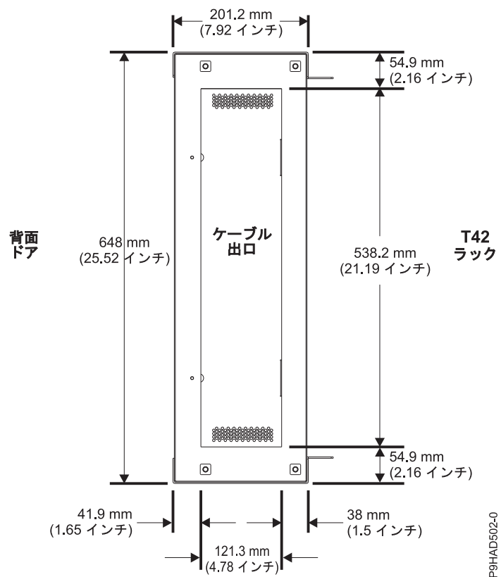
図 7. FC ERGO 背面ラック・エクステンダー (上から見た図)
