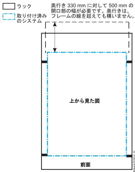
図 41. 取り付けフランジの限界寸法
