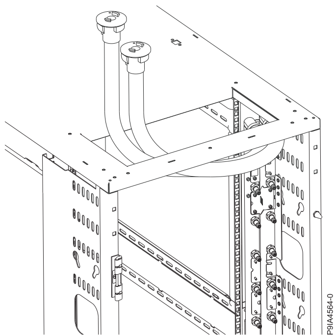
図 19. 上部ホース出口の位置
