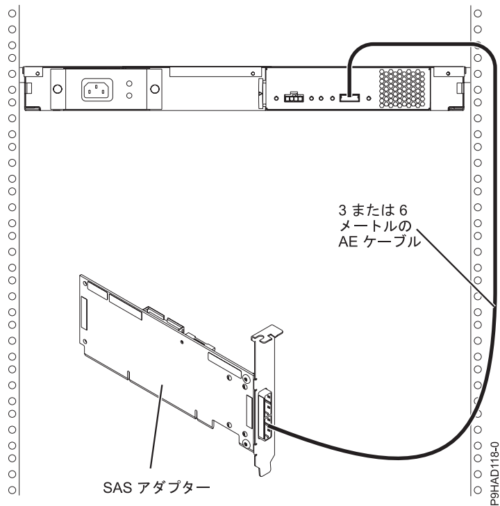
図 56. SAS アダプターとメディア拡張ドロワー間
