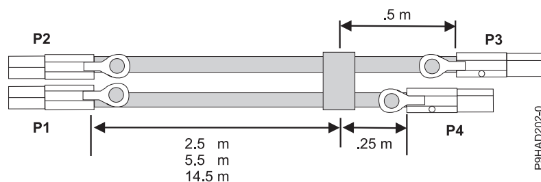
図 50. SAS 外付け YO ケーブル・アセンブリのケーブルの長さ
