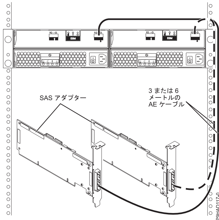
図 69. 2 つの RAID SAS アダプターと 1 つのディスク拡張ドロワー間 (マルチ・イニシエーター HA JBOD 構成)
