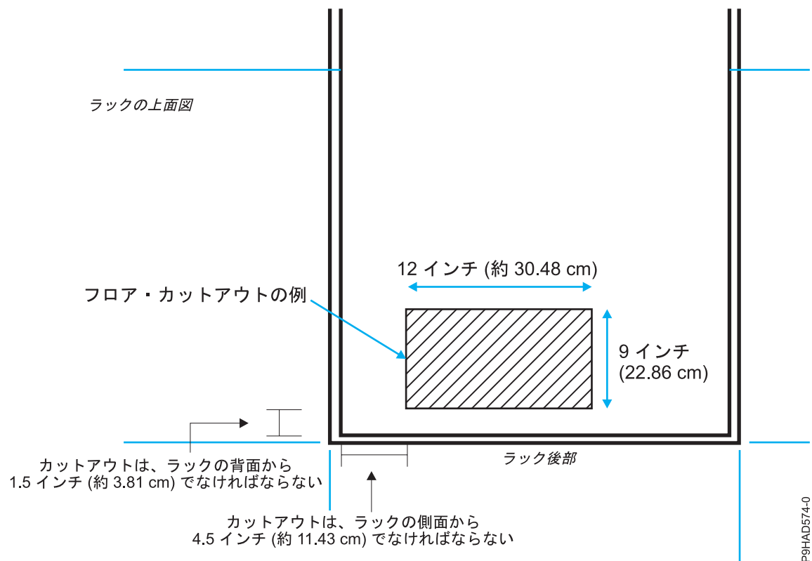
図 25. フロア・カットアウト
