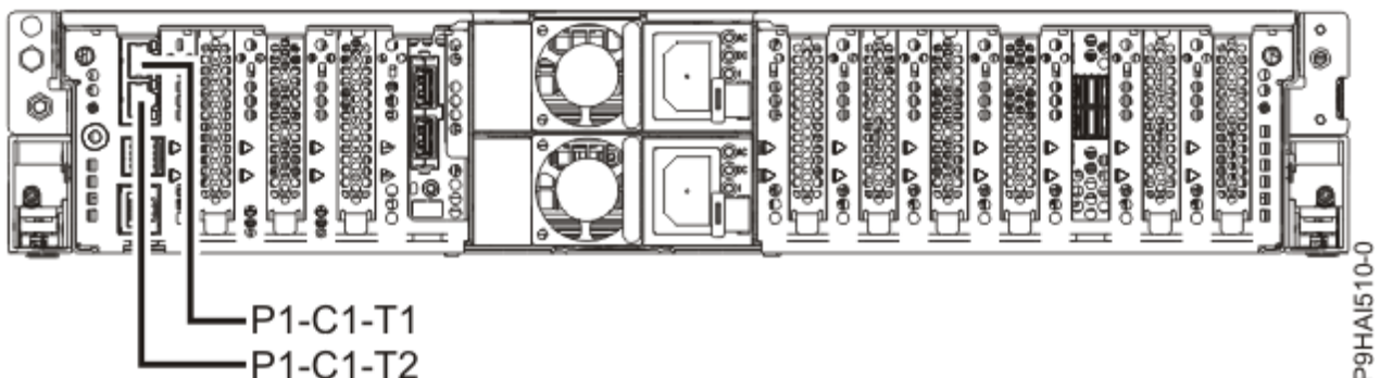
10. ábra: 5105-22E, 9008-22L, 9009-22A, 9009-22G, 9223-22H és 9223-22S HMC porthelyek
