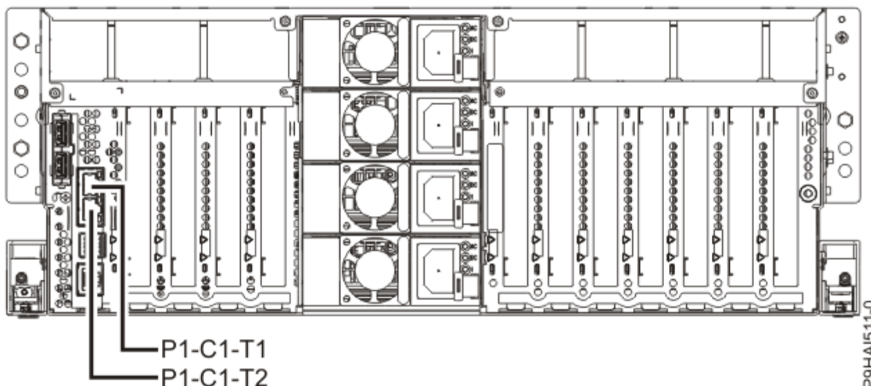
11. ábra: 9009-41A, 9009-41G, 9009-42A, 9009-42G, 9223-42H és 9223-42S HMC porthelyek
