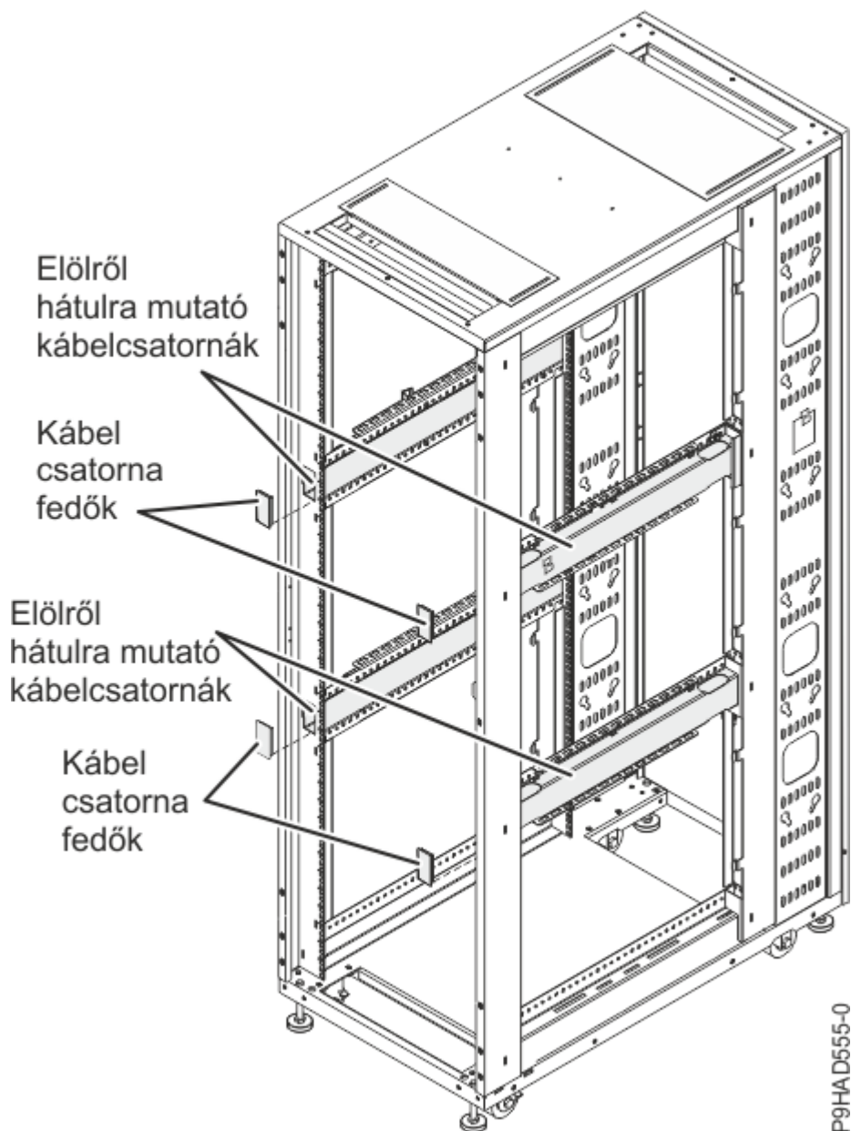
8. ábra: Kábelezés a rack szekrényen belül
