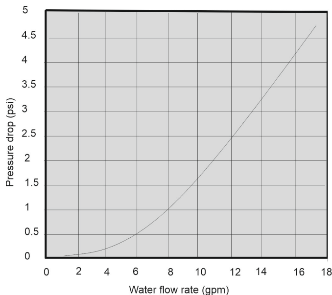
24. ábra: Nyomásesés (szabványos mértékegységek)
