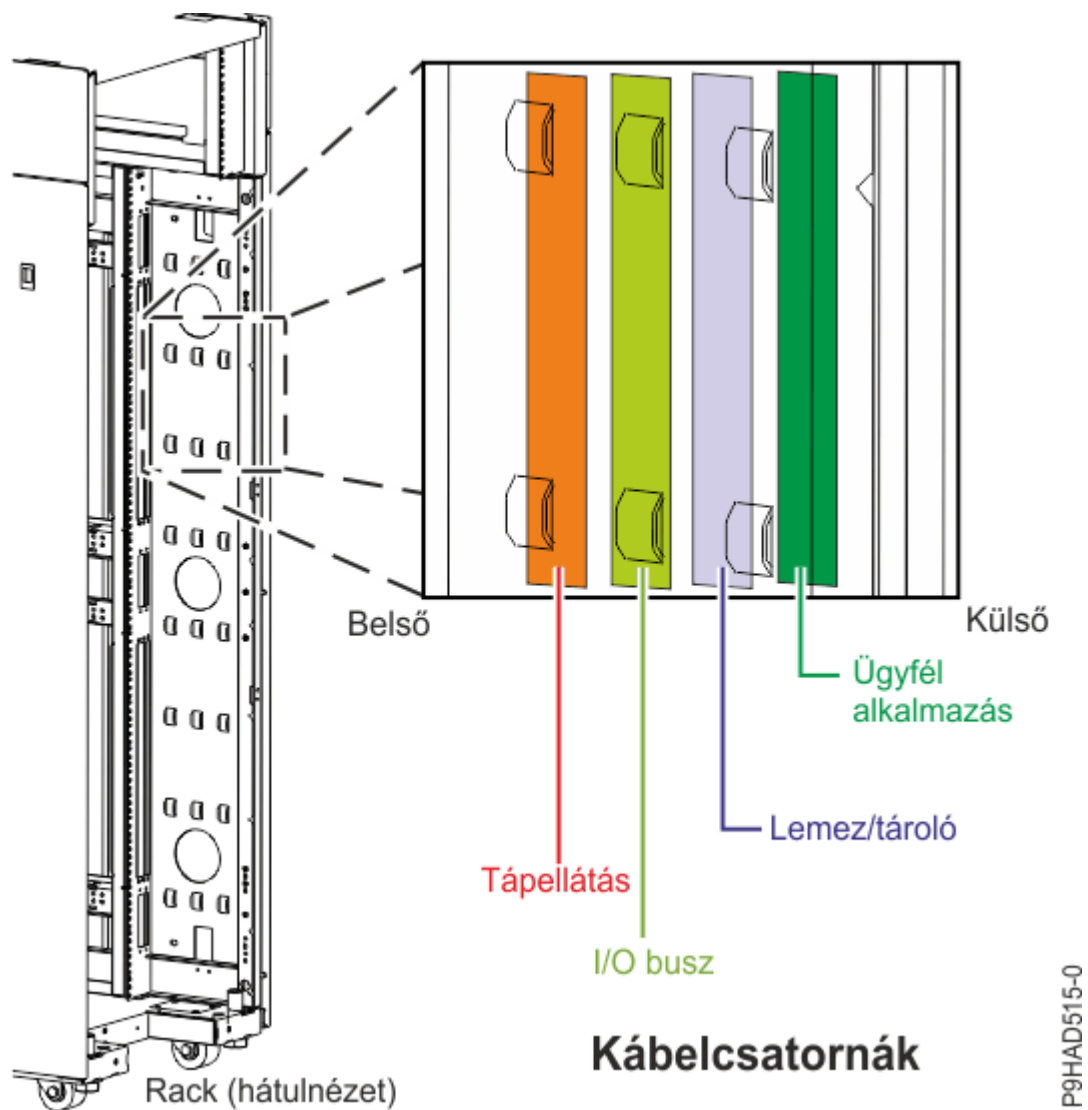
43. ábra: Kábelrendező hídkezelő
