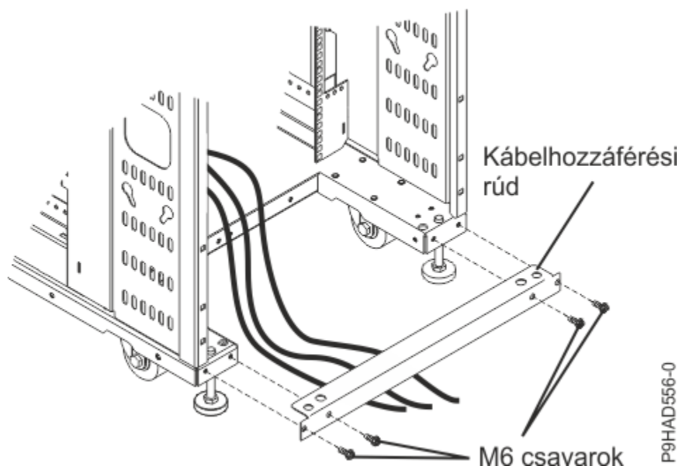
9. ábra: Kábelhozzáférési-rúd
