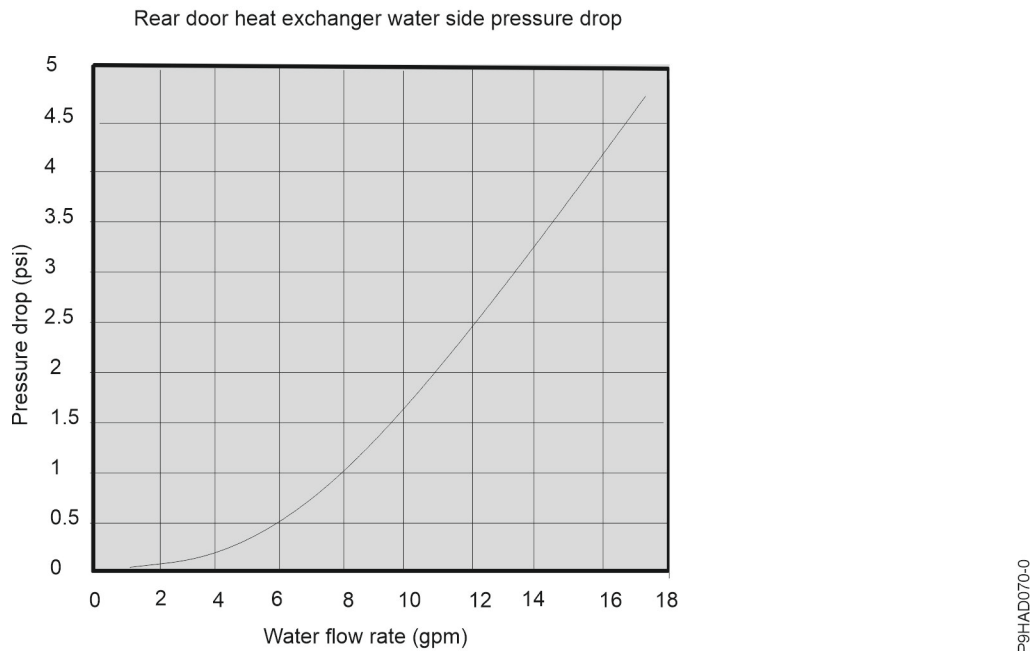
24. ábra: Nyomásesés (szabványos mértékegységek)
