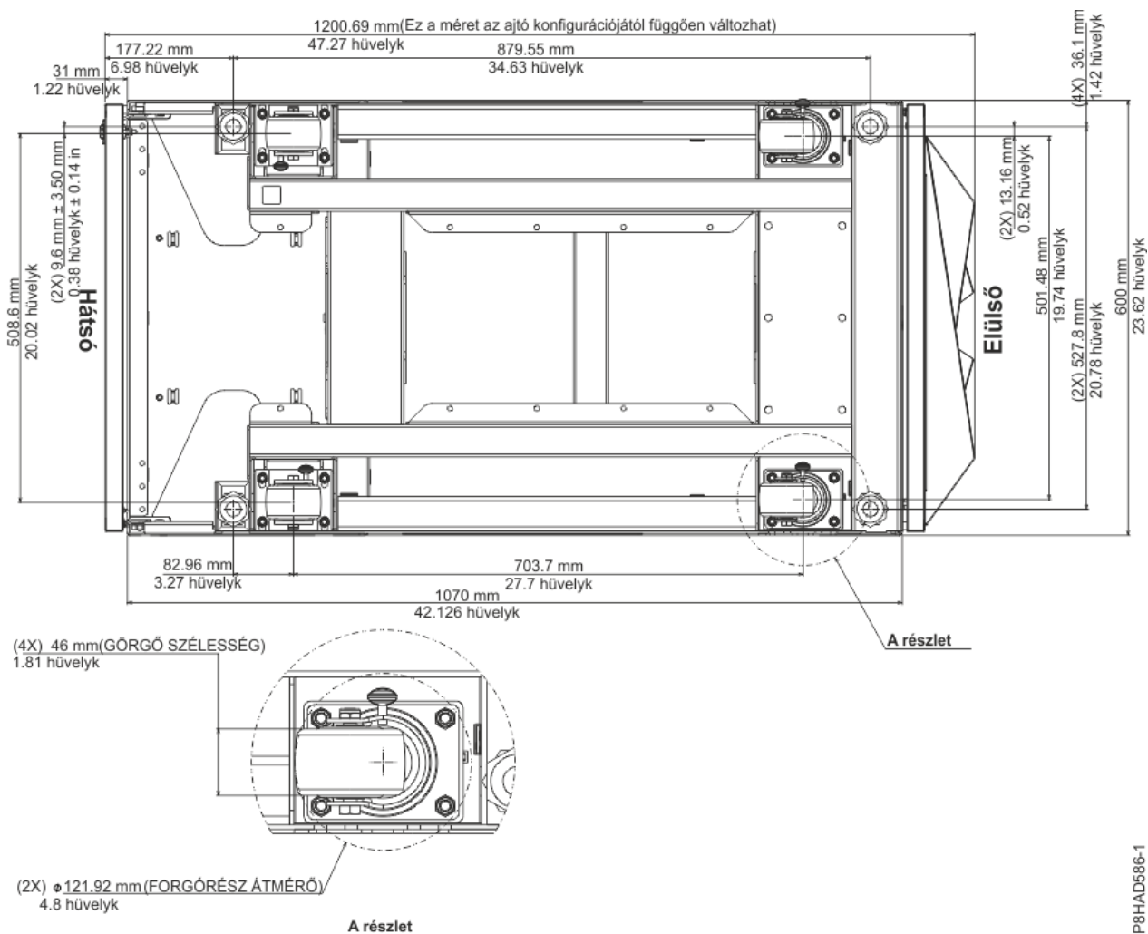
14. ábra: Görgők és kiegyenlítő helye
