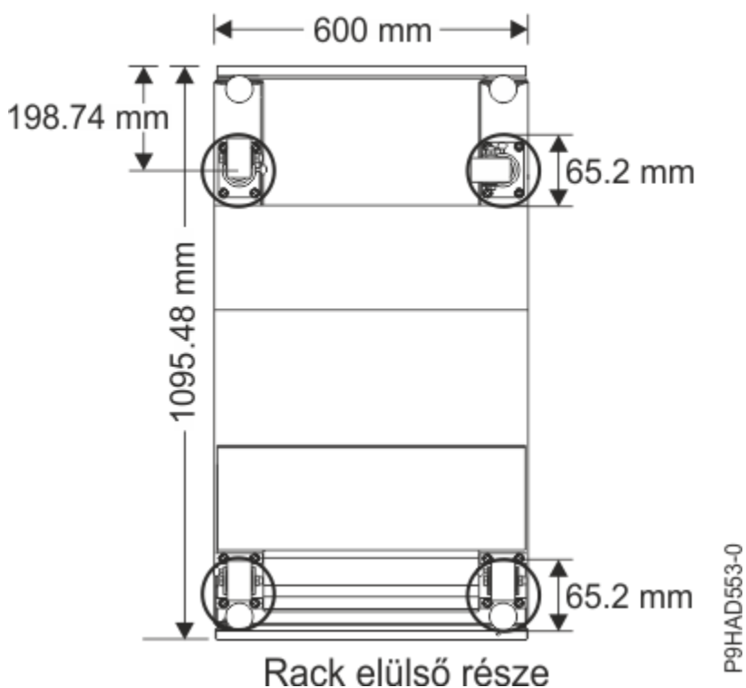
7. ábra: Görgőhelyek
