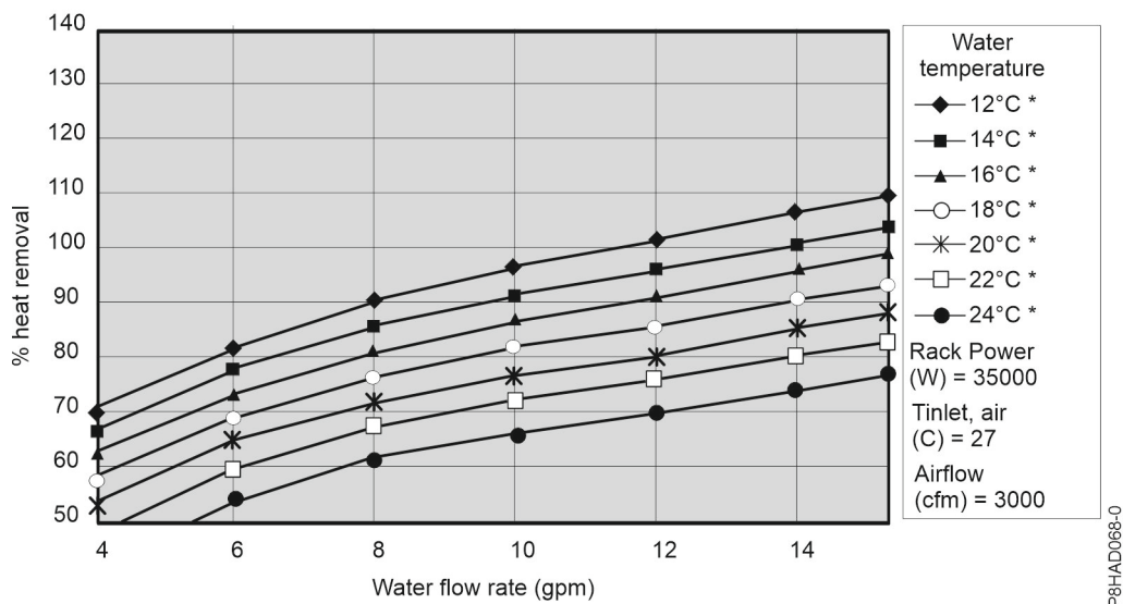
22. ábra: A hőcserélő tipikus teljesítménye, 35 kW hőterhelés
