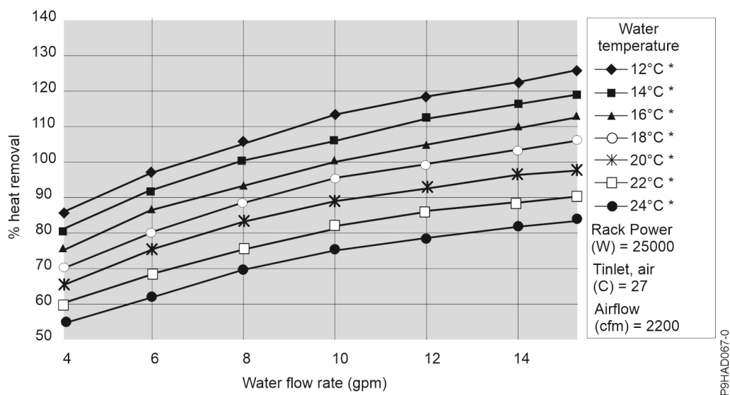
20. ábra: A hőcserélő tipikus teljesítménye, 25 kW hőterhelés
