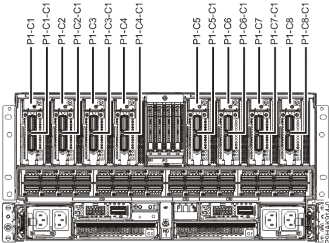
1. ábra: Rackbe szerelt 9080-M9S rendszer hátulnézete PCIe bővítőhelyek elhelyezési kódjaival
