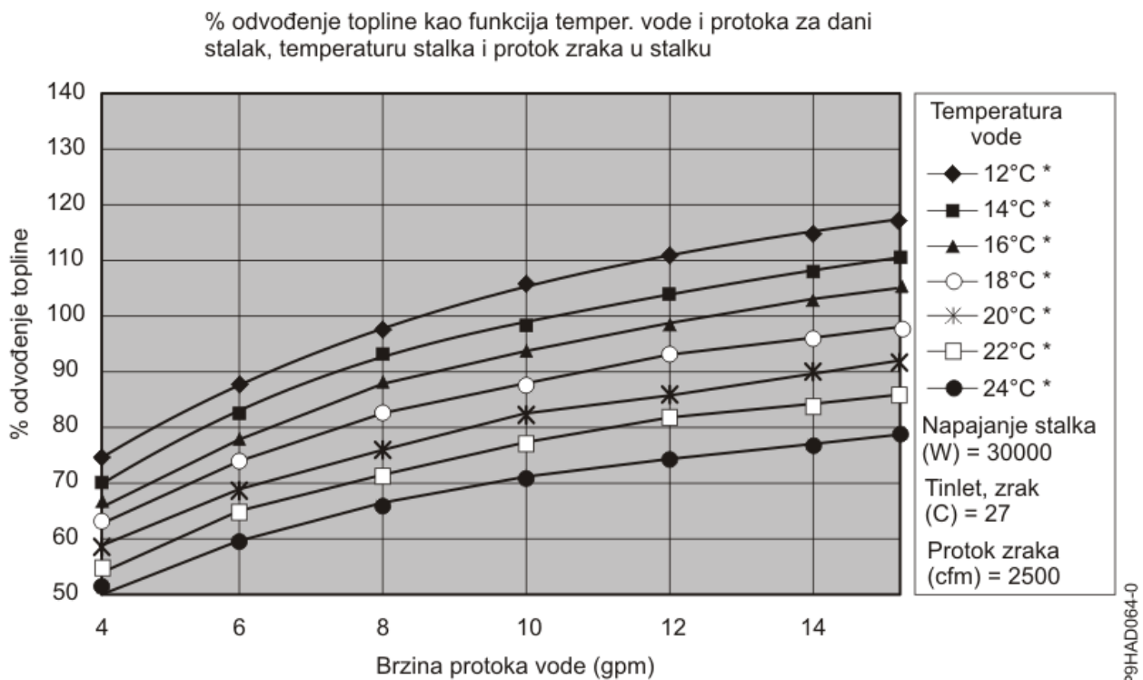
Slika 29. Tipične performanse izmjenjivača topline, 30 kW opterećenje toplotom
