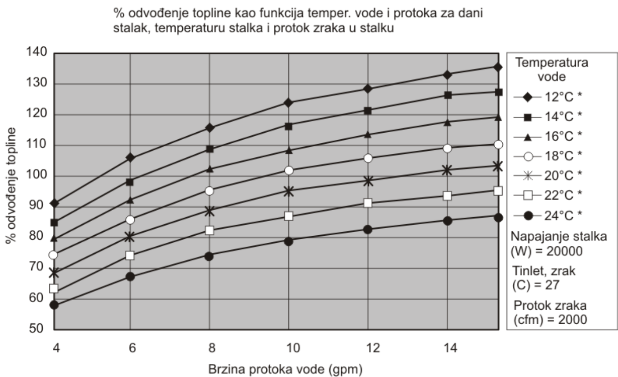
Slika 13. Tipične performanse izmjenjivača topline, 20 kW opterećenje toplotinom
