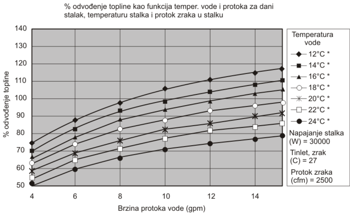
Slika 14. Tipične performanse izmjenjivača topline, 30 kW opterećenje toplotinom
