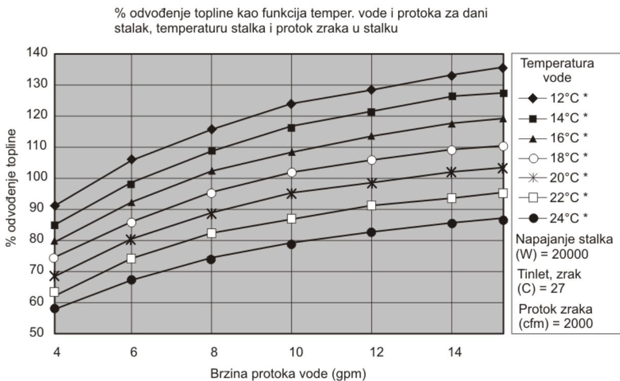
Slika 28. Tipične performanse izmjenjivača topline, 20 kW opterećenje topline
