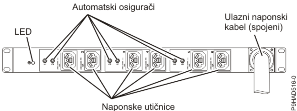
Slika 42. HVDC PDU
