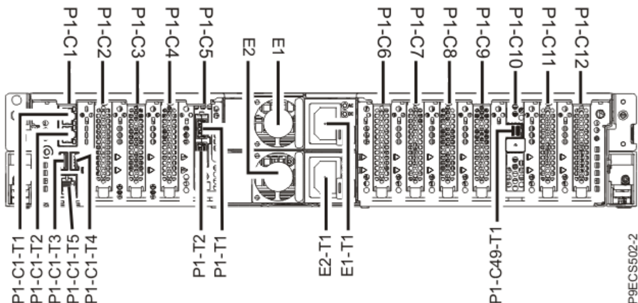
Slika 2. Pogled straga na sistem montiran u stalak 9008-22L, 9009-22A ili 9223-22H sistem s kodovima lokacija PCIe priključnica
