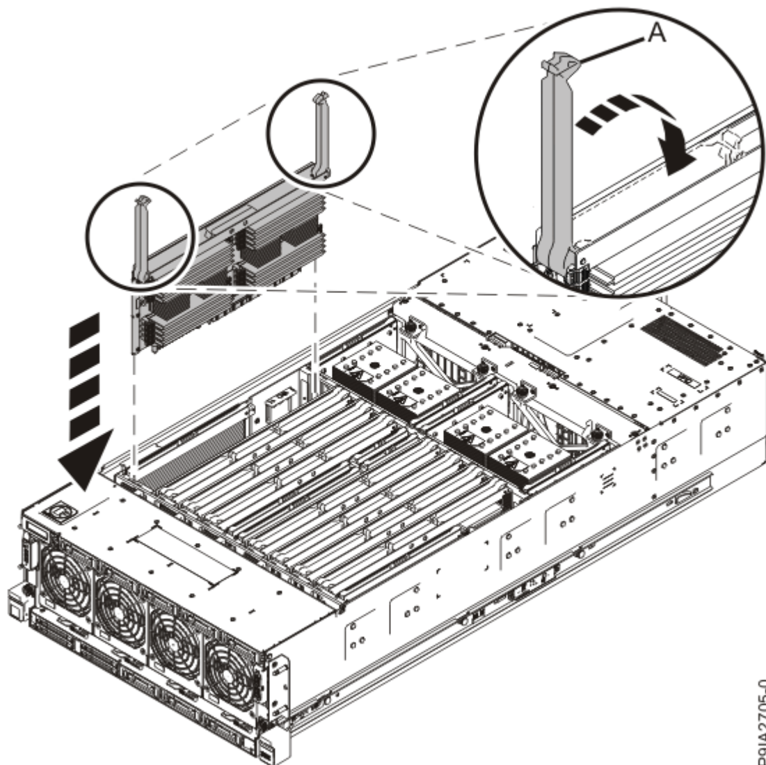
Figure 9. Remise en place de la carte de bus mémoire à l'emplacement P1-C26
