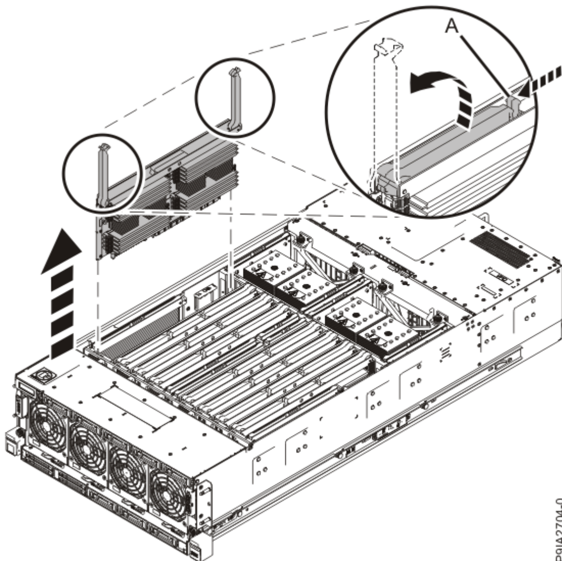
Figure 6. Retrait de la carte de bus mémoire de l'emplacement P1-C26
