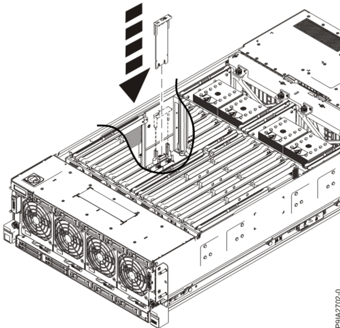
Figure 8. Remise en place de la carte TPM
