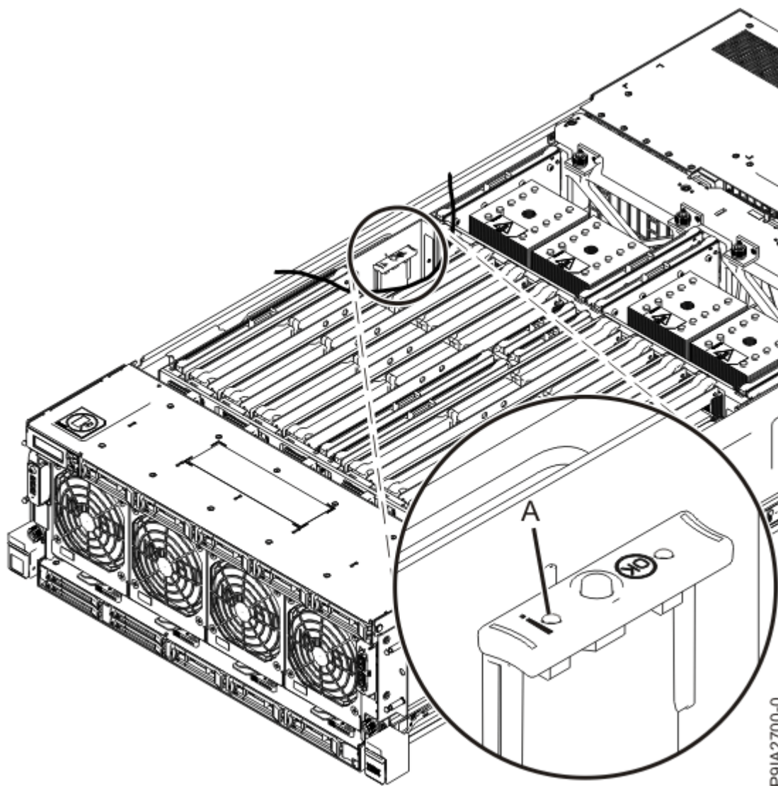
Figure 5. Emplacement du voyant d'activité de la carte TPM
