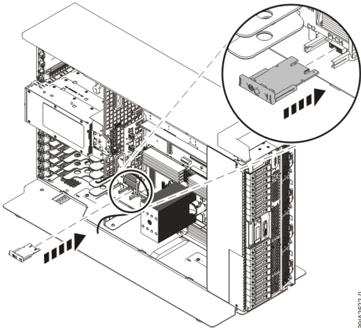
Figure 13. Remplacement de la carte TPM dans un système autonome
