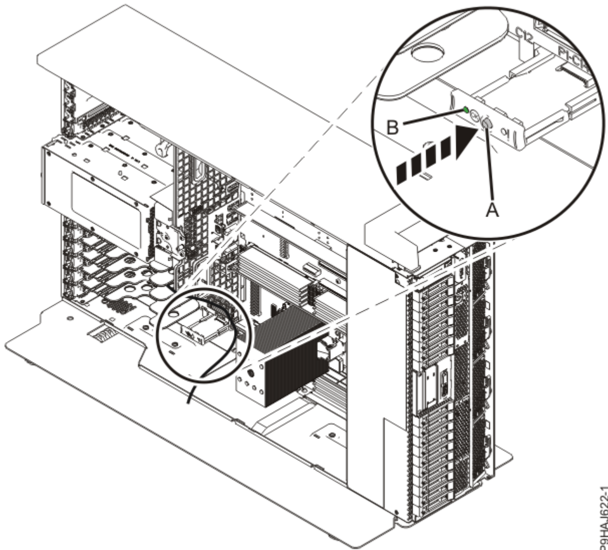
Figure 7. Activation du voyant d'identification d'un système autonome
