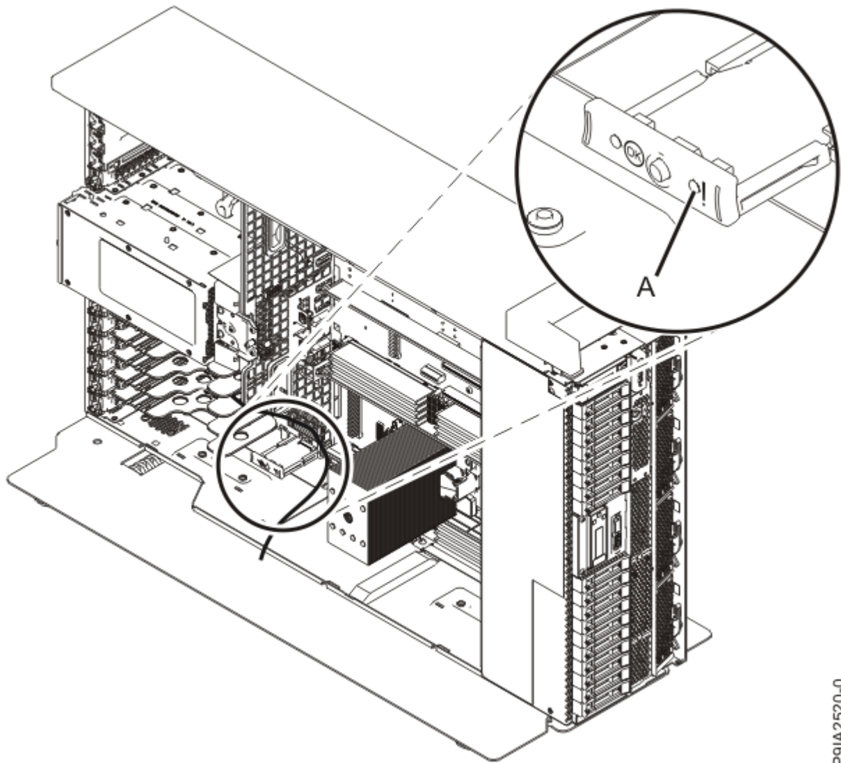
Figure 9. Emplacement du voyant d'activité de la carte TPM sur un serveur autonome
