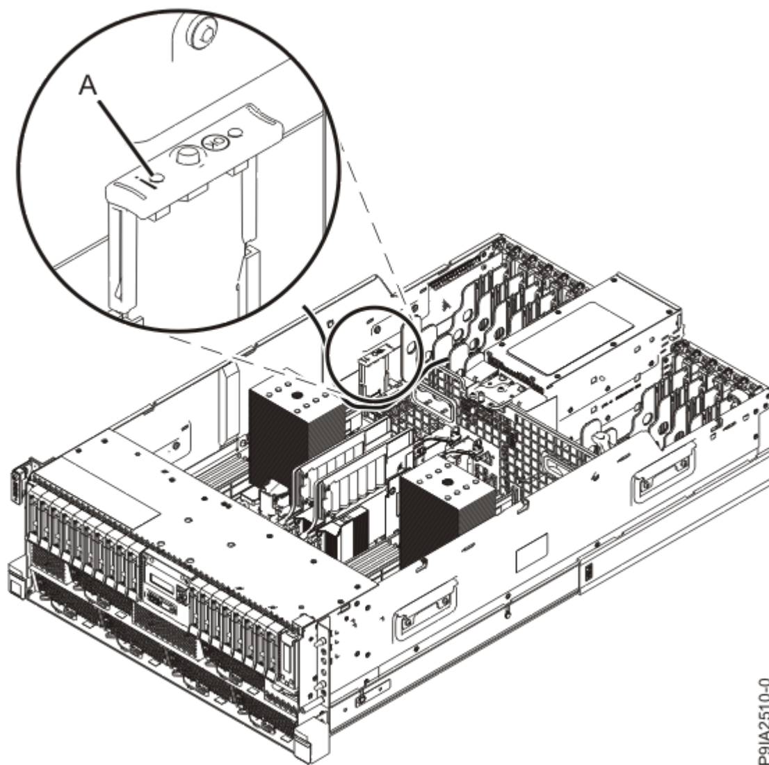
Figure 8. Emplacement du voyant d'activité de la carte TPM sur un serveur monté en armoire
