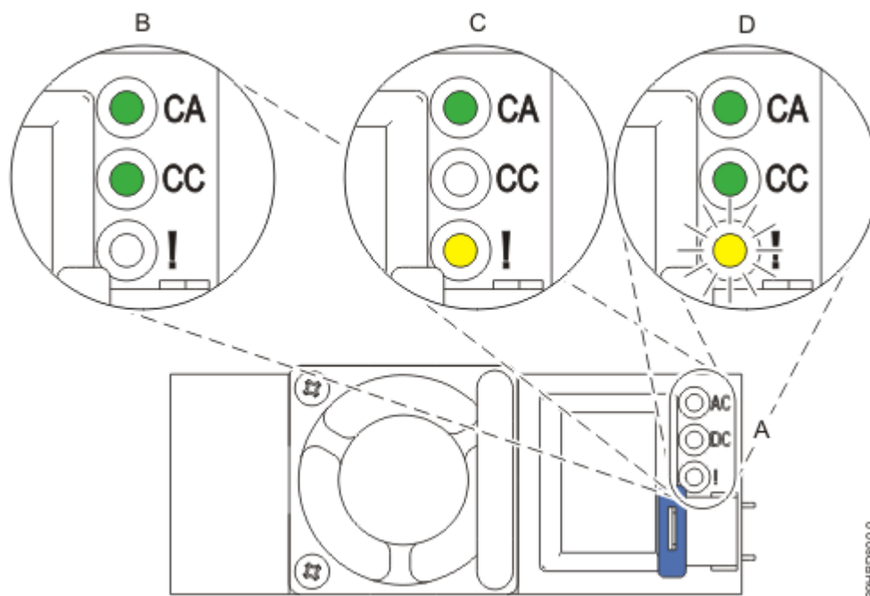
Figure 2. Voyants d'une alimentation fonctionnelle (B) et d'une alimentation défectueuse (C, D) dans un système monté en armoire
