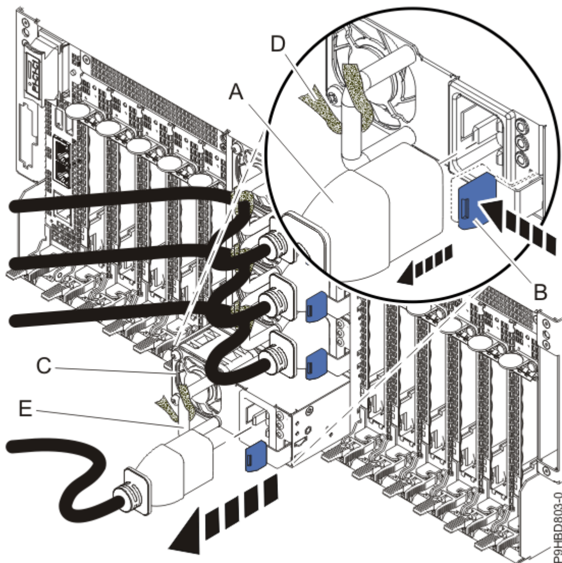
Figure 4. Retrait d'une alimentation
