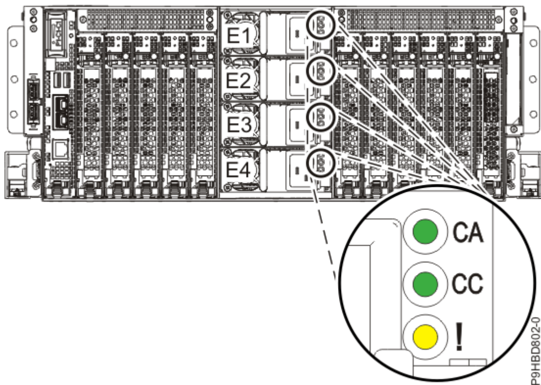
Figure 1. Emplacement des alimentations et des voyants
