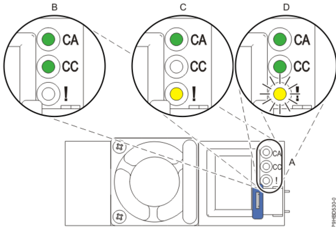
Figure 2. Voyants d'une alimentation fonctionnelle (B) et d'une alimentation défectueuse (C, D)
