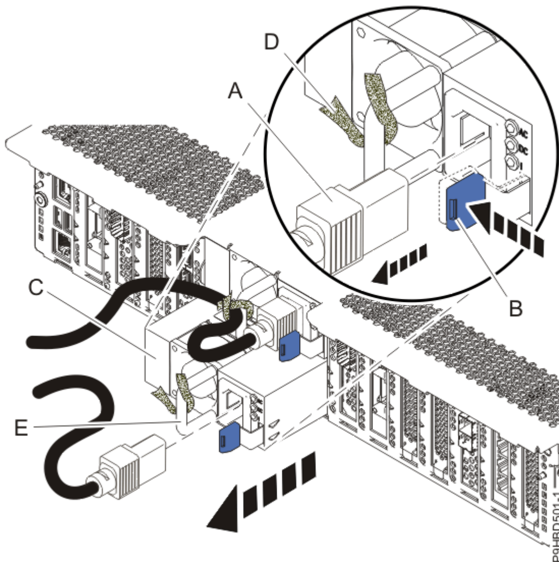
Figure 5. Retrait d'une alimentation
