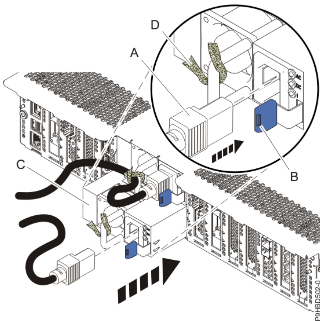
Figure 6. Remise en place d'une alimentation
