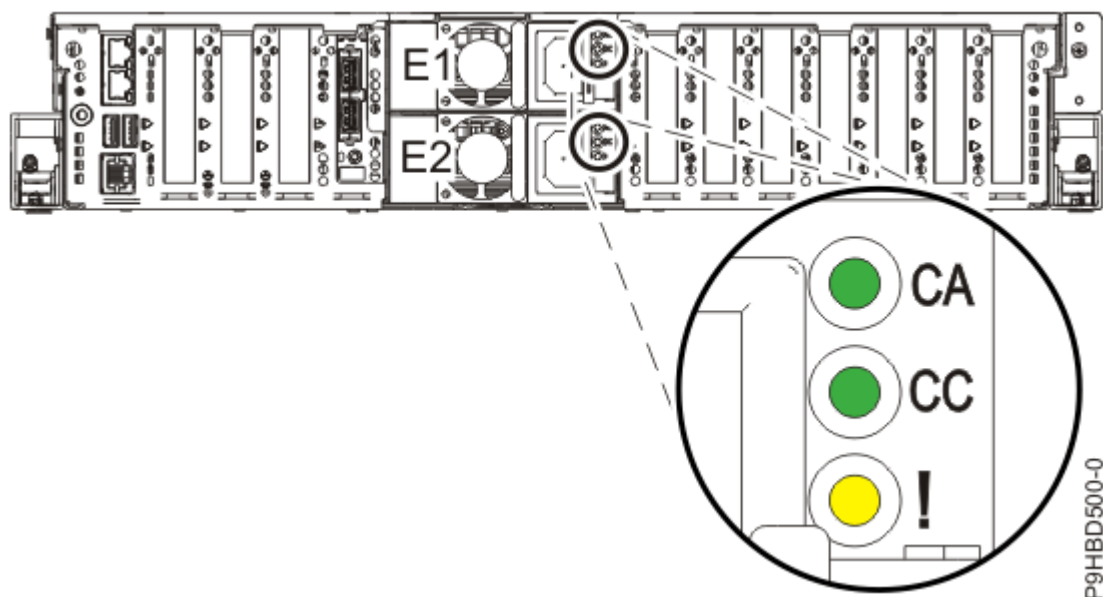
Figure 1. Emplacement des alimentations et des voyants dans le système
