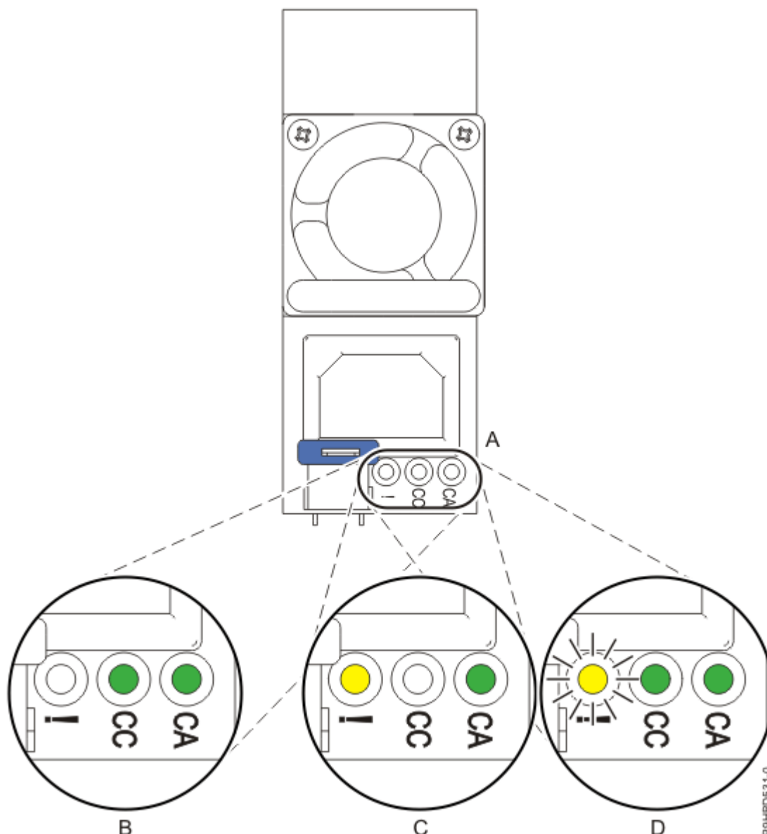
Figure 4. Voyants d'une alimentation fonctionnelle ( B ) et d'une alimentation défectueuse ( C, D ) dans un système autonome
