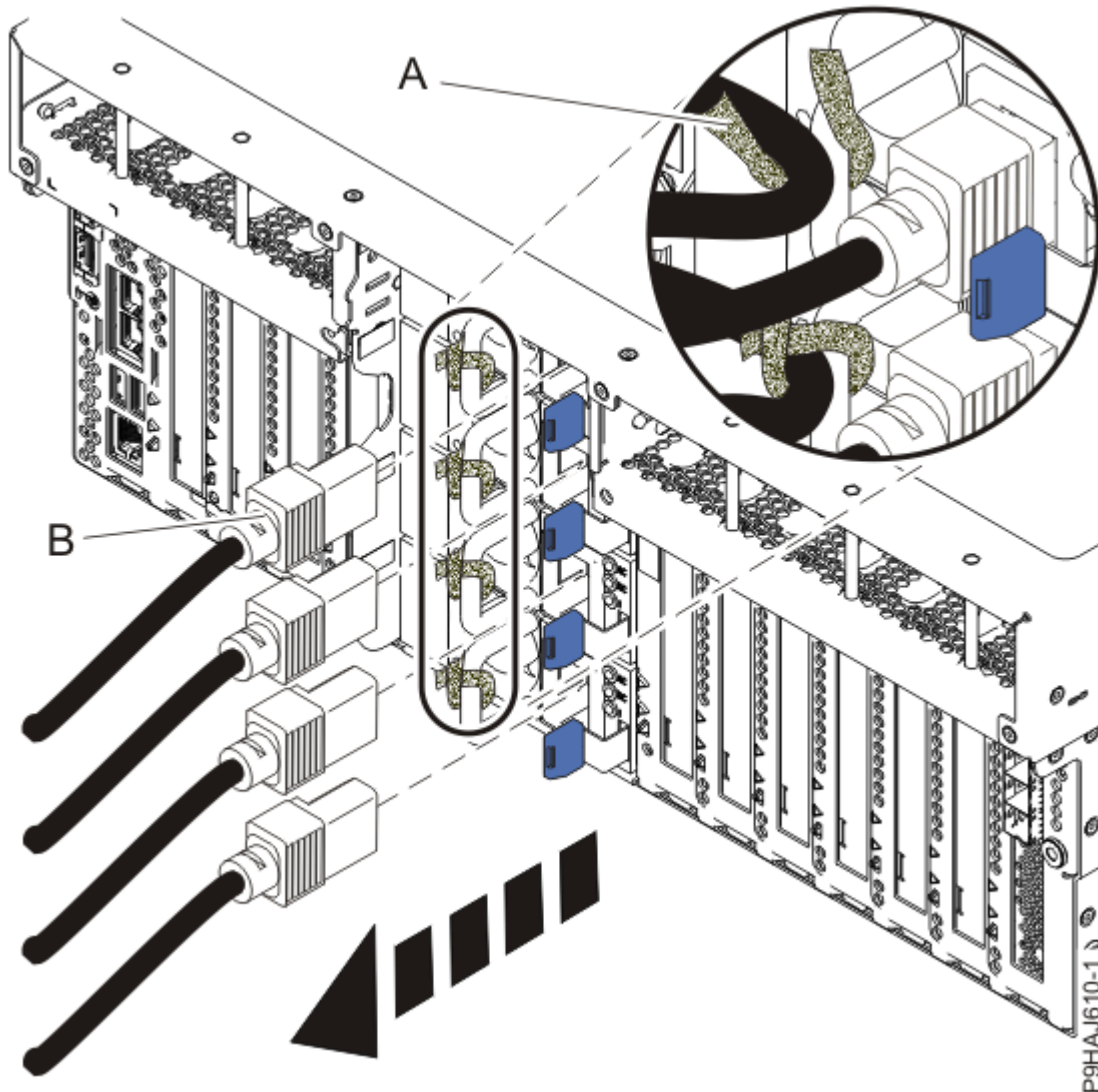
Figure 5. Retrait des cordons d'alimentation d'un serveur monté en armoire
