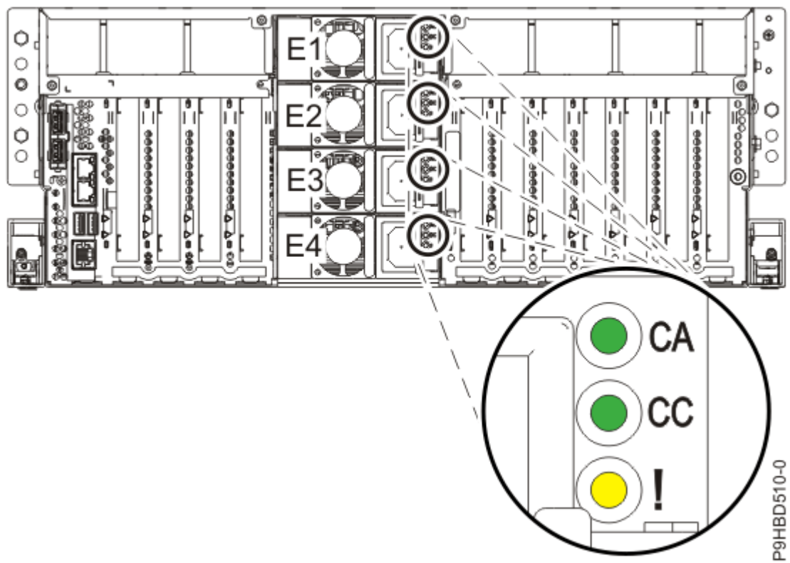
Figure 1. Emplacement des alimentations et des voyants dans le système monté en armoire
