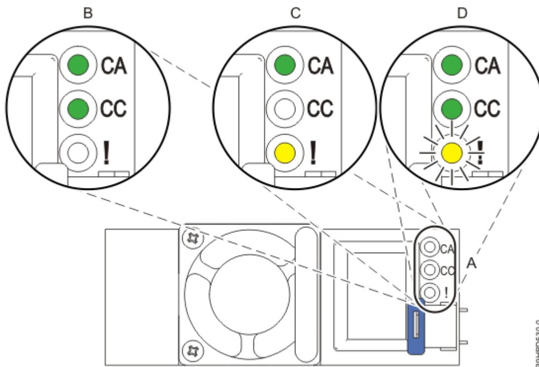
Figure 3. Voyants d'une alimentation fonctionnelle (B) et d'une alimentation défectueuse (C, D) dans un système monté en armoire
