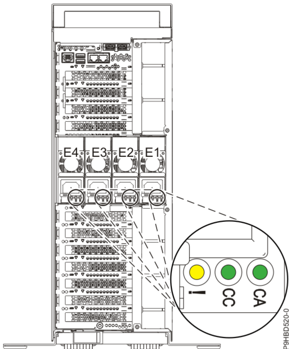
Figure 2. Emplacement des alimentations et des voyants dans le système autonome
