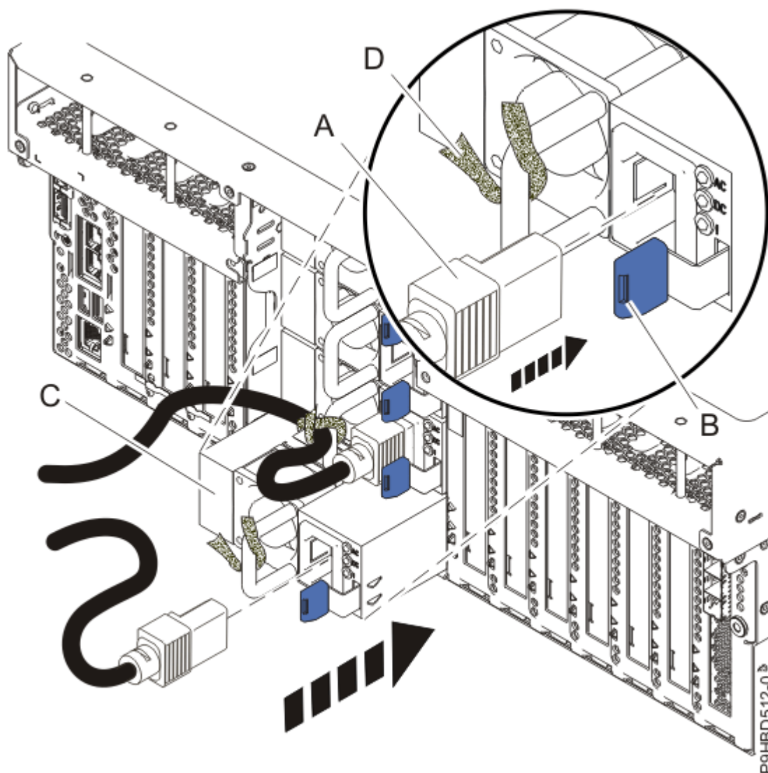
Figure 9. Remise en place d'une alimentation
