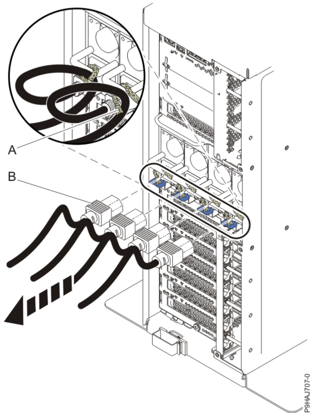
Figure 6. Retrait des cordons d'alimentation d'un serveur autonome
