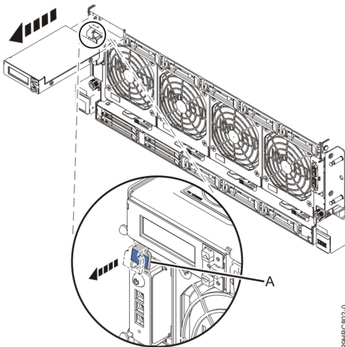
Figure 8. Retrait de l'écran du panneau de commande
