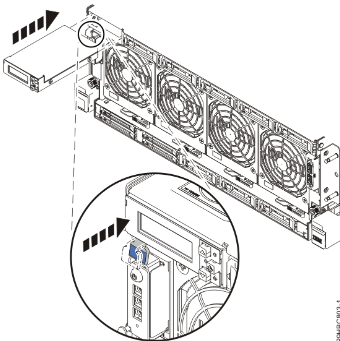
Figure 9. Remise en place de l'écran du panneau de commande
