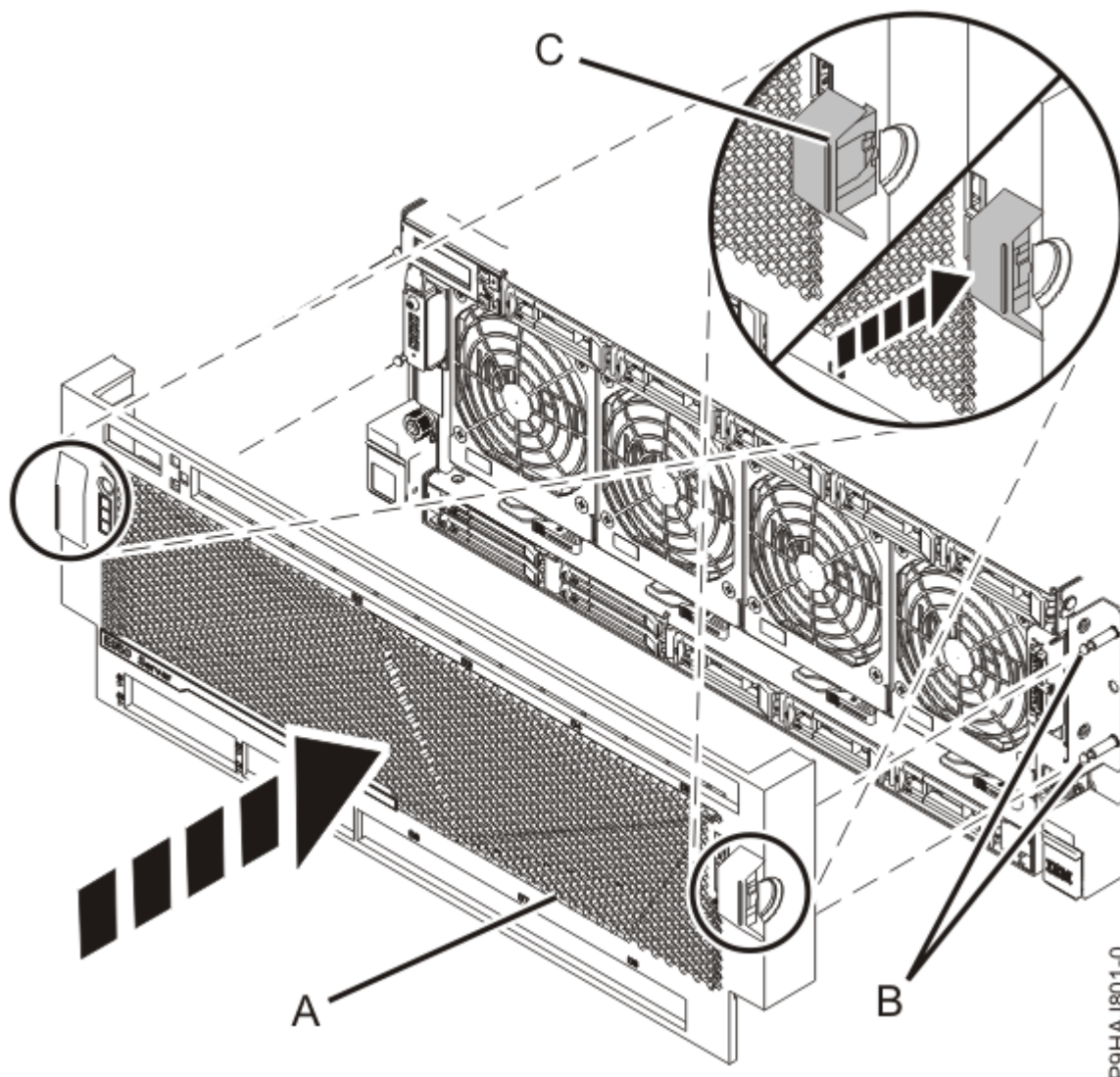
Figure 10. Installation du capot avant
