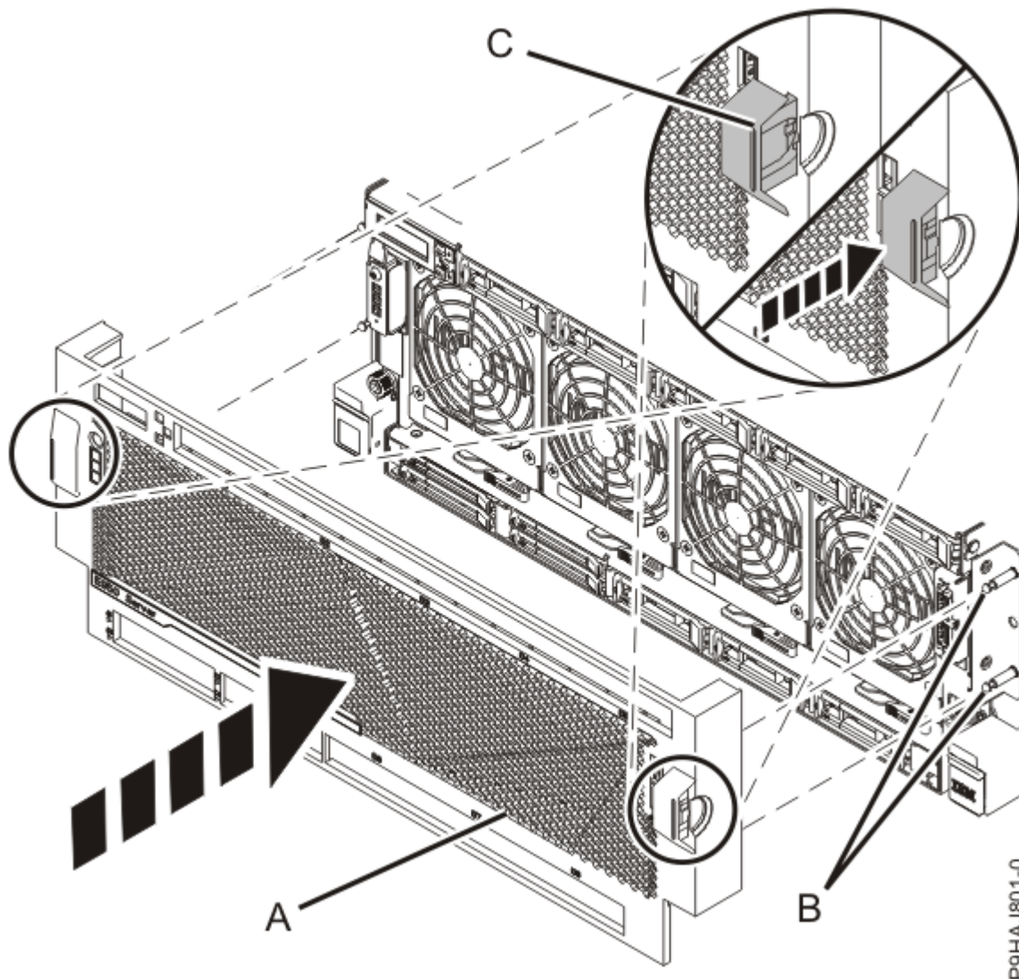
Figure 5. Installation du capot avant
