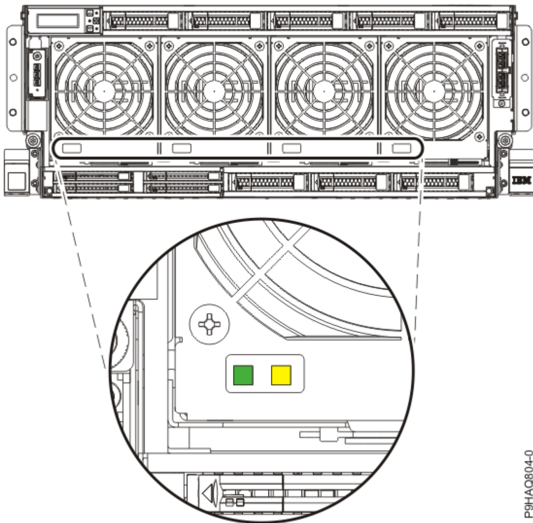
Figure 2. Voyants des ventilateurs sur le système
