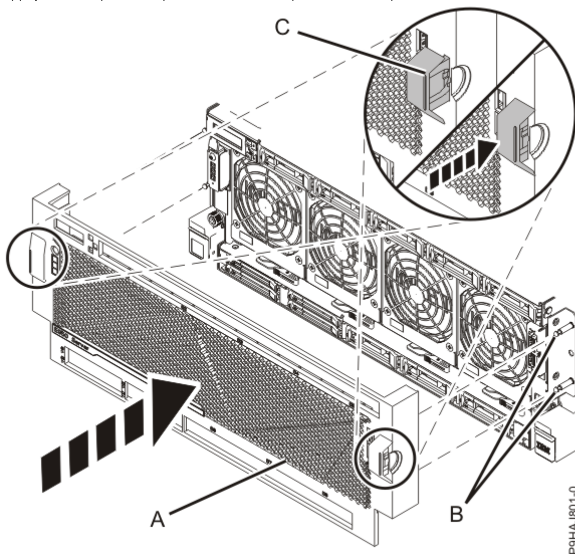
Figure 6. Installation du capot avant
