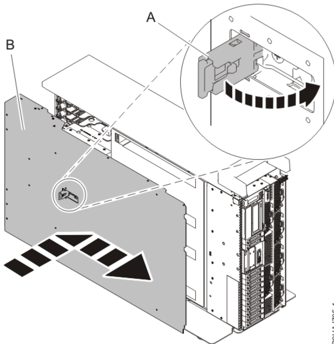
Figure 34. Installation du capot d'accès
