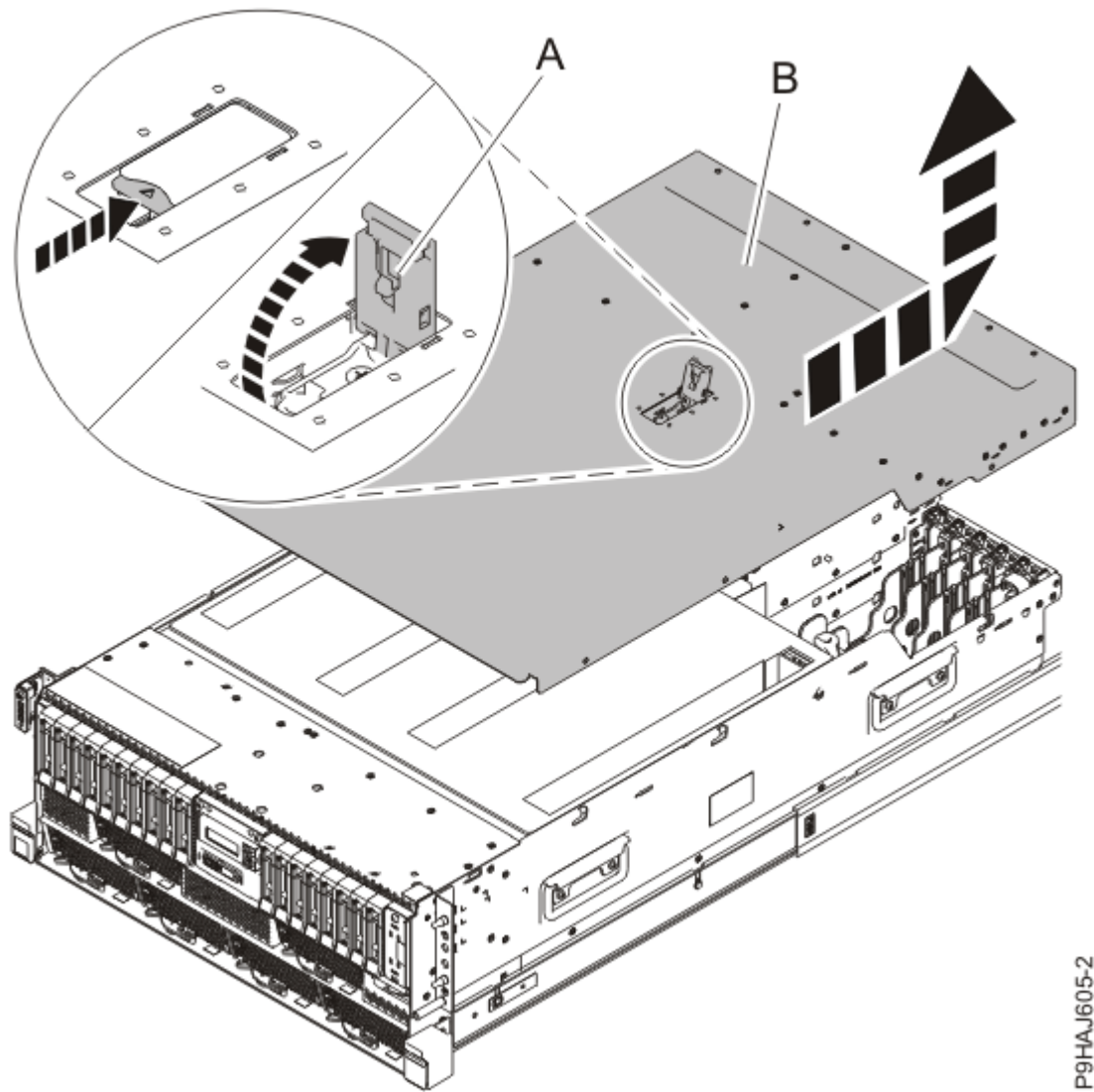
Figure 20. Retrait du capot d'accès d'un système monté en armoire
