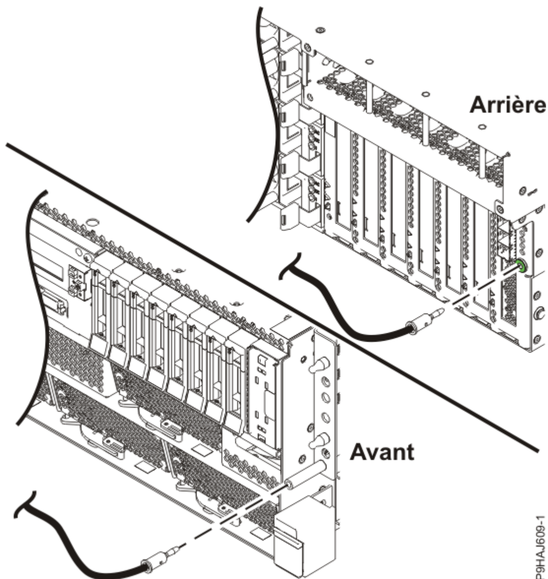
Figure 9. Emplacement des fiches de décharge électrostatique
