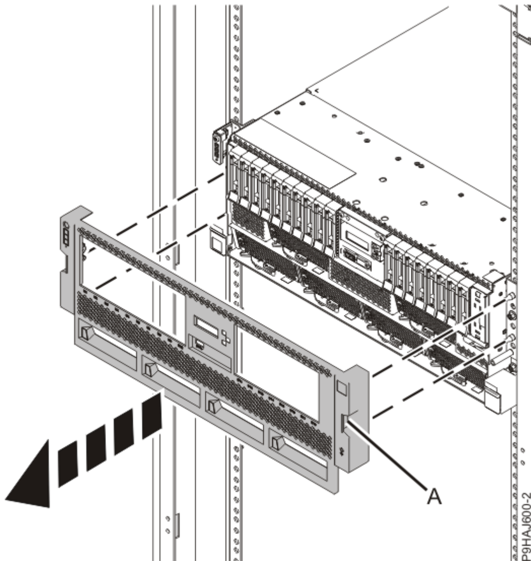
Figure 1. Retrait du capot avant
