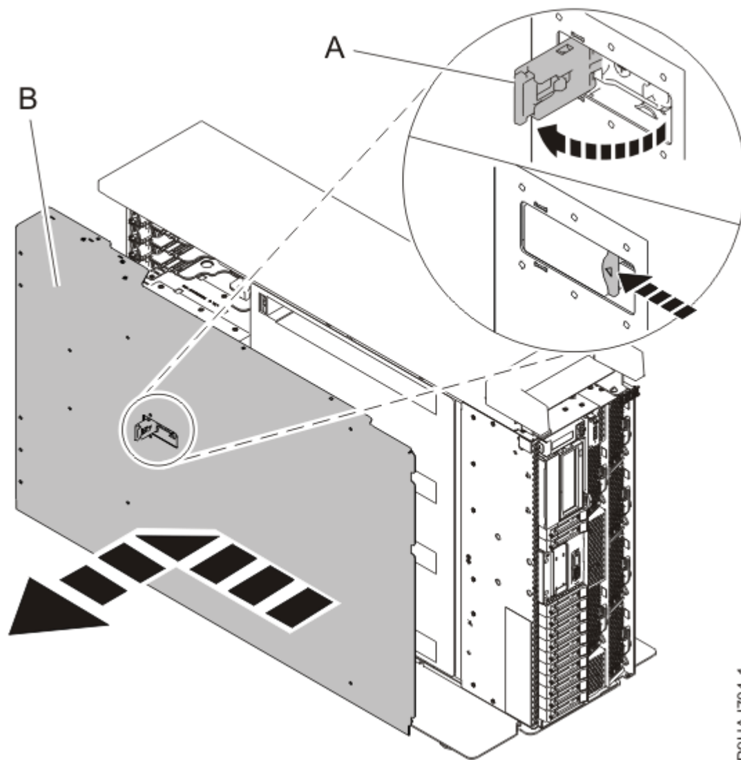
Figure 21. Retrait du capot d'accès
