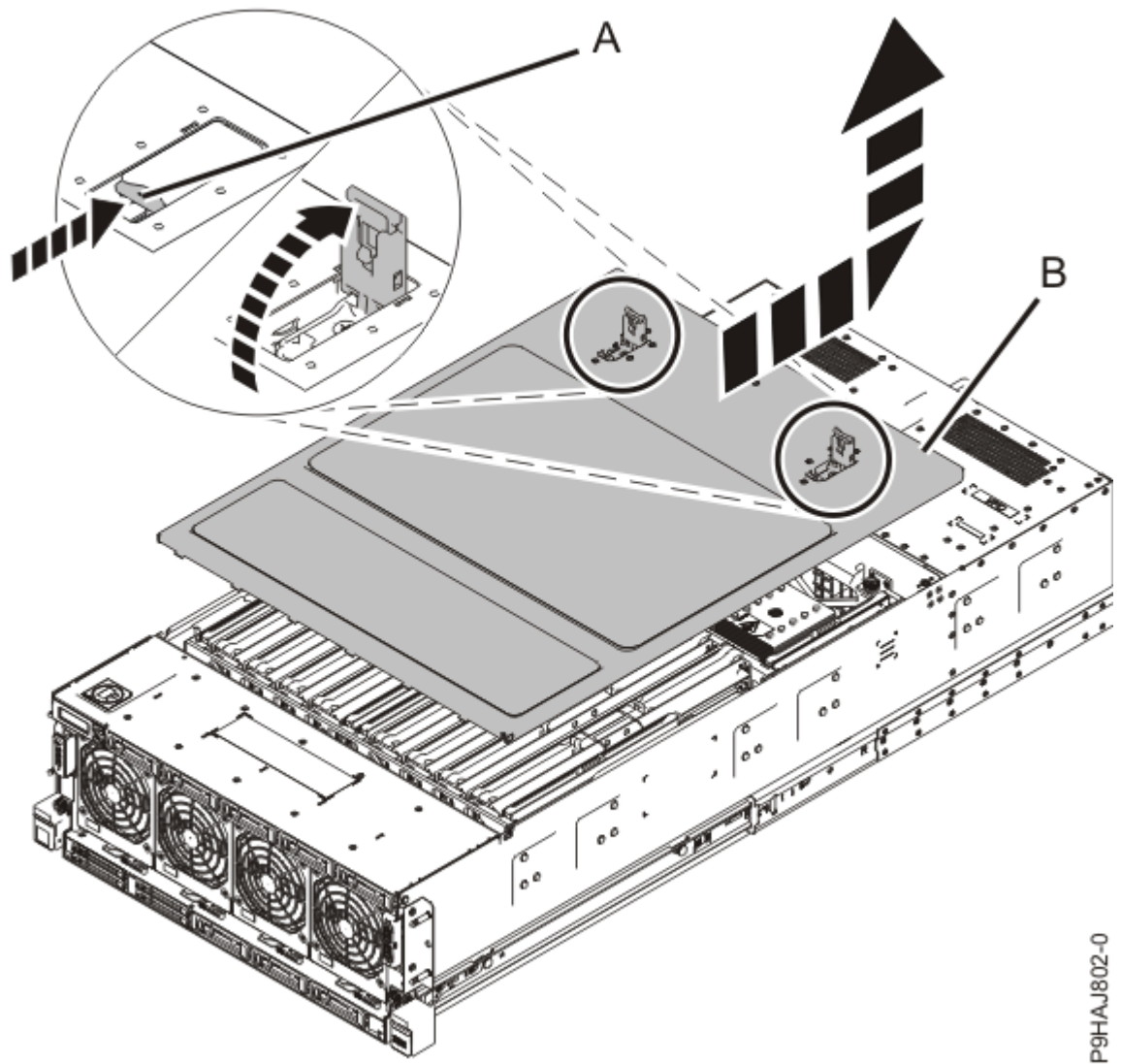
Figure 12. Retrait du capot d'accès
