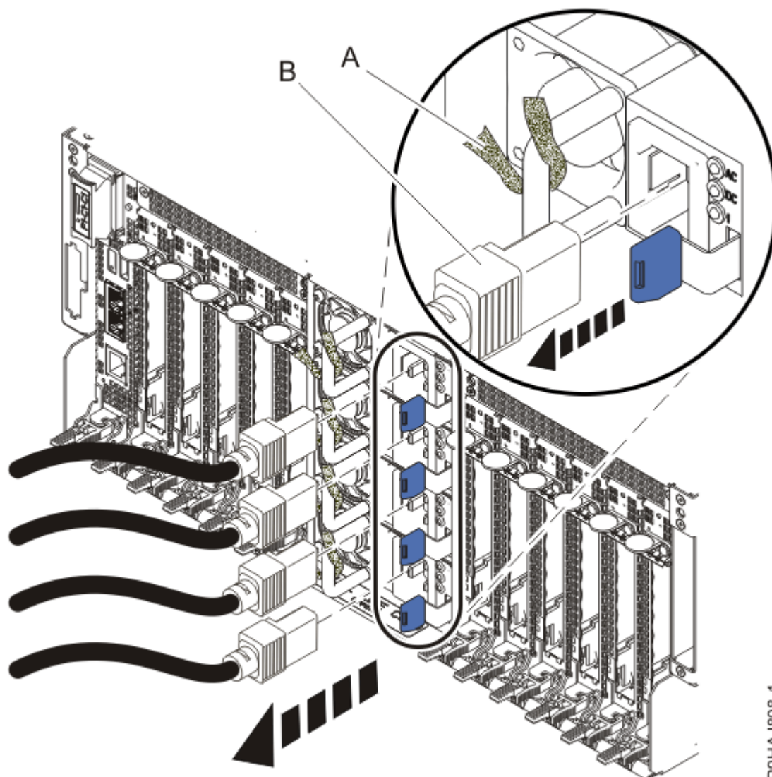
Figure 23. Retrait des cordons d'alimentation
