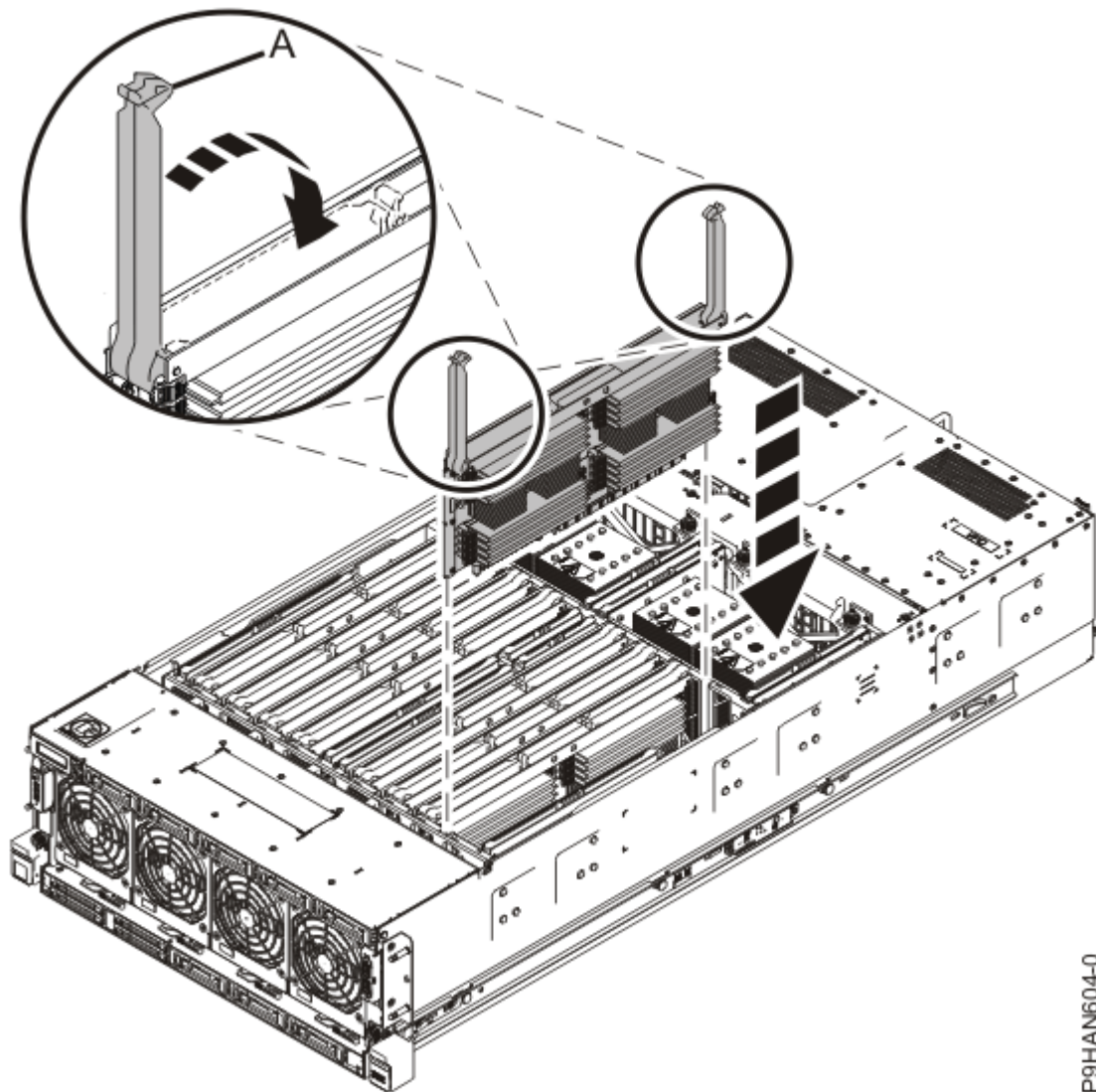
Figure 19. Insertion d'une carte d'extension de mémoire
