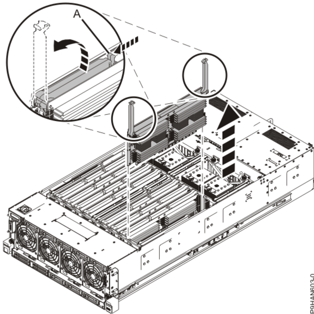
Figure 45. Retrait d'une carte d'extension de mémoire
