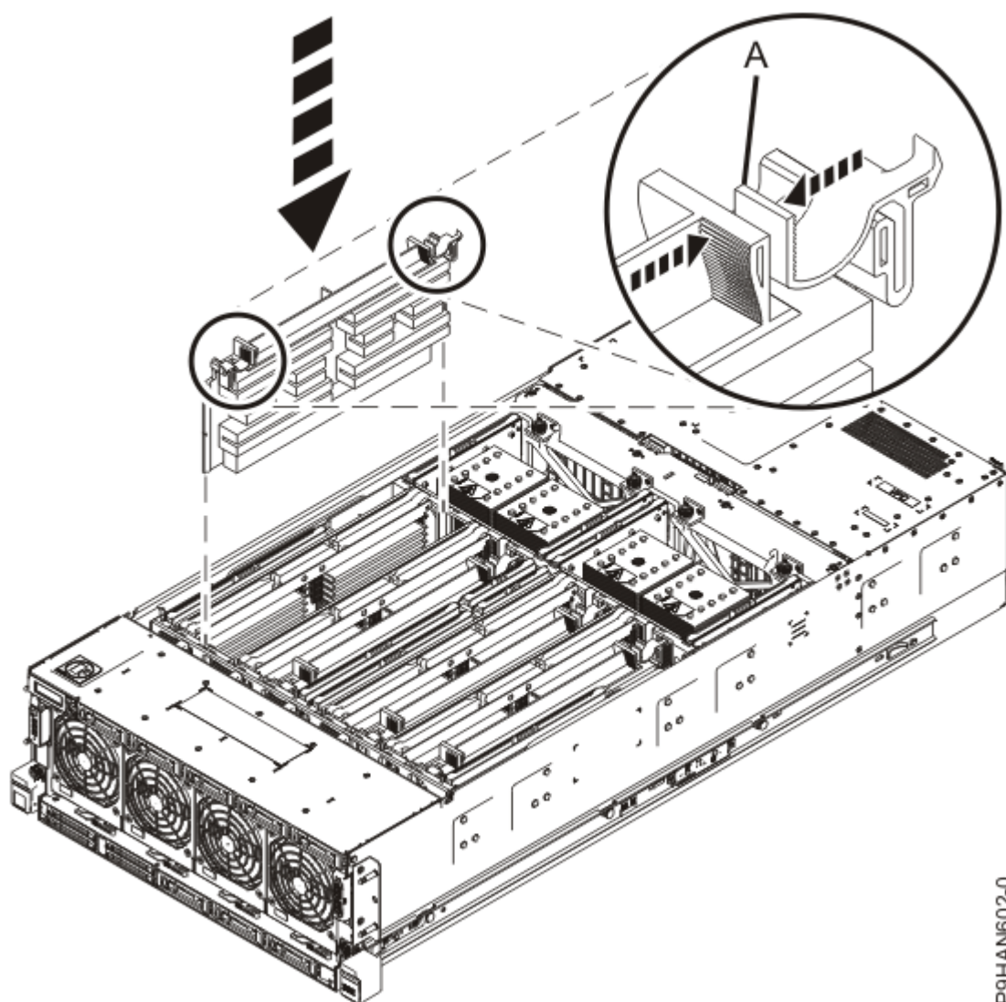
Figure 54. Insertion d'un obturateur de carte d'extension de mémoire
