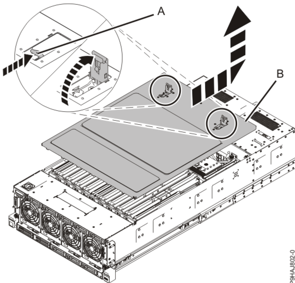
Figure 25. Retrait du capot d'accès
