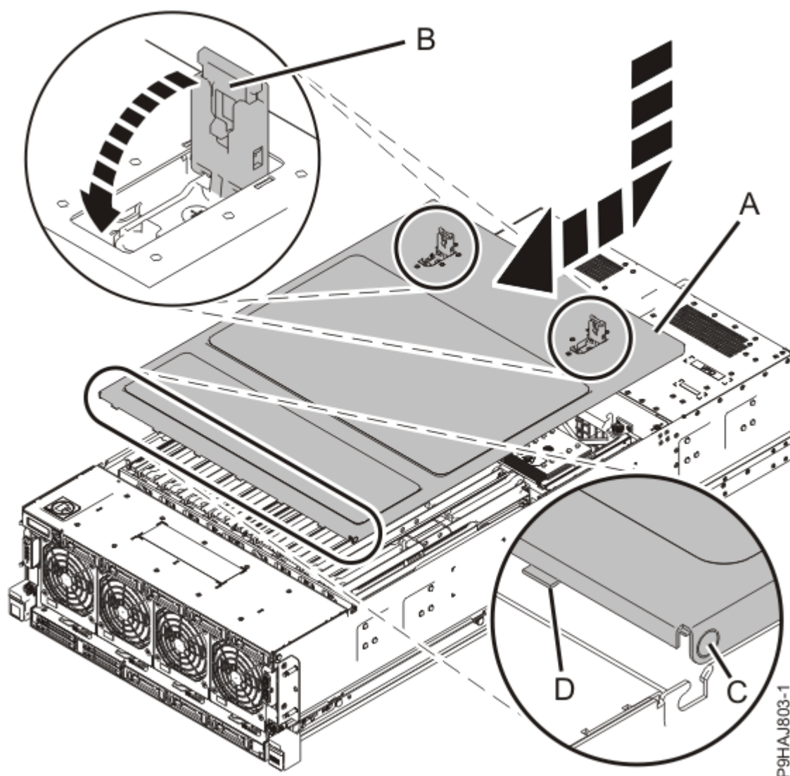
Figure 47. Installation du capot d'accès
