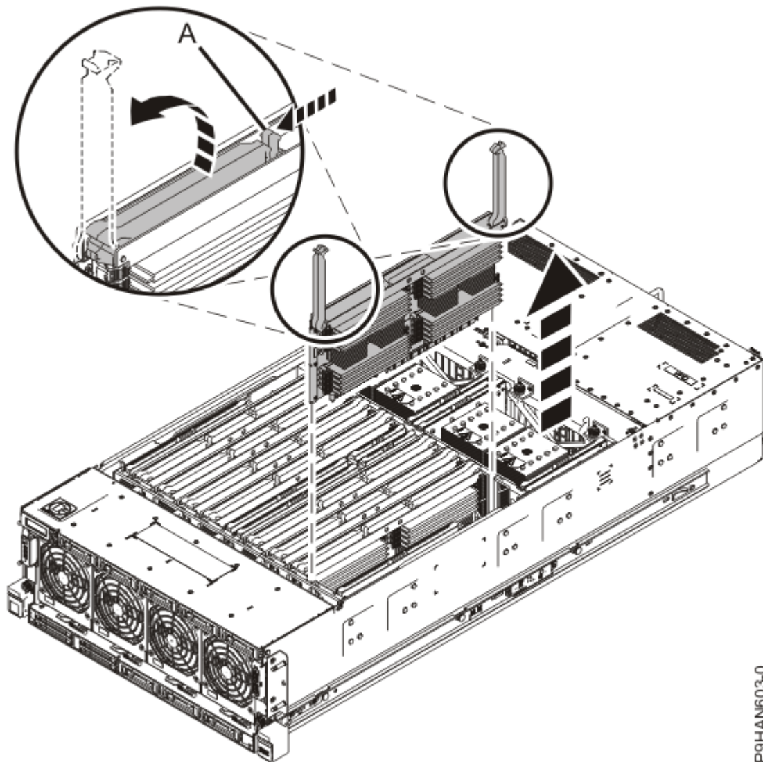
Figure 26. Retrait d'une carte d'extension de mémoire
