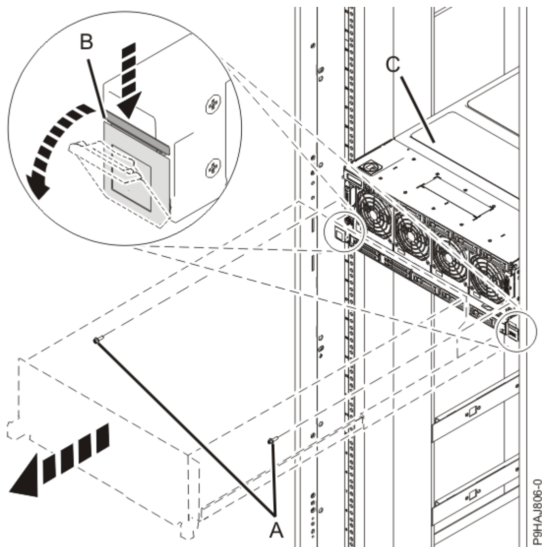
Figure 51. Mise en position de maintenance du système
