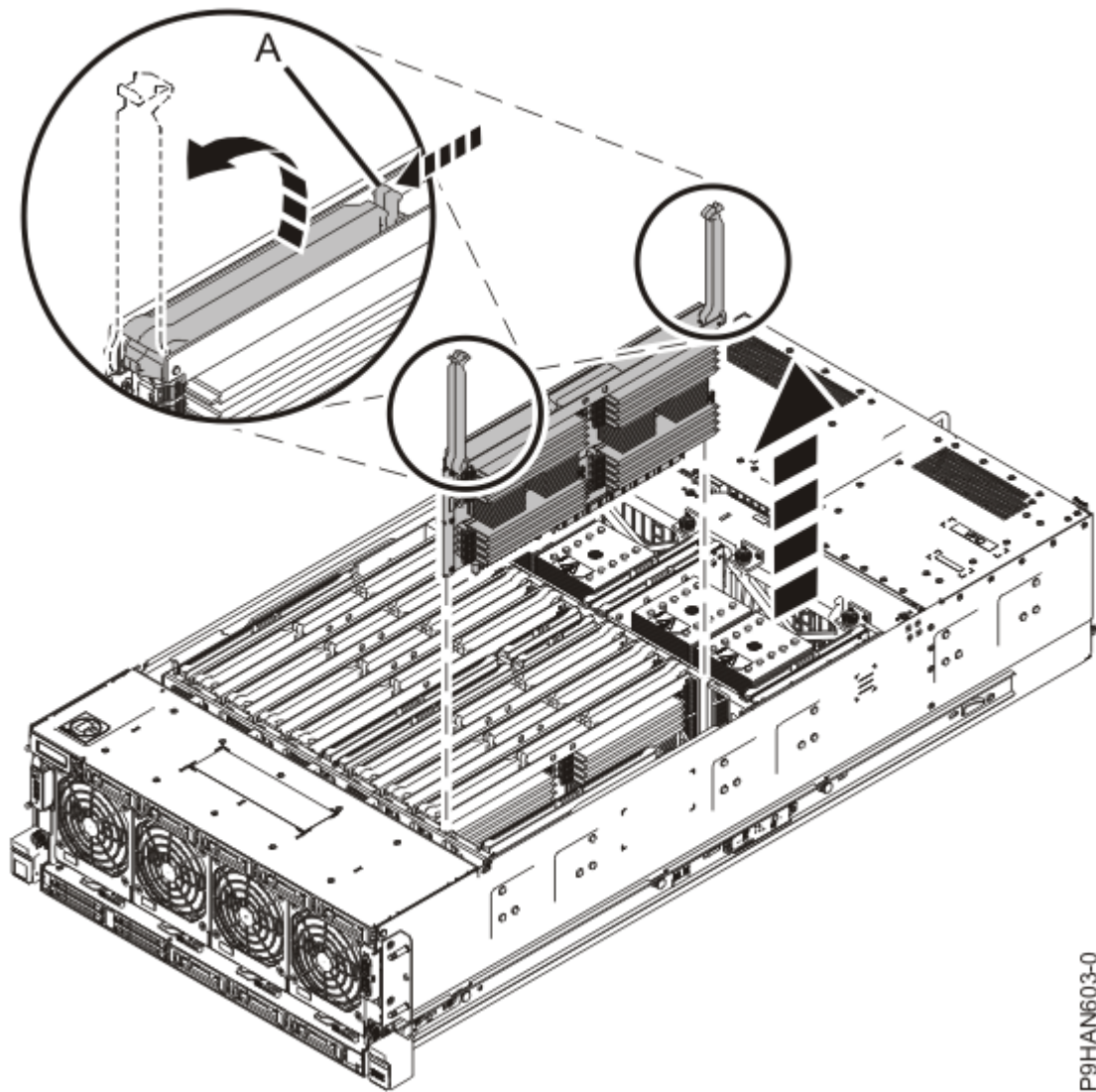
Figure 15. Retrait d'une carte d'extension de mémoire
