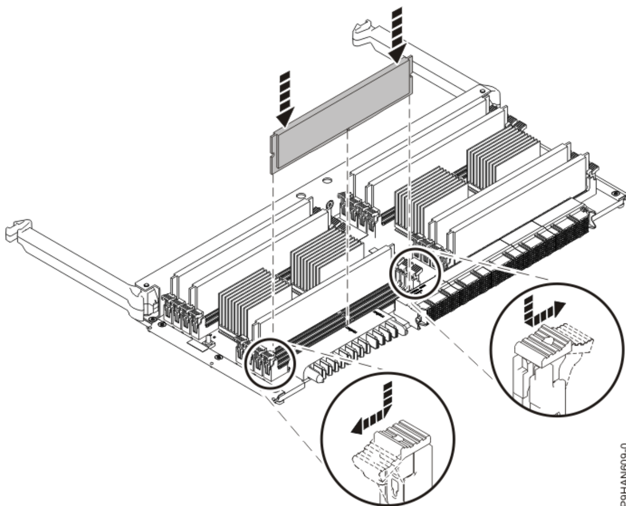
Figure 5. Installation de modules de mémoire dans une carte d'extension de mémoire
