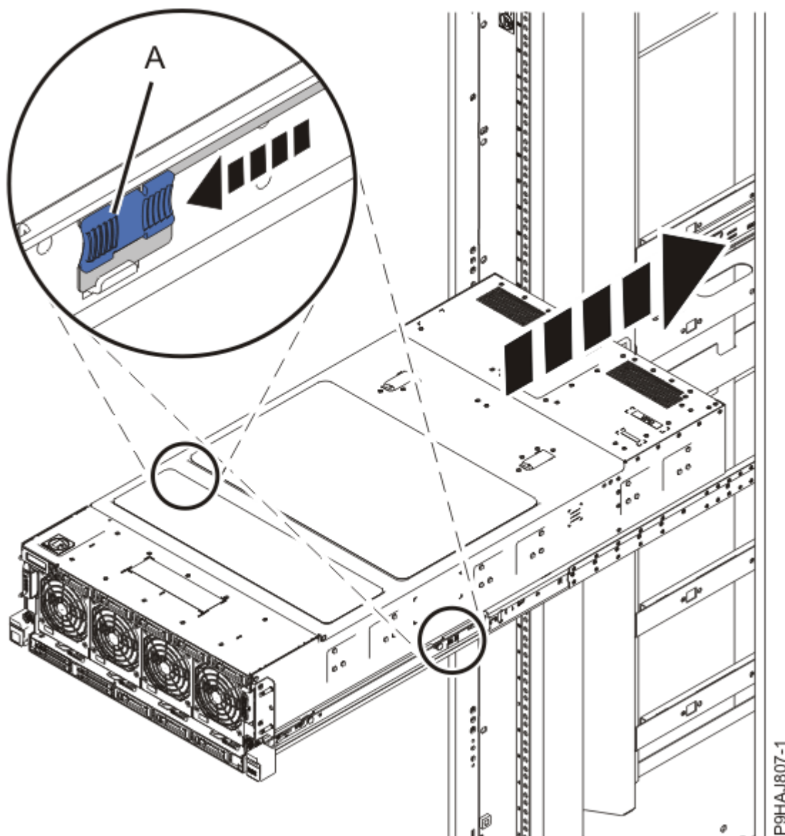
Figure 30. Mise en position de fonctionnement du système
