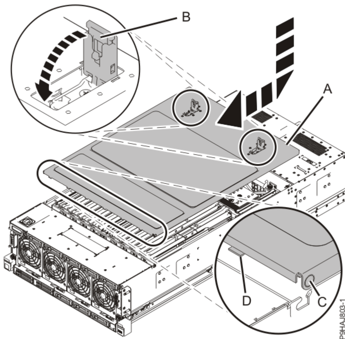
Figure 7. Installation du capot d'accès
