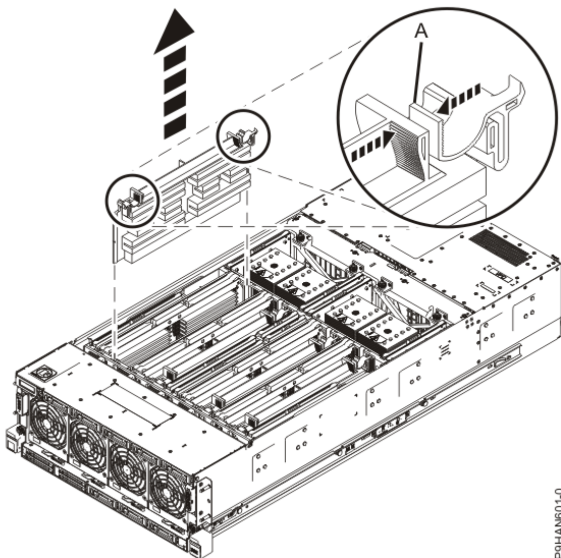
Figure 35. Retrait d'un obturateur de carte d'extension de mémoire
