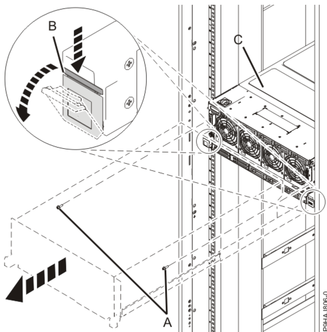
Figure 33. Mise en position de maintenance du système
