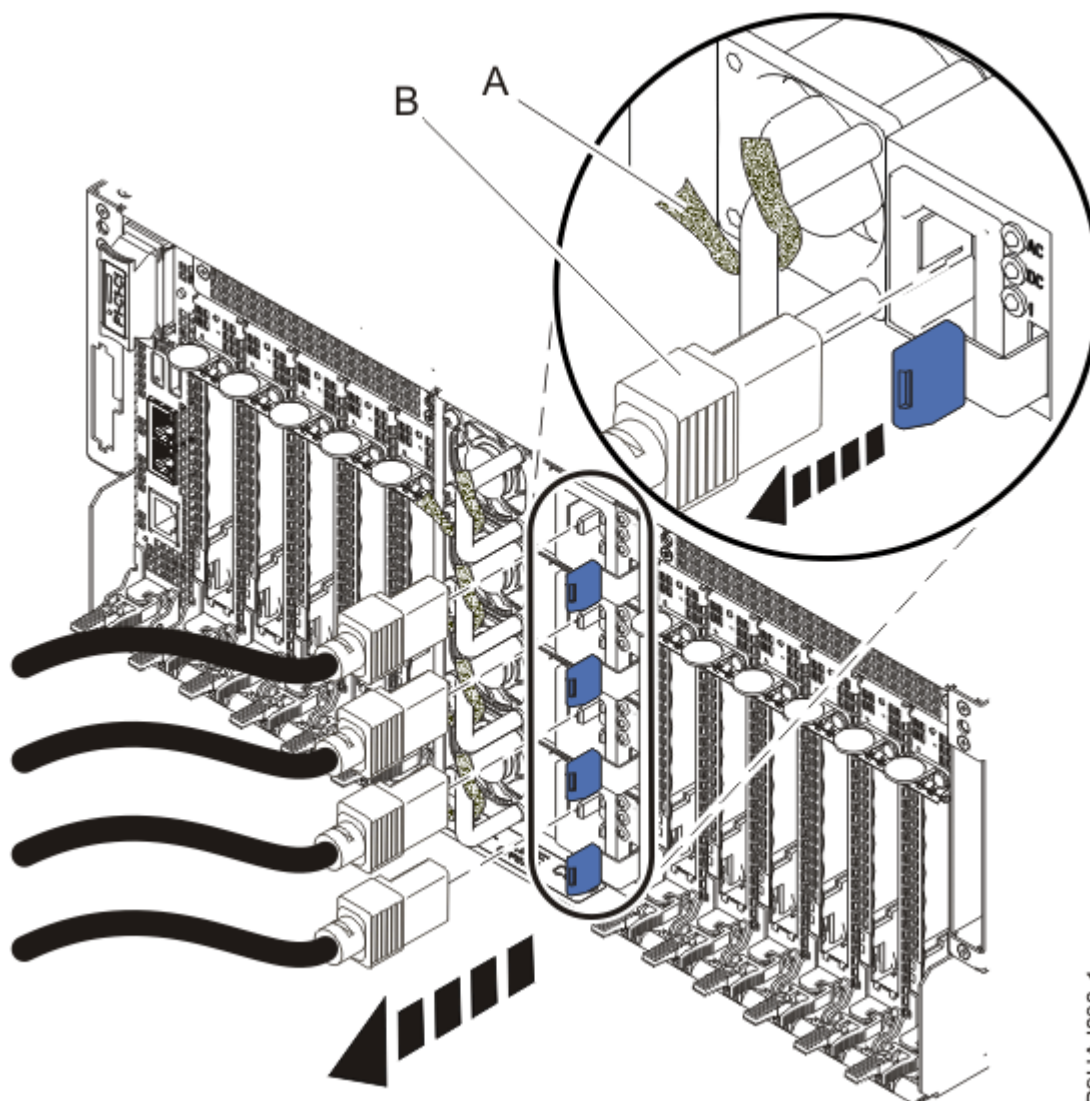
Figure 10. Retrait des cordons d'alimentation
