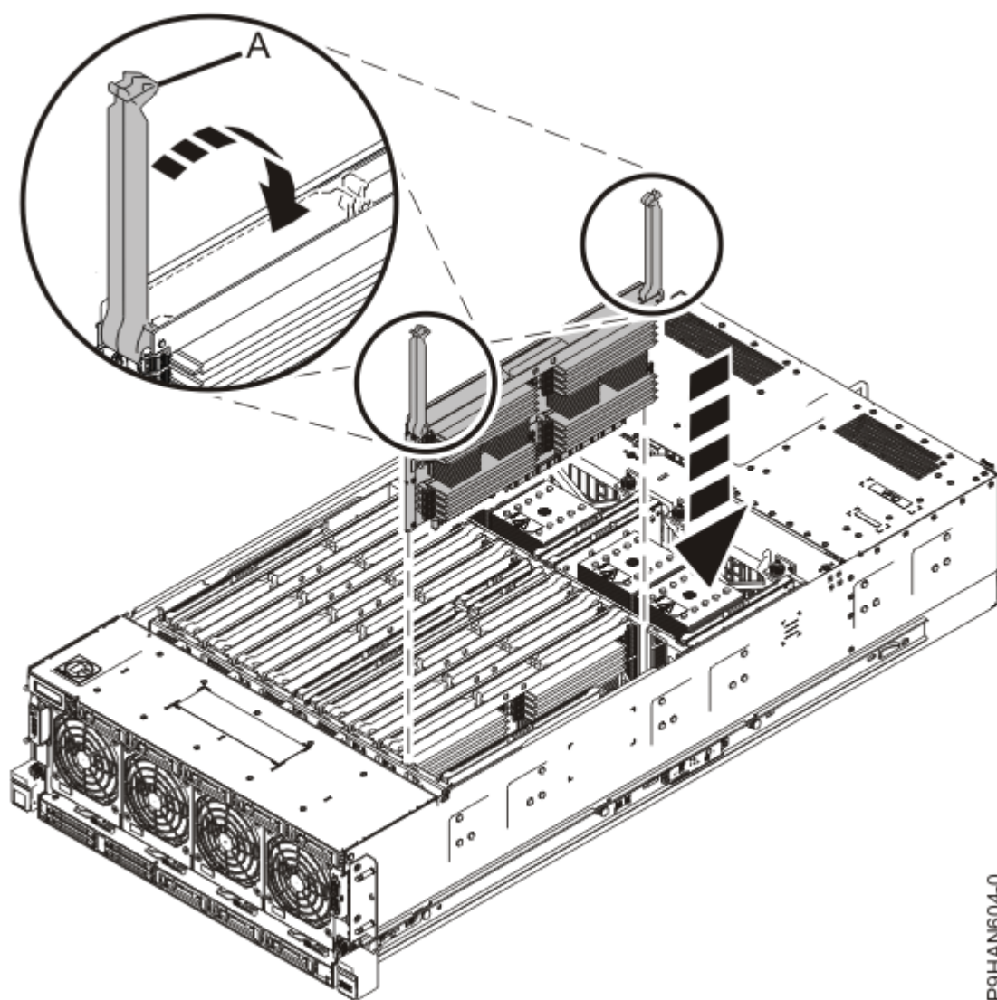
Figure 28. Insertion d'une carte d'extension de mémoire
