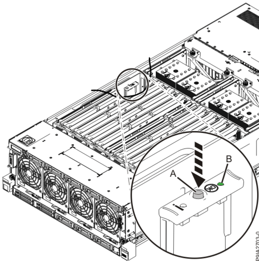
Figure 13. Activation du voyant d'identification
