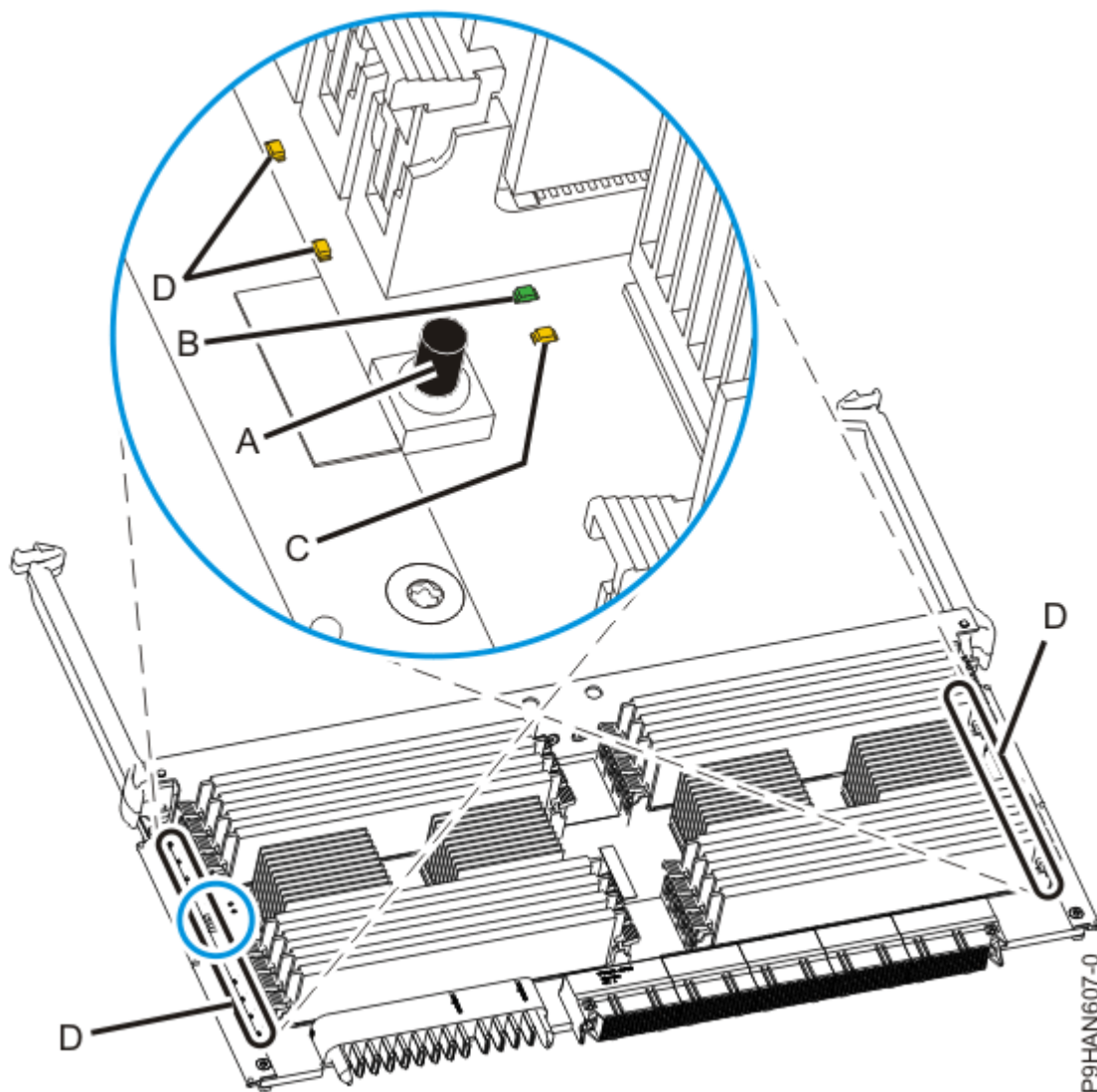
Figure 16. Identification d'un module de mémoire
