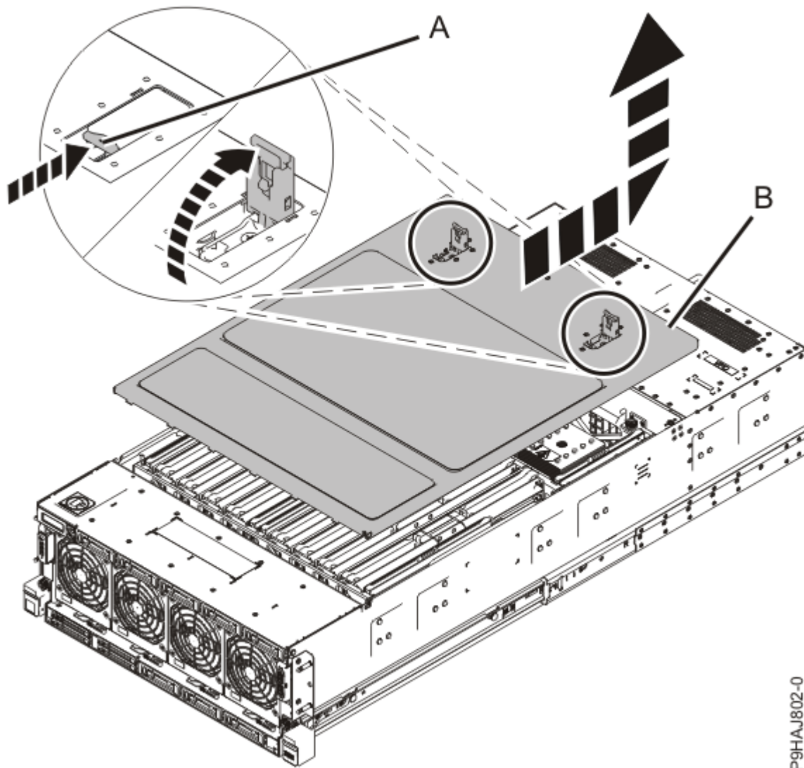
Figure 34. Retrait du capot d'accès
