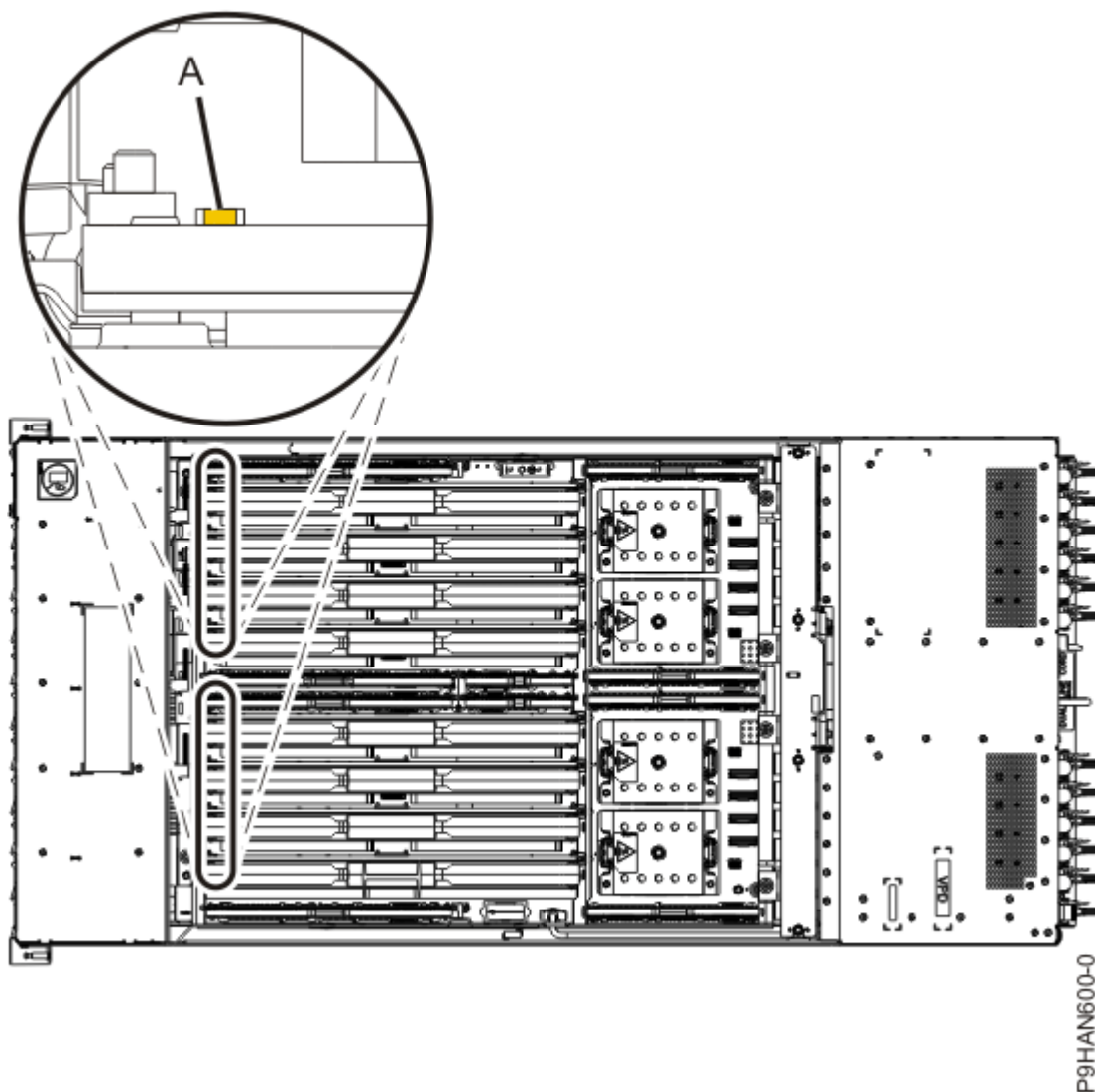
Figure 44. Voyants d'une carte d'extension de mémoire
