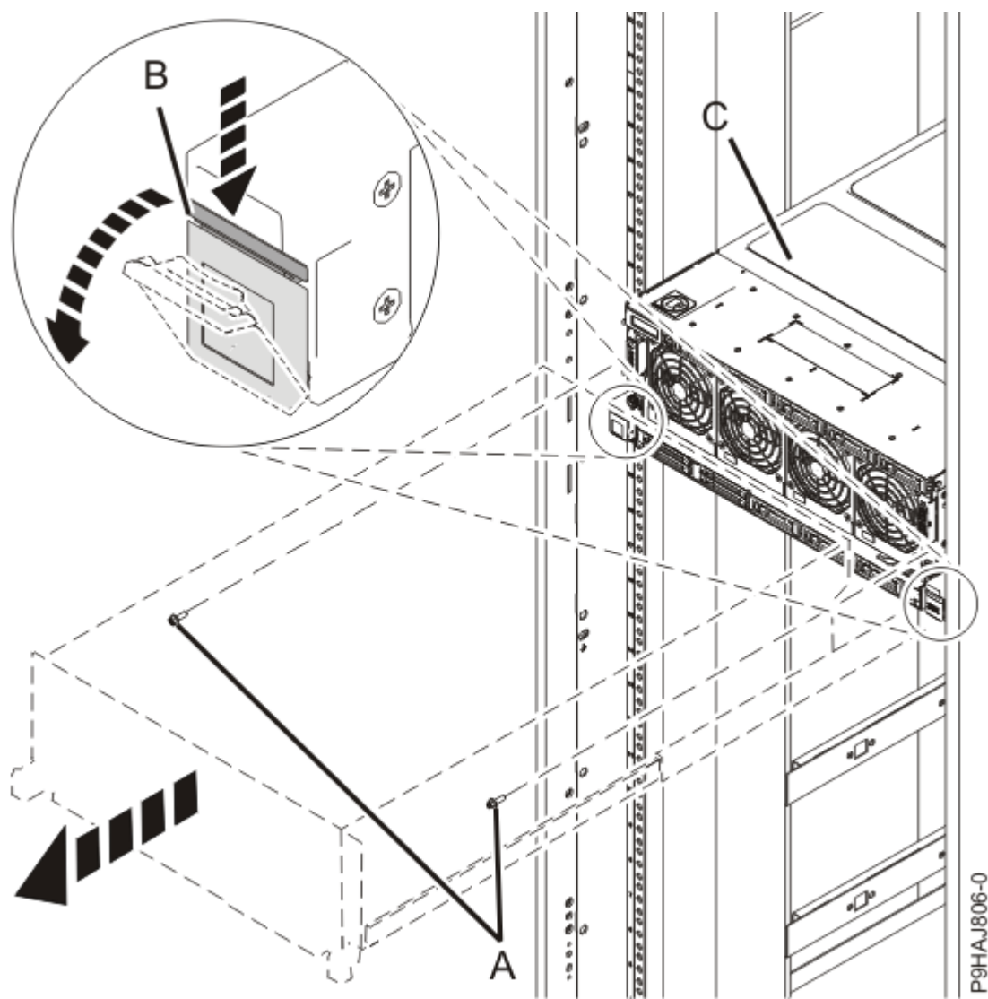
Figure 11. Mise en position de maintenance du système
