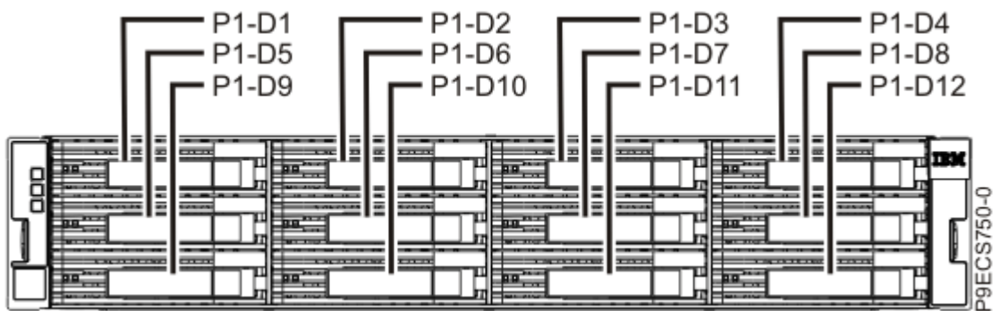
Figure 9. Vue avant de l'armoire de stockage ESLL montrant les emplacements des unités
