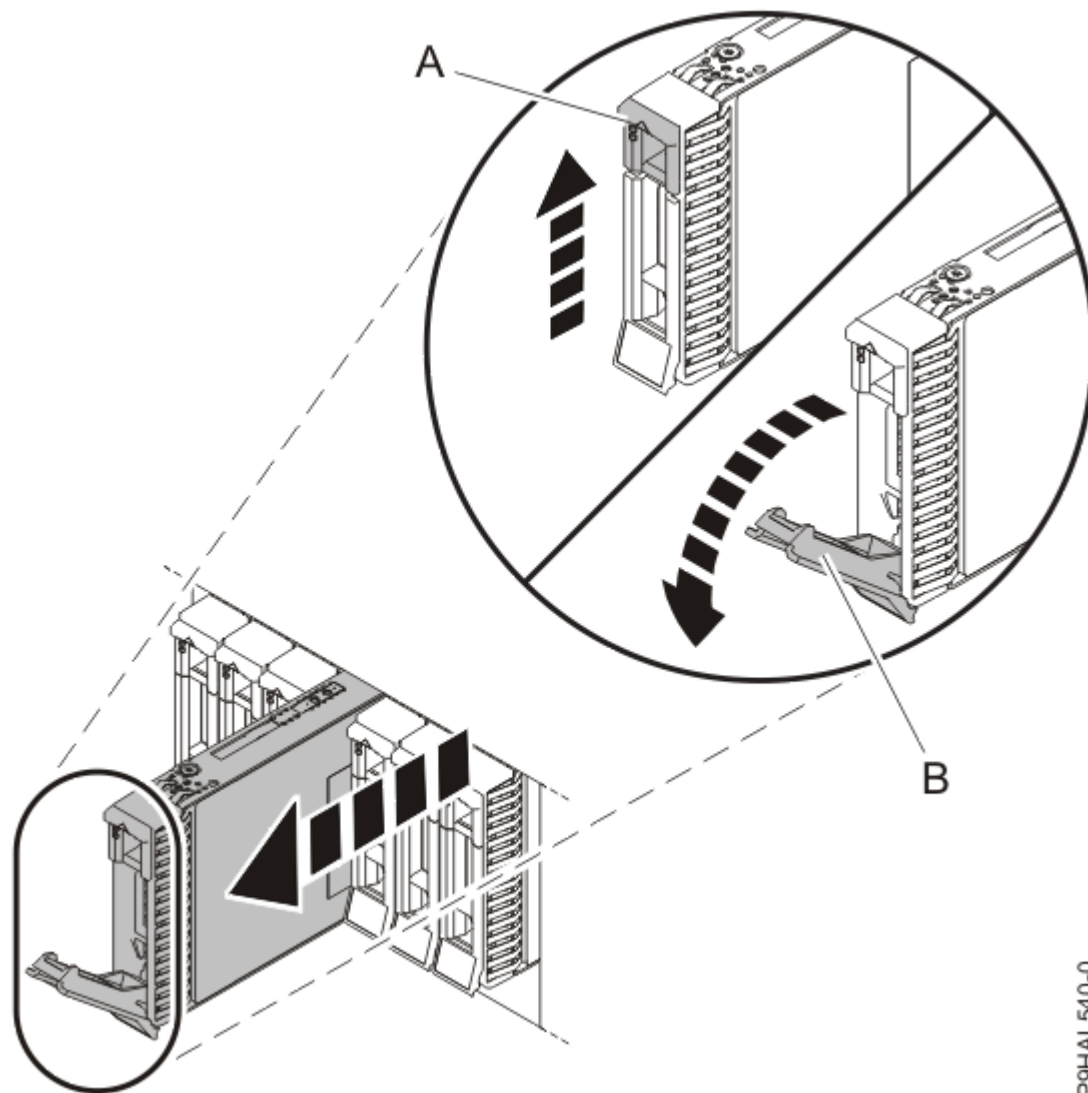
Figure 16. Déverrouillage et retrait de l'unité
