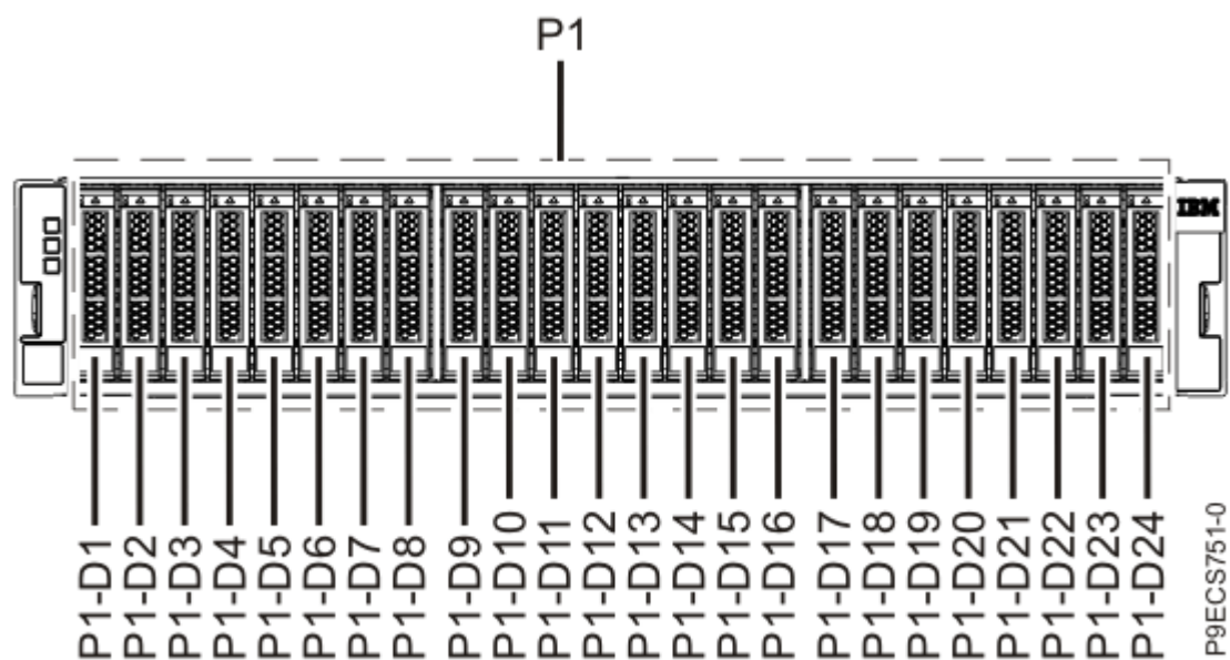
Figure 10. Vue avant de l'armoire de stockage ESLS montrant les emplacements des unités
