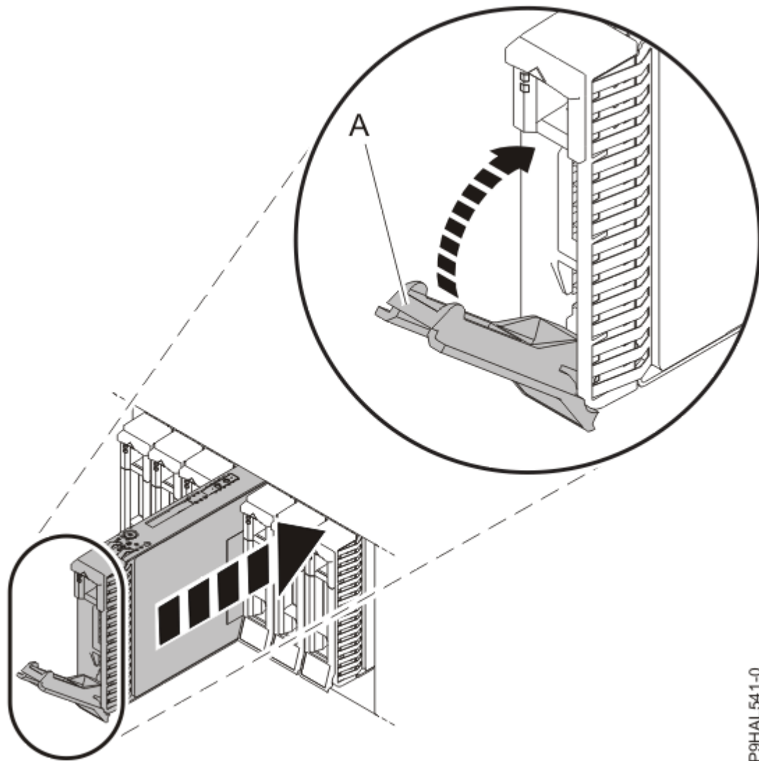
Figure 18. Remise en place d'une unité dans un boîtier
