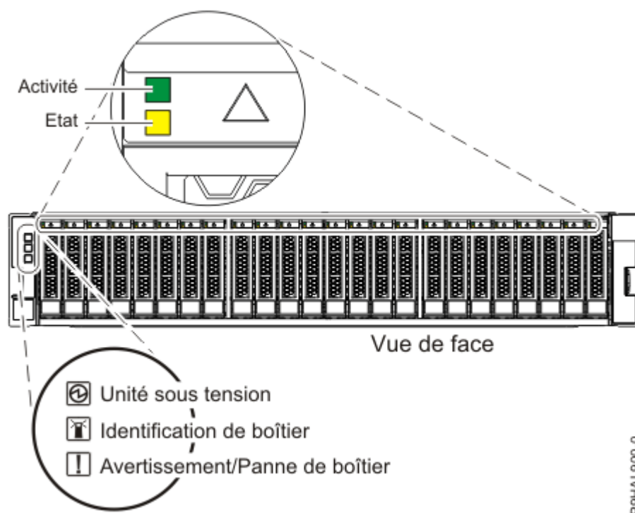
Figure 4. Vue avant de l'armoire de stockage montrant les voyants d'activité
