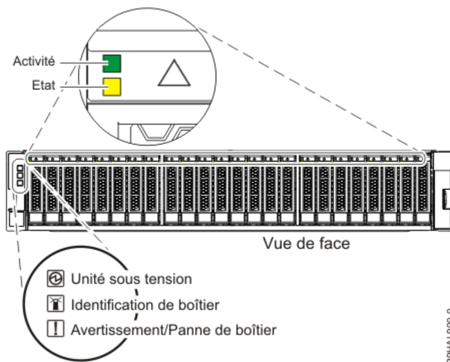
Figure 12. Vue avant de l'armoire de stockage montrant les voyants d'activité
