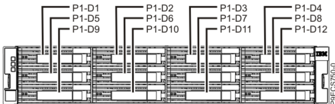
Figure 1. Vue avant de l'armoire de stockage ESLL montrant les emplacements des unités
