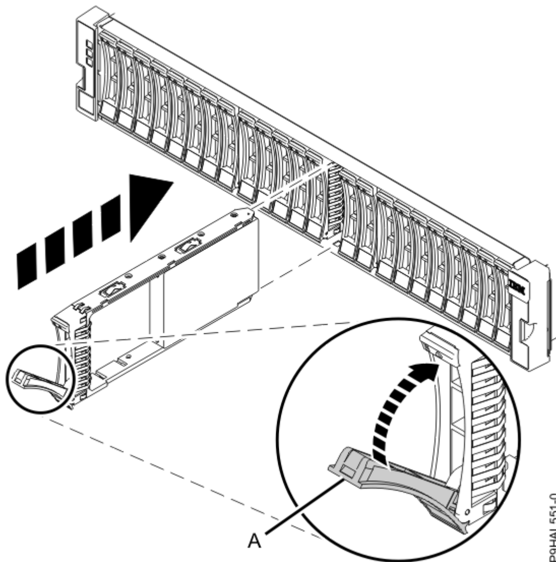
Figure 6. Installation ou remise en place d'une unité dans un boîtier
