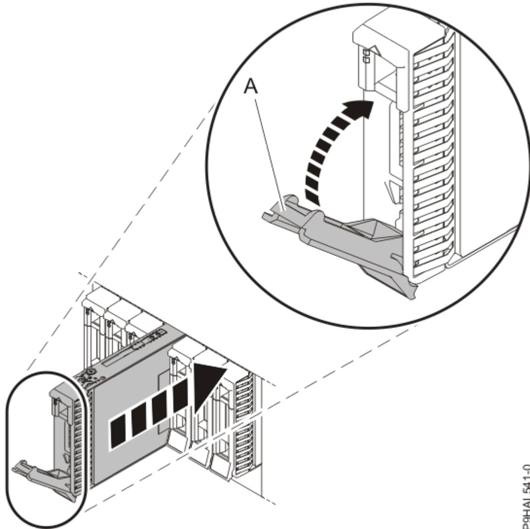
Figure 20. Installation d'une unité dans un système
