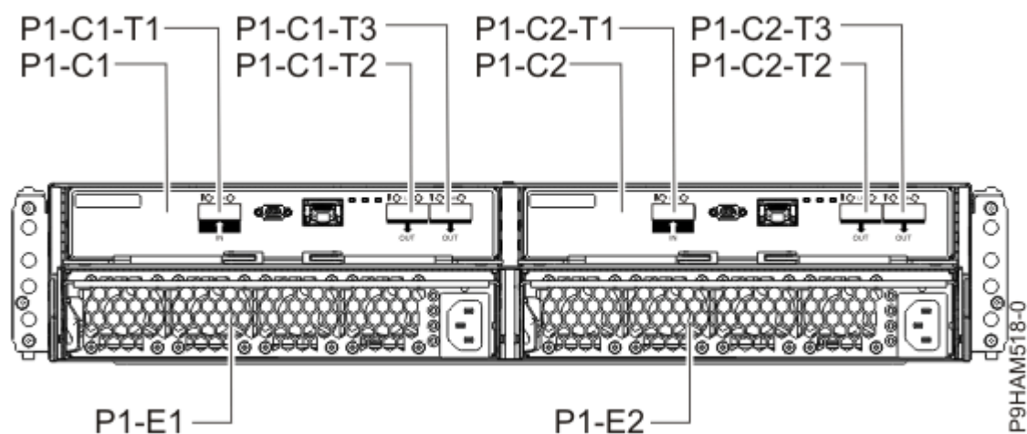
Figure 2. Vue arrière du 5887
