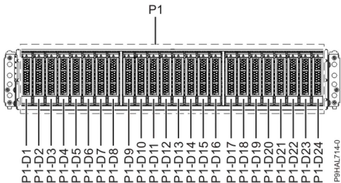
Figure 1. Vue avant du 5887 illustrant les emplacements des unités de disque
