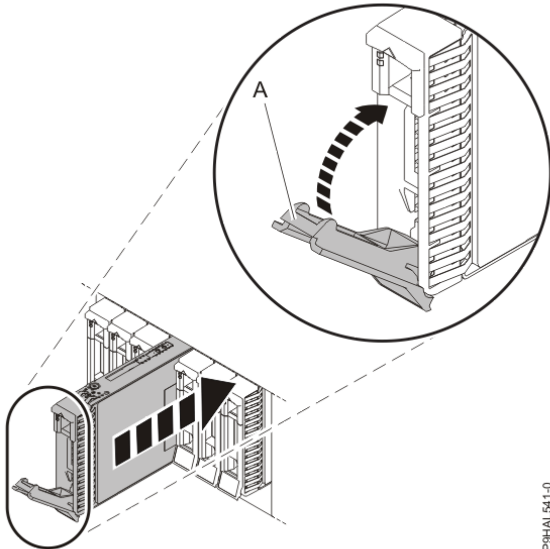
Figure 17. Remise en place d'une unité dans un boîtier
