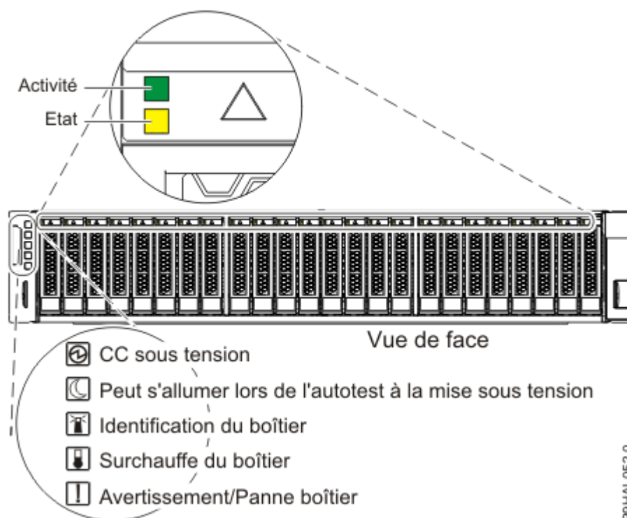
Figure 3. Vue avant du 5887 illustrant les emplacements des voyants d'activité
