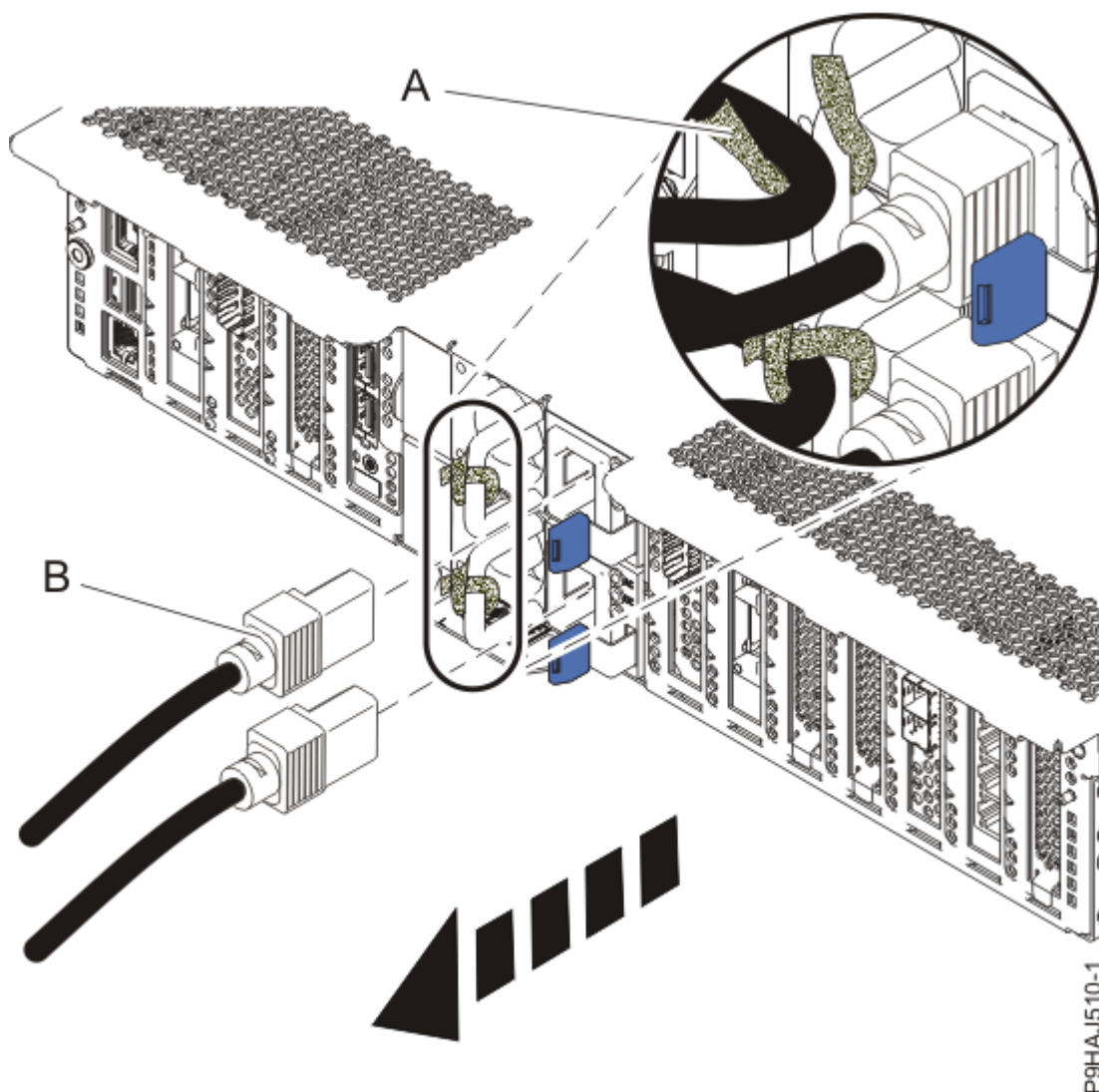
Figure 34. Retrait des cordons d'alimentation
