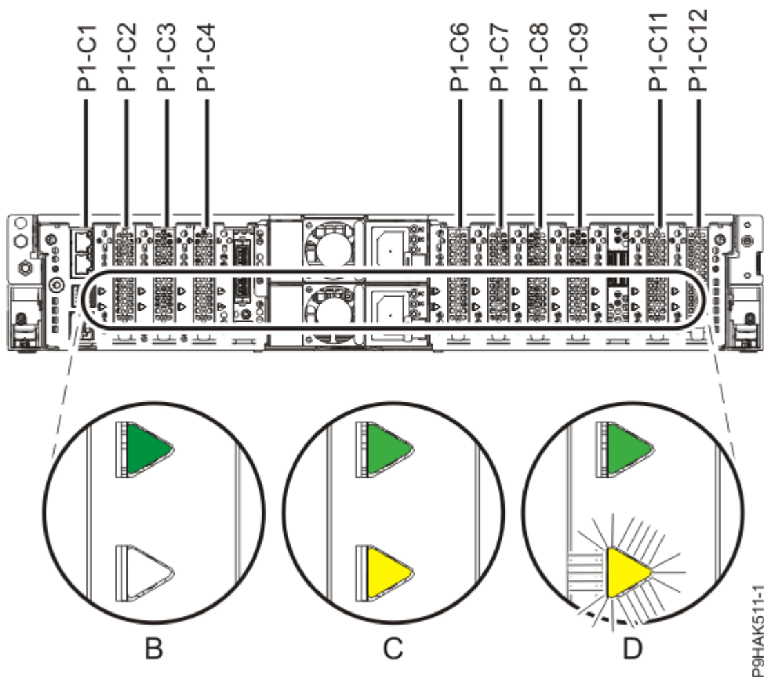
Figure 32. Localisations des emplacements d'adaptateur et des voyants sur le système 5105-22E, 9008-22L, 9009-22A, 9009-22G, 9223-22H ou 9223-22S
