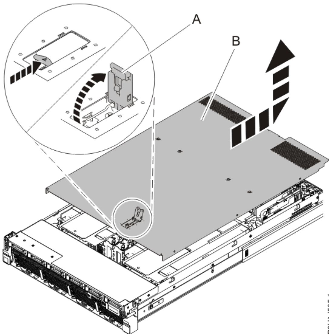
Figure 37. Retrait du capot d'accès
