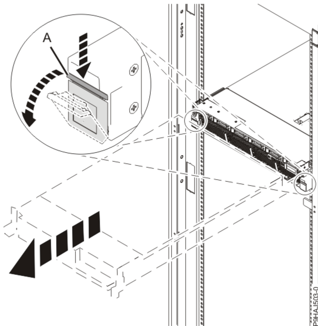
Figure 9. Déblocage des loquets latéraux
