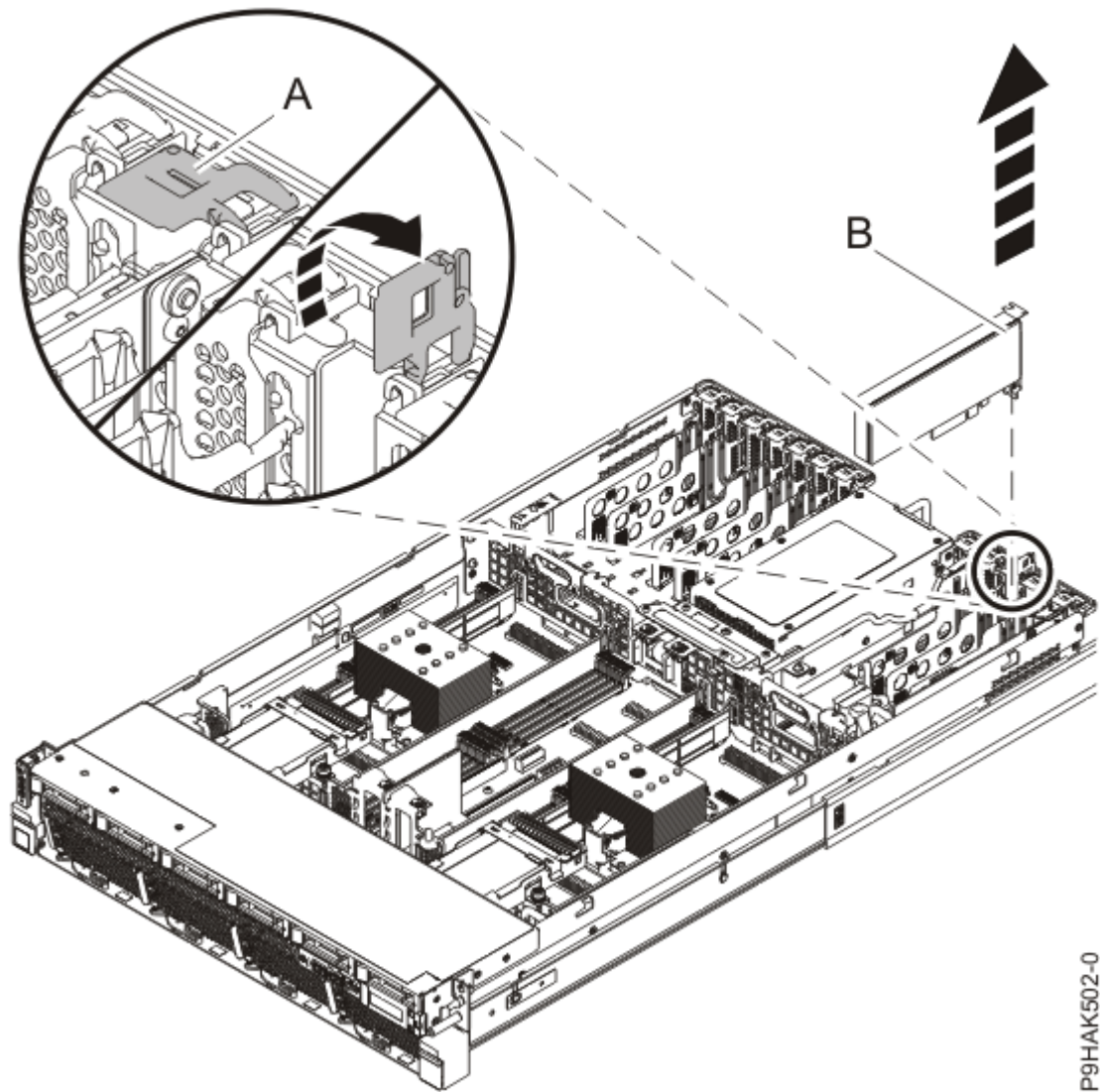
Figure 25. Retrait d'un adaptateur du système 5105-22E, 9008-22L, 9009-22A, 9009-22G, 9223-22H ou 9223-22S
