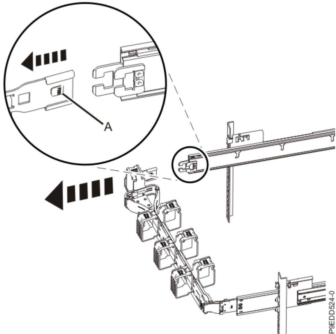
Figure 17. Libération du crochet de montage
