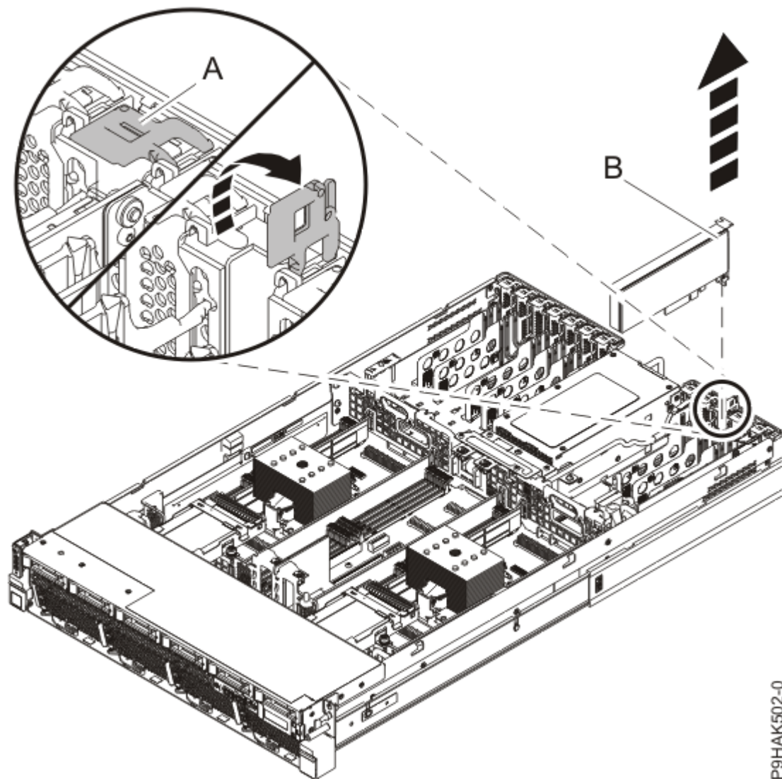
Figure 38. Retrait d'un adaptateur du système 5105-22E, 9008-22L, 9009-22A, 9009-22G, 9223-22H ou 9223-22S
