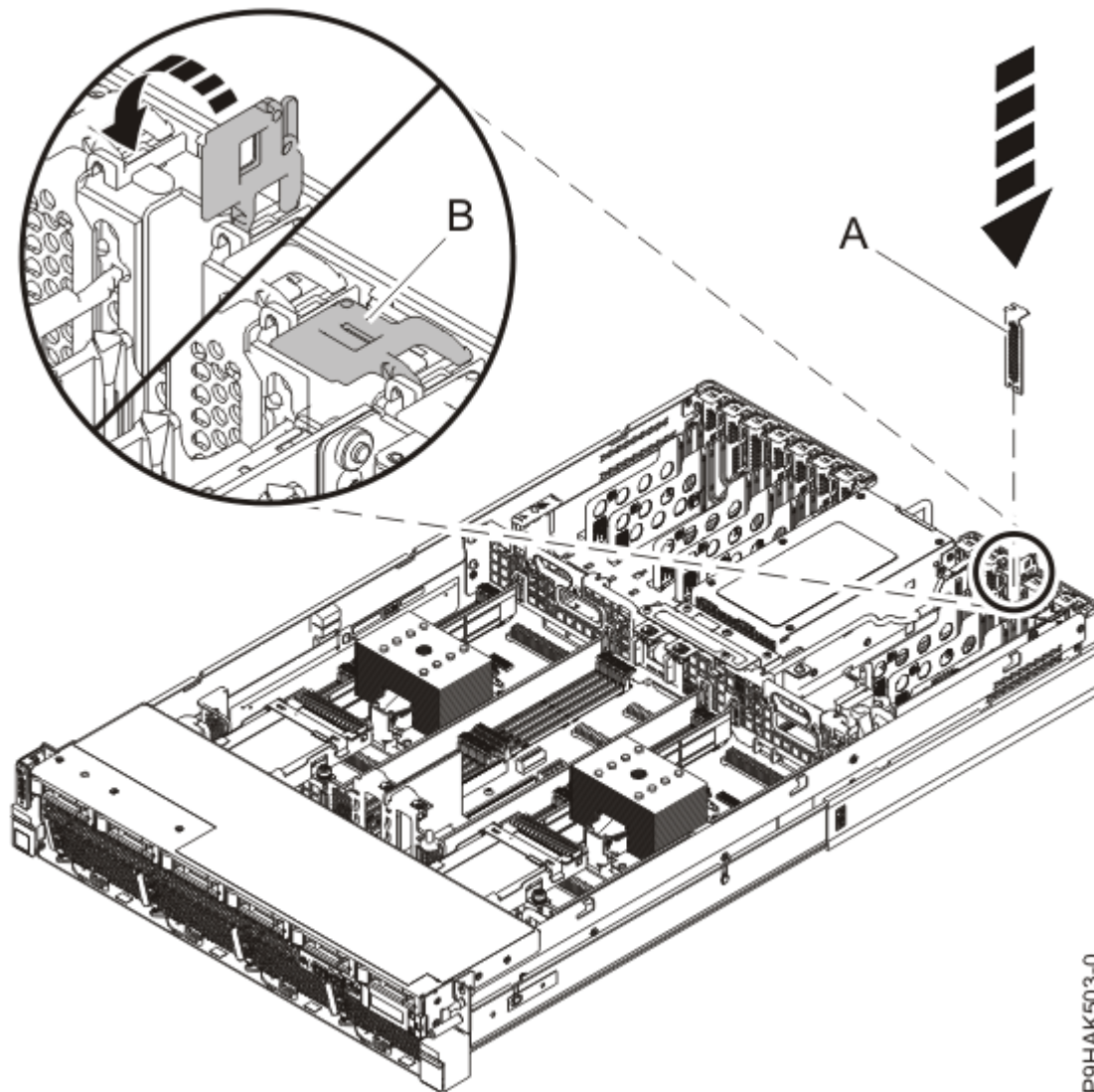
Figure 39. Installation d'un obturateur dans un emplacement d'un système 5105-22E, 9008-22L, 9009-22A, 9009-22G, 9223-22H ou 9223-22S
