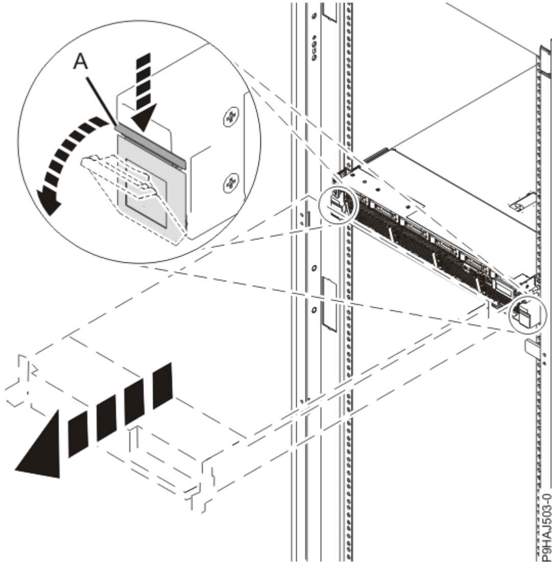
Figure 23. Déblocage des loquets latéraux
