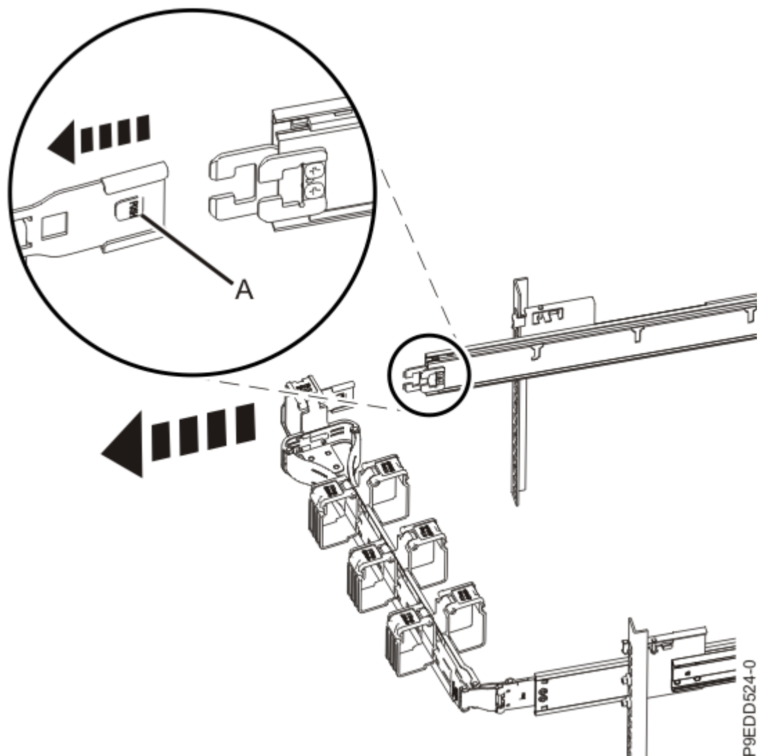
Figure 5. Libération du crochet de montage
