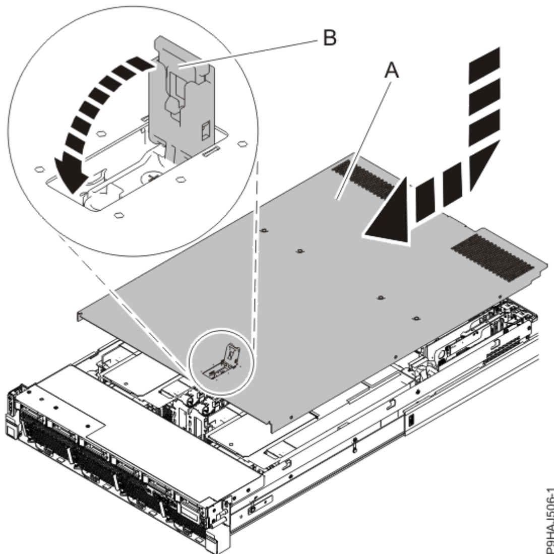
Figure 12. Installation du capot d'accès
