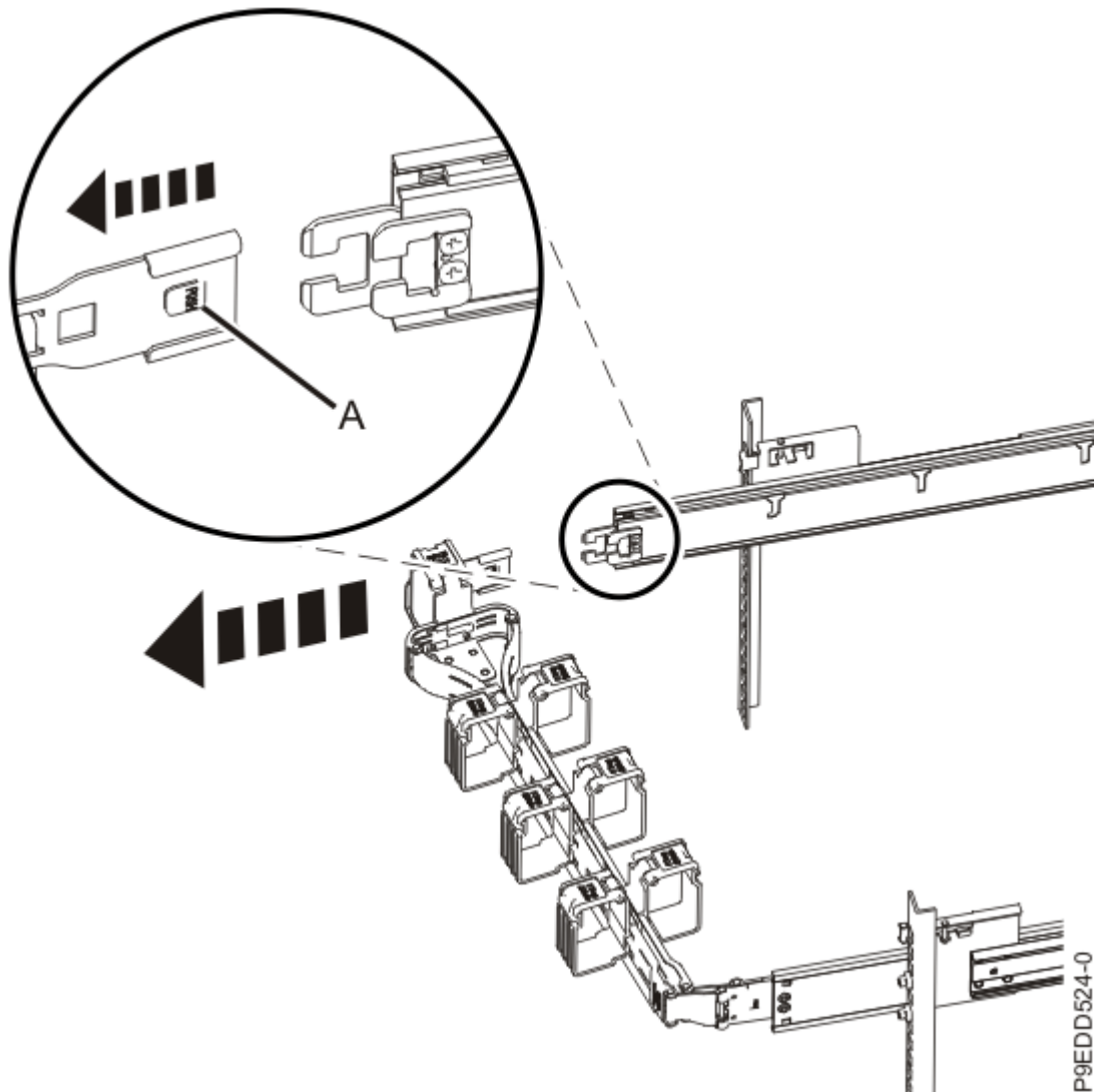
Figure 2. Libération du crochet de montage
