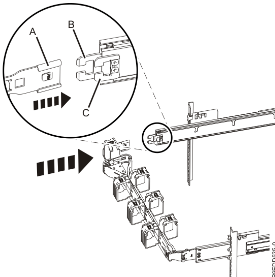
Figure 7. Fermeture du bras de routage des câbles
