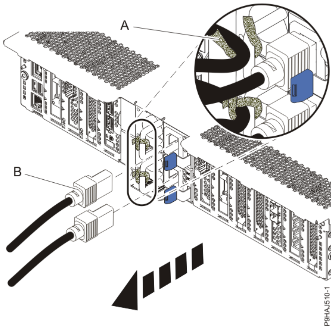
Figure 18. Retrait des cordons d'alimentation
