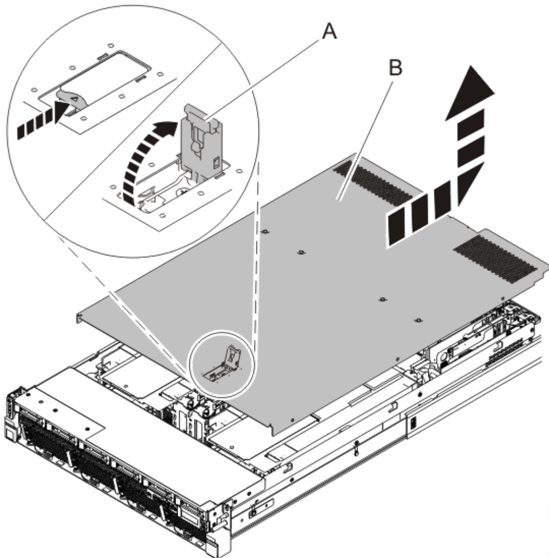
Figure 24. Retrait du capot d'accès
