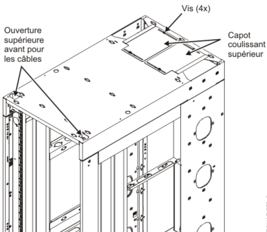
Figure 17. Câblage aérien
