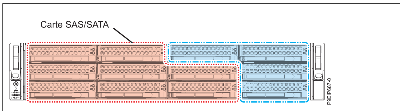
Figure 5. Jusqu'à huit unités SAS ou SATA connectées à une carte SAS/SATA, jusqu'à quatre unités SAS ou SATA connectées à un contrôleur intégré et jusqu'à deux disques sur module (DOM)
