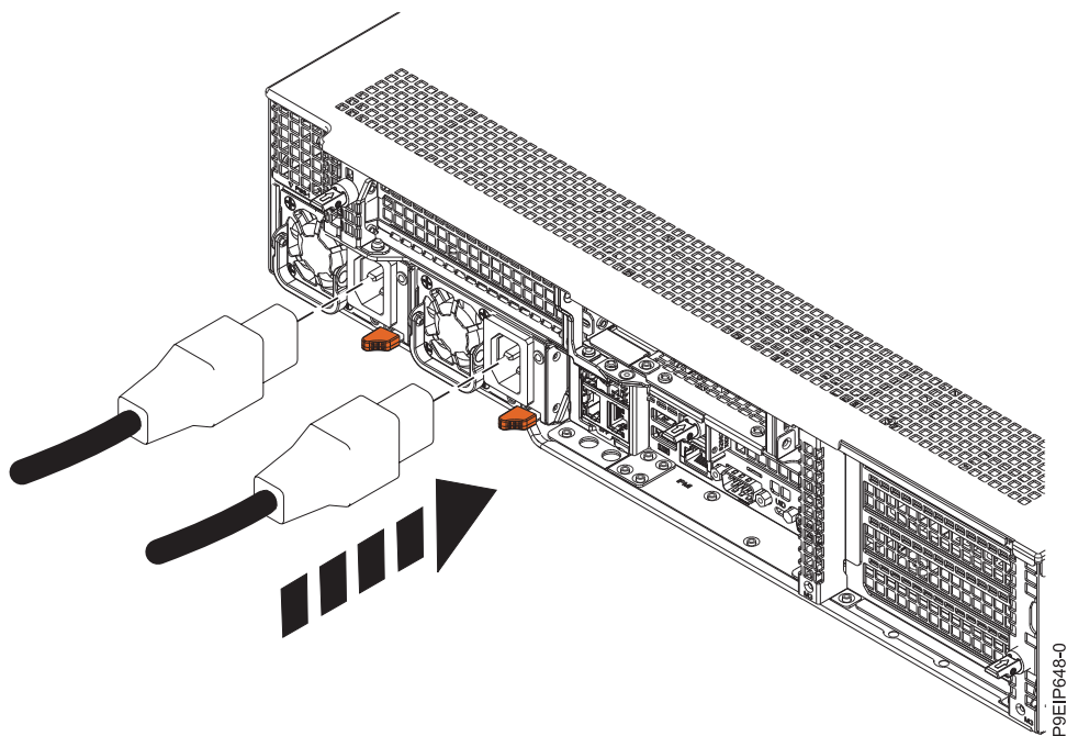
Figure 72. Connexion des cordons d'alimentation au système
