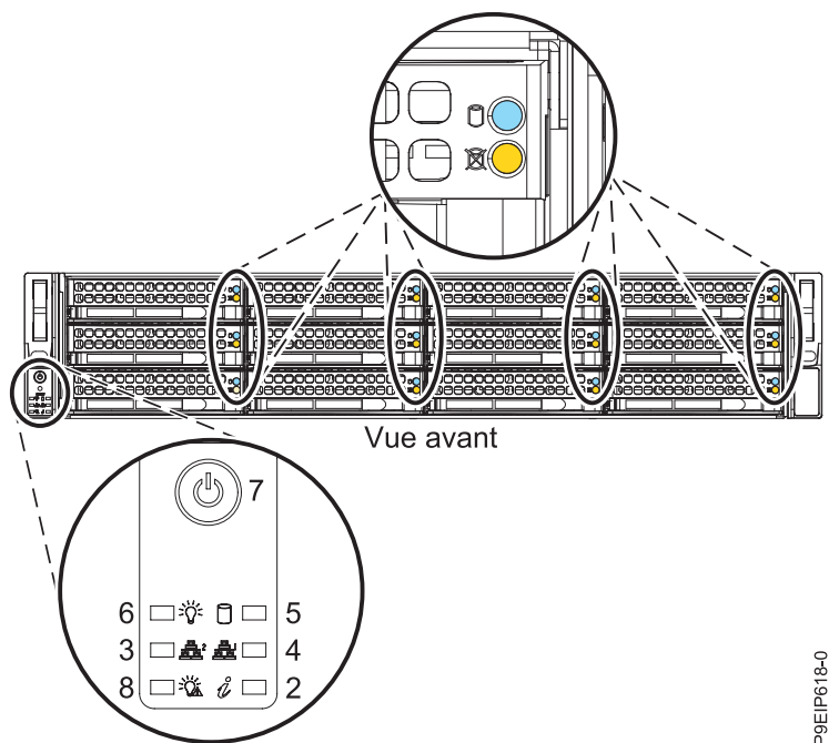
Figure 63. Voyants situés sur le devant du système
