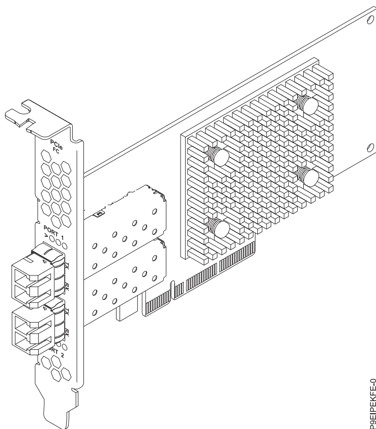
Figure 46. Carte Carte Fibre Channel Qlogic QLE2742 32 Go PCIe3 x8 2 ports LP
