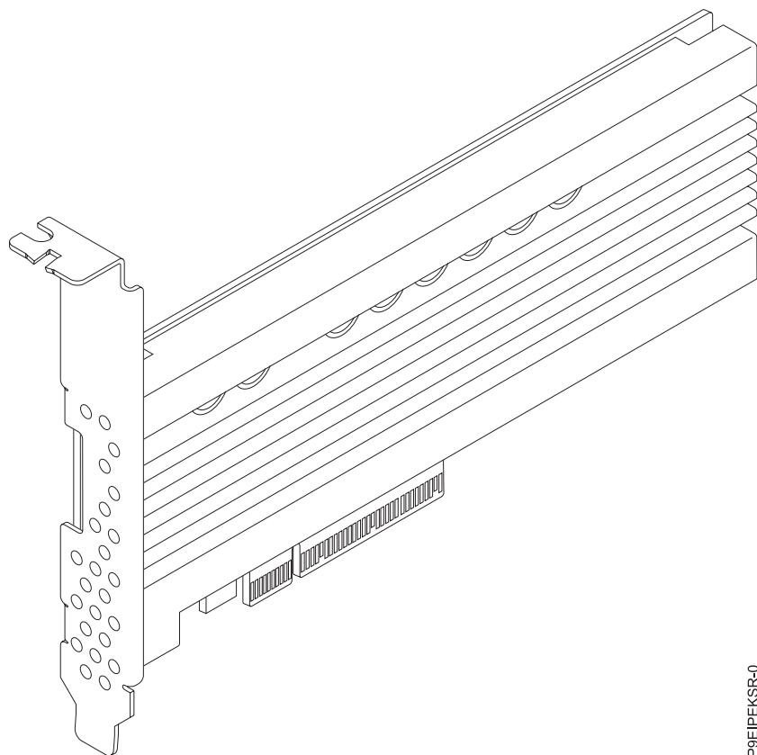
Figure 52. Carte Samsung PM1725a NVMe 3,2 To 5DWPD PCIe3.0 x8 LP
