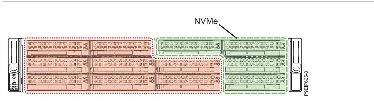
Figure 8. Jusqu'à huit unités SAS ou SATA ou un mélange d'unités de disque dur SAS et d'unités SSD SATA (huit unités au total), une carte SAS/SATA, quatre unités NVMe connectées à une carte NVMe et jusqu'à deux disques sur module (DOM)
