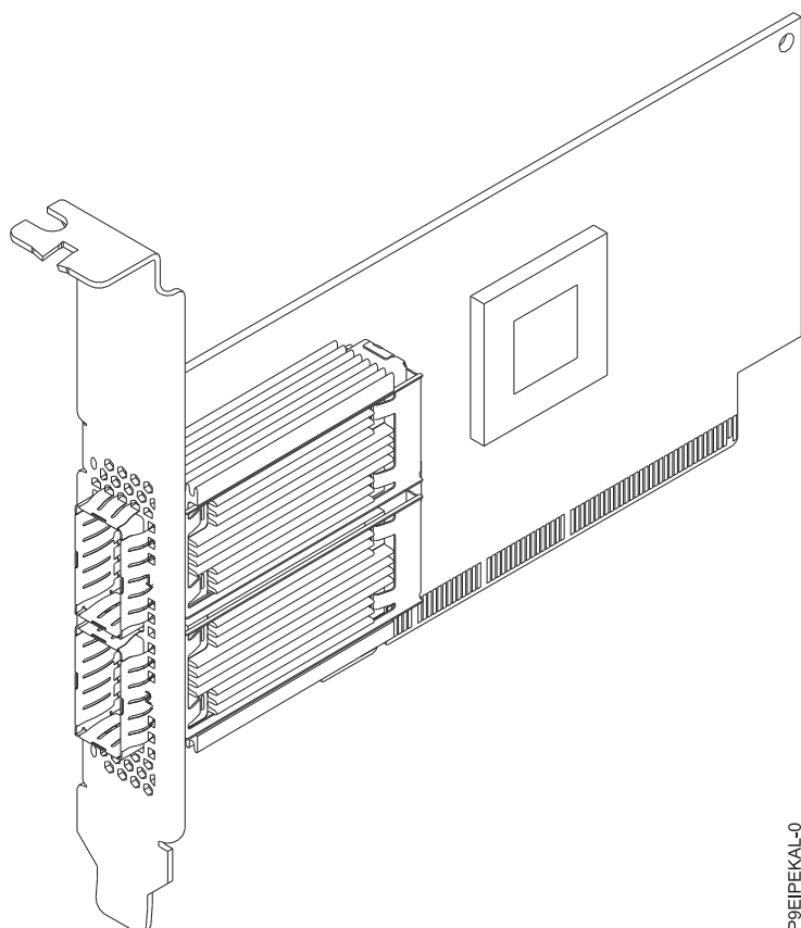
Figure 34. Carte Mellanox MCX456A-ECAT ConnectX-4 VPI EDR InfiniBand 100 Gb/s et 100 GbE double port QSFP28 PCIe3.0 x16 LP
