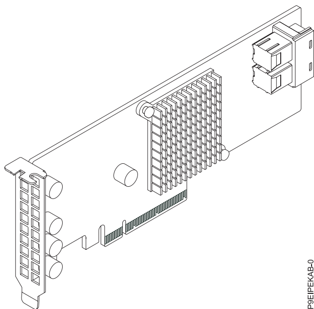
Figure 30. SMC AOC-K-S3008L-L8i 12 Gbps SAS3/RAID 0,1 et 10 PCIe3.0 x8 LP avec câbles
