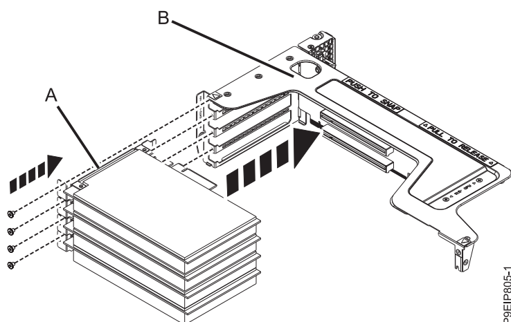
Figure 61. Insertion d'une carte PCIe dans le connecteur de bus
