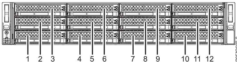
Figure 10. Les unités NVMe vont dans les emplacements 9 à 12
