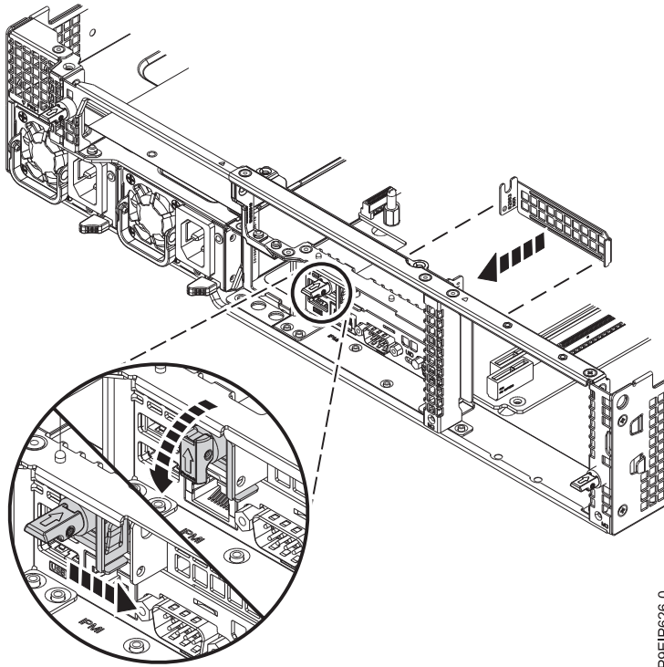
Figure 59. Passage du crochet de retenue de l'équerre de fixation en position fermée
