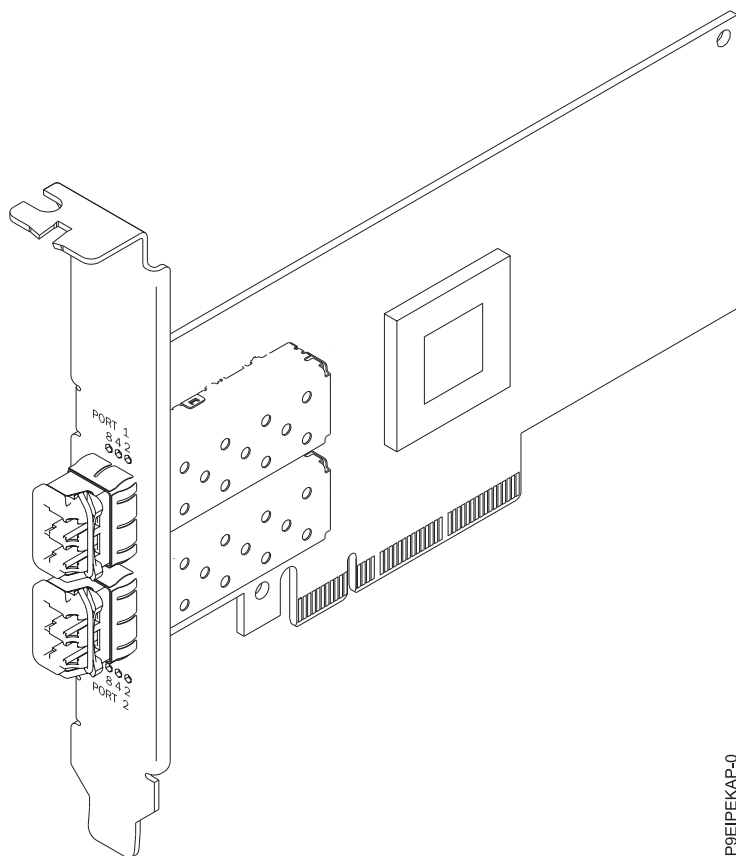
Figure 36. Carte Mellanox MCX415A-CCAT ConnectX-4 EN 100 GbE un port QSFP28 PCIe3.0 x16 LP
