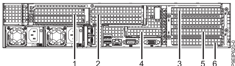
Figure 24. Vue arrière d'un système 9006-22P avec emplacements PCIe indiqués
