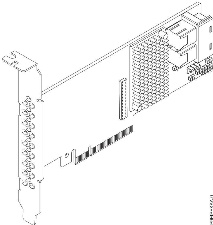
Figure 42. Broadcom (LSI) MegaRAID 9361-8i SAS3 Controller avec 8 ports internes (mémoire cache de 1 Go) PCIe3.0 x8 LP avec câbles
