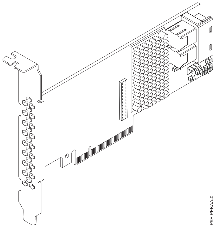
Figure 29. Broadcom (LSI) MegaRAID 9361-8i SAS3 Controller avec 8 ports internes (mémoire cache de 1 Go) PCIe3.0 x8 LP avec câbles
