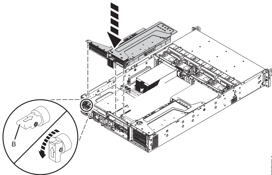
Figure 57. Insertion du connecteur de bus aux positions 1 et 2
