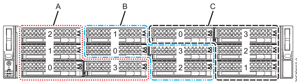
Figure 9. Port au mappage de baie d'unité
