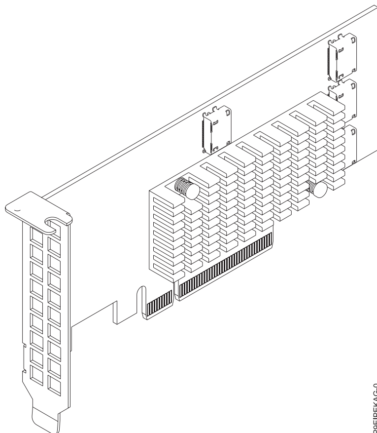
Figure 32. Adaptateur de bus hôte SMC quatre ports NVMe (PEX9733) PCIe3.0 x8 LP avec câbles
