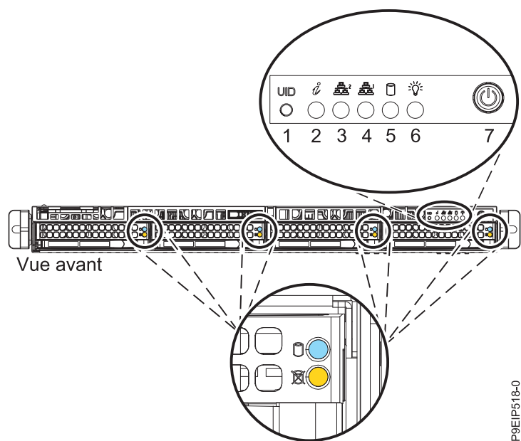
Figure 65. Interrupteur d'alimentation du système 9006-12P
