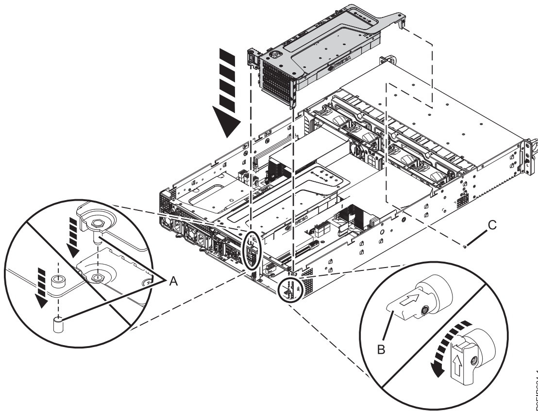
Figure 62. Insertion d'un connecteur de bus de carte PCIe
