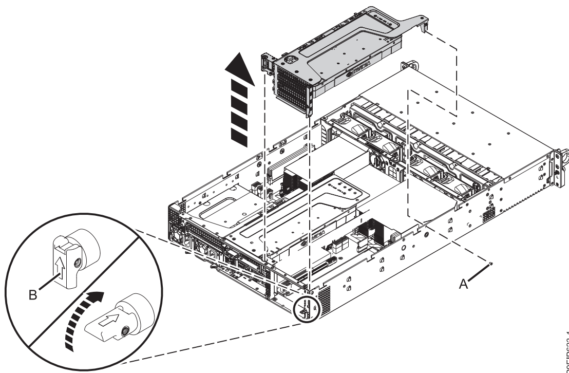
Figure 60. Retrait du connecteur de bus PCIe
