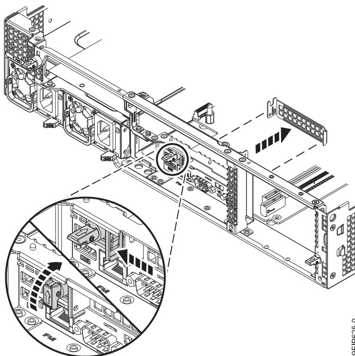
Figure 58. Libération de l'équerre de fixation
