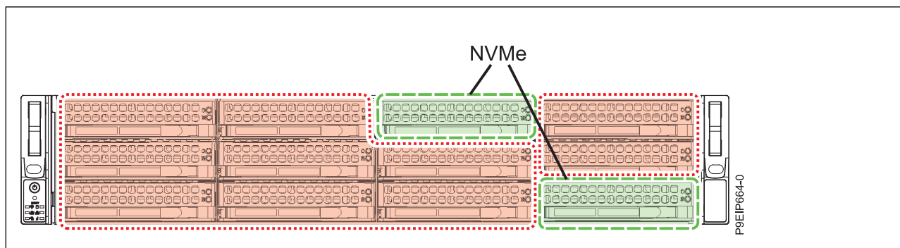
Figure 7. Jusqu'à 10 unités SAS ou SATA ou un mélange d'unités de disque dur SAS et d'unités SSD SATA (10 unités au total), une carte SAS/SATA, deux unités NVMe connectées à une carte NVMe et jusqu'à deux disques sur module (DOM)
