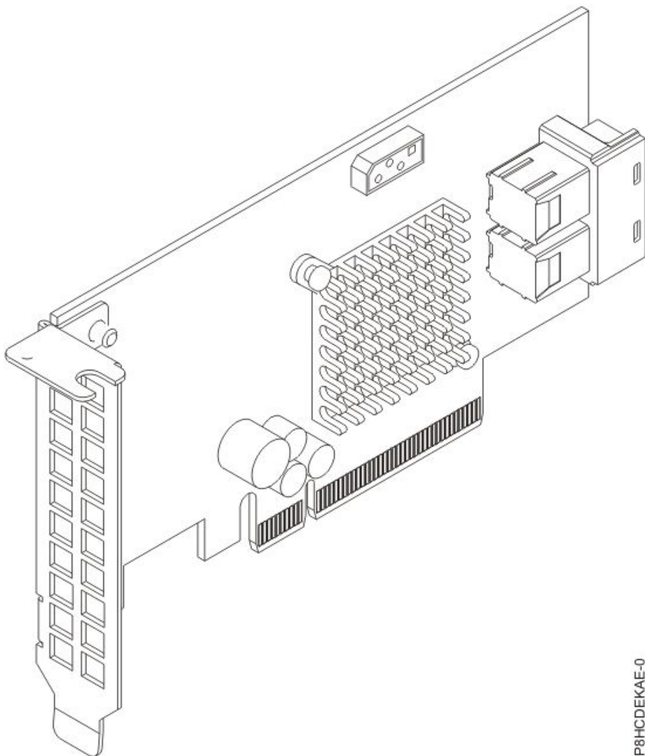
Figure 33. Broadcom (LSI) MegaRAID 9361-8i SAS3 Controller avec 8 ports internes (mémoire cache de 2 Go) PCIe3.0 x8 avec câbles
