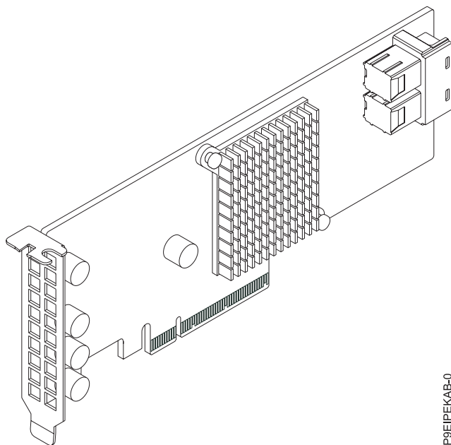
Figure 43. SMC AOC-K-S3008L-L8i 12 Gbps SAS3/RAID 0,1 et 10 PCIe3.0 x8 LP avec câbles
