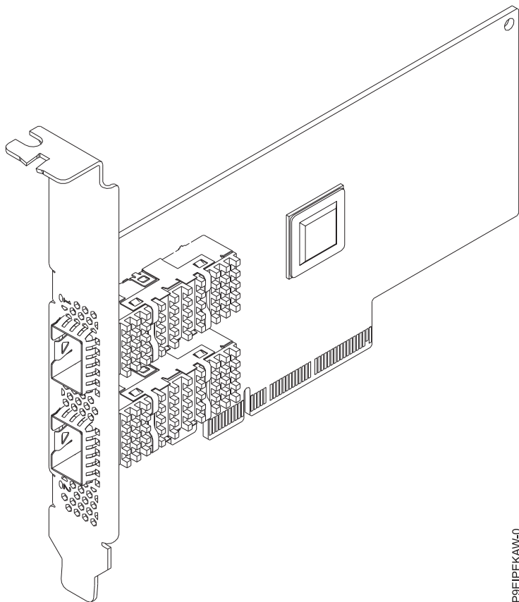
Figure 40. Carte Mellanox MCX414A-BCAT ConnectX-3 Pro EN double port 40/56 GbE PCIe3.0 x8 LP
