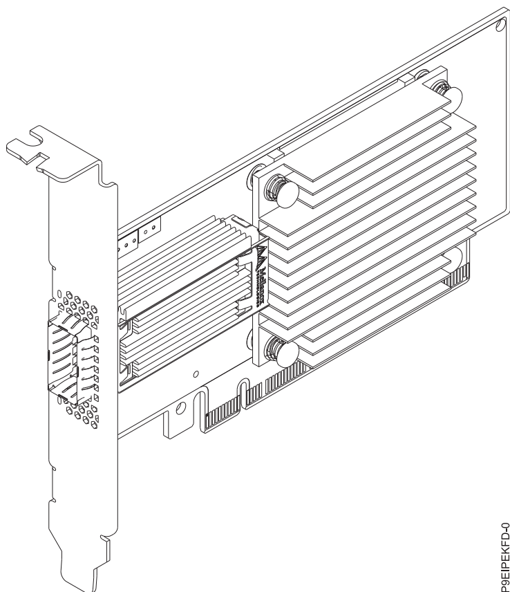
Figure 45. Carte Mellanox MCX555A-ECAT ConnectX-5 VPI EDR InfiniBand 100 Go/s et 100 GbE un port QSFP28 PCIe3.0 x16 LP
