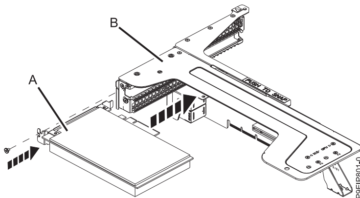
Figure 56. Insertion d'une carte dans la position 2 du connecteur de bus PCIe
