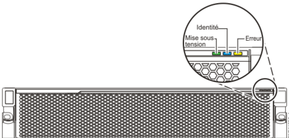
Figure 34. Voyants avant avec panneau en place
