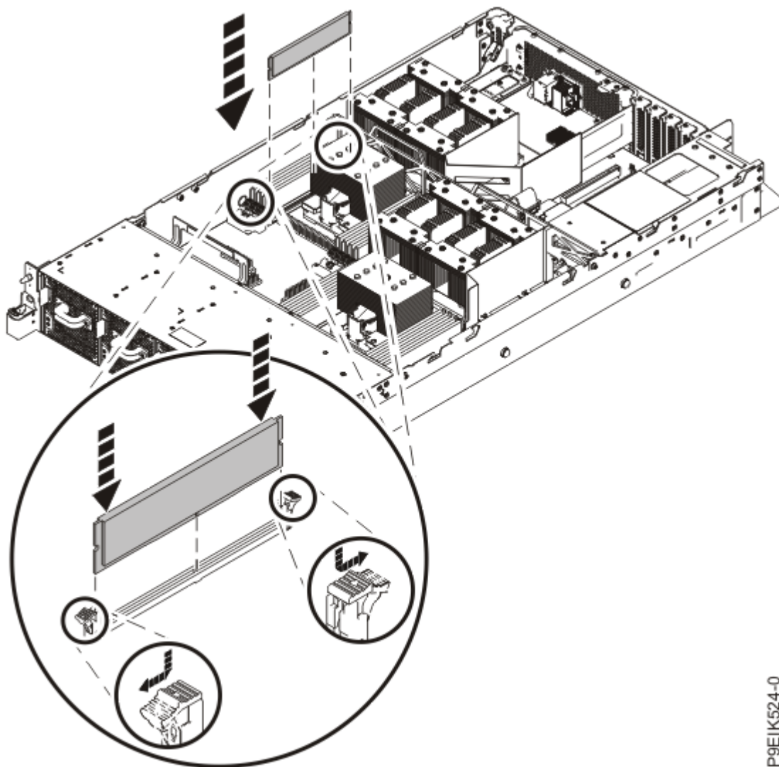
Figure 10. Installation de modules de mémoire
