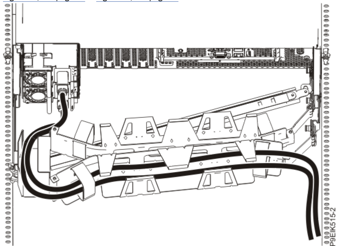
Figure 47. Routage de la boucle du cordon d'alimentation dans le bras de routage des câbles
