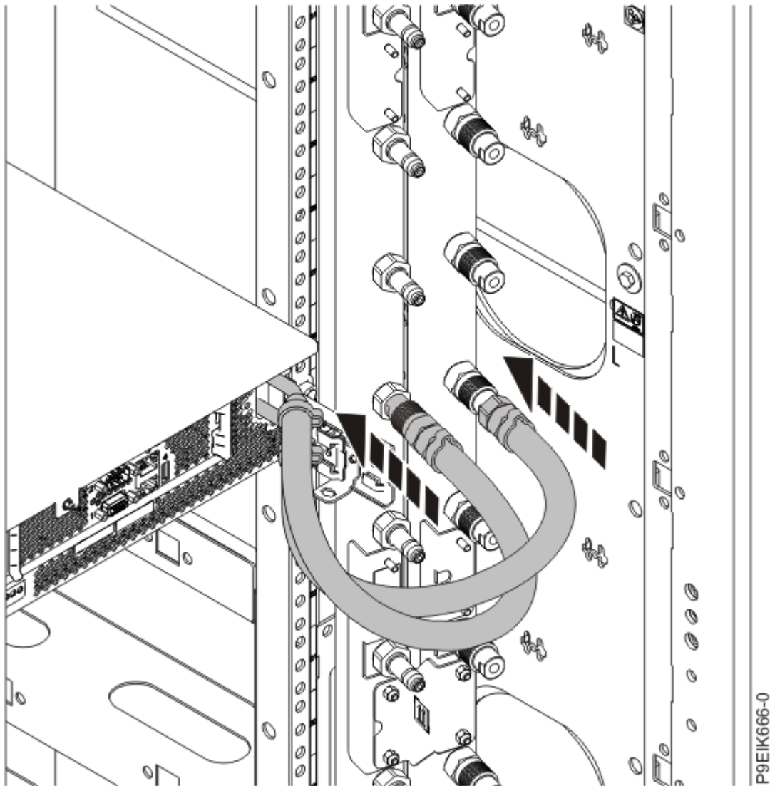
Figure 3. Raccordement des conduites d'eau
