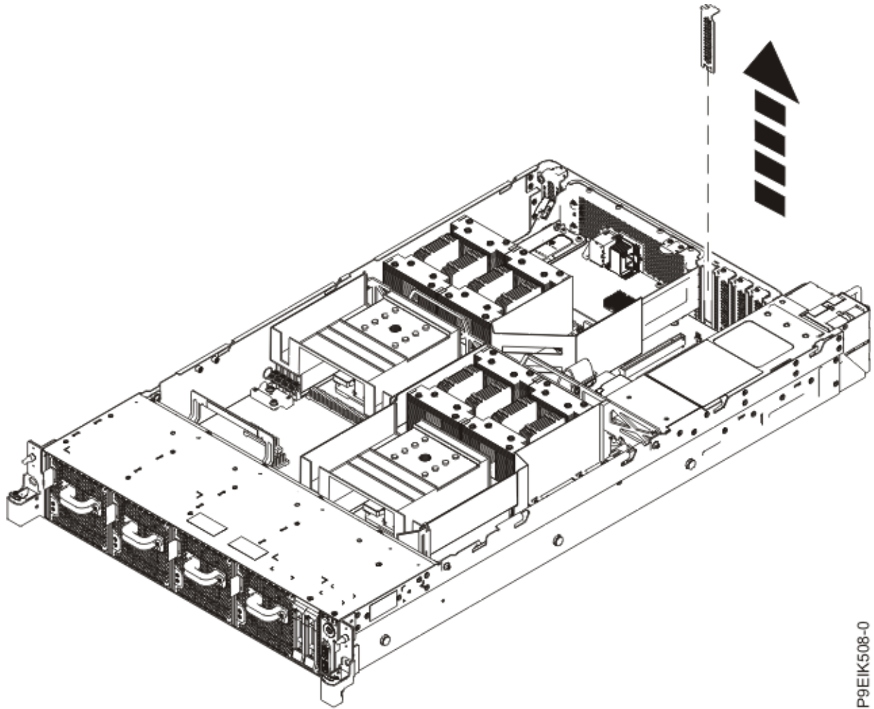
Figure 32. Retrait du capot de l'emplacement PCIe
