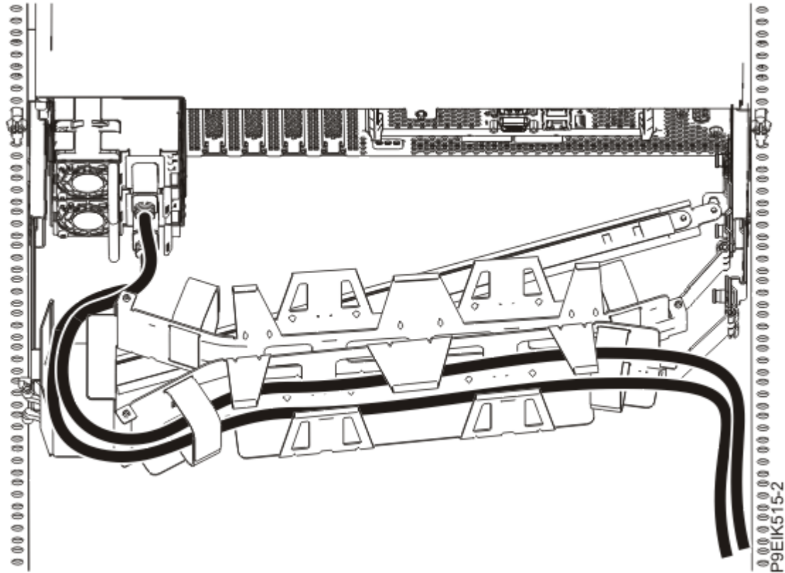
Figure 51. Routage de la boucle du cordon d'alimentation dans le bras de routage des câbles
