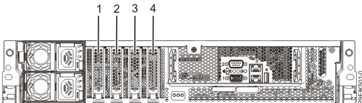
Figure 31. Vue arrière d'un système avec emplacements PCIe indiqués
