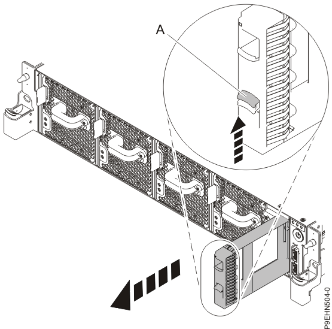
Figure 5. Retrait d'un obturateur d'unité de disque d'un système
