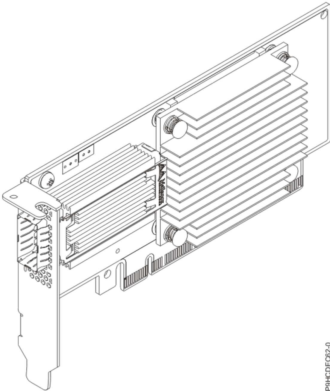
Figure 21. Carte PCIe4 x16 1 port EDR 100 GB IB ConnectX-5 compatible CAPI
