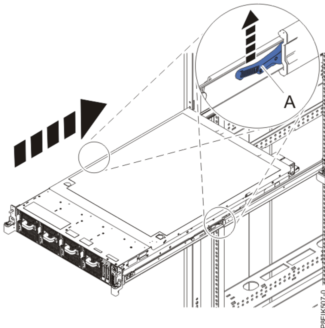
Figure 45. Mise en position de fonctionnement du système
