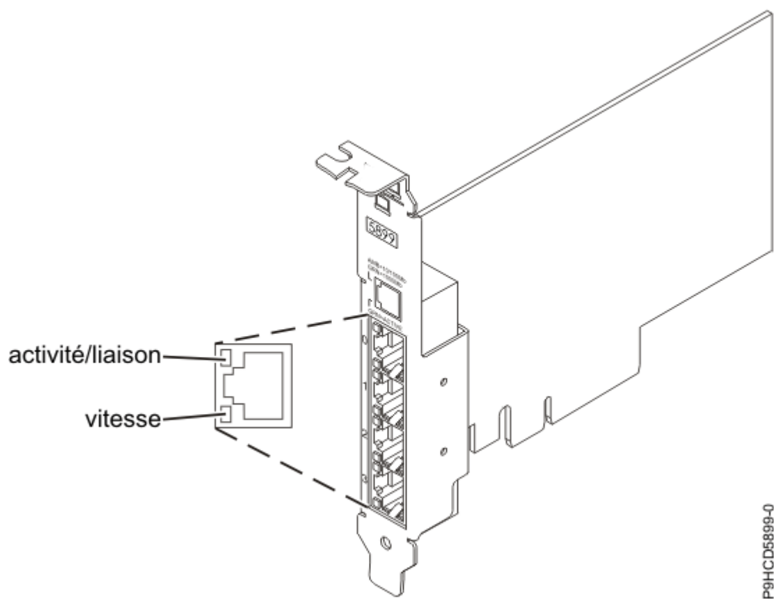
Figure 27. Carte PCIe2 4 ports 1 GbE FC 5899 et FC EL4L
