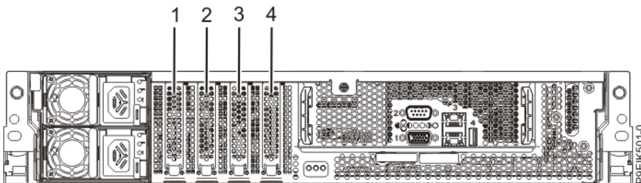
Figure 12. Vue arrière d'un système avec emplacements PCIe indiqués
