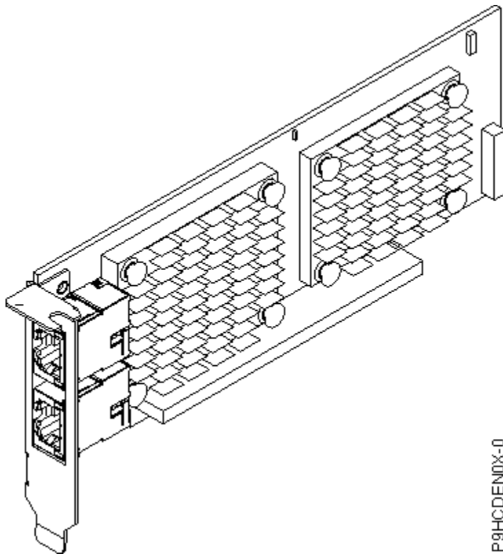
Figure 24. Carte PCIe2 LP 2 ports 10 GbE BaseT RJ45 (FC EL3Z ou FC EN0X)
