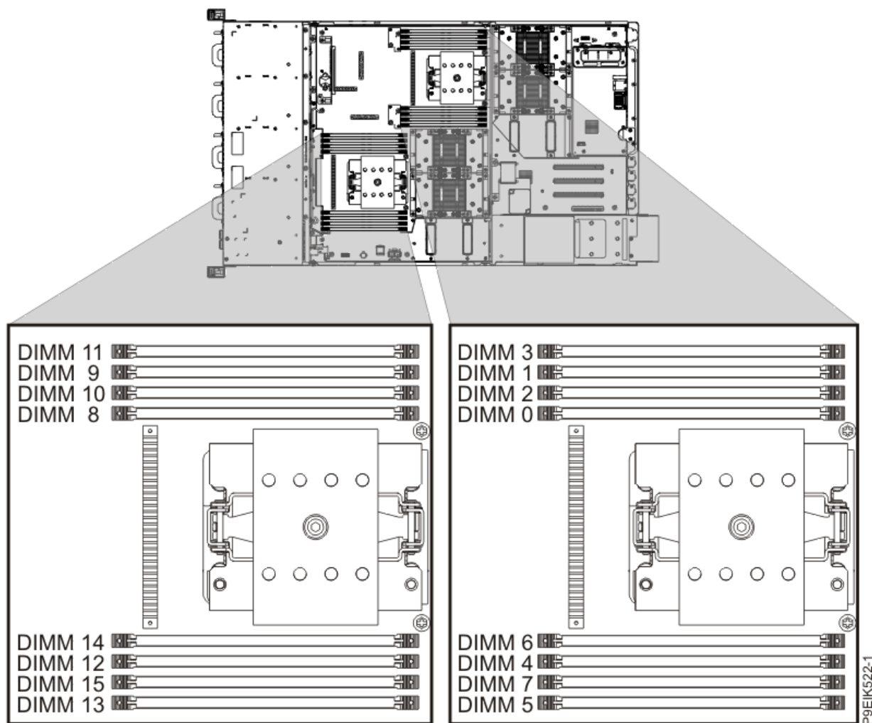
Figure 8. Emplacement des modules de mémoire
