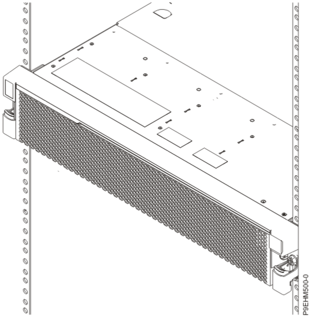
Figure 2. Installation du serveur dans l'armoire
