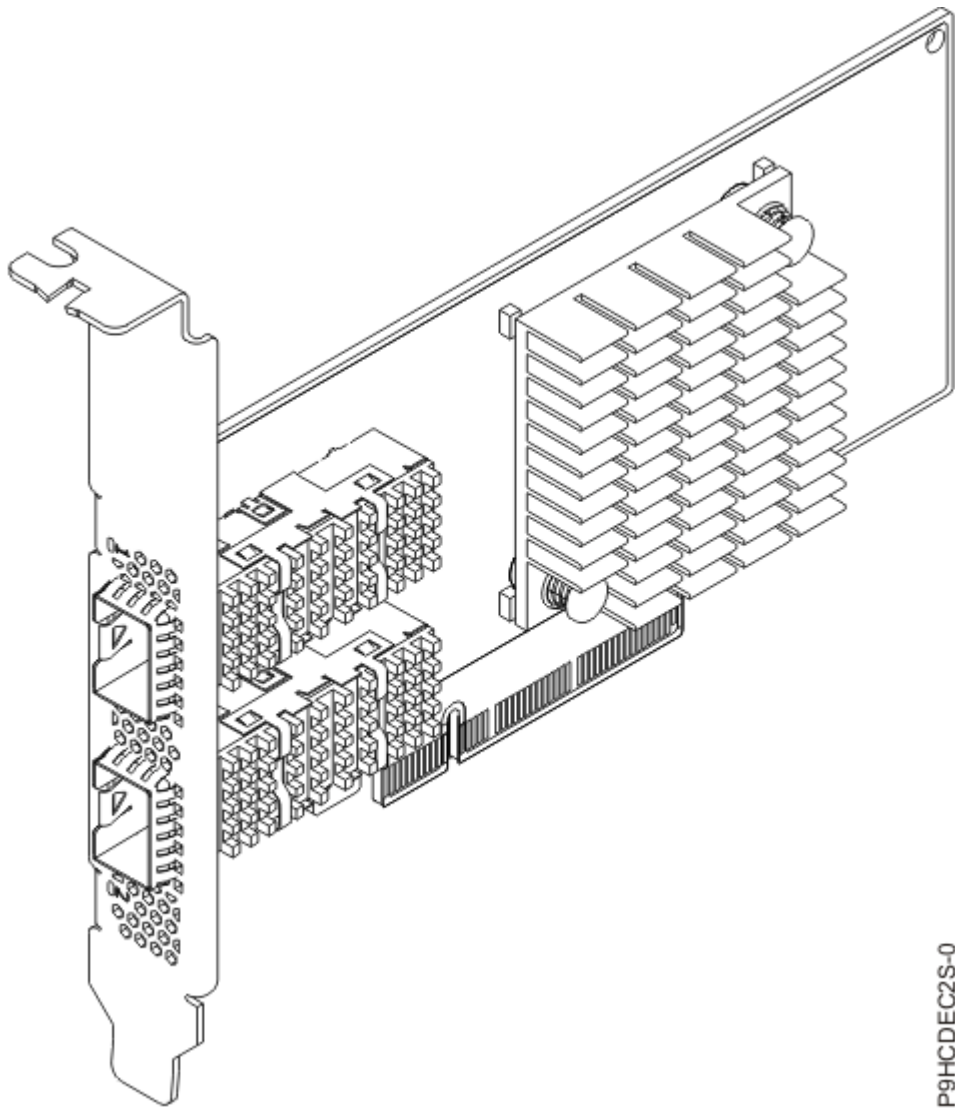
Figure 14. Carte PCIe3 2 ports 10 Gb NIC avec RoCE SR/Cu (FC EC2S)
