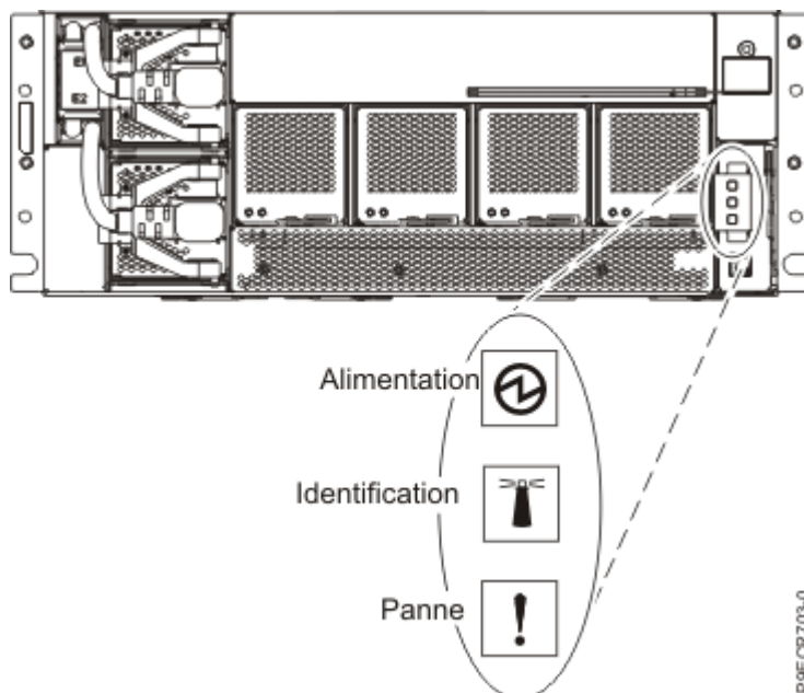
Figure 7. Voyant d'alimentation avant du tiroir d'extension EMX0 PCIe3
