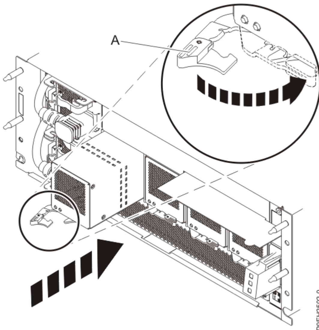
Figure 5. Installation d'un ventilateur dans le tiroir d'extension EMX0 PCIe3
