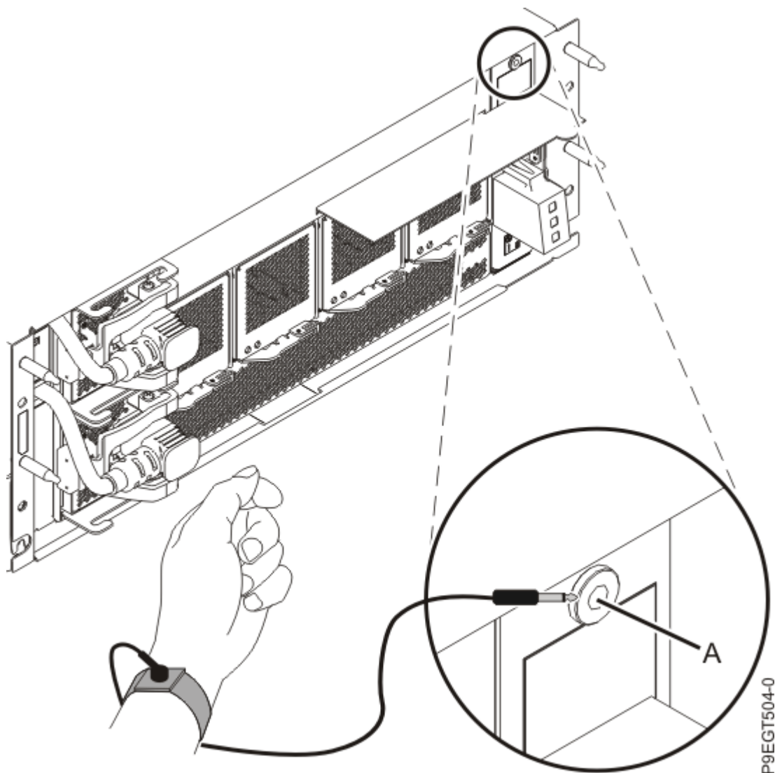
Figure 2. Fixation du bracelet antistatique à la prise de décharge électrostatique
