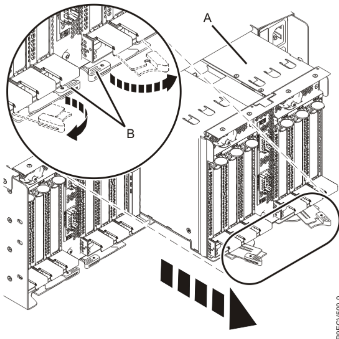
Figure 4. Ouverture des taquets de déverrouillage
