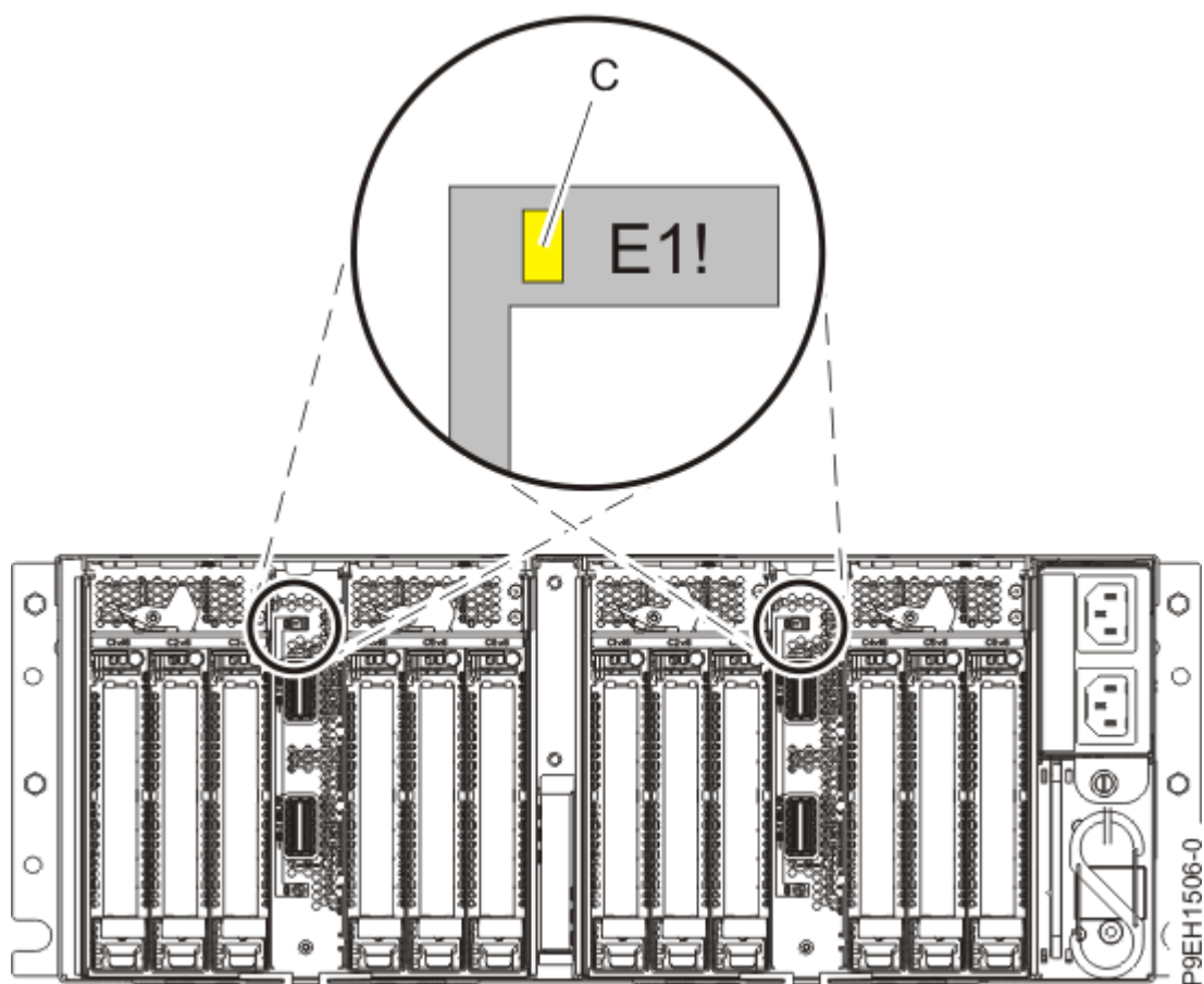
Figure 3. Voyant de régulateur de tension
