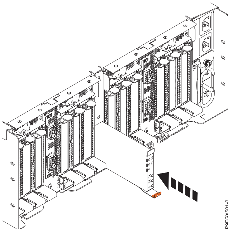
Figure 4. Remise en place du conduit fibre optique dans le tiroir d'extension EMX0 PCIe3
