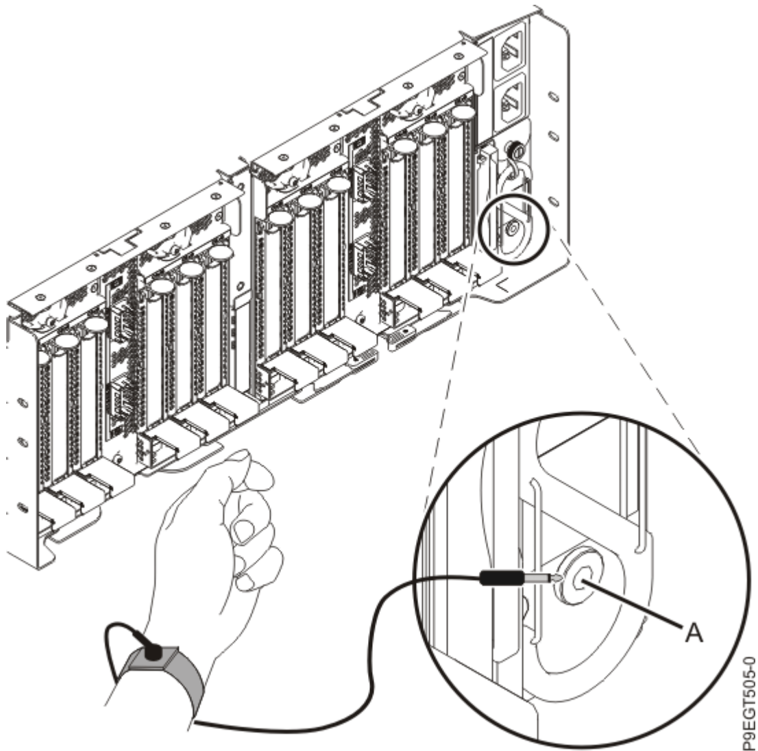
Figure 1. Emplacement de la broche de décharge électrostatique à l'arrière du tiroir d'extension MX0 PCIe3
