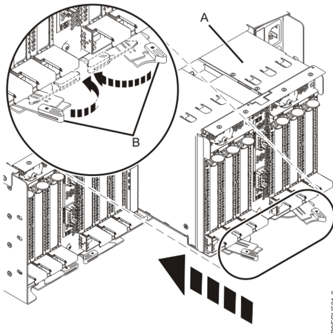
Figure 4. Fermeture des loquets de déverrouillage du module de sortance à 6 emplacements PCIe3
