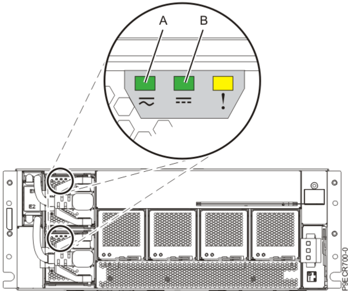
Figure 7. Vérification des voyants d'alimentation électrique en position allumée
