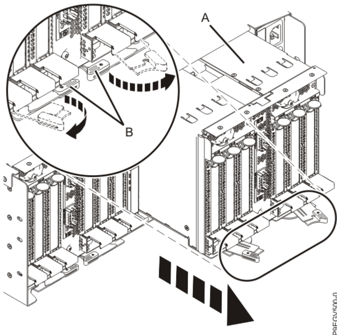
Figure 10. Ouverture des loquets de déverrouillage
