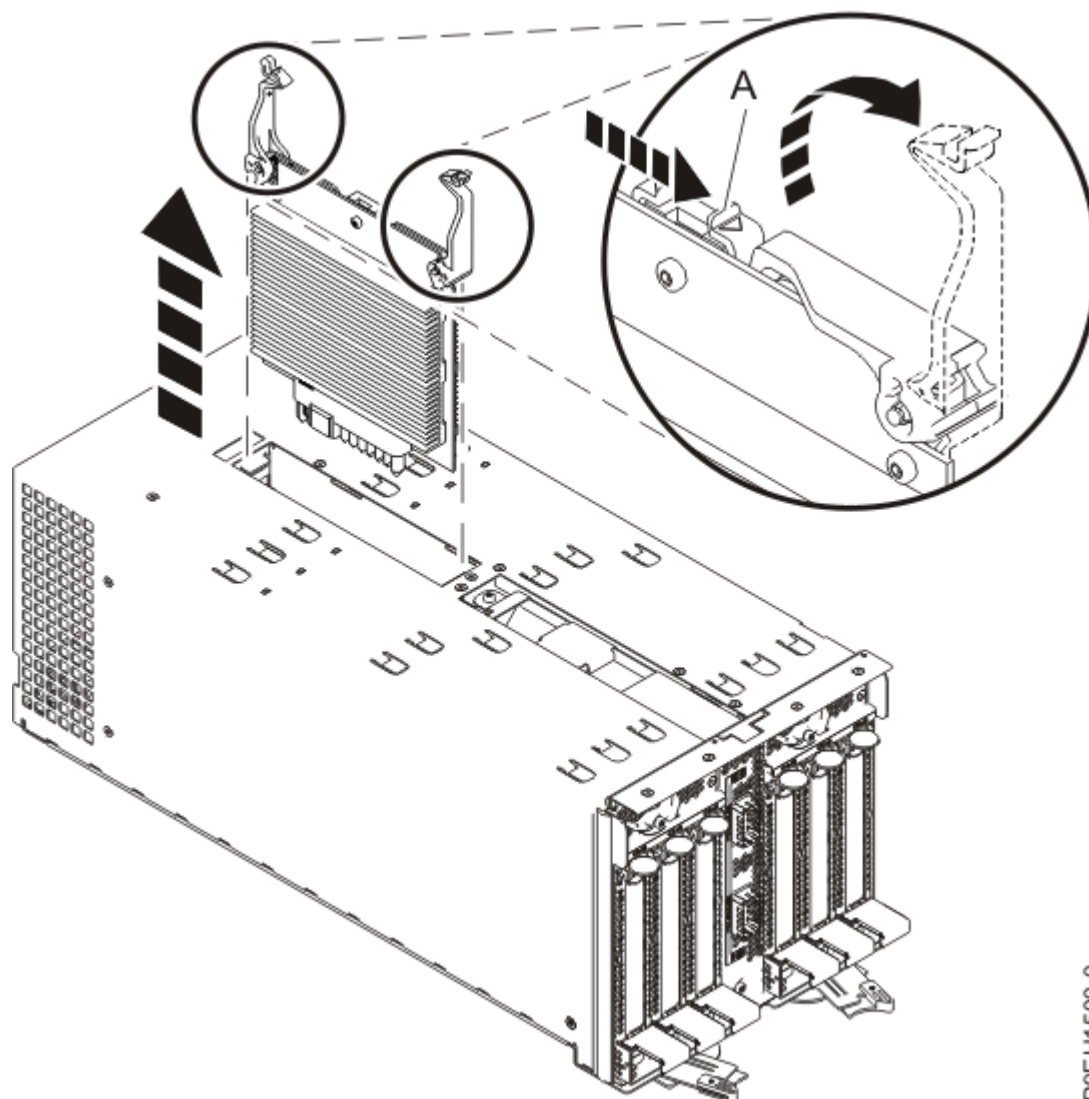
Figure 11. Retrait du régulateur de tension
