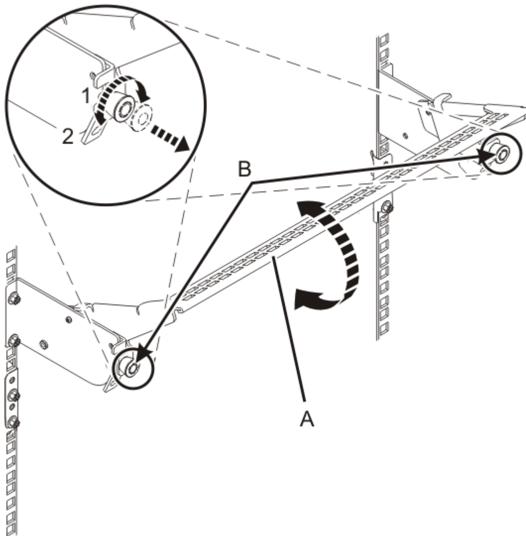
Figure 5. Placement du crochet de routage des câbles en position de fonctionnement
