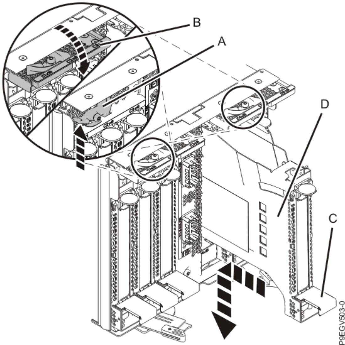
Figure 13. Installation d'une cassette de cartes PCIe
