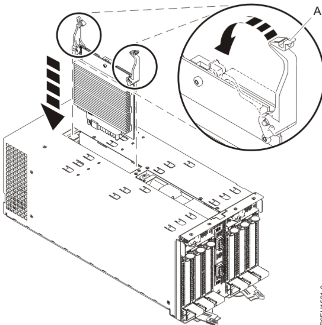
Figure 14. Remise en place du régulateur de tension
