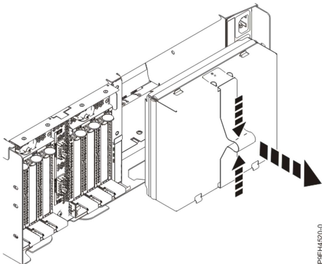
Figure 3. Retrait de l'élément de remplissage
