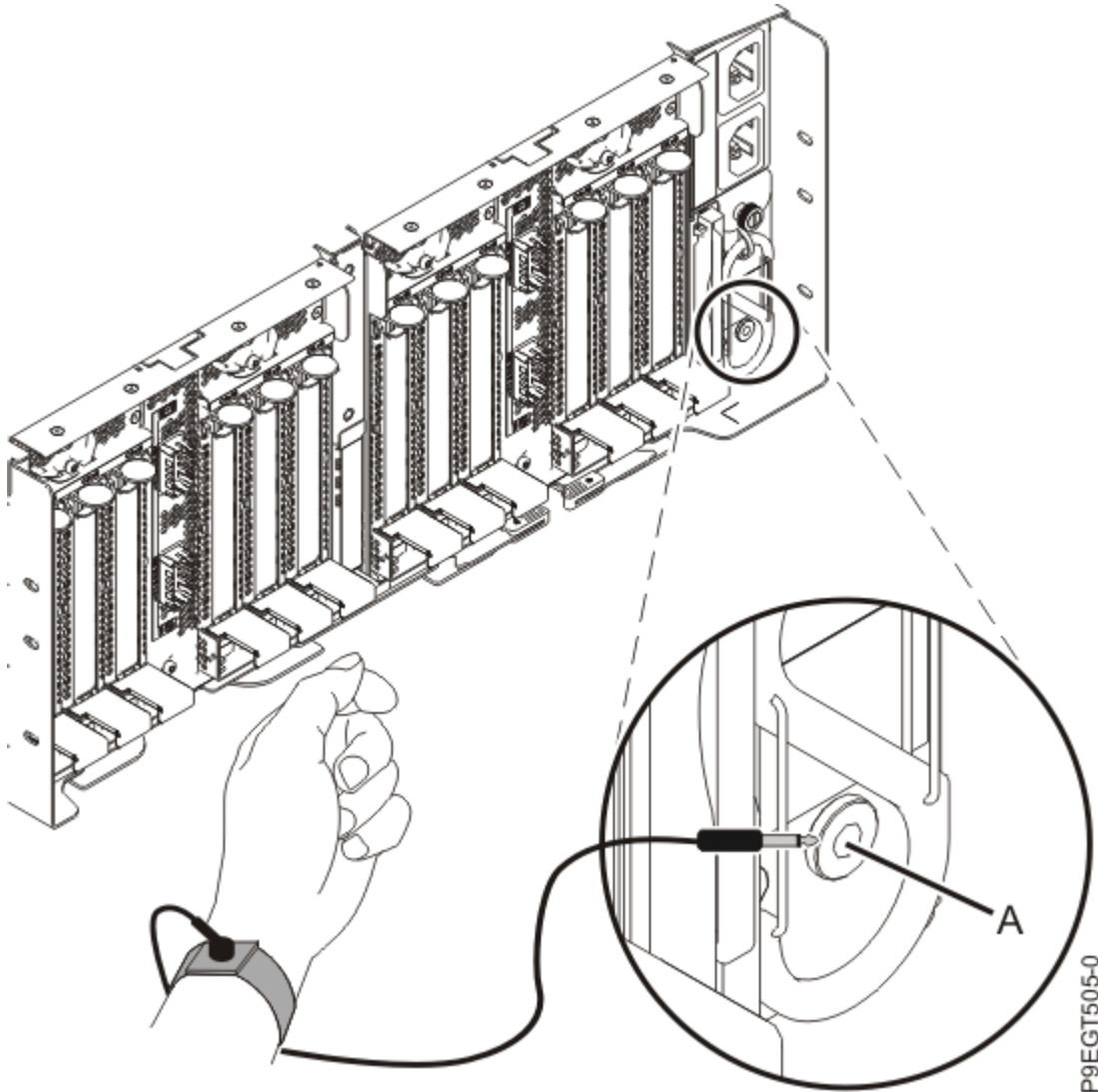
Figure 18. Emplacement de la broche de décharge électrostatique à l'arrière du tiroir d'extension EMX0 PCIe3
