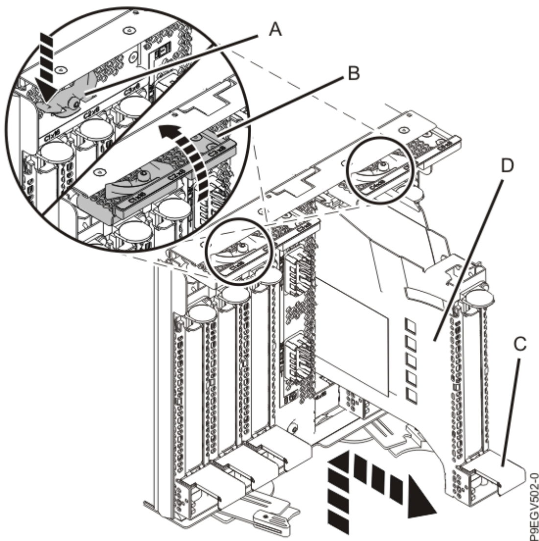
Figure 12. Retrait d'une cassette de cartes PCIe
