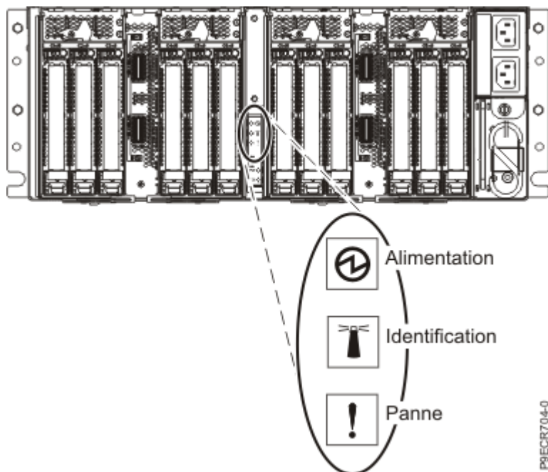
Figure 24. Voyant d'alimentation arrière du tiroir d'extension EMX0 PCIe3
