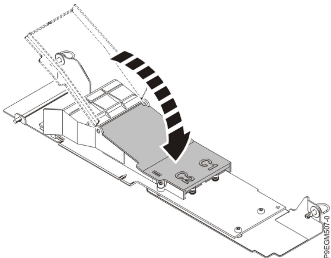
Figure 7. Fermeture du capot noir de la carte porteuse NVMe M.2
