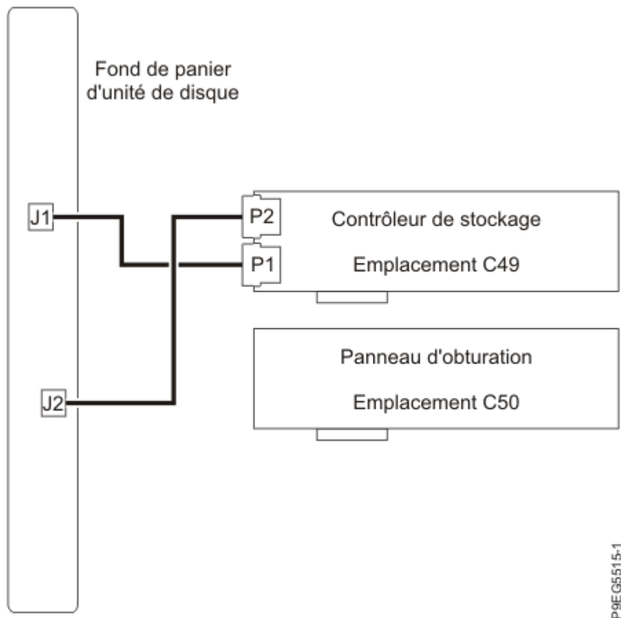
Figure 5. Reconnexion du câble SAS dans une configuration de stockage de base
