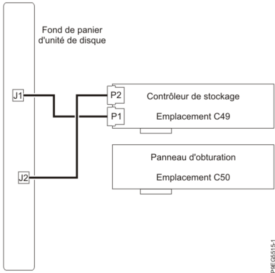
Figure 24. Reconnexion du câble SAS dans une configuration de stockage de base
