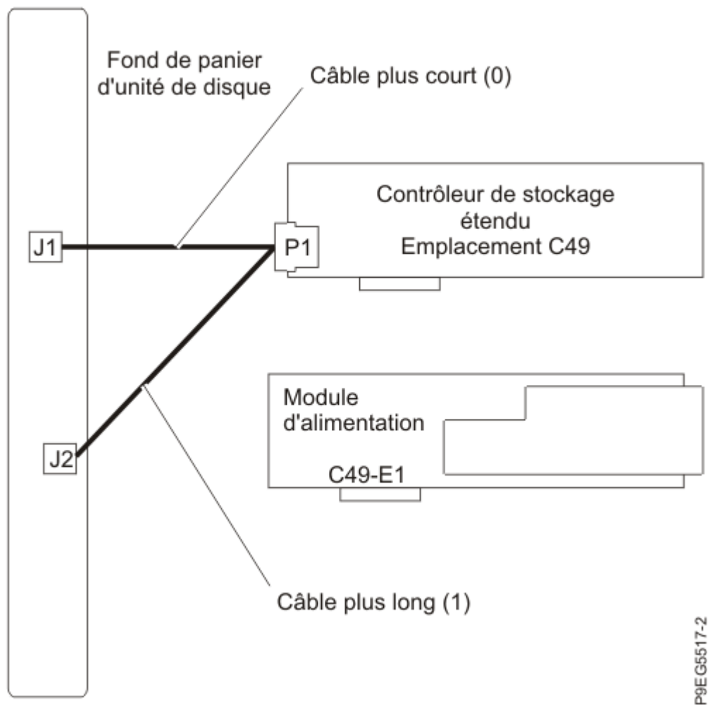
Figure 26. Reconnexion du câble SAS en "Y" dans une configuration de contrôleur de stockage hautes performances
