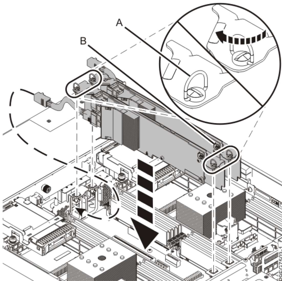
Figure 27. Remise en place de l'adaptateur SAS RAID
