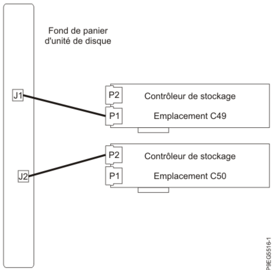
Figure 6. Reconnexion du câble SAS dans une configuration de disque partagé
