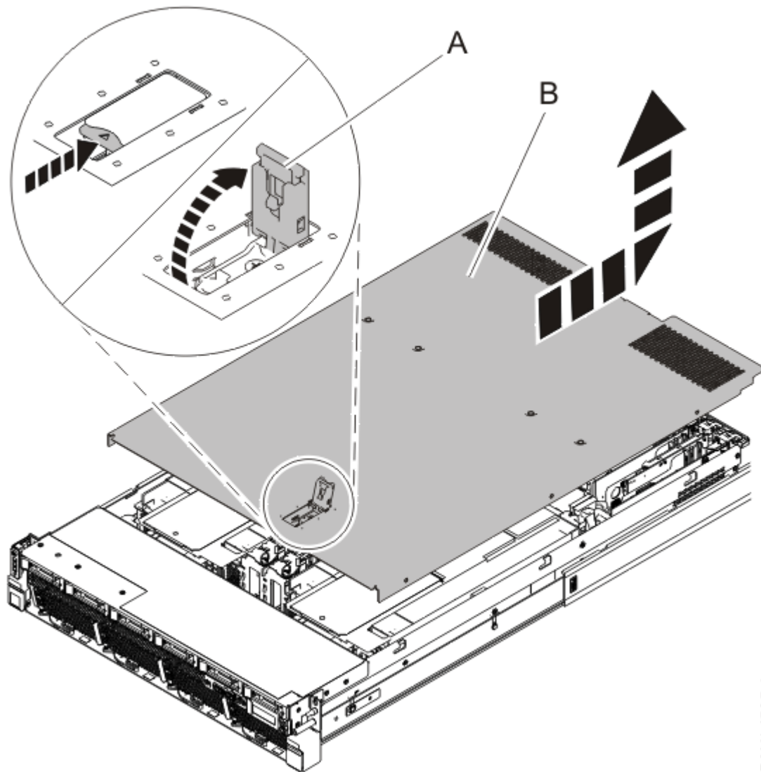
Figure 18. Retrait du capot d'accès
