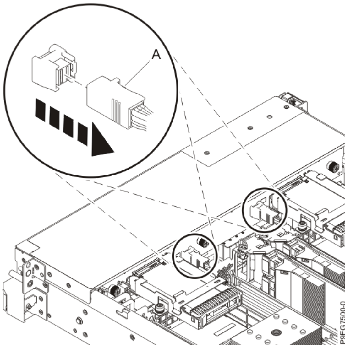
Figure 20. Déconnexion des câbles SAS avant
