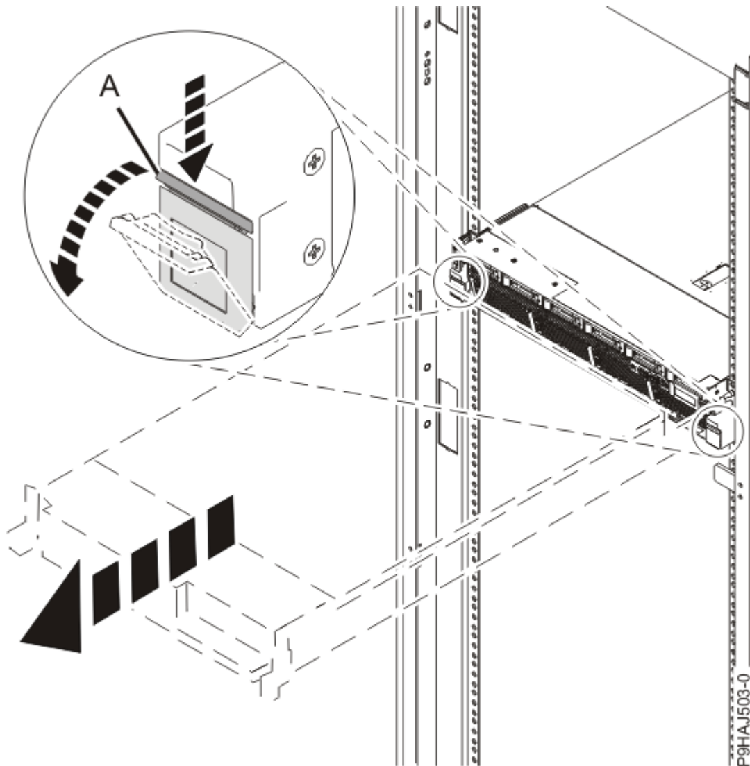
Figure 17. Déblocage des loquets latéraux
