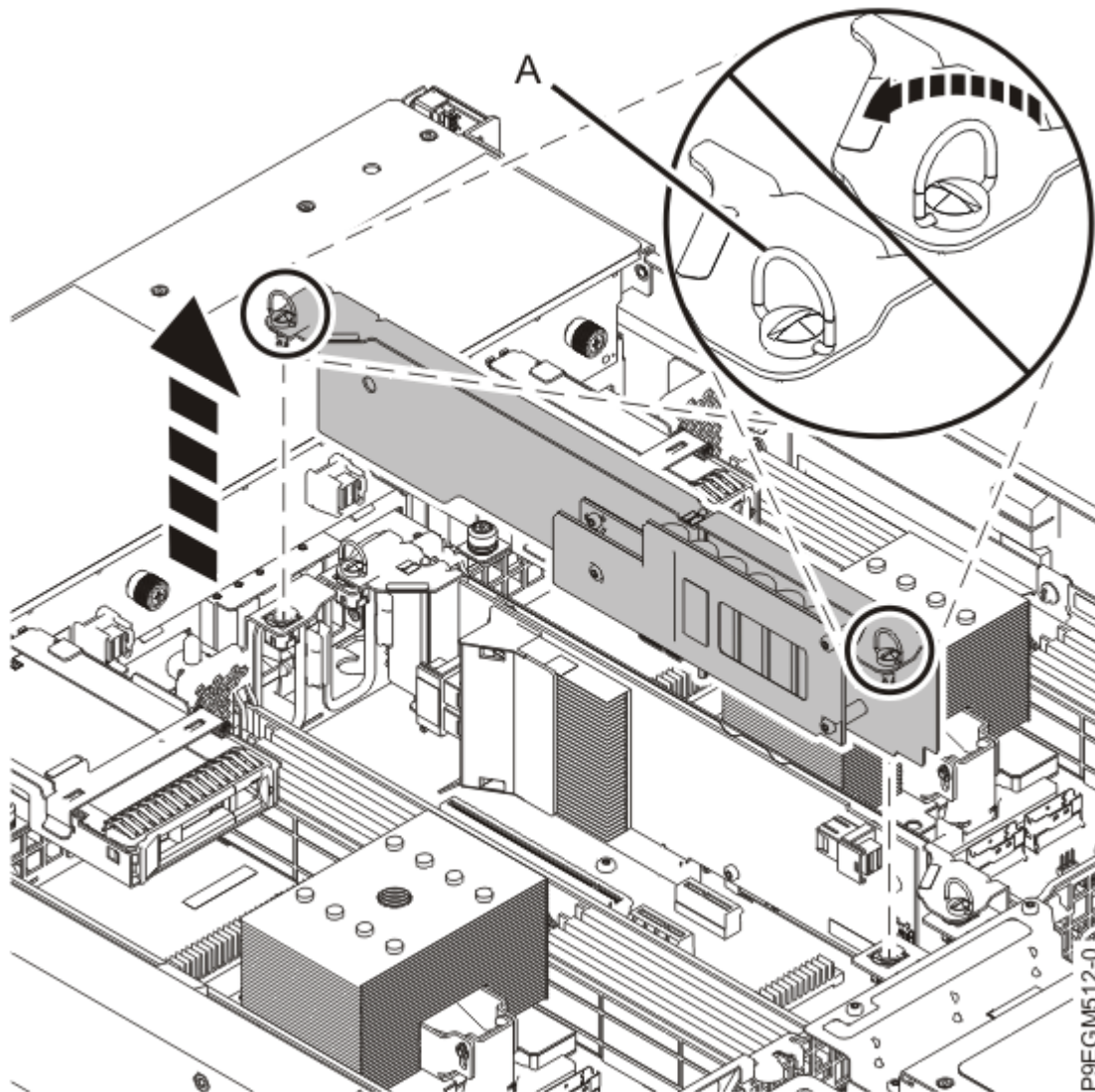
Figure 23. Retrait du module d'alimentation de secours
