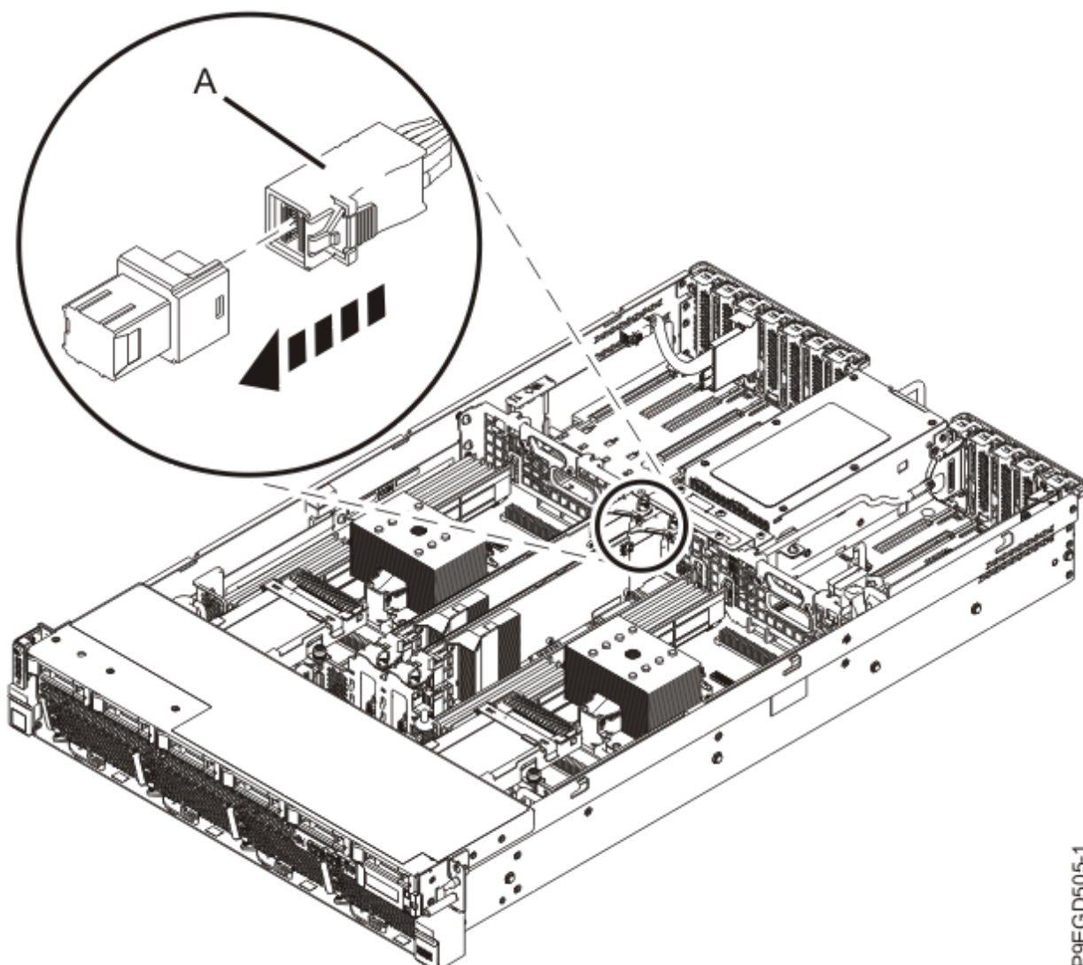
Figure 9. Reconnexion des câbles SAS arrière
