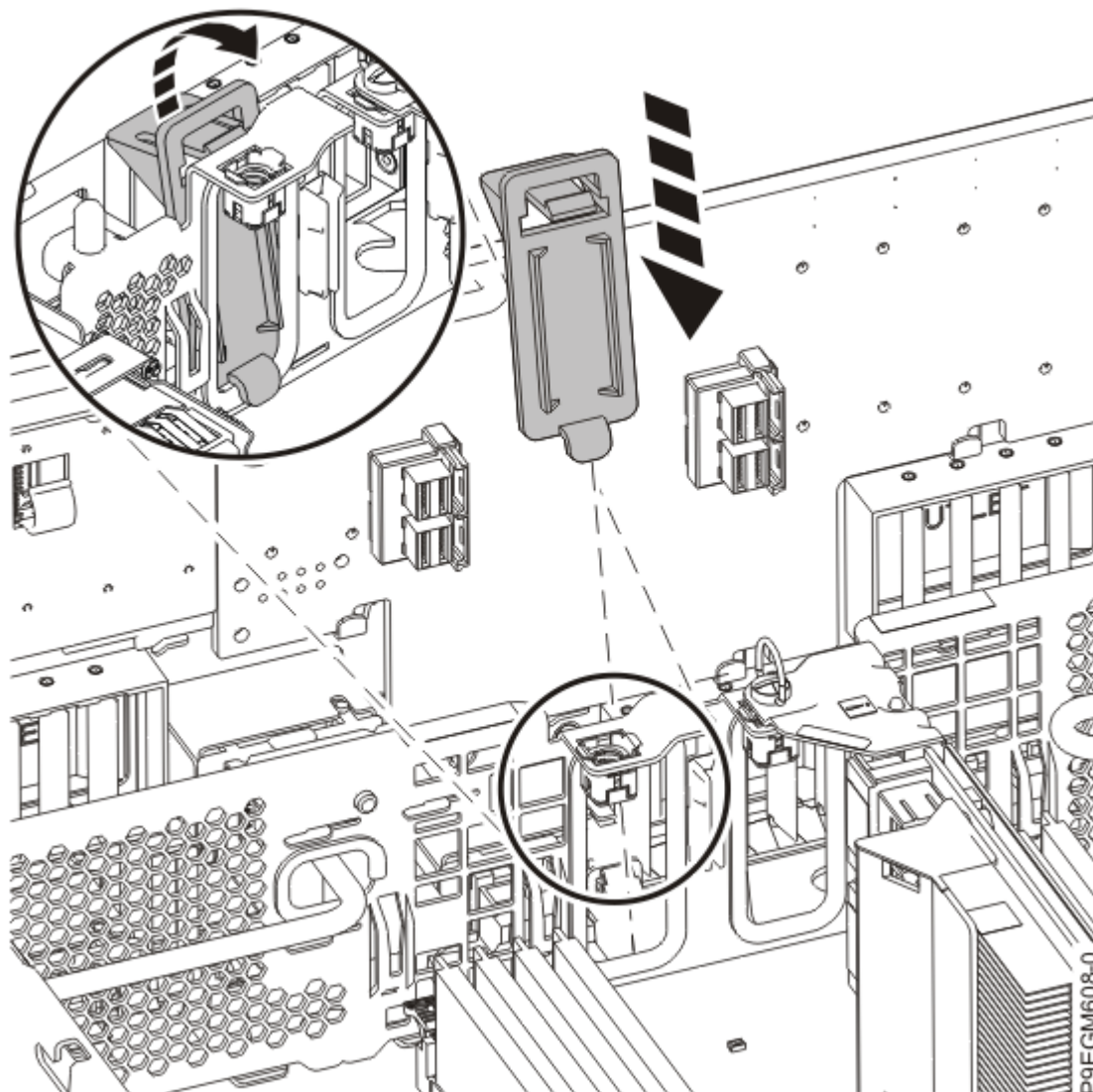
Figure 30. Installation du panneau d'obturation à ergots
