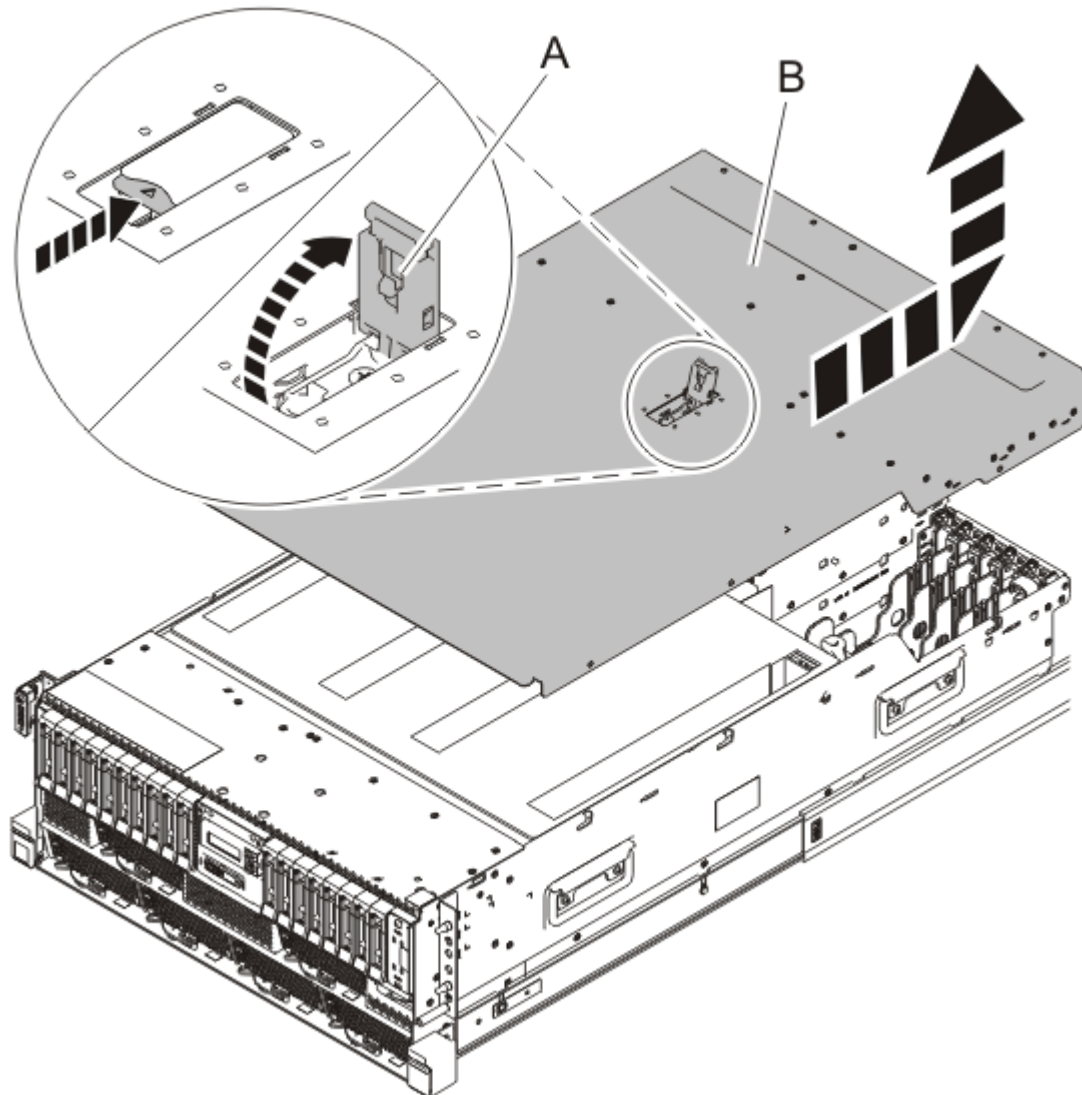
Figure 22. Retrait du capot d'accès d'un système monté en armoire
