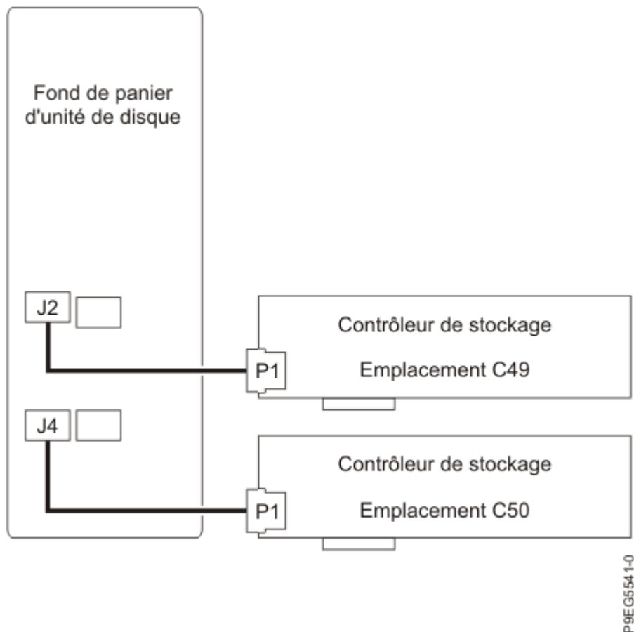
Figure 10. Reconnexion du câble SAS dans la configuration de fonction étendue 12 unités
