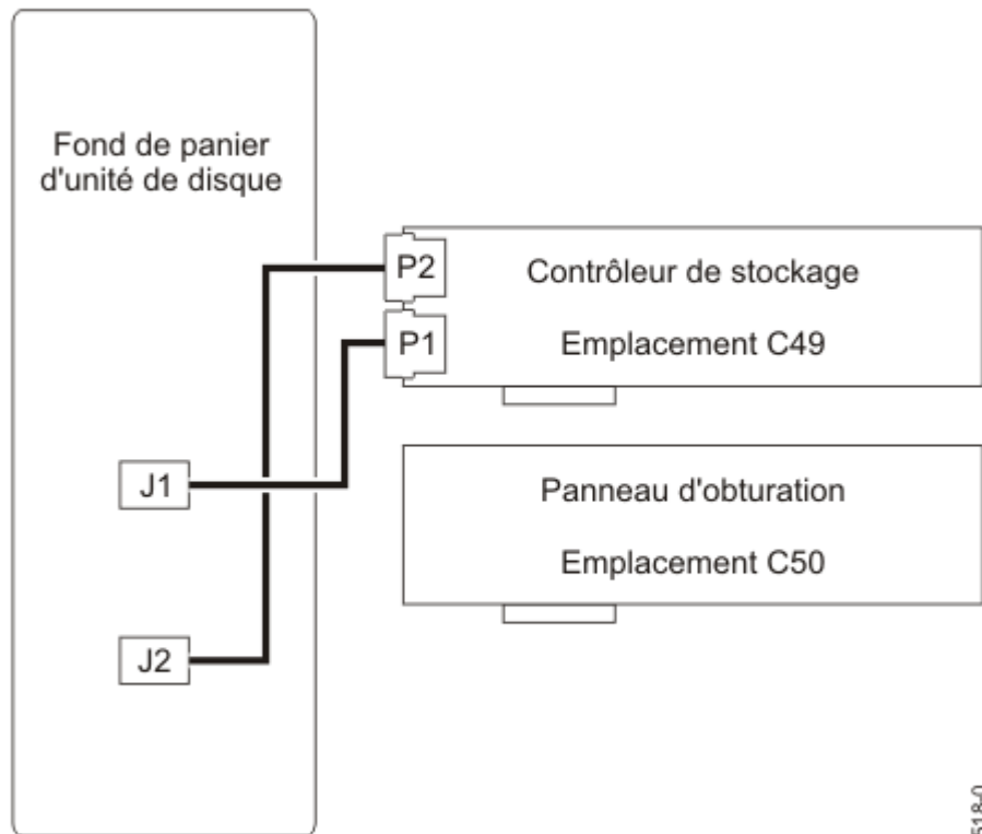
Figure 33. Reconnexion du câble SAS dans une configuration de stockage de base
