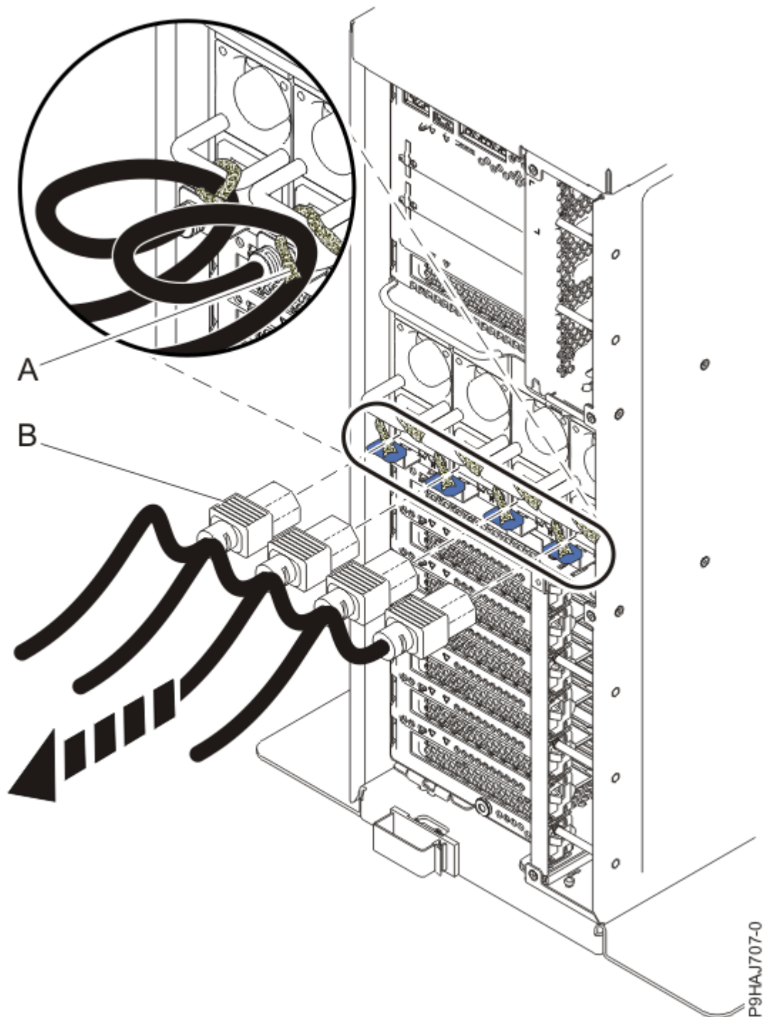
Figure 24. Retrait des cordons d'alimentation d'un serveur autonome
