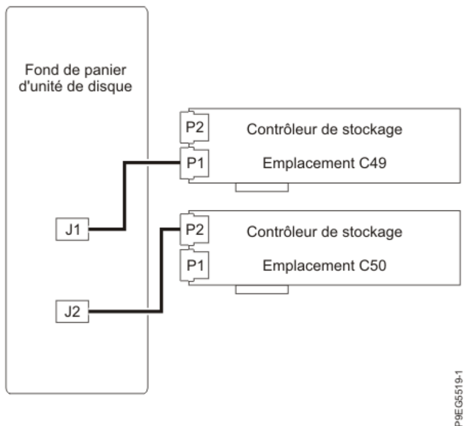
Figure 9. Reconnexion du câble SAS dans une configuration de disque partagé
