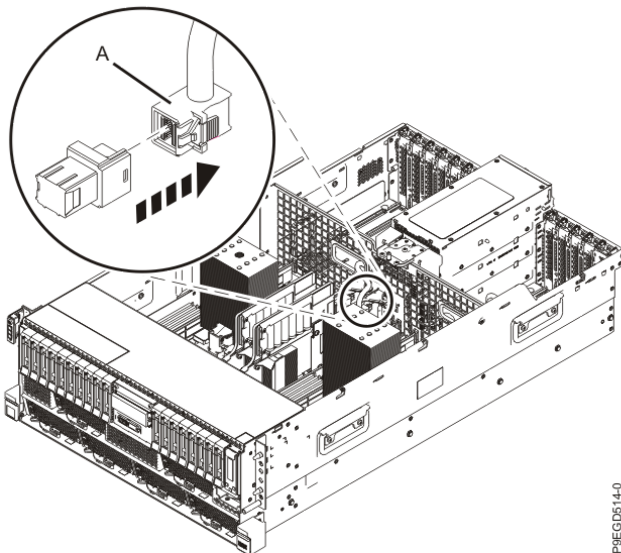
Figure 31. Débranchement des câbles SAS arrière de la carte interne RAID SAS dans les emplacements P1-C49 et P-C50
