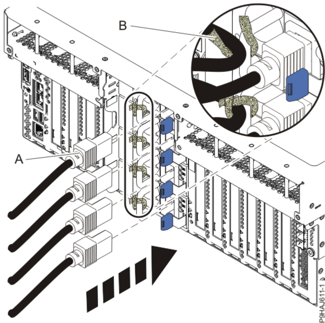
Figure 21. Connexion des cordons d'alimentation à un système monté en armoire
