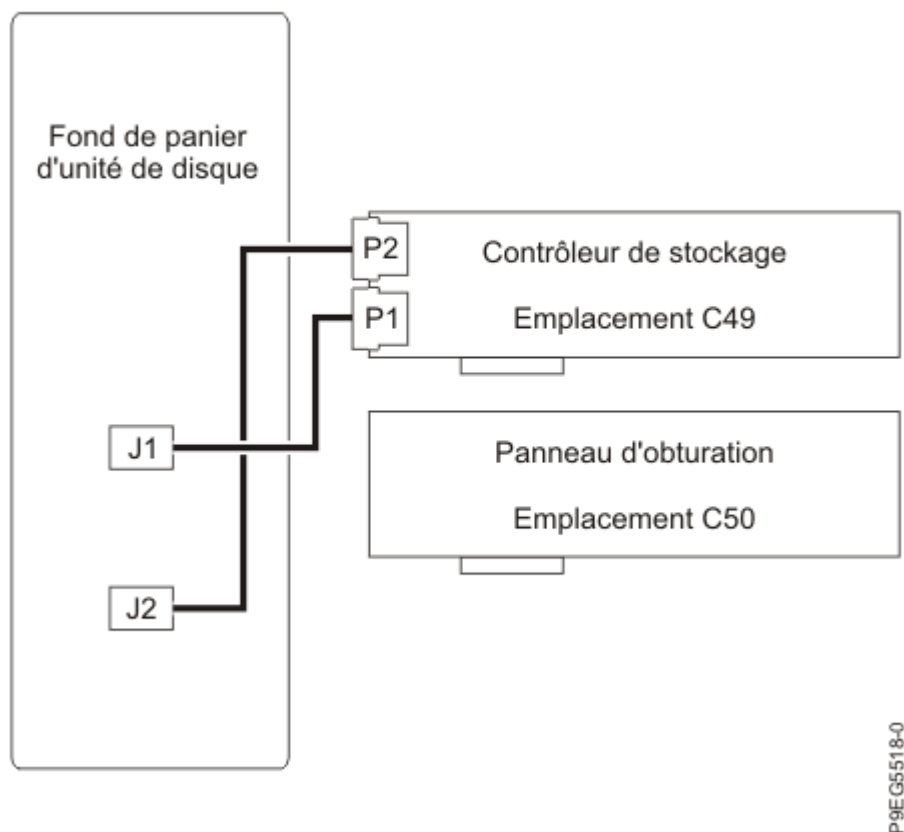
Figure 8. Reconnexion du câble SAS dans une configuration de stockage de base
