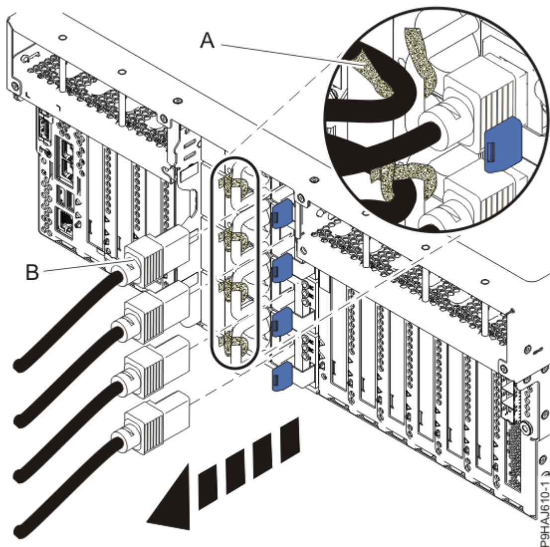
Figure 23. Retrait des cordons d'alimentation d'un serveur monté en armoire
