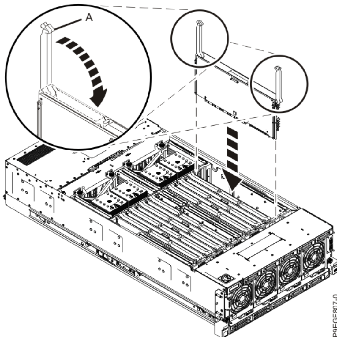
Figure 12. Installation d'une carte d'extension de mémoire
