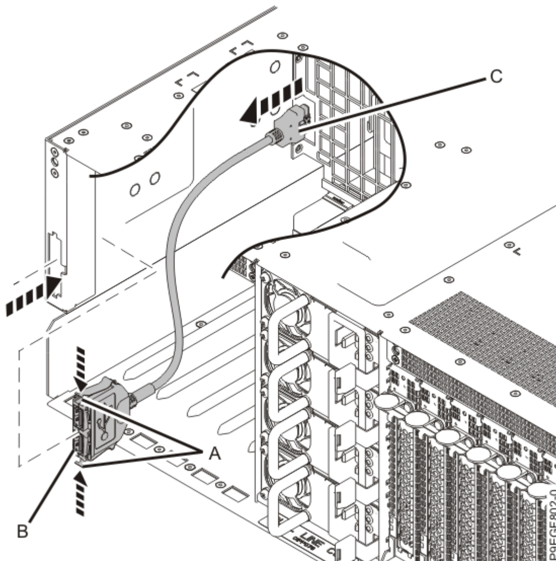
Figure 8. Retrait du connecteur de port USB arrière
