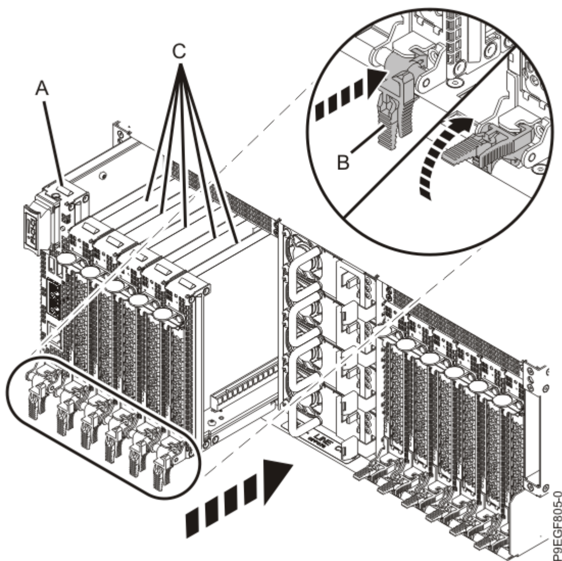
Figure 15. Remise en place de la carte de processeur de service et des cassettes PCIe
