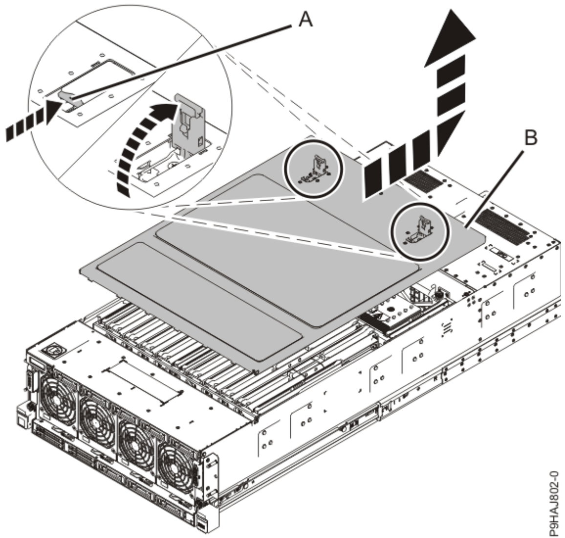
Figure 4. Retrait du capot d'accès
