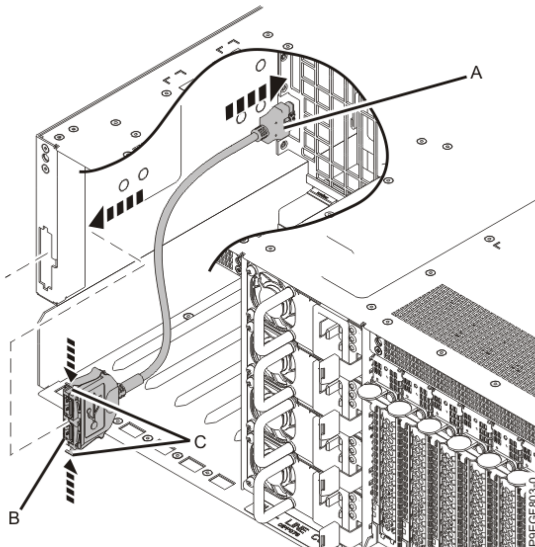
Figure 9. Remise en place du connecteur de port USB arrière
