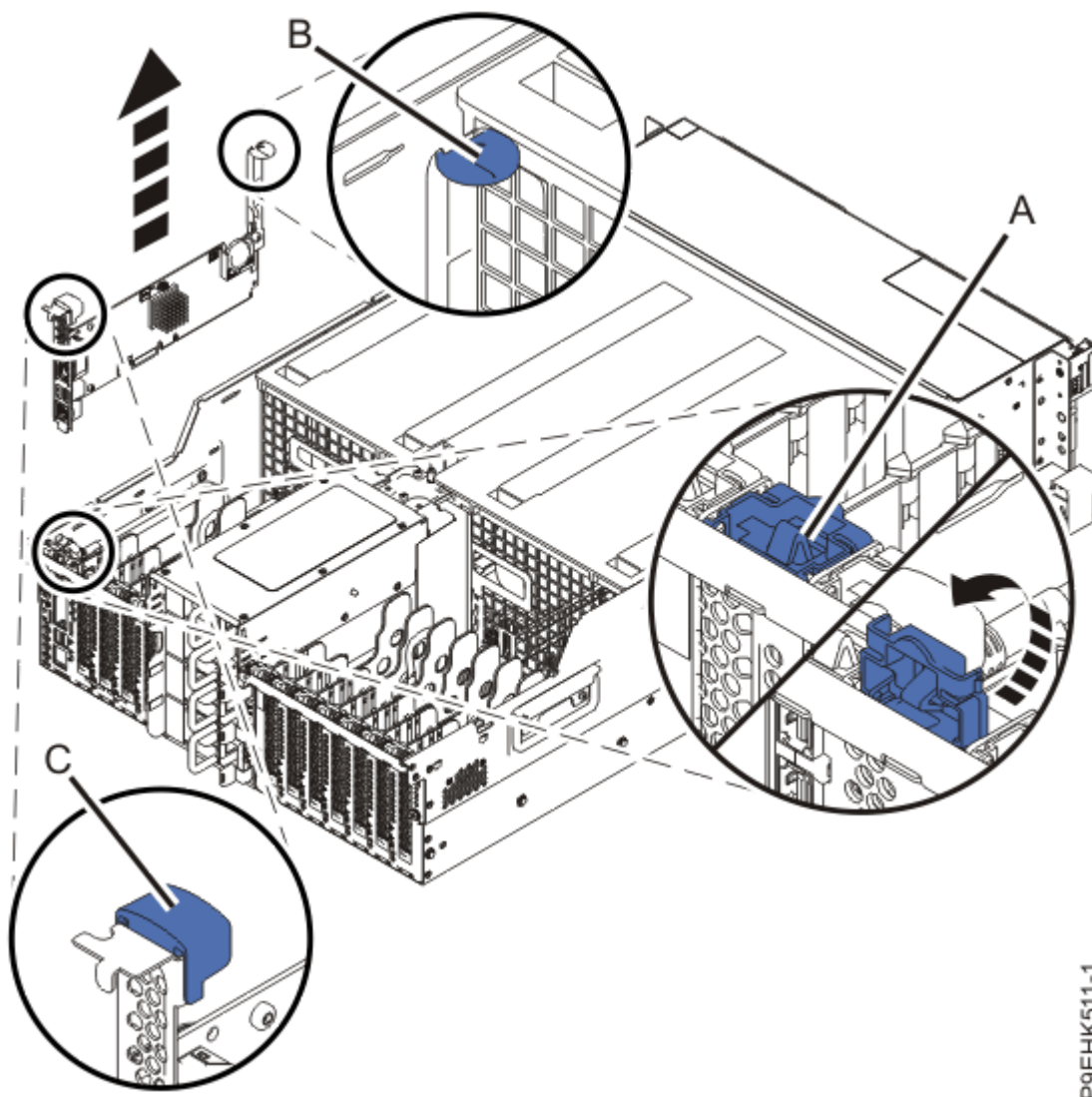
Figure 9. Retrait de la carte de processeur de service
