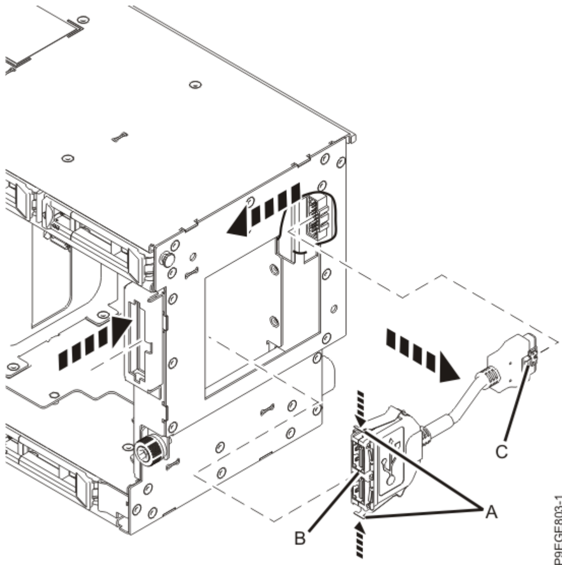
Figure 9. Retrait du connecteur de port USB avant
