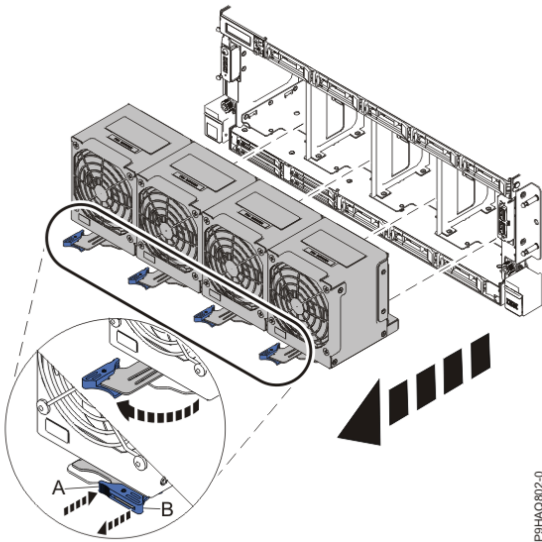
Figure 2. Retrait des ventilateurs
