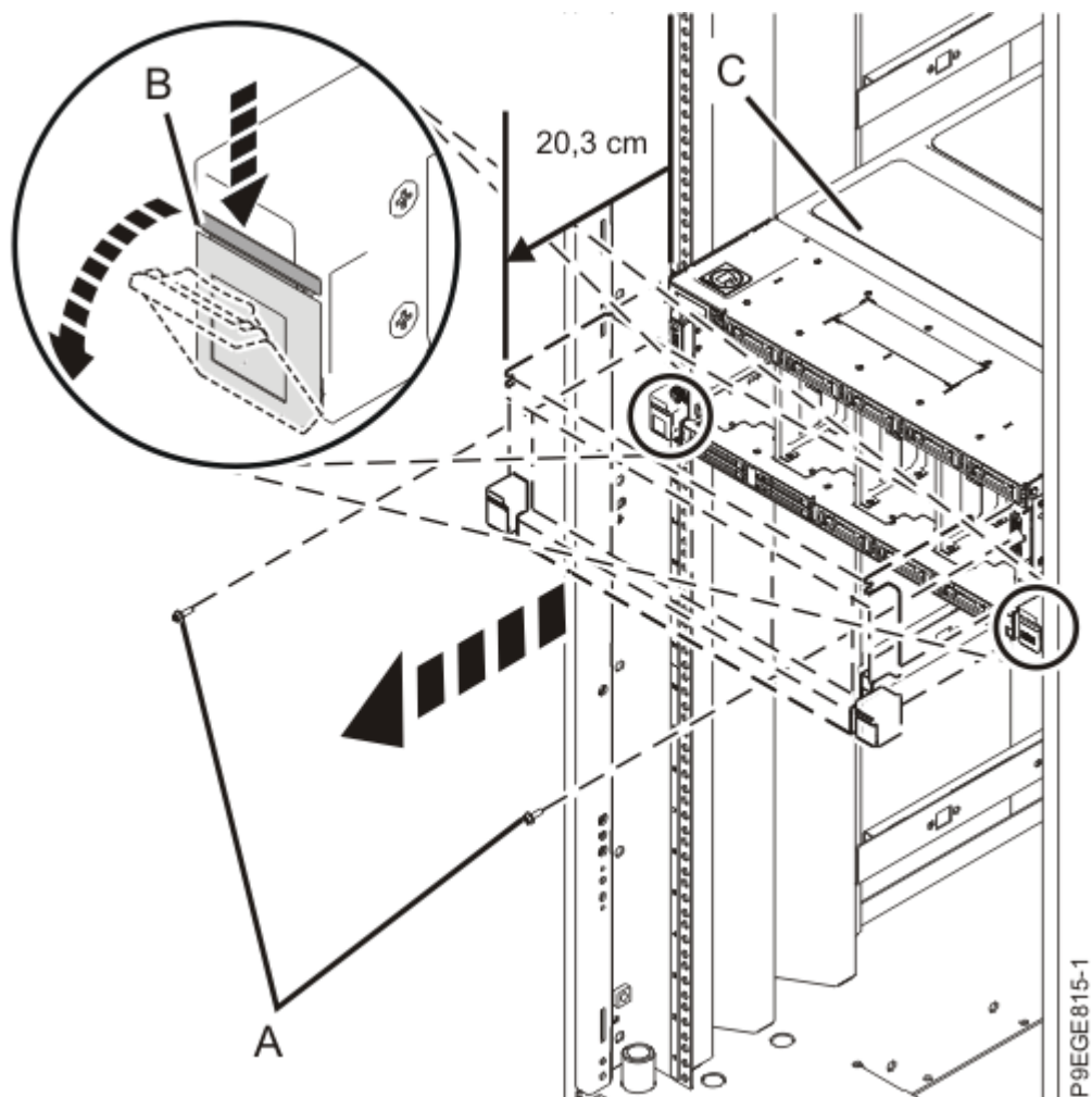
Figure 5. Glissement partiel du système hors de l'armoire
