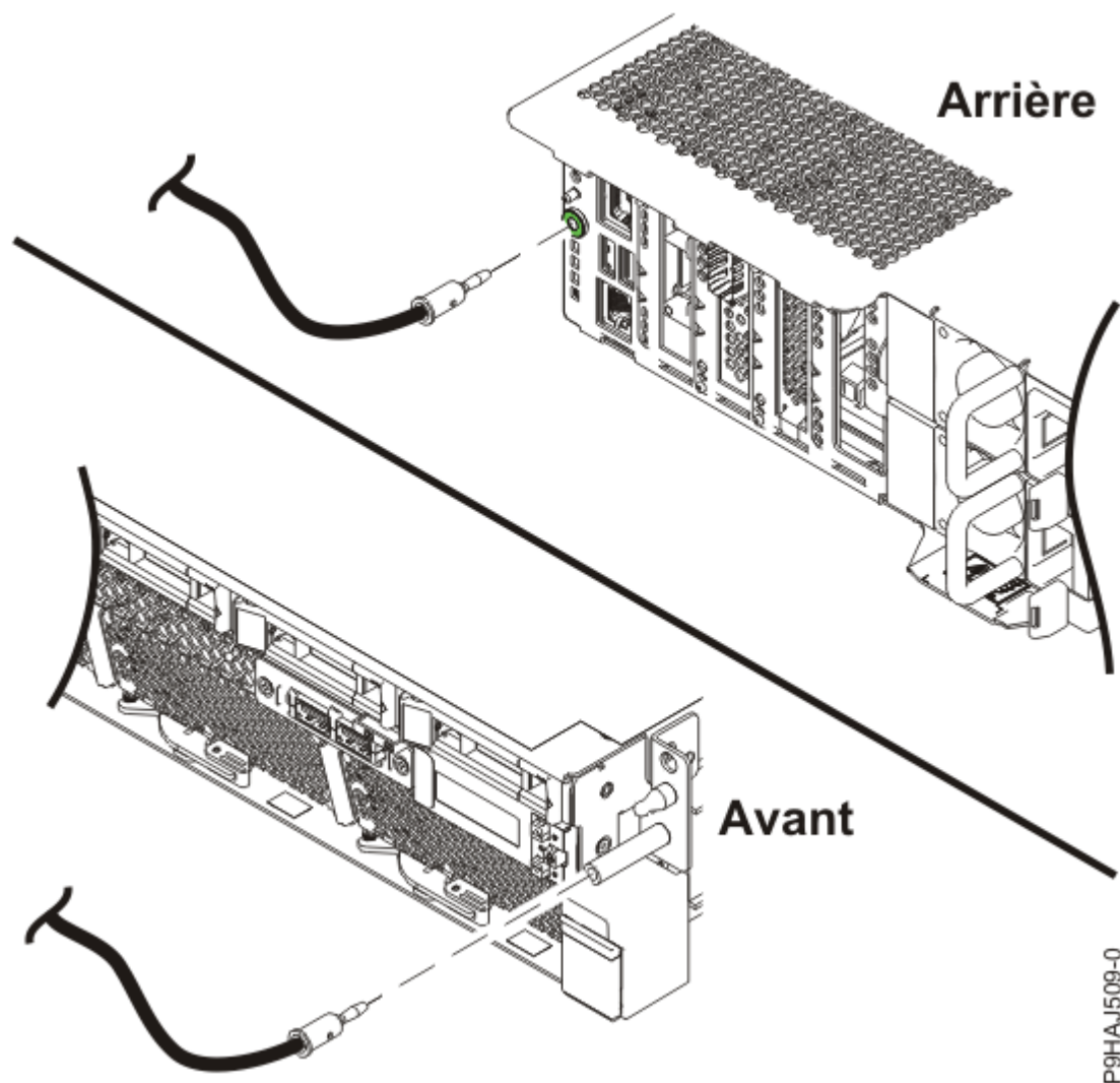
Figure 4. Emplacement des fiches de décharge électrostatique
