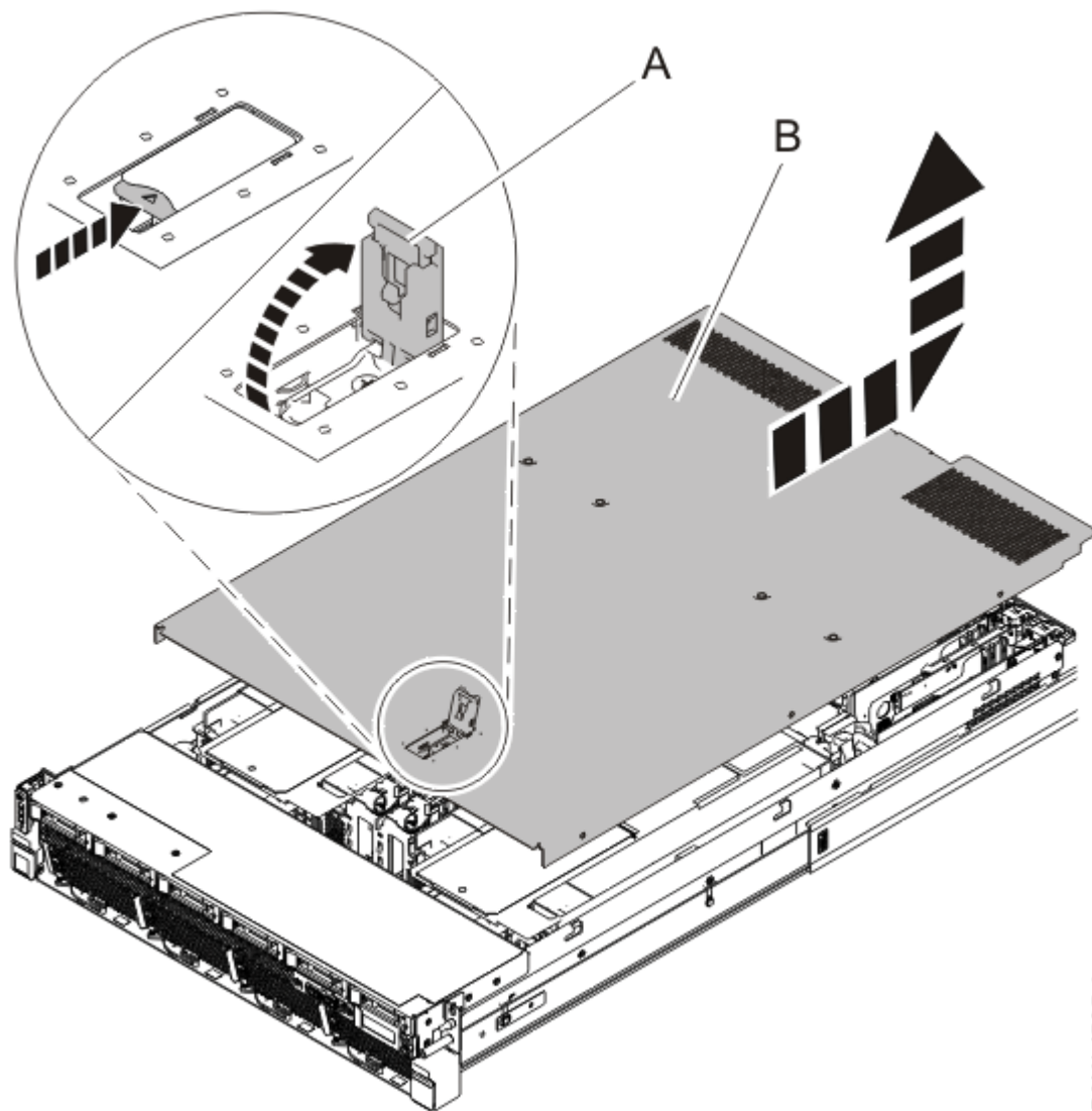
Figure 5. Retrait du capot d'accès
