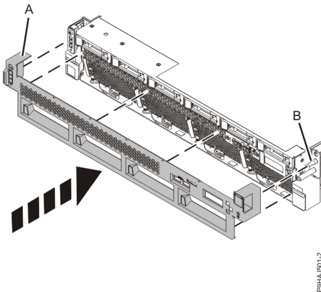
Figure 15. Installation du capot avant
