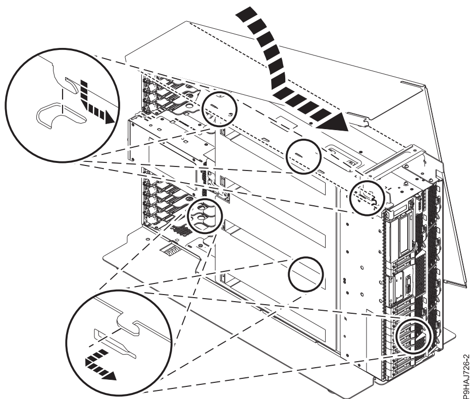
Figure 26. Installation du capot latéral
