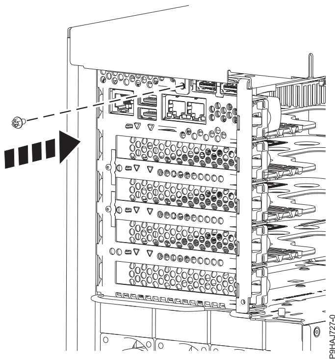
Figure 27. Installation de la vis du capot latéral
