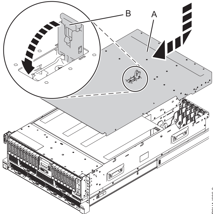
Figure 32. Installation du capot d'accès
