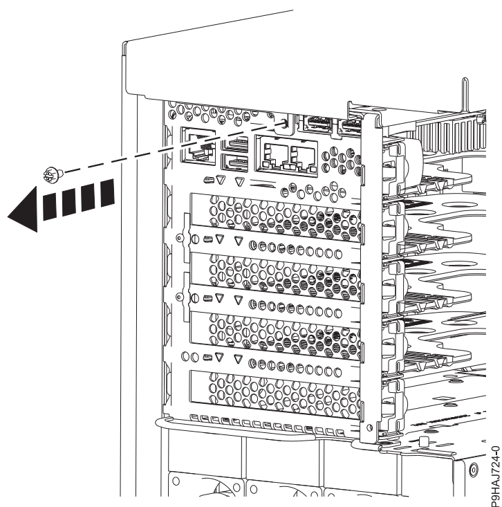
Figure 20. Retrait de la vis du capot latéral
