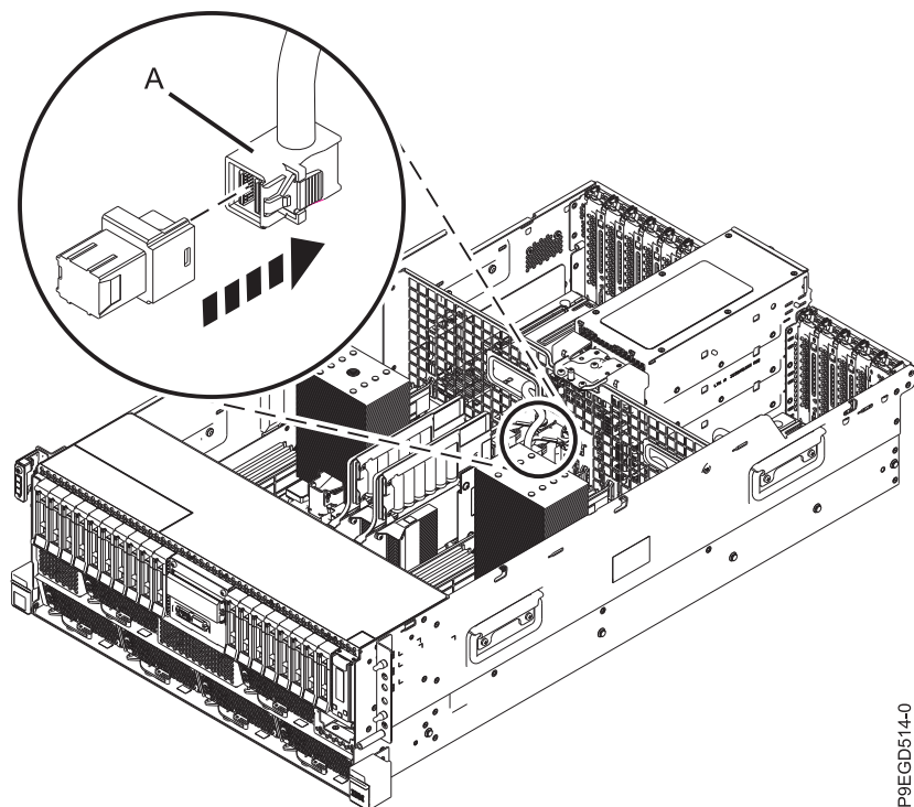
Figure 4. Débranchement des câbles SAS arrière de la carte interne SAS RAID dans les emplacements P1-C49 et P-C50
