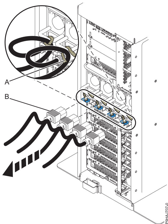
Figure 43. Retrait des cordons d'alimentation d'un serveur autonome
