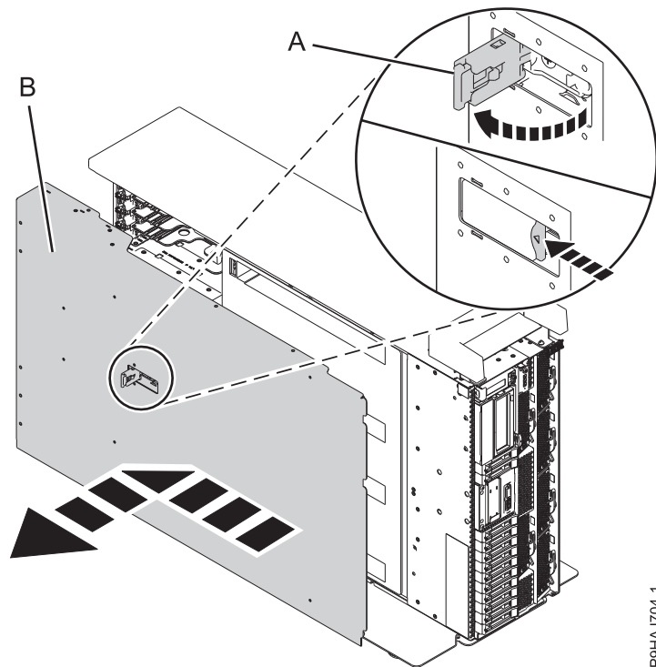
Figure 31. Retrait du capot d'accès
