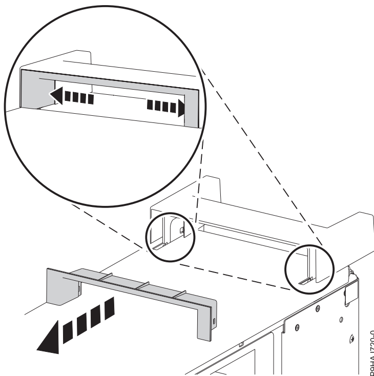
Figure 18. Retrait de la pièce plastique de la poignée
