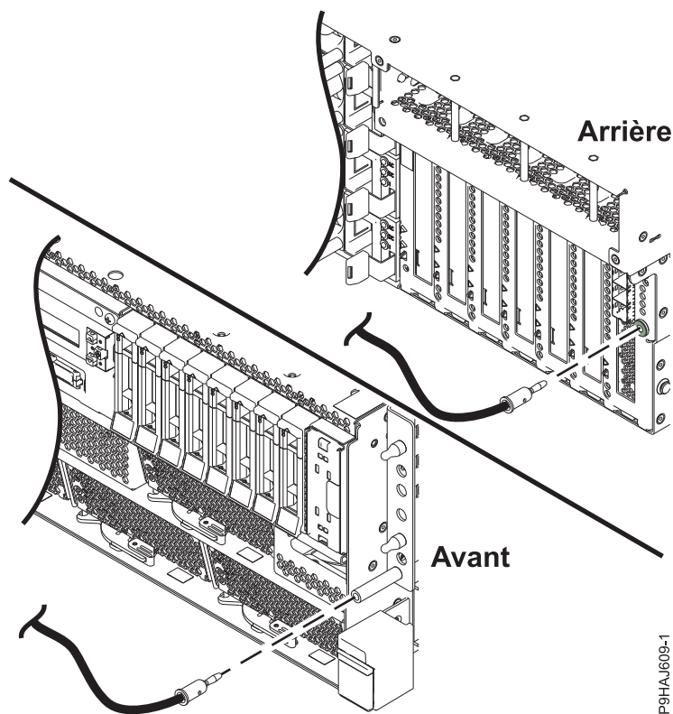
Figure 1. Emplacement des fiches de décharge électrostatique
