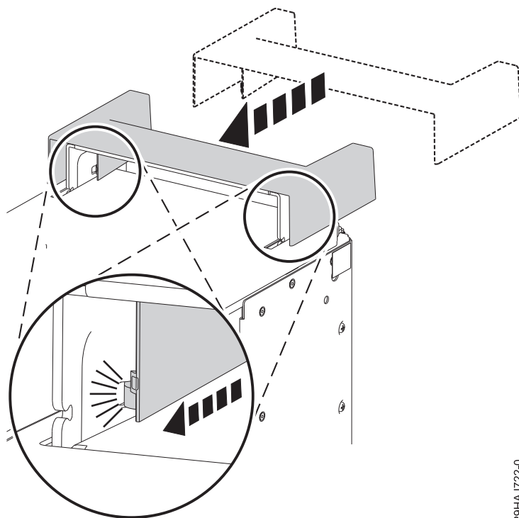
Figure 28. Fixation de la poignée
