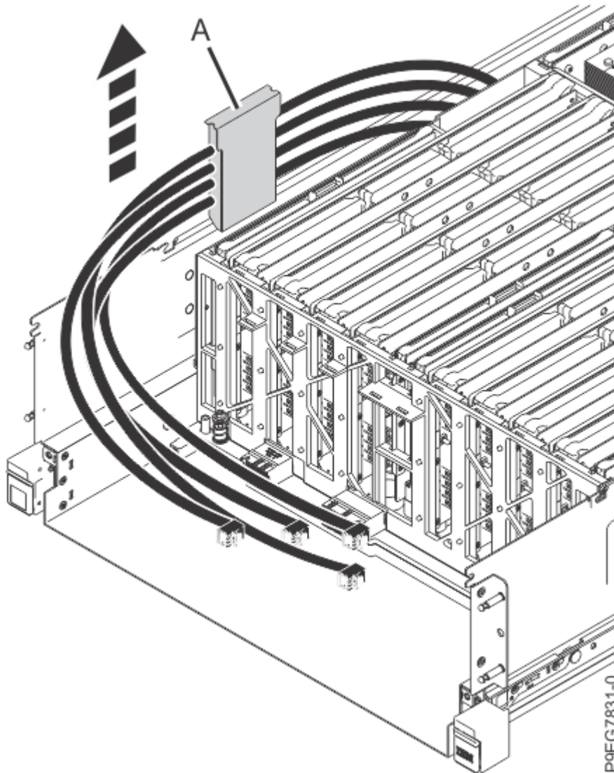
Figure 17. Retrait du support de câble SAS pour un fond de panier d'unité de disque à fonction étendue 6. Remettez le capot d'accès en place.
