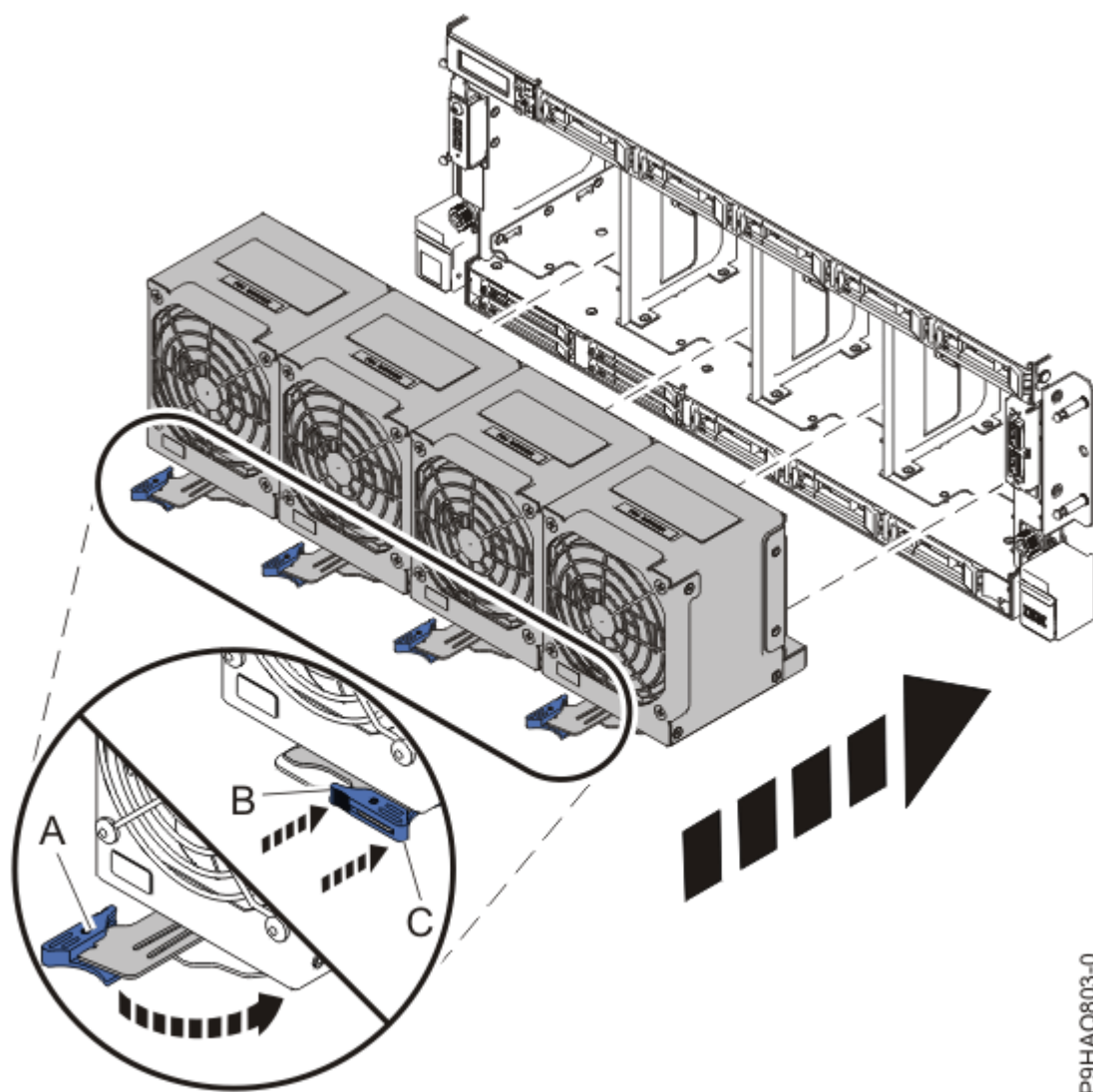
Figure 45. Remise en place des ventilateurs
