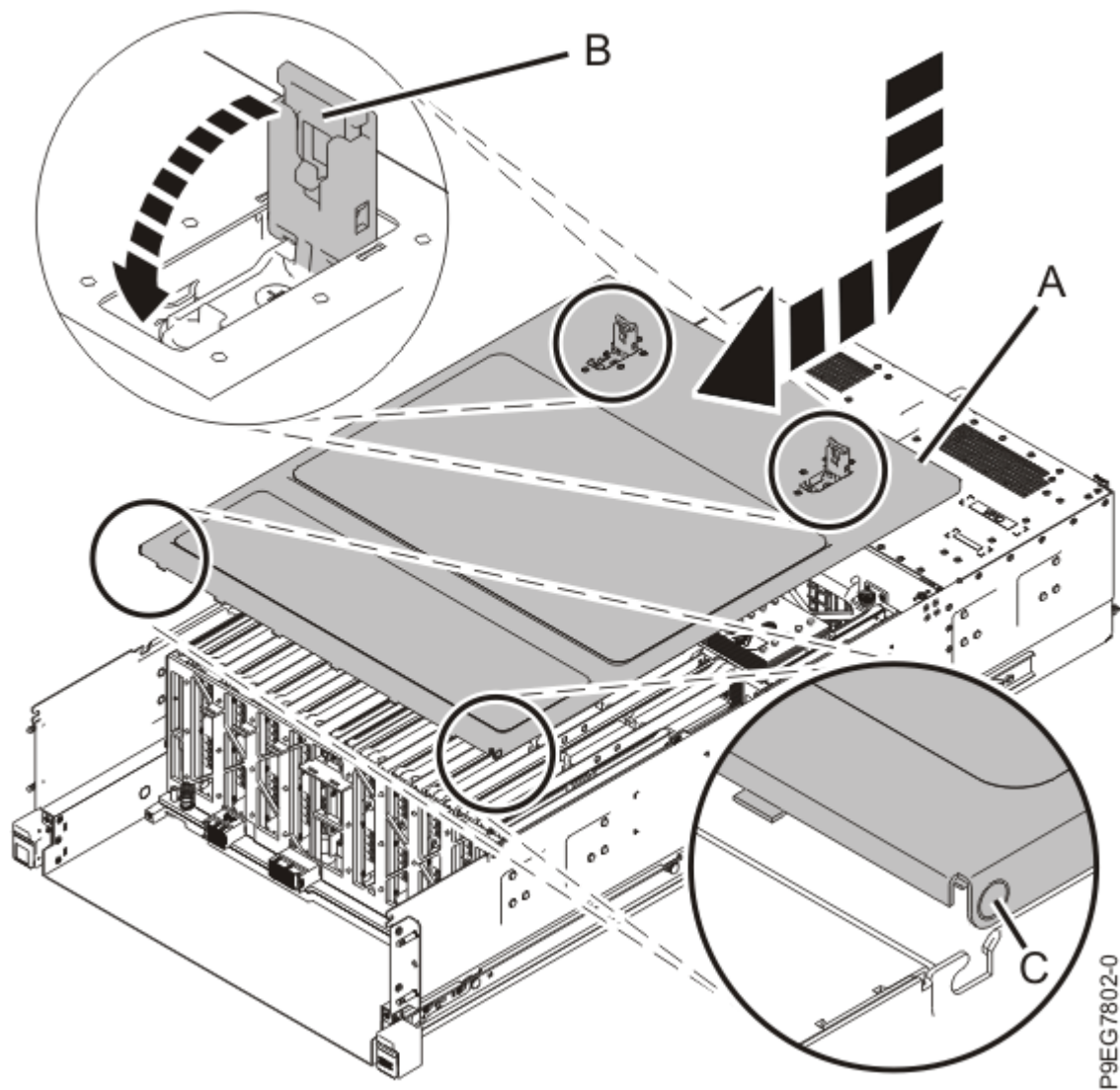
Figure 18. Installation du capot d'accès
