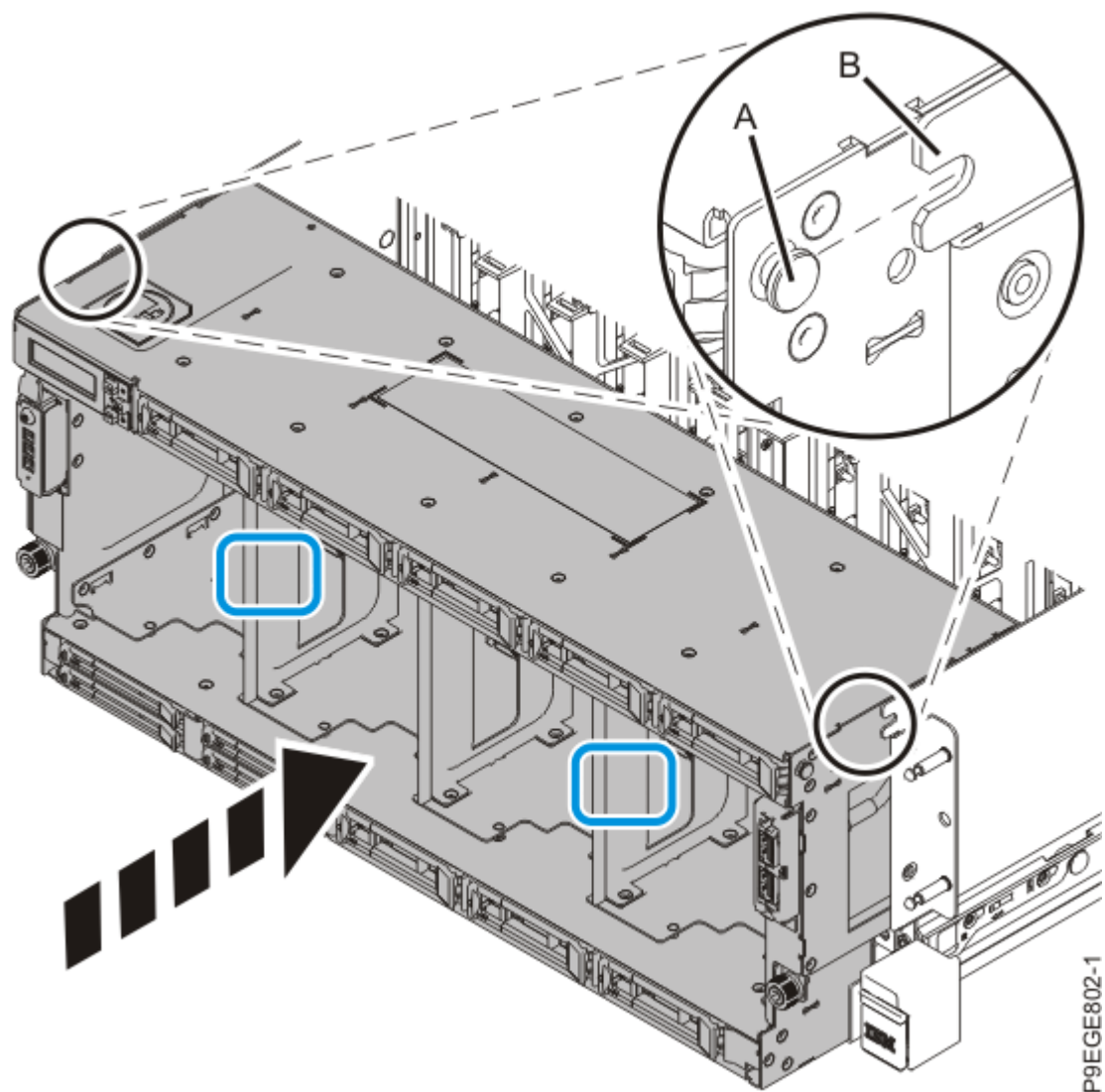
Figure 42. Remise en place du fond de panier d'unité de disque
