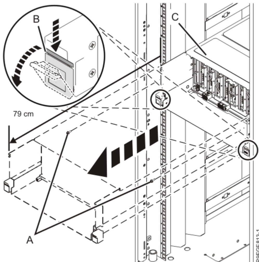
Figure 32. Glissement partiel du système hors de l'armoire
