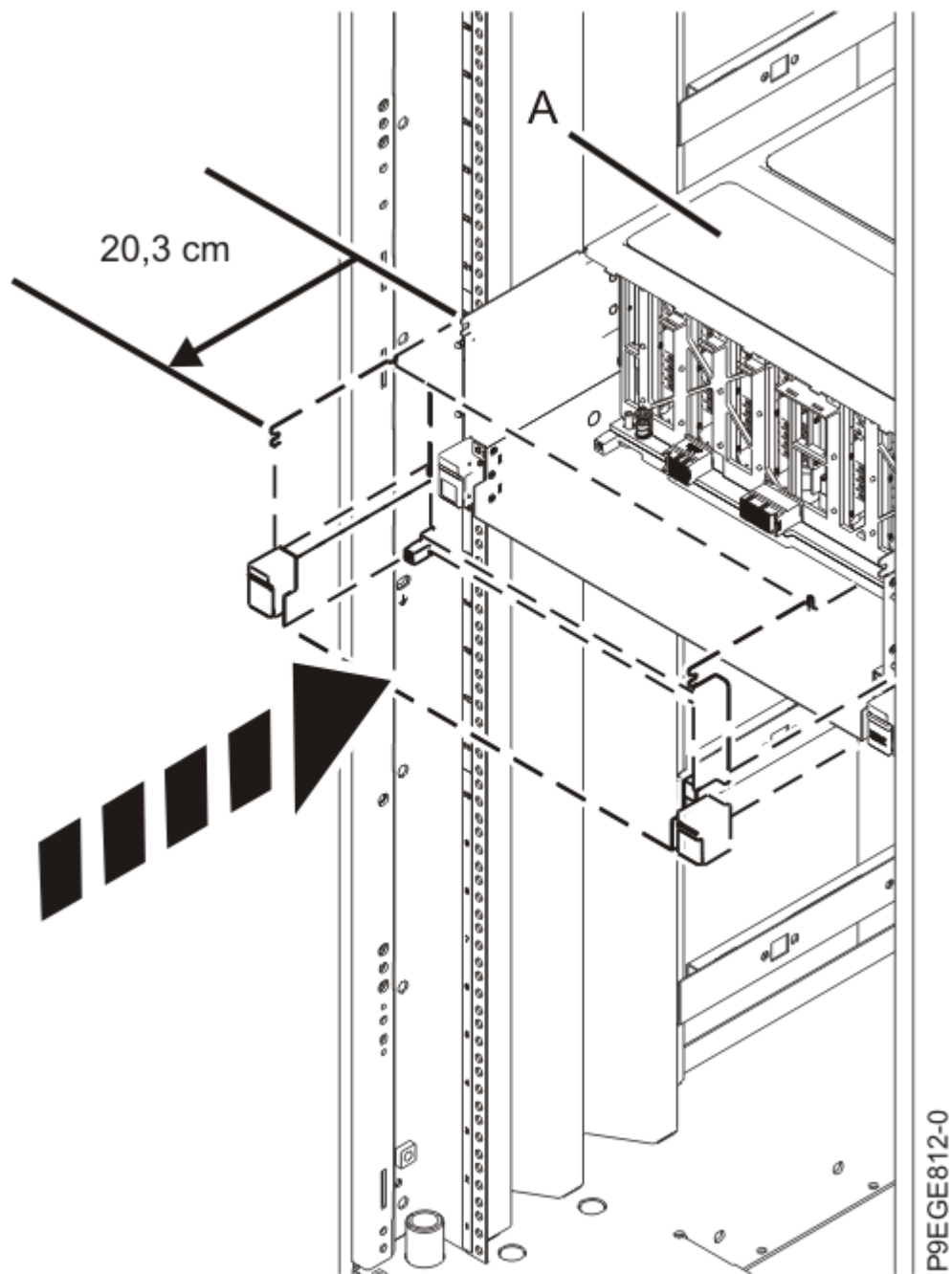
Figure 39. Glissement partiel du système dans l'armoire
