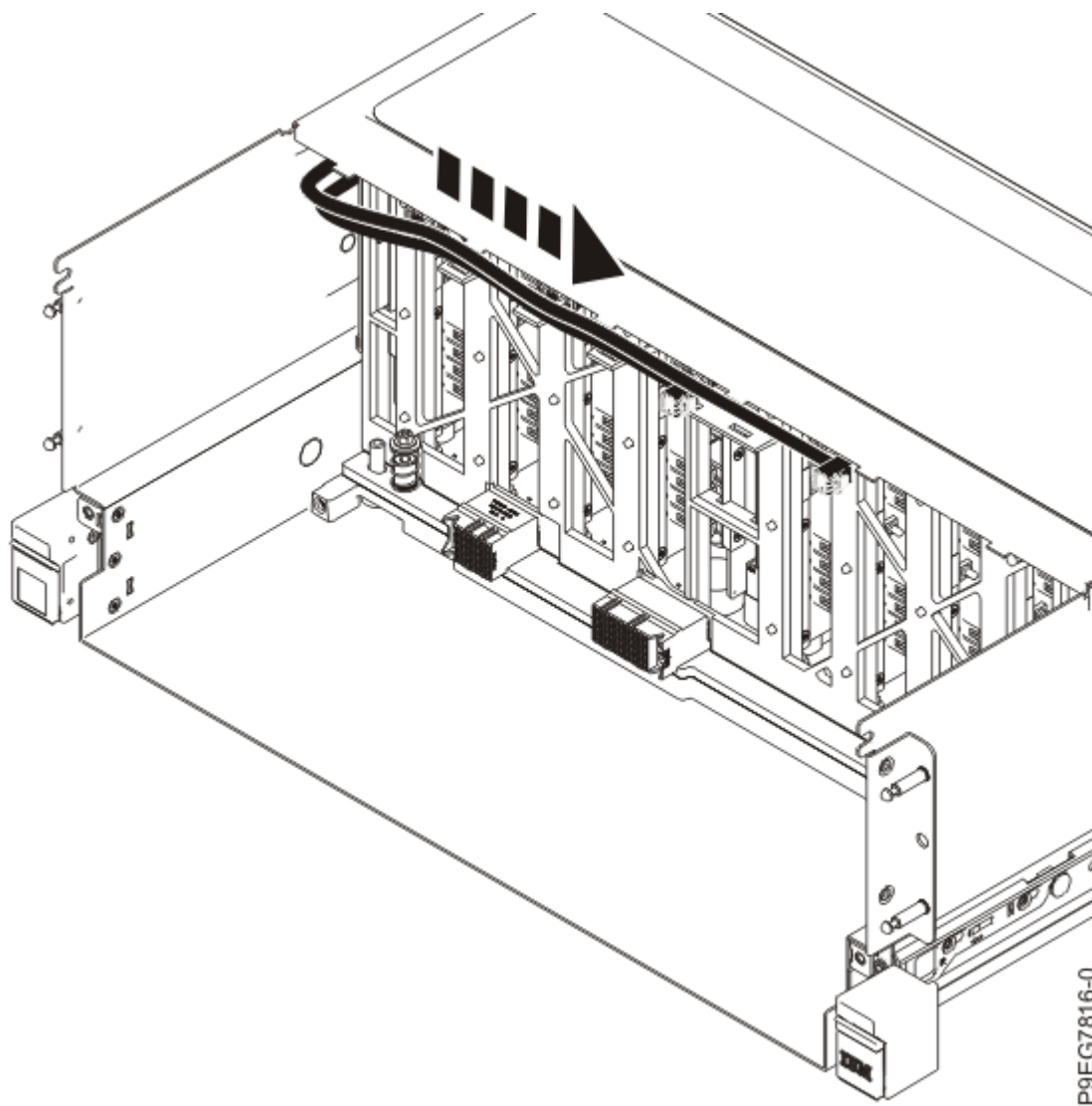
Figure 36. Routage des câbles SAS pour un fond de panier d'unité de disque (fonction de base)
