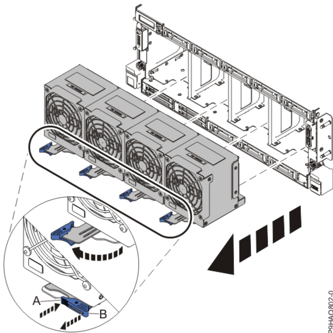
Figure 8. Retrait des ventilateurs
