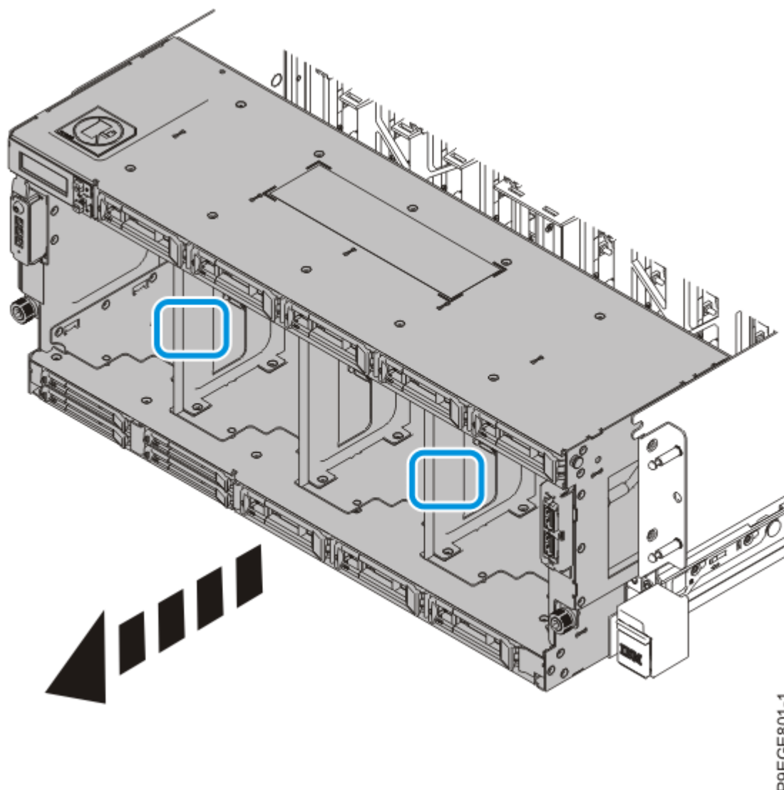
Figure 10. Retrait partiel du fond de panier d'unité de disque
