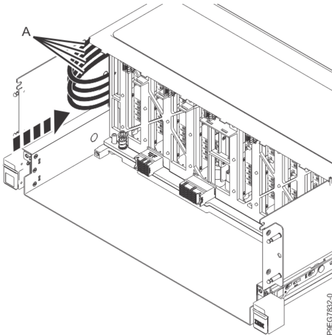
Figure 20. Enrouler et pousser les câbles SAS à l'intérieur du système pour le fond de panier d'unité de disque (fonction étendue)
