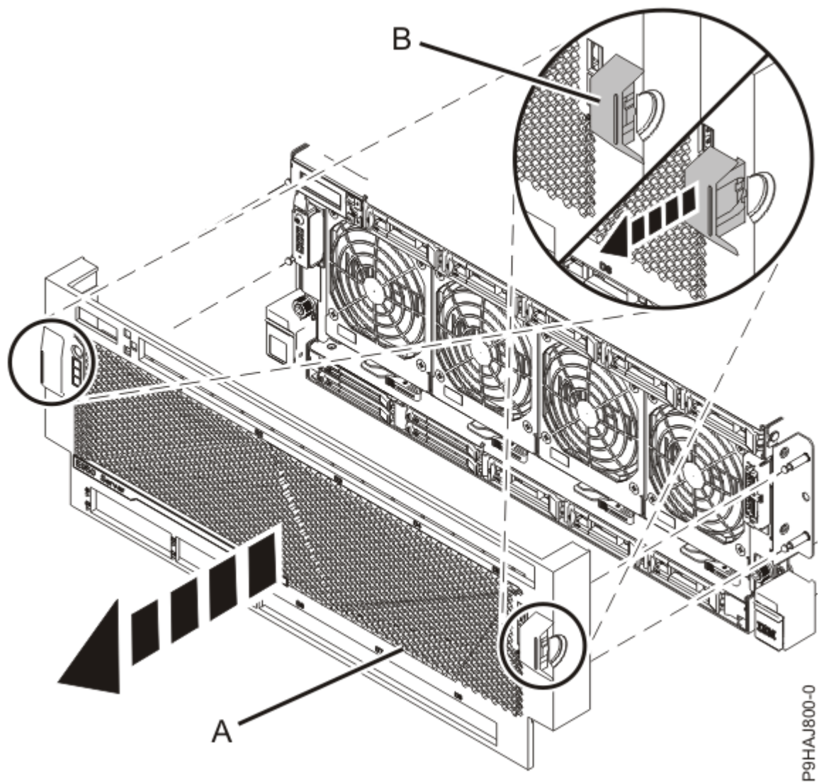
Figure 4. Retrait du capot avant
