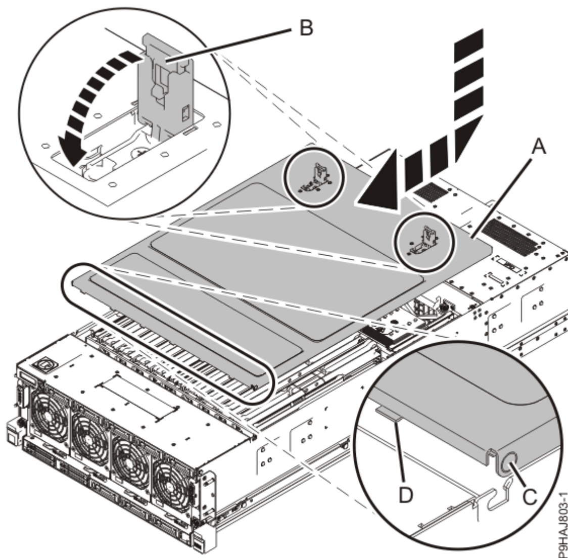
Figure 48. Installation du capot d'accès
