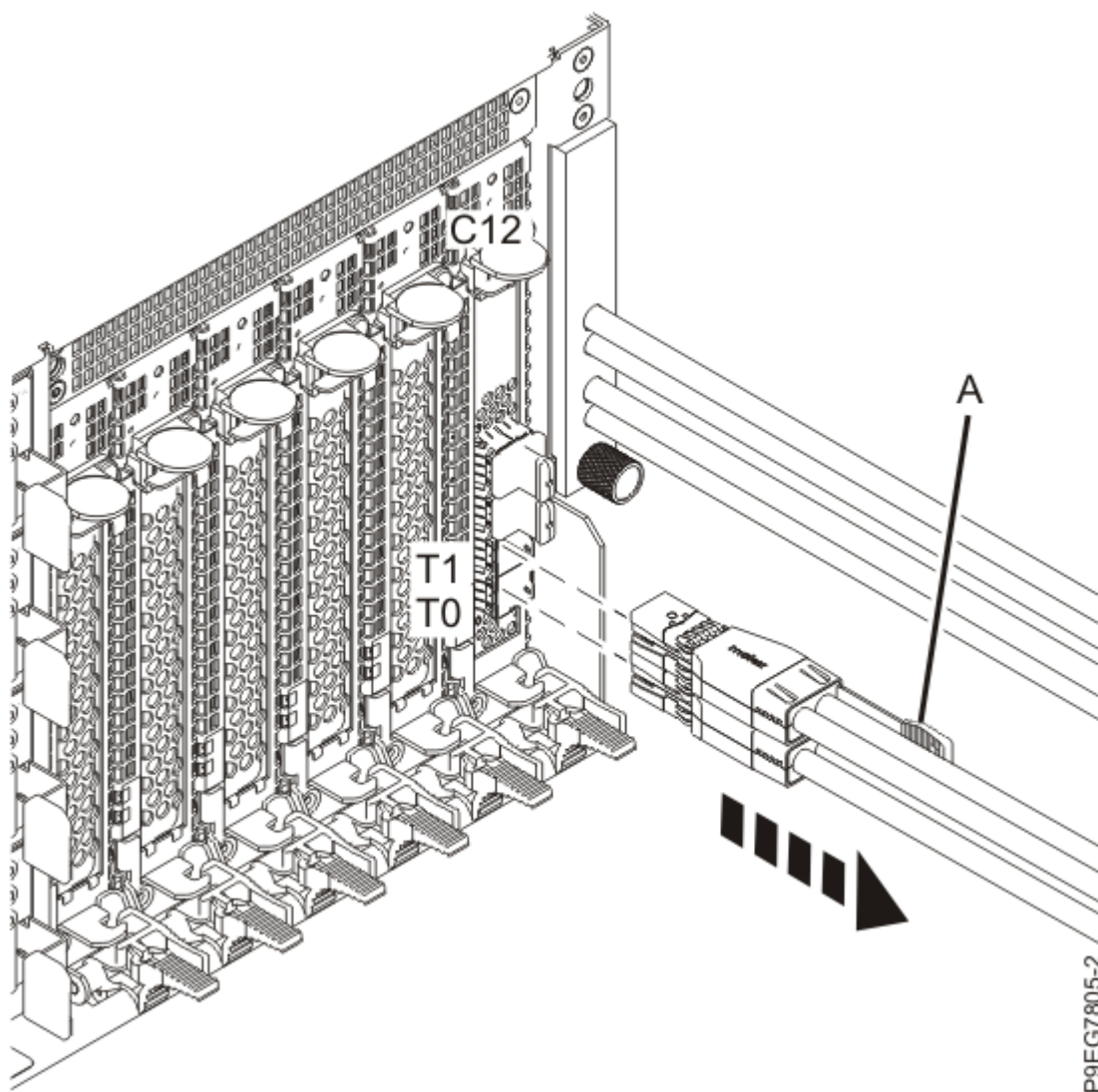
Figure 22. Déconnexion des câbles SAS pour la configuration de base pour le fond de panier d'unité de disque (fonction de base)
