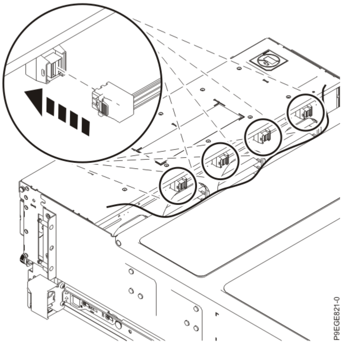
Figure 41. Connexion des câbles SAS au fond de panier d'unité de disque (fonction étendue)
