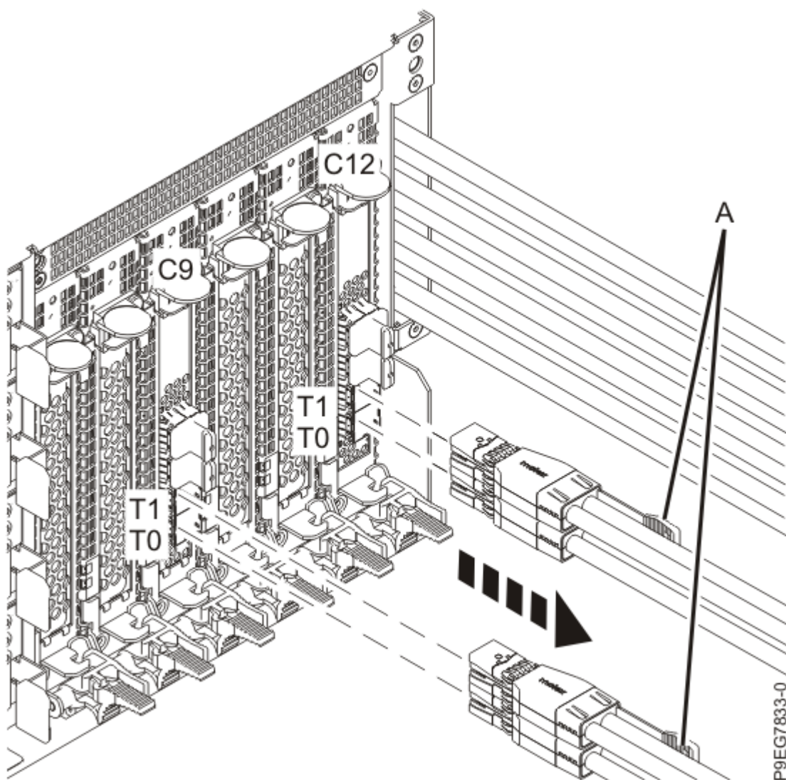
Figure 24. Déconnexion des câbles SAS pour un fond de panier d'unité de disque à fonction étendue 10. Dévissez la vis (A) de fixation du support de câble SAS (B) à l'arrière du système. Retirez le support de câble et les câbles SAS de l'arrière du système.
