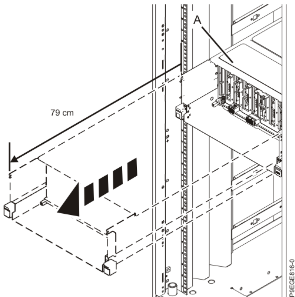
Figure 15. Faire glisser partiellement le système hors de l'armoire
