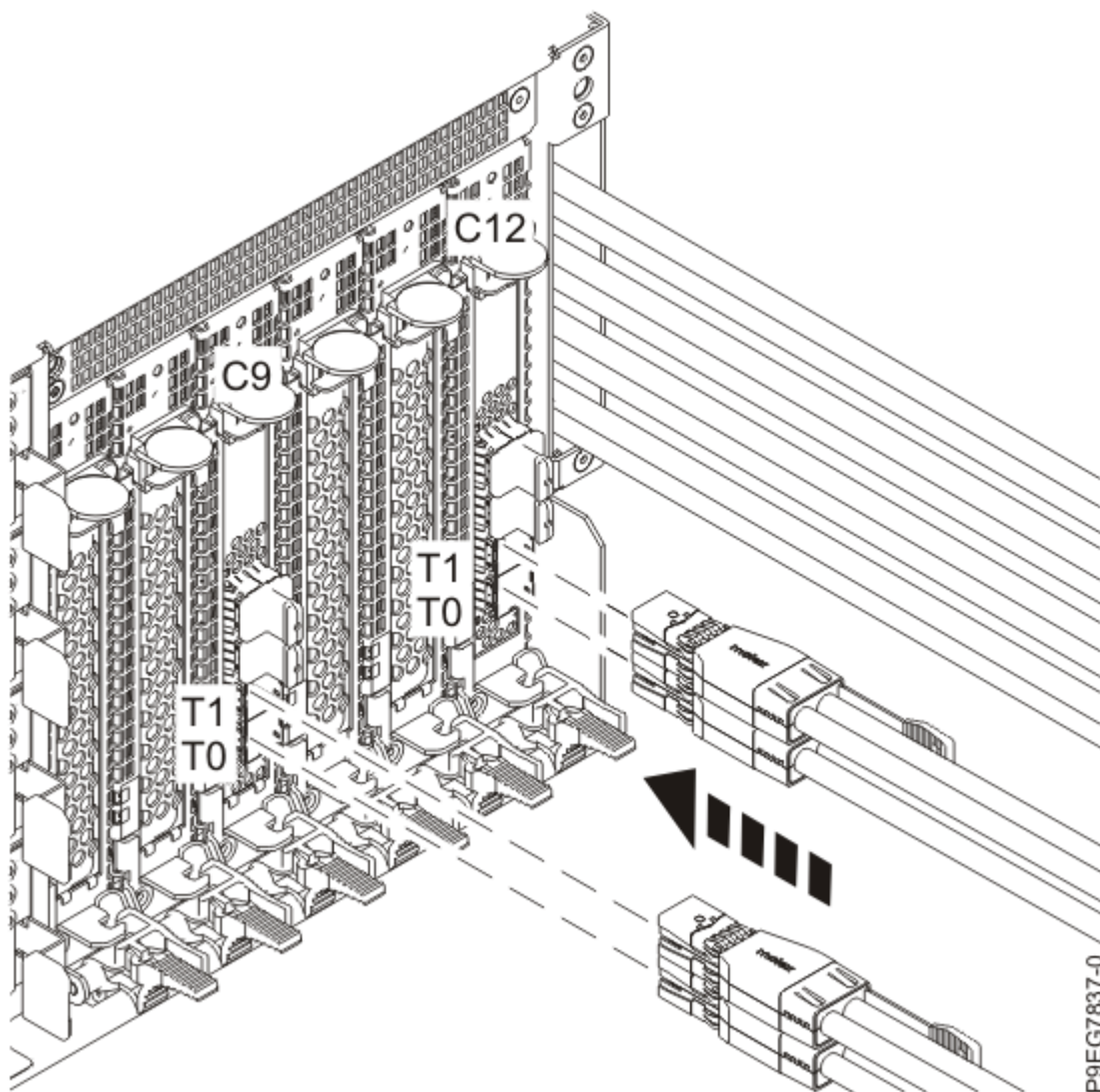
Figure 31. Branchement des câbles SAS pour un fond de panier d'unité de disque à fonction étendue
