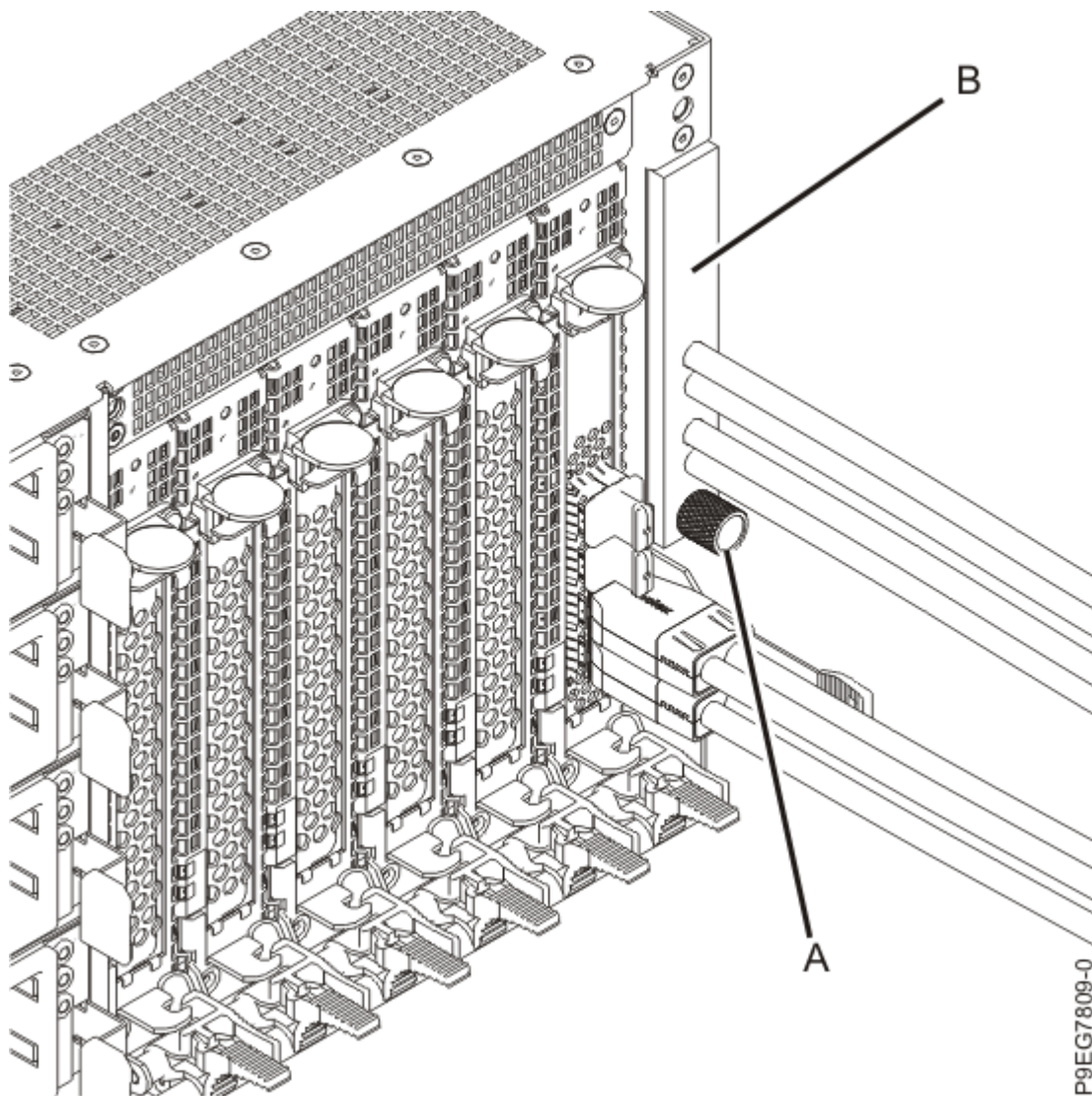
Figure 2. Identification des câbles SAS fixés à l'extérieur
