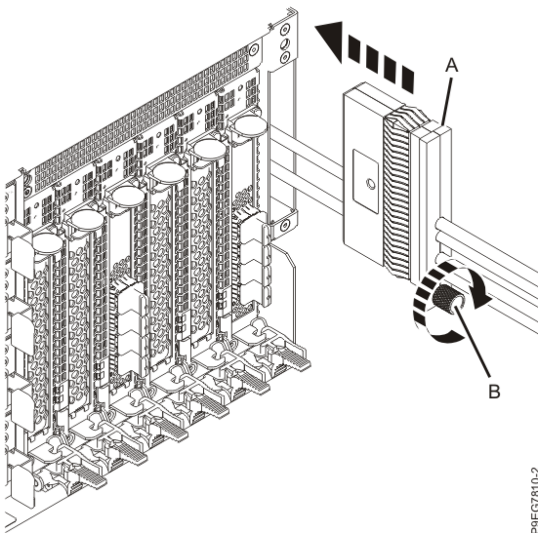
Figure 27. Insertion des câbles SAS et du support de câble SAS pour le fond de panier d'unité de disque (fonction de base)
