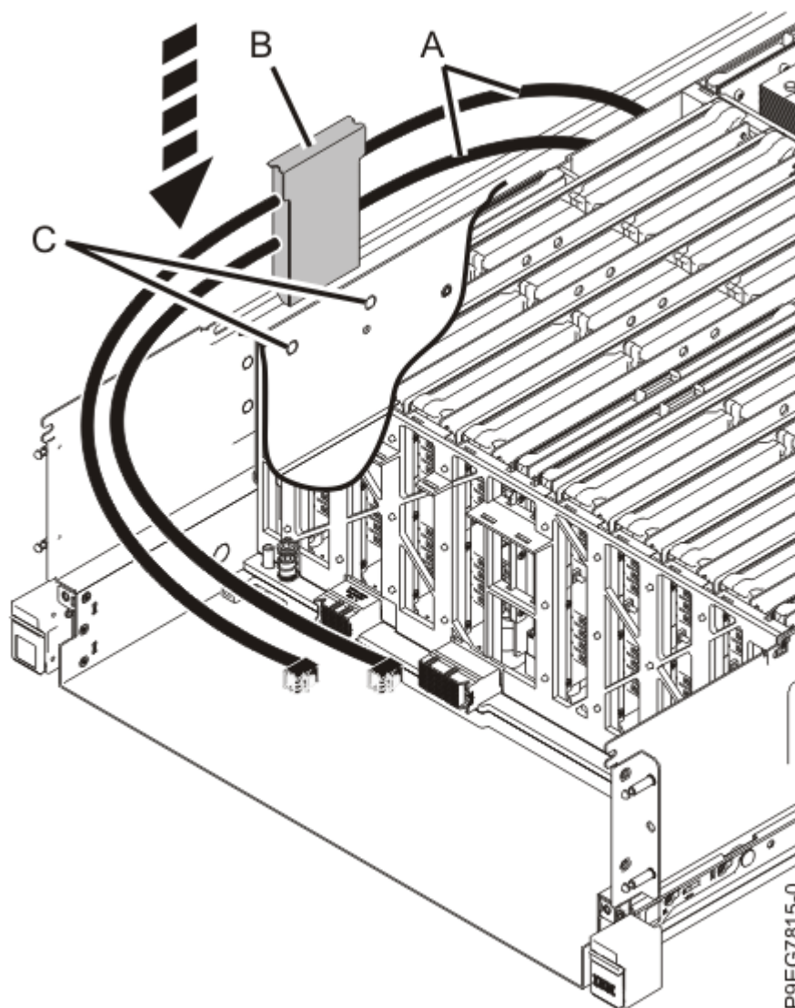
Figure 34. Remise en place du support de câble SAS pour le fond de panier d'unité de disque (fonction de base)
