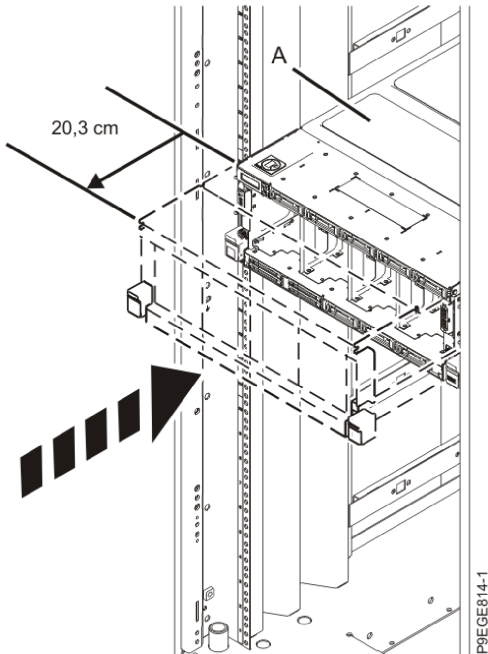
Figure 43. Mise en position de fonctionnement du système
