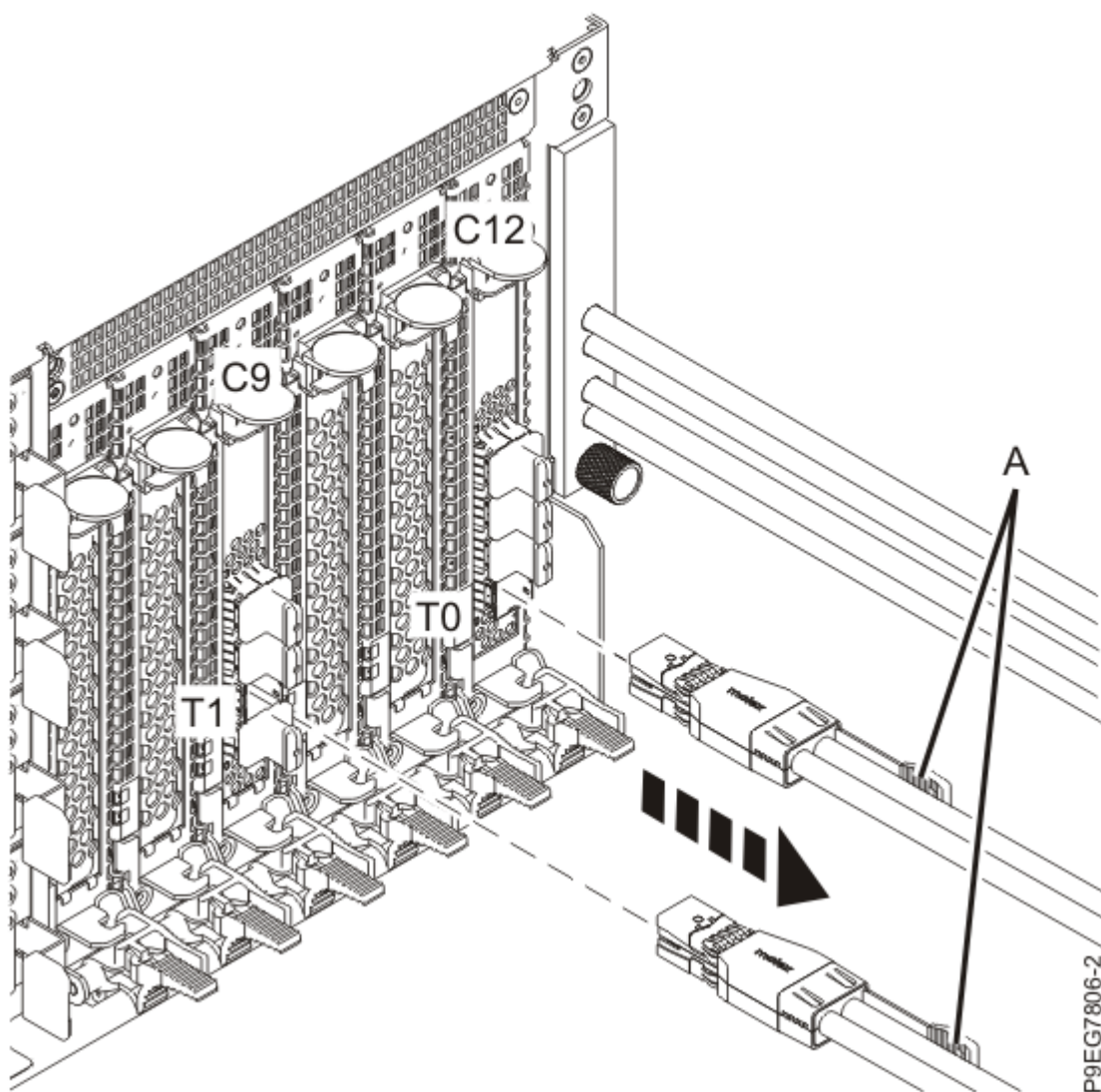
Figure 23. Déconnexion des câbles SAS pour la configuration de fractionnement pour le fond de panier d'unité de disque (fonction de base)
