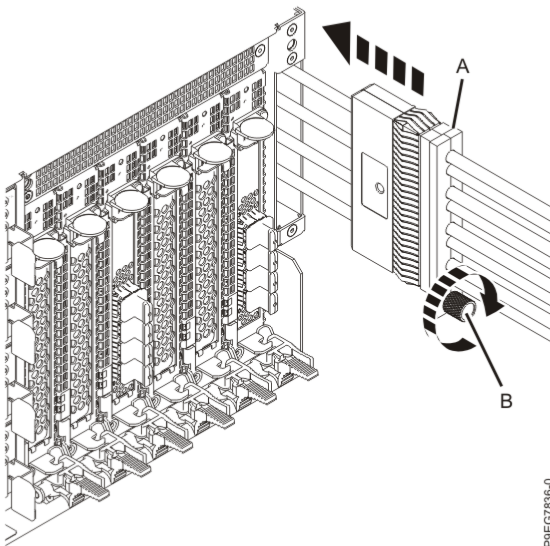
Figure 28. Insertion des câbles SAS et du support de câble SAS pour le fond de panier d'unité de disque (fonction étendue)
