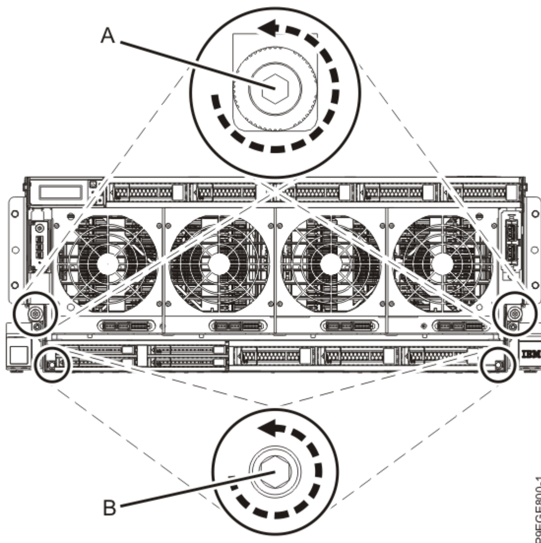
Figure 9. Desserrage des vis du fond de panier d'unité de disque
