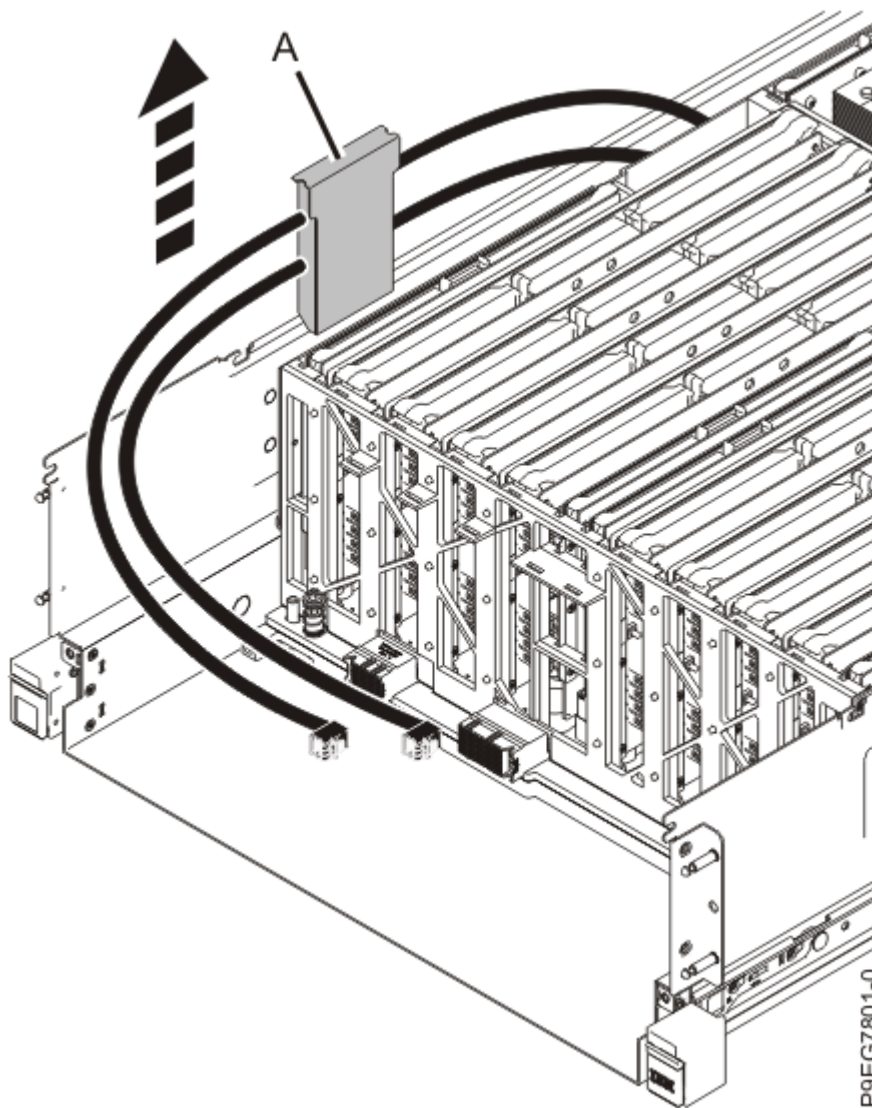
Figure 16. Retrait du support de câble SAS pour le fond de panier d'unité de disque (fonction de base)
