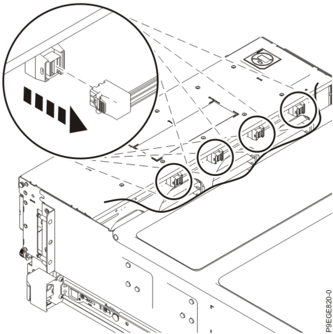
Figure 13. Débranchement des câbles SAS du fond de panier d'unité de disque étendu f) Avec les deux mains, retirez complètement le fond de panier d'unité de disque du système.
