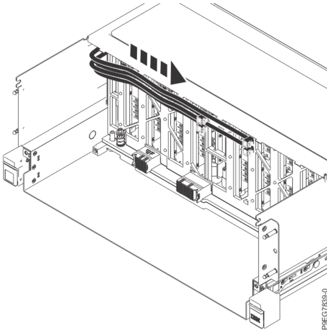
Figure 37. Routage des câbles SAS pour un fond de panier d'unité de disque (fonction étendue)
