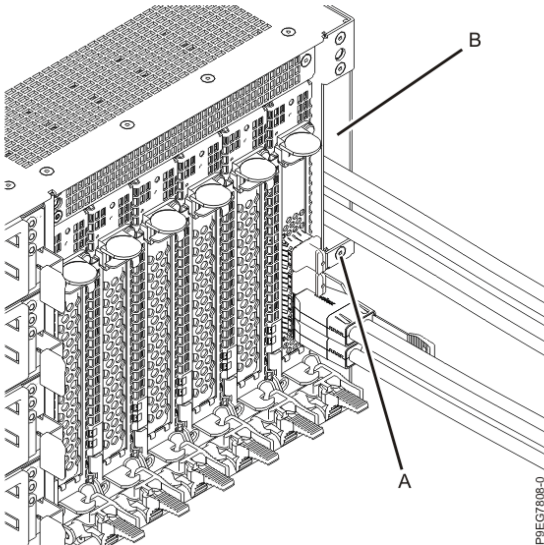
Figure 1. Identification des câbles SAS fixés à l'intérieur
