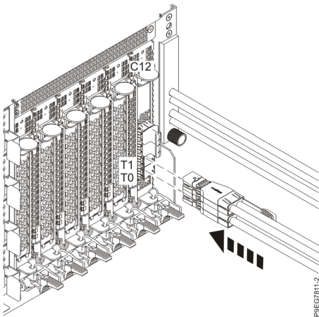
Figure 29. Branchement des câbles SAS pour la configuration de base pour le fond de panier d'unité de disque (fonction de base)
