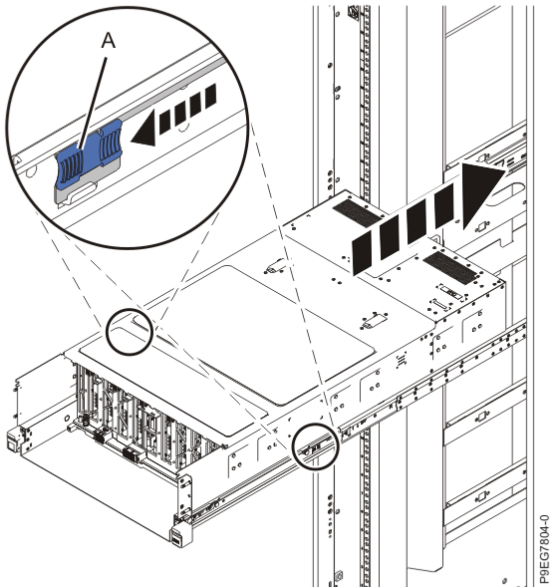
Figure 21. Mise en position de fonctionnement du système
