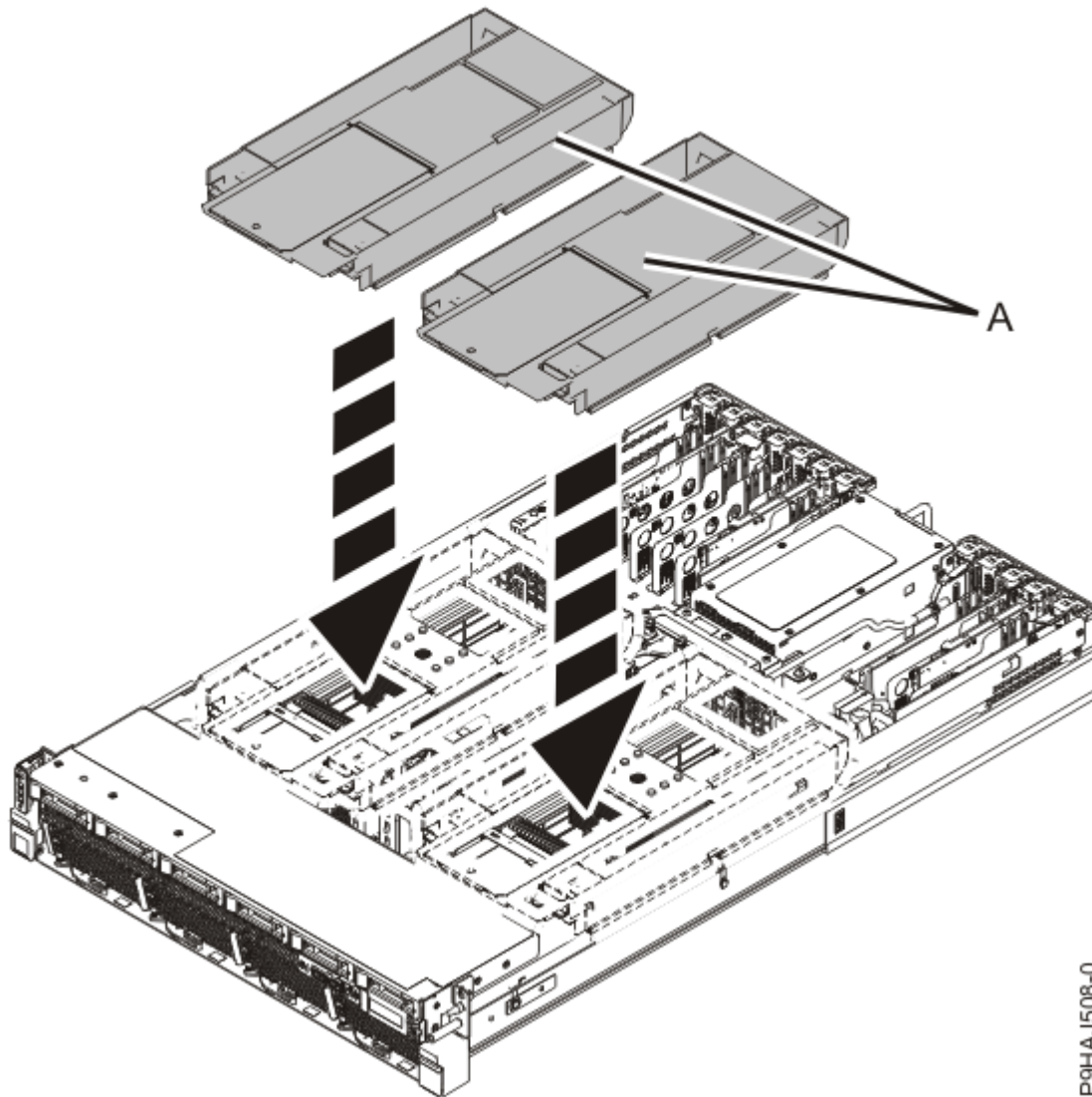
Figure 13. Remise en place de la grille d'aération
