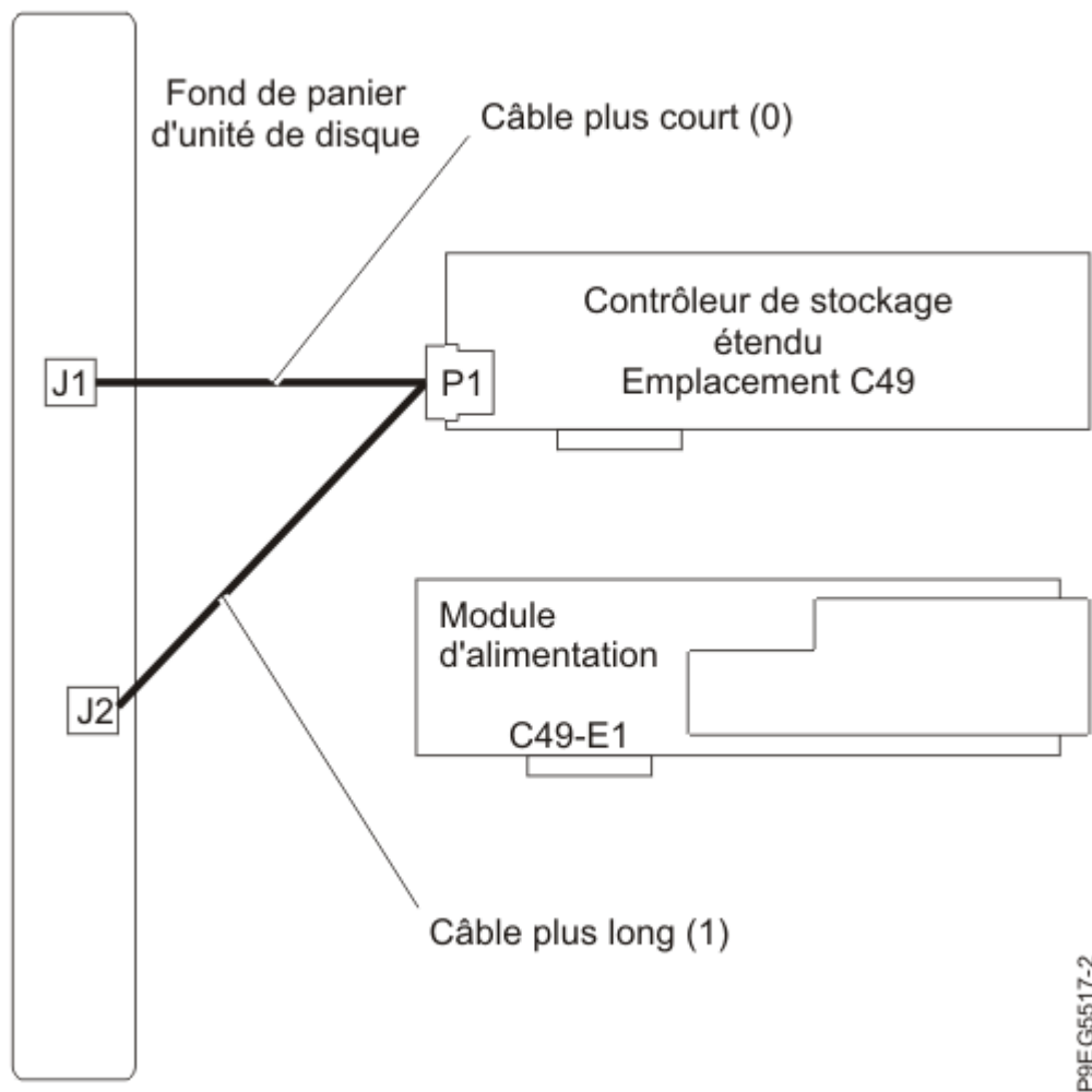
Figure 11. Reconnexion du câble SAS en "Y" dans une configuration de contrôleur de stockage hautes performances
