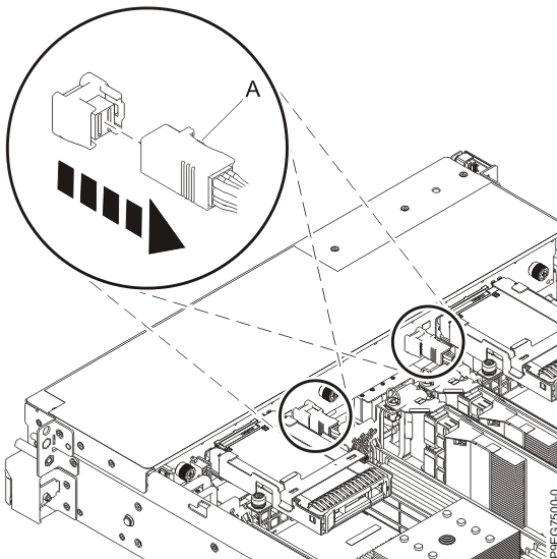
Figure 6. Déconnexion des câbles SAS avant
