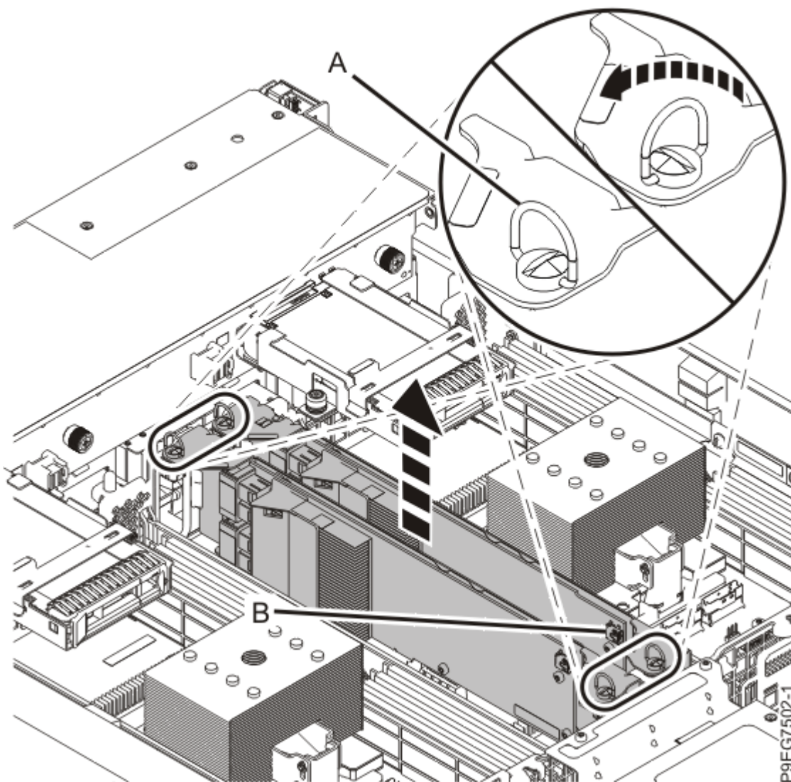
Figure 7. Retrait de l'adaptateur SAS RAID
