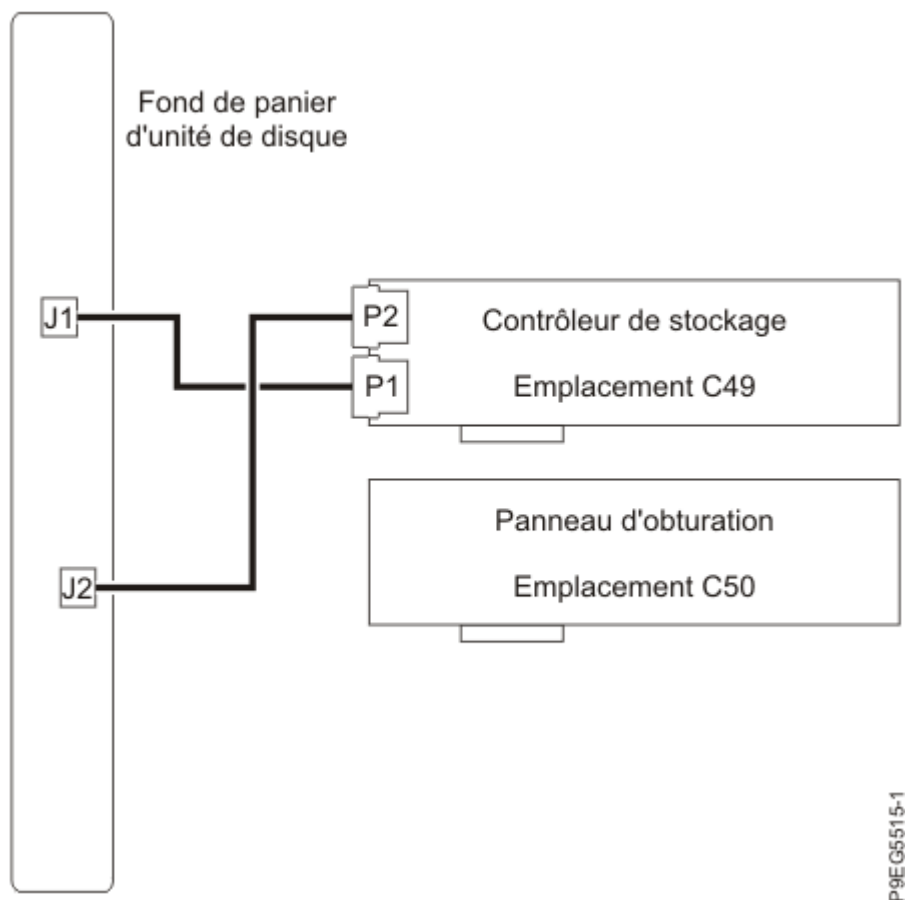
Figure 9. Reconnexion du câble SAS dans une configuration de stockage de base
