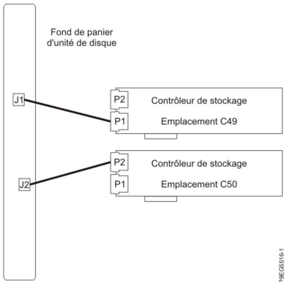
Figure 10. Reconnexion du câble SAS dans une configuration de disque partagé
