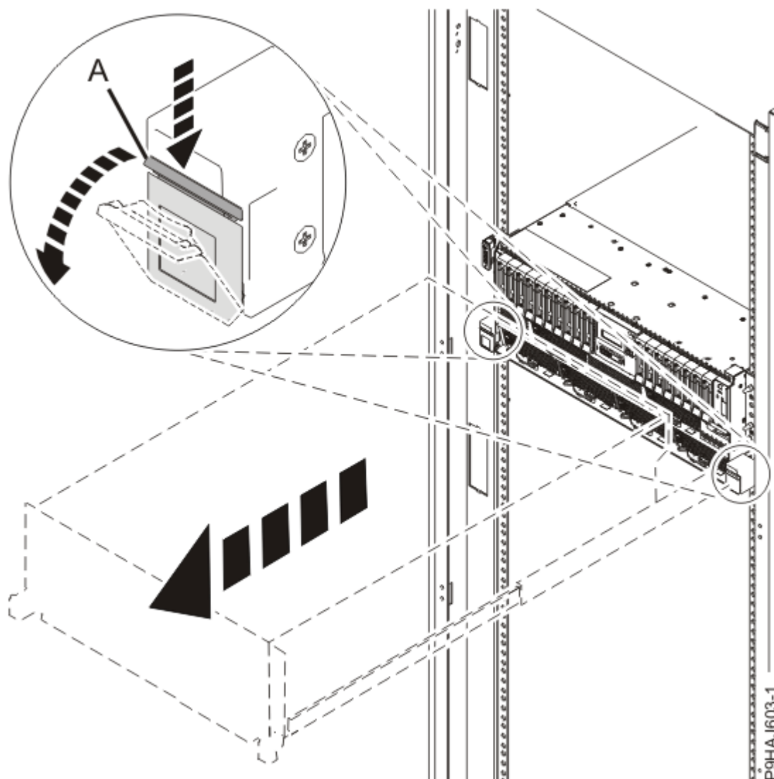
Figure 3. Déblocage des loquets latéraux
