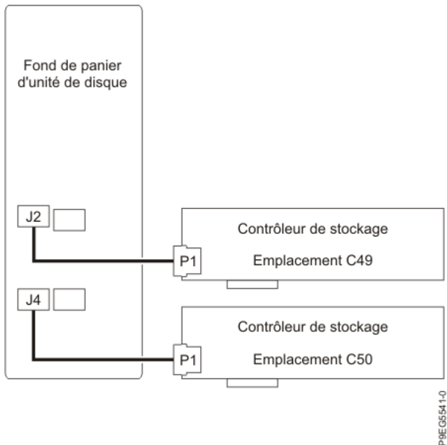
Figure 15. Reconnexion du câble SAS dans la configuration de fonction étendue 12 unités
