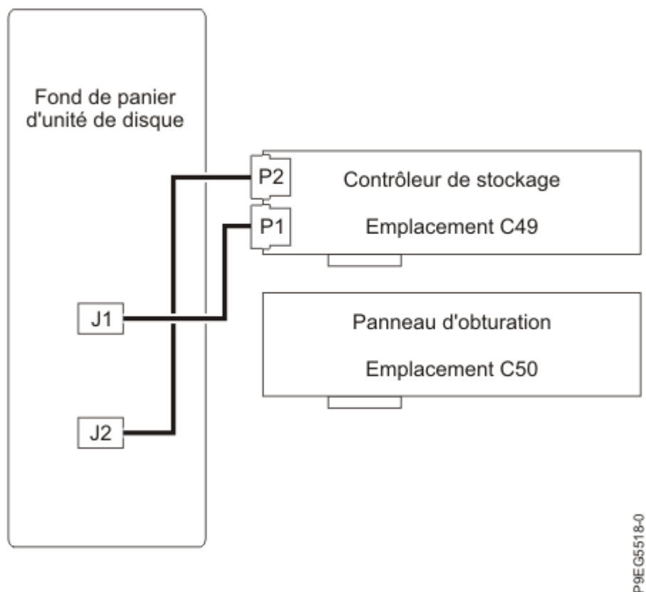
Figure 13. Reconnexion du câble SAS dans une configuration de stockage de base
