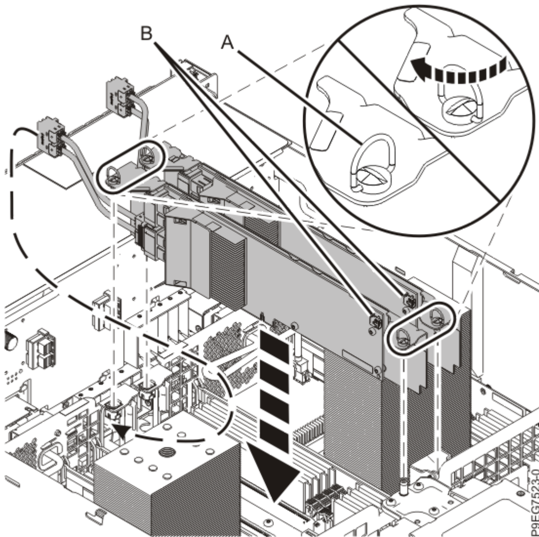
Figure 17. Remplacement de l'adaptateur SAS RAID
