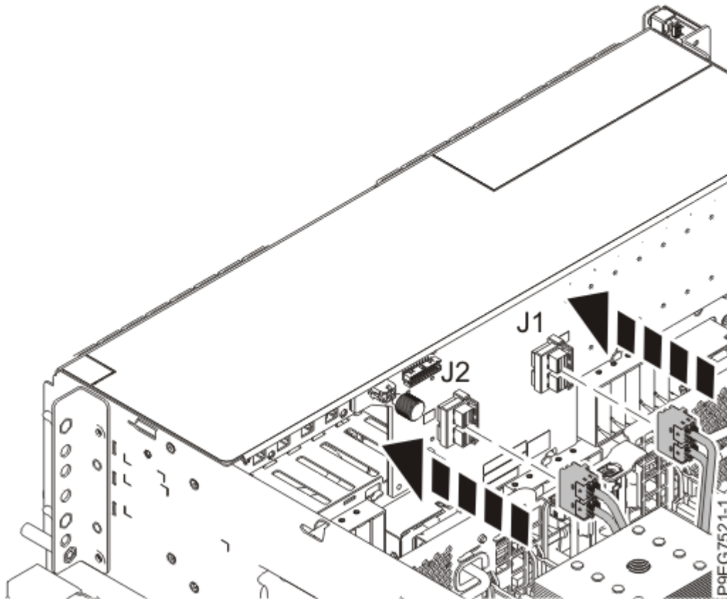
Figure 11. Reconnexion des câbles SAS avant au fond de panier d'unité de disque de la fonction de base
