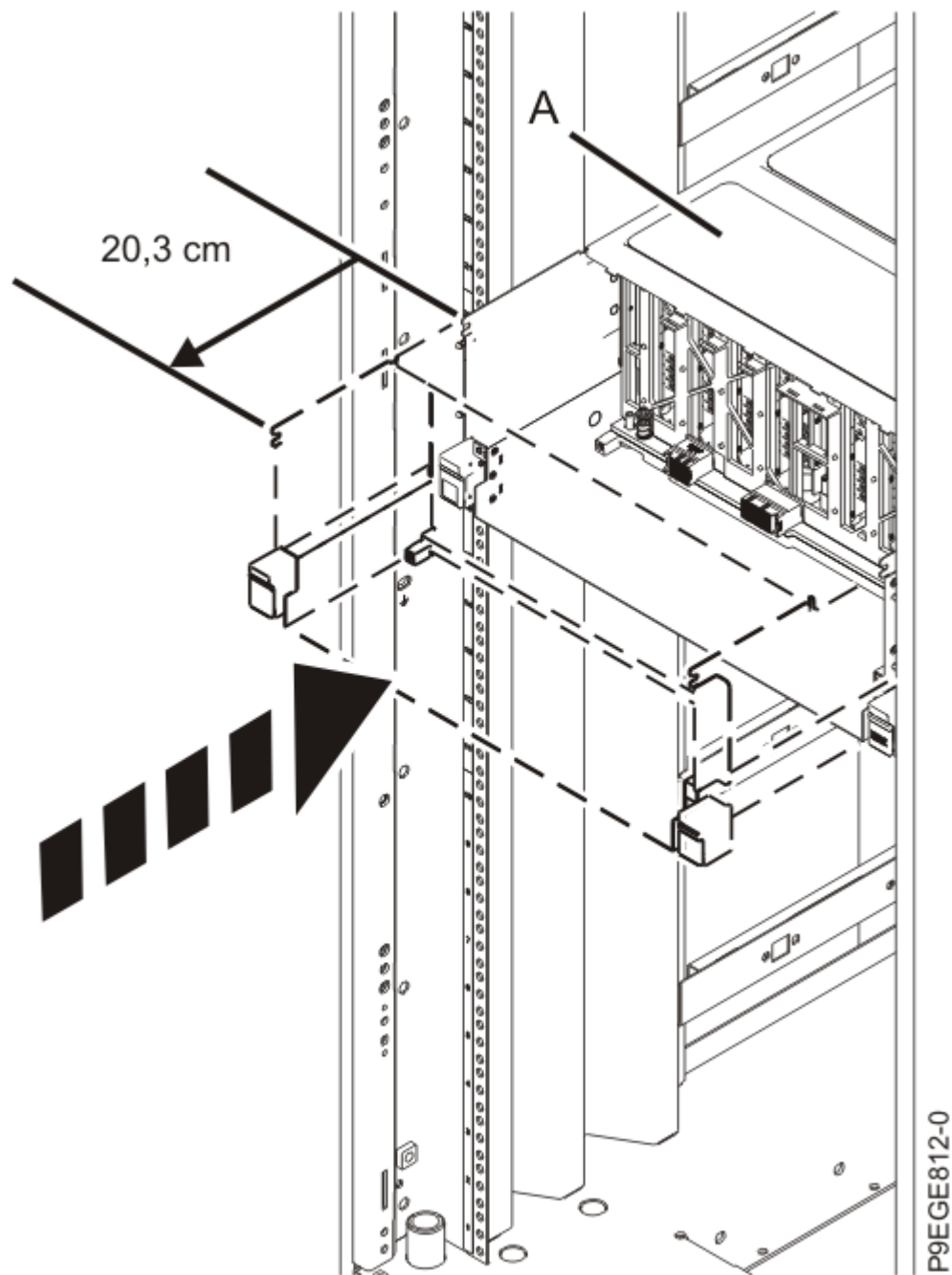
Figure 20. Glissement partiel du système dans l'armoire
