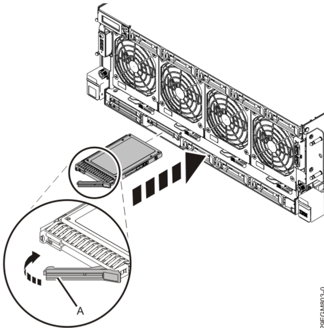
Figure 29. Installation ou remise en place d'une unité NVMe U.2 dans le système 9040-MR9
