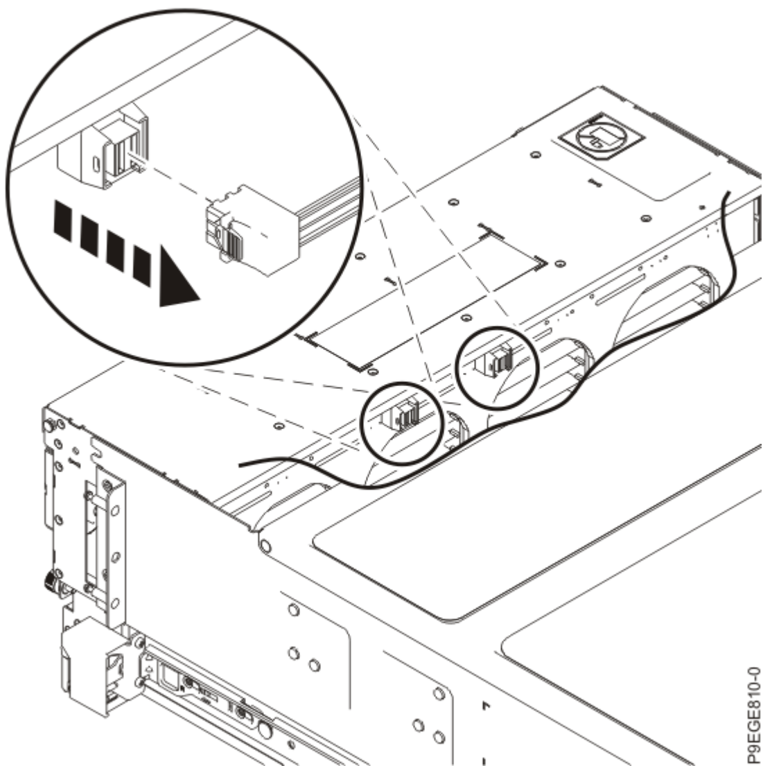
Figure 14. Débranchement des câbles SAS du fond de panier d'unité de disque de base
