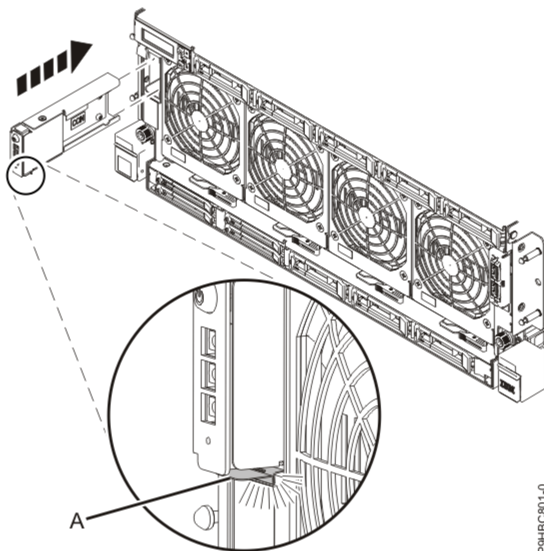
Figure 27. Remise en place du panneau de commande
