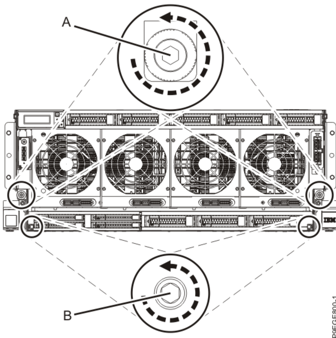
Figure 11. Desserrage des vis du fond de panier d'unité de disque
