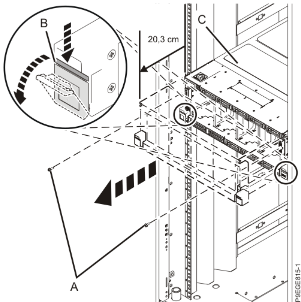
Figure 13. Glissement partiel du système hors de l'armoire
