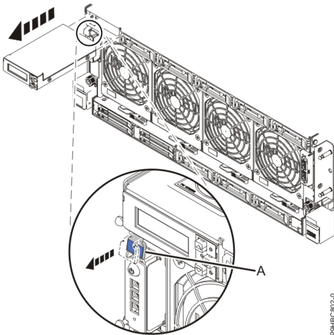
Figure 9. Retrait de l'écran du panneau de commande
