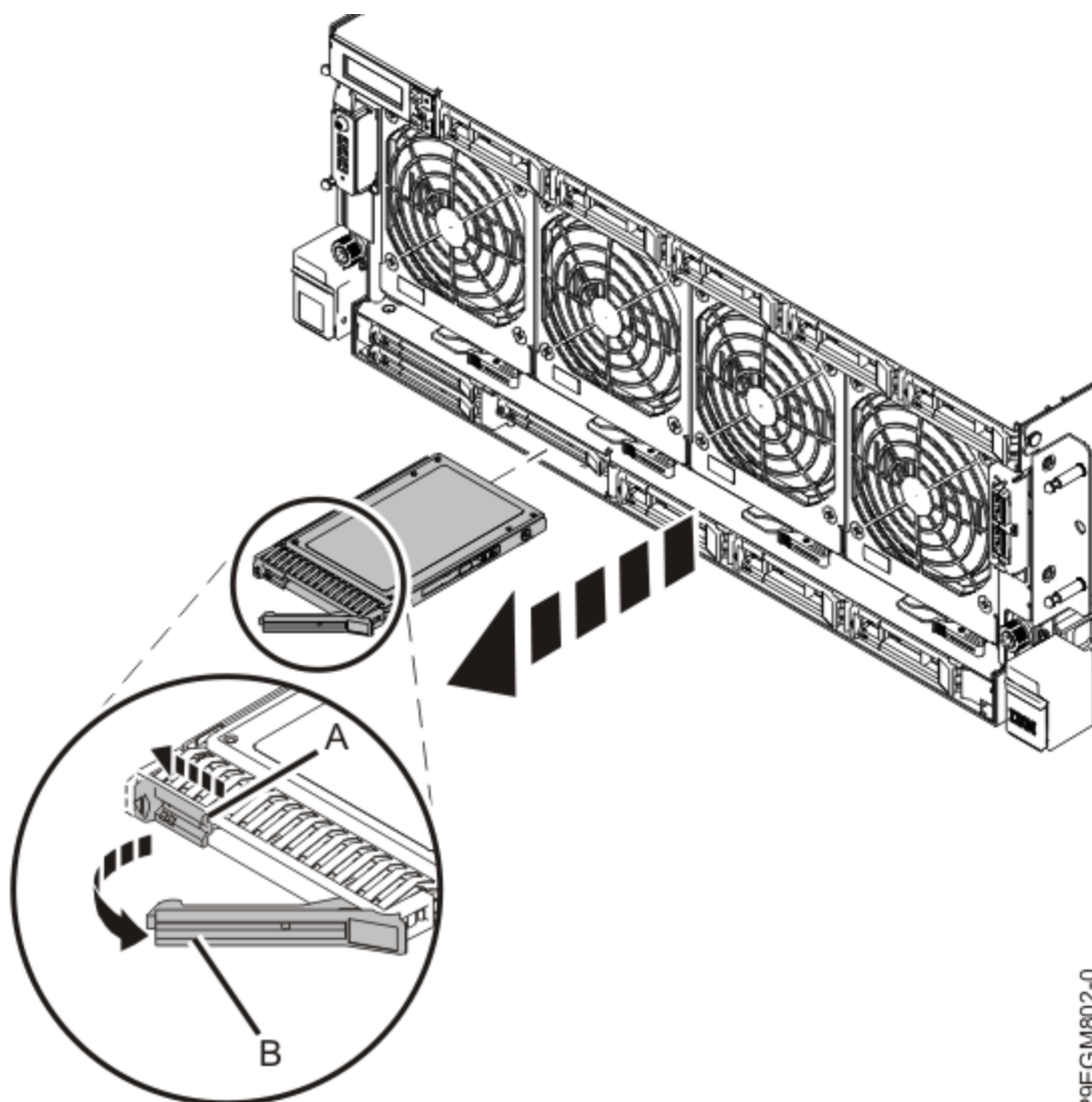
Figure 7. Retrait d'une unité de disque NVMe U.2 du système 9040-MR9
