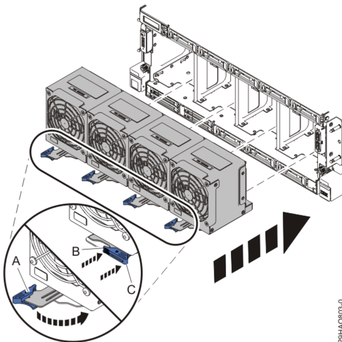
Figure 26. Remise en place des ventilateurs
