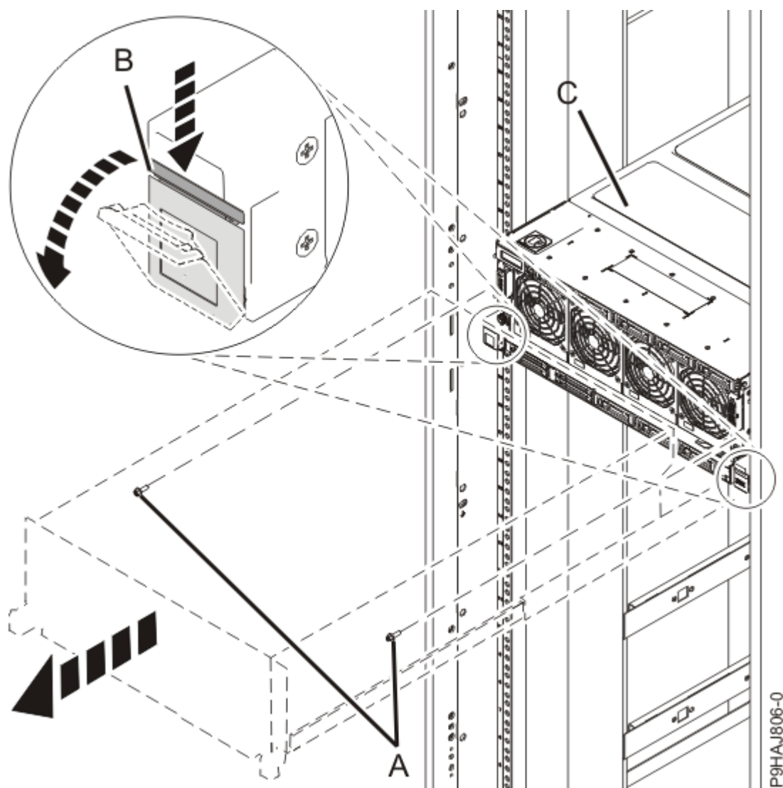
Figure 3. Mise en position de maintenance du système
