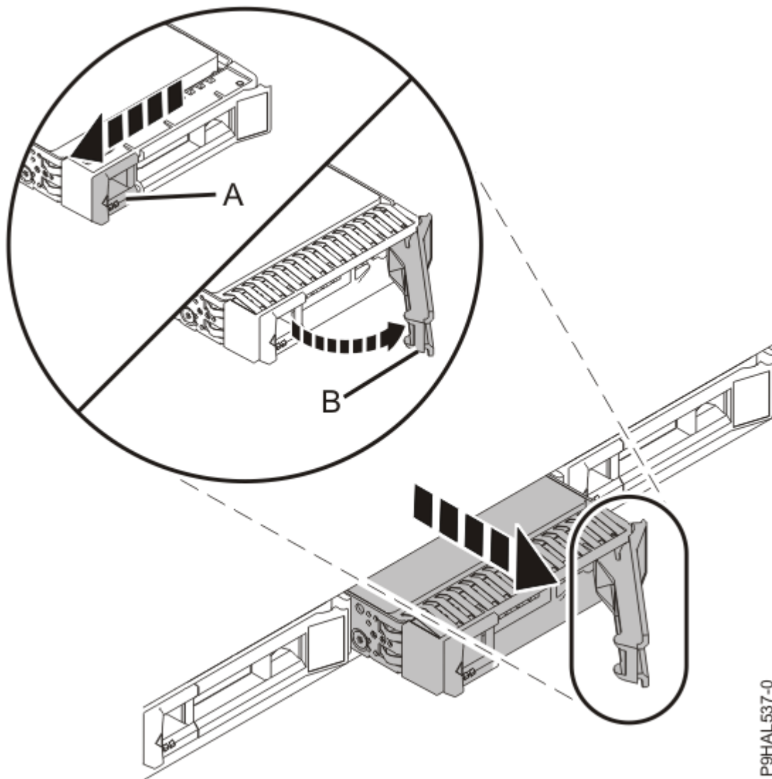
Figure 6. Déverrouillage et retrait de l'unité
