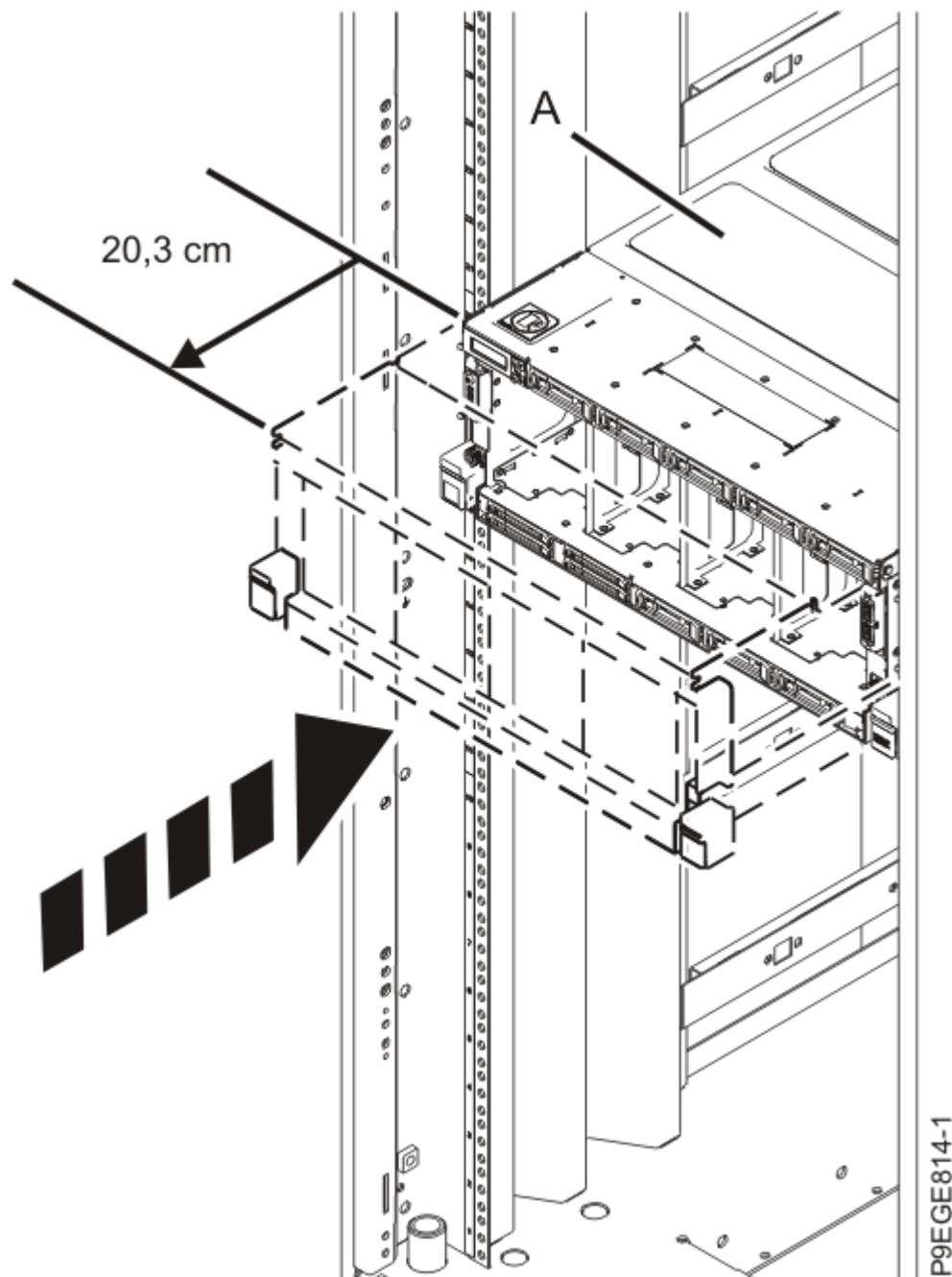
Figure 24. Mise en position de fonctionnement du système
