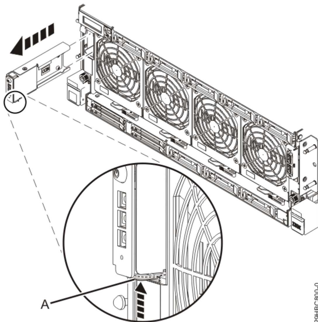
Figure 8. Retrait du panneau de commande
