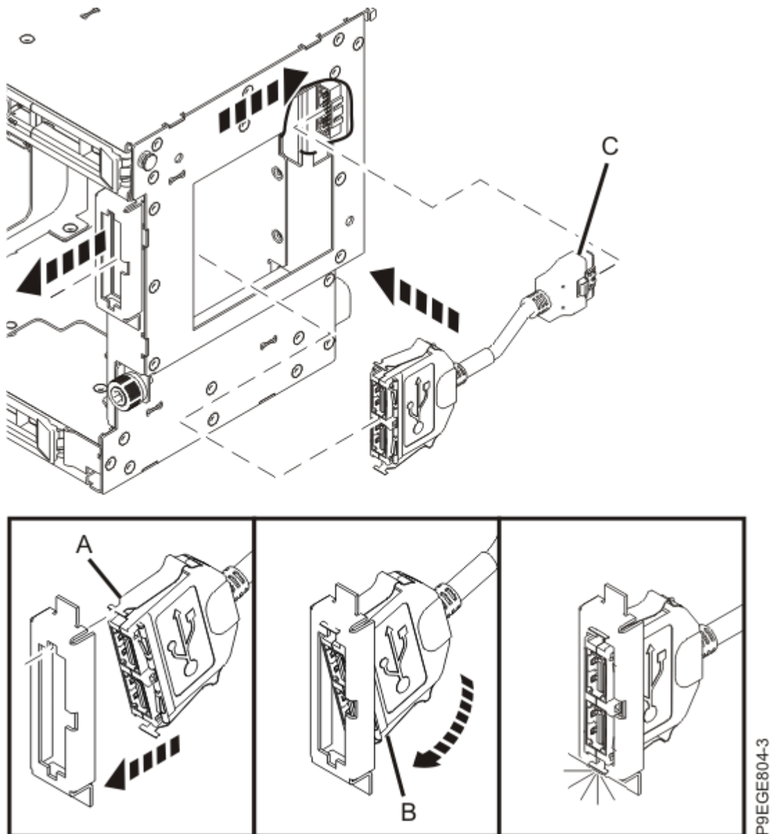
Figure 18. Remise en place du connecteur de port USB avant
