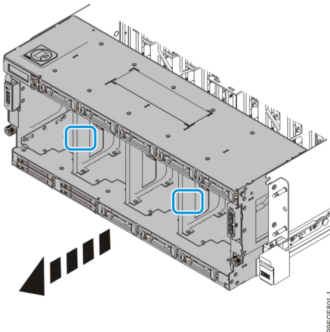
Figure 12. Retrait partiel du fond de panier d'unité de disque
