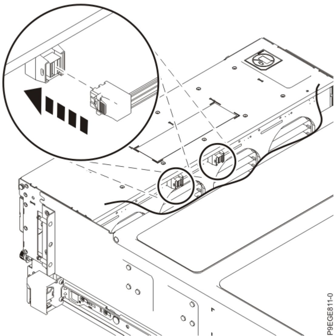
Figure 21. Connexion des câbles SAS au fond de panier d'unité de disque (fonction de base)
