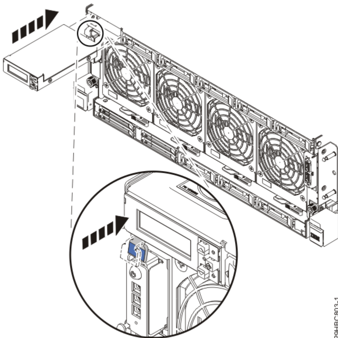
Figure 28. Remise en place de l'écran du panneau de commande
