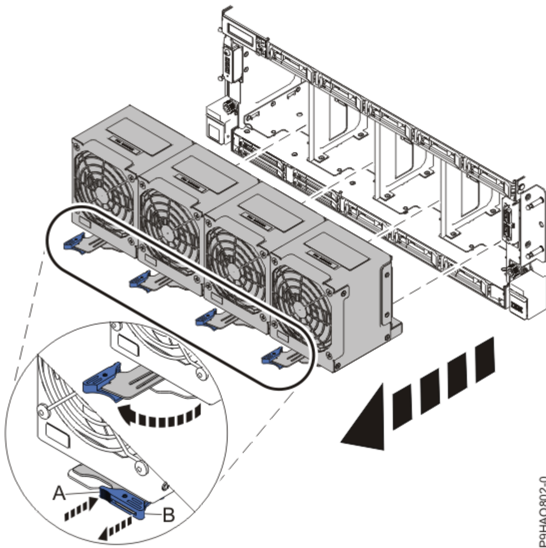
Figure 10. Retrait des ventilateurs
