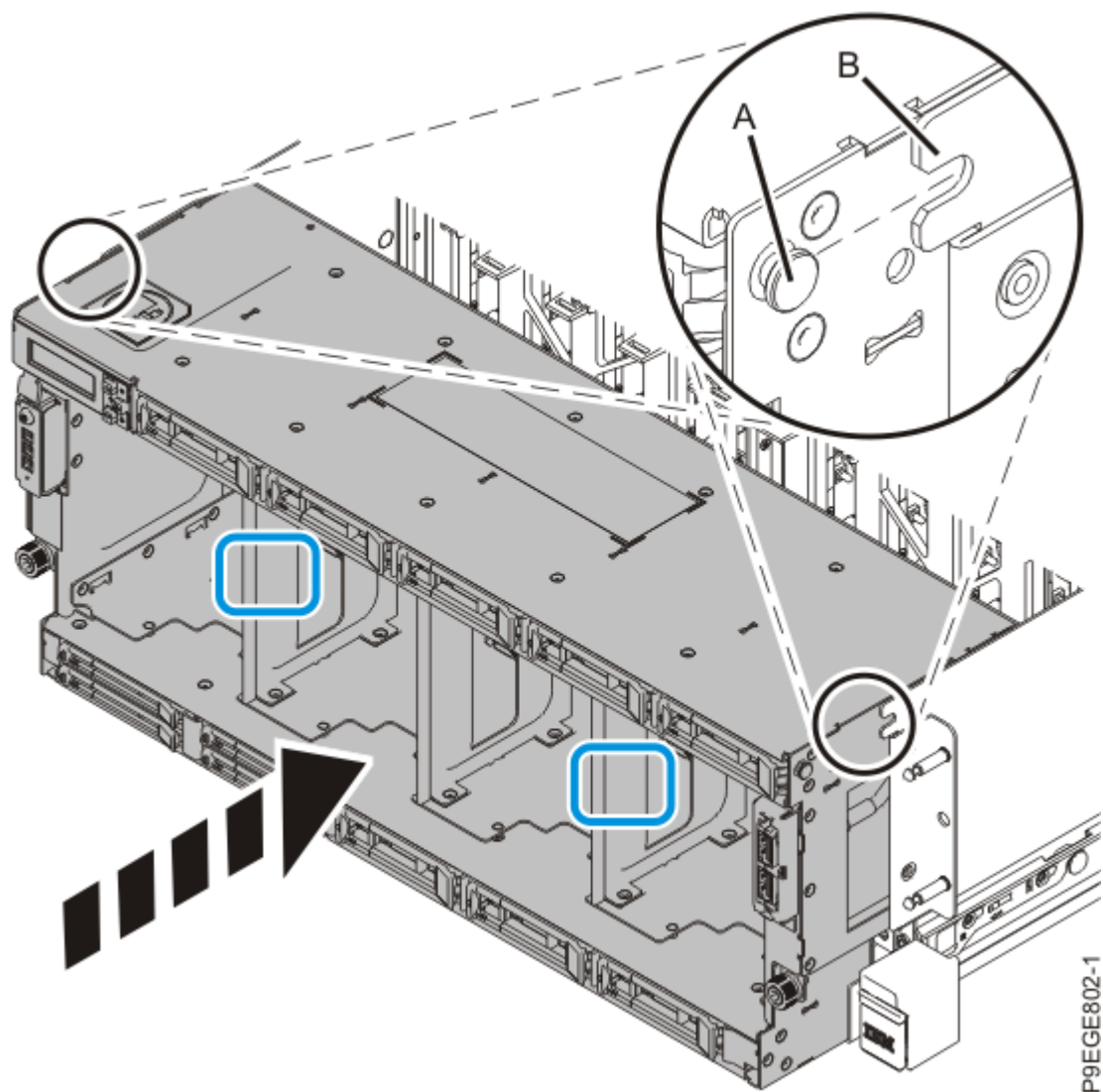
Figure 19. Remise en place partielle du fond de panier d'unité de disque
