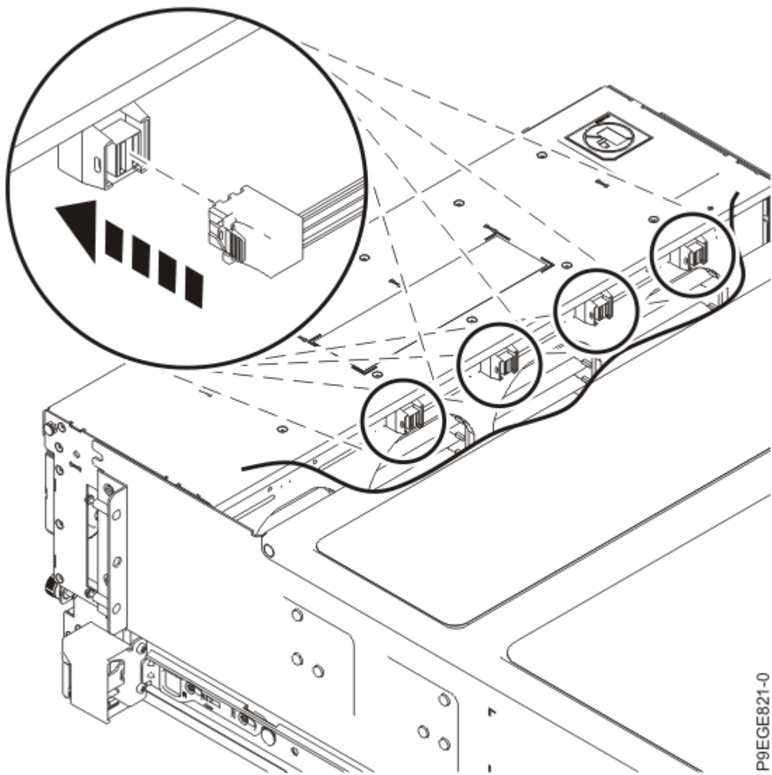
Figure 22. Connexion des câbles SAS au fond de panier d'unité de disque (fonction étendue)
