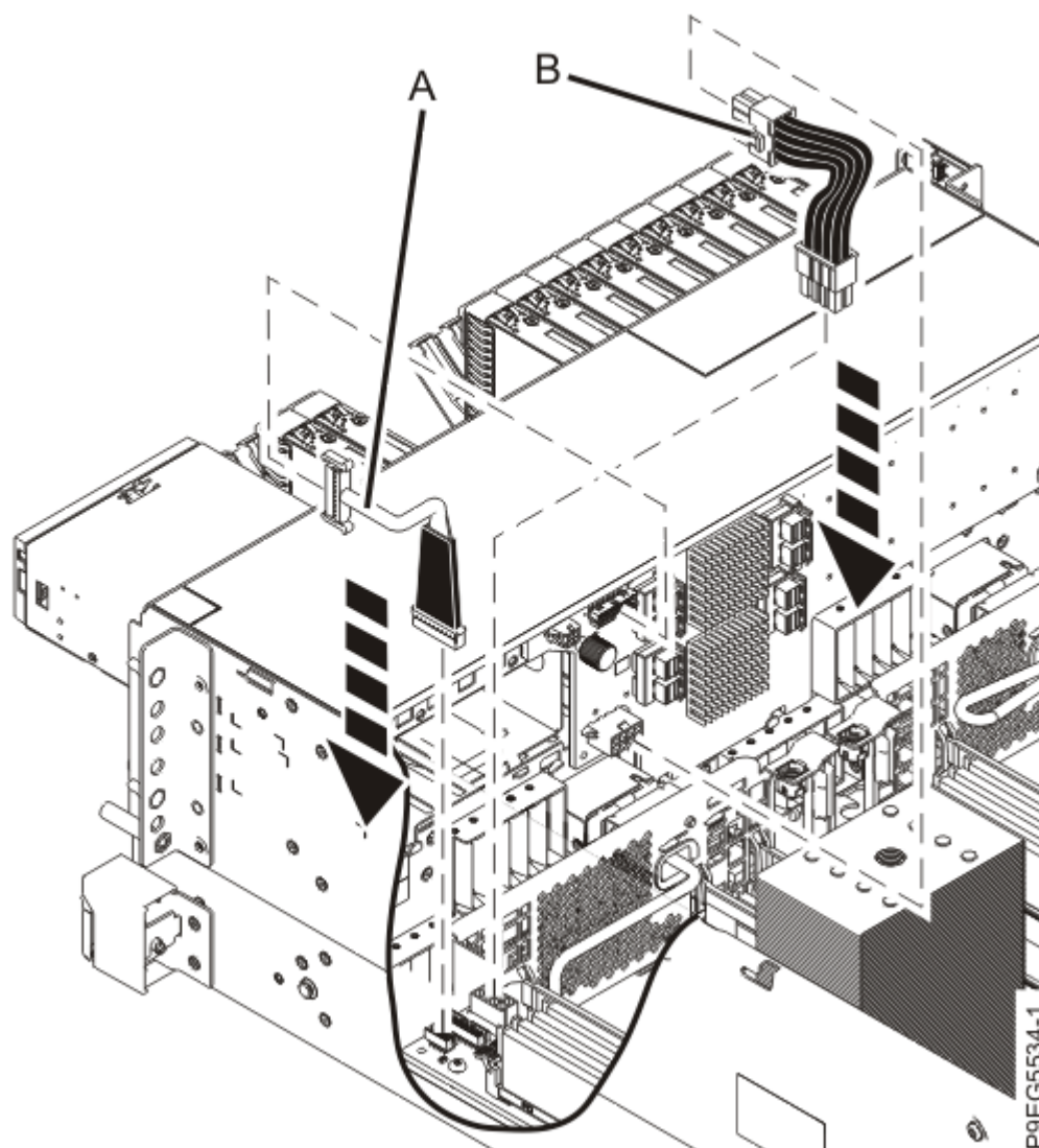
Figure 95. Reconnexion du câble d'alimentation et du cordon d'interface au fond de panier d'unité de disque
