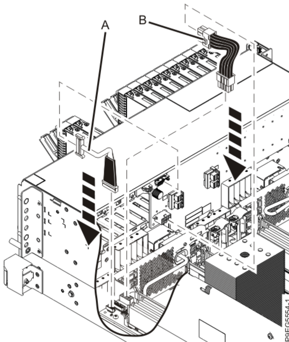
Figure 18. Reconnexion du câble d'alimentation et du cordon d'interface au fond de panier d'unité de disque
