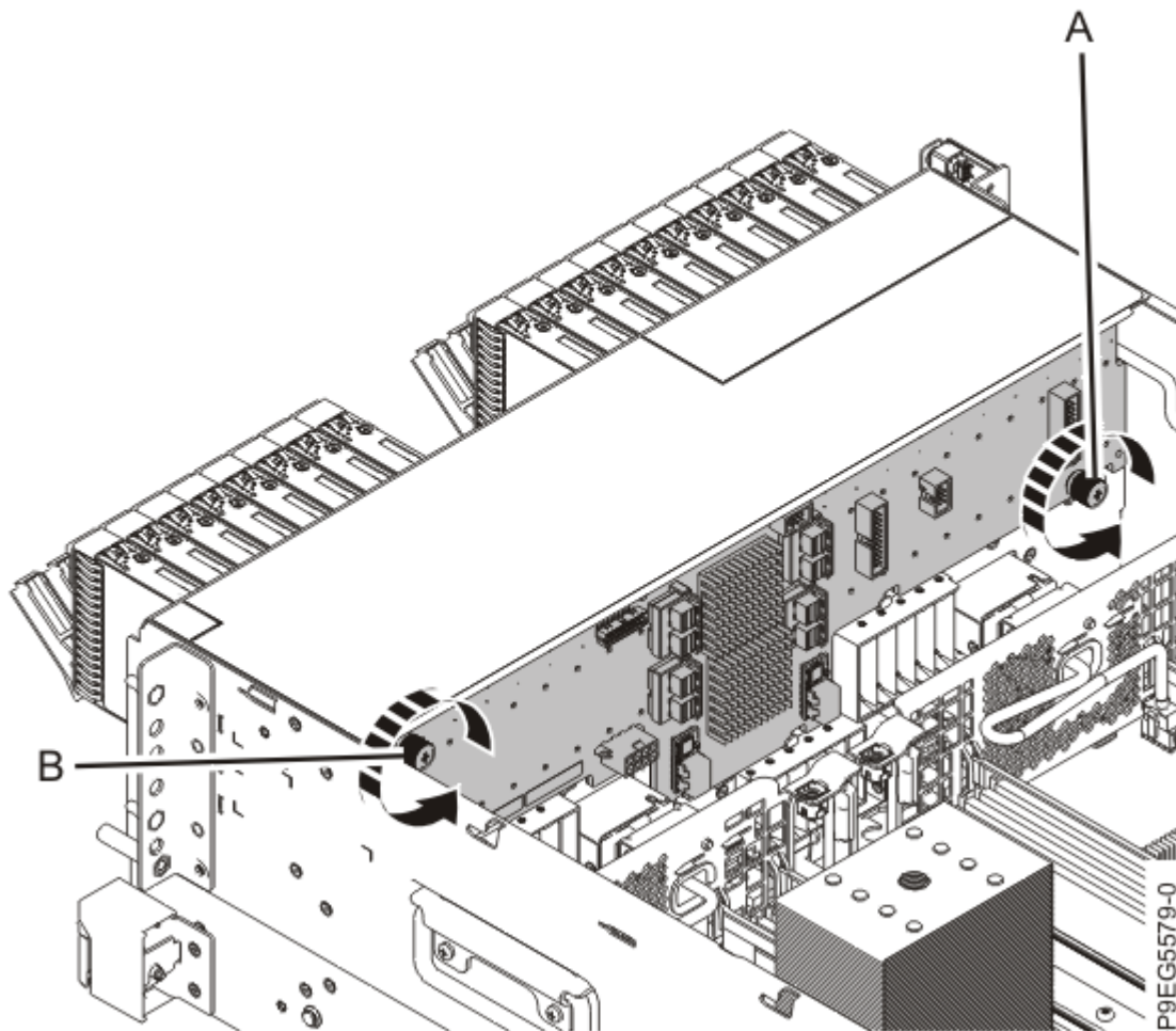
Figure 73. Desserrage des vis du fond de panier de l'unité de disque
