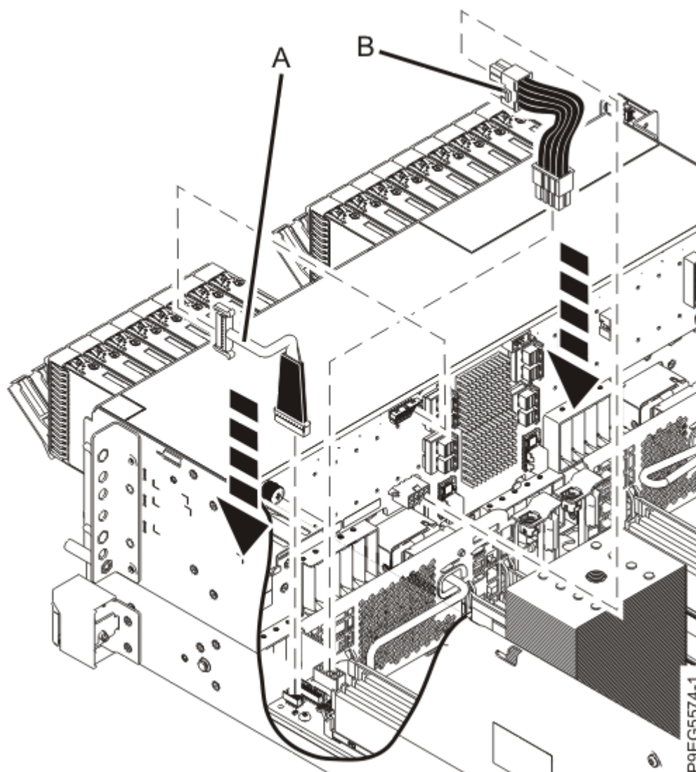
Figure 77. Reconnexion du câble d'alimentation et du cordon d'interface au fond de panier d'unité de disque
