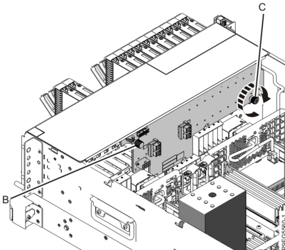
Figure 17. Remise en place du fond de panier d'unité de disque
