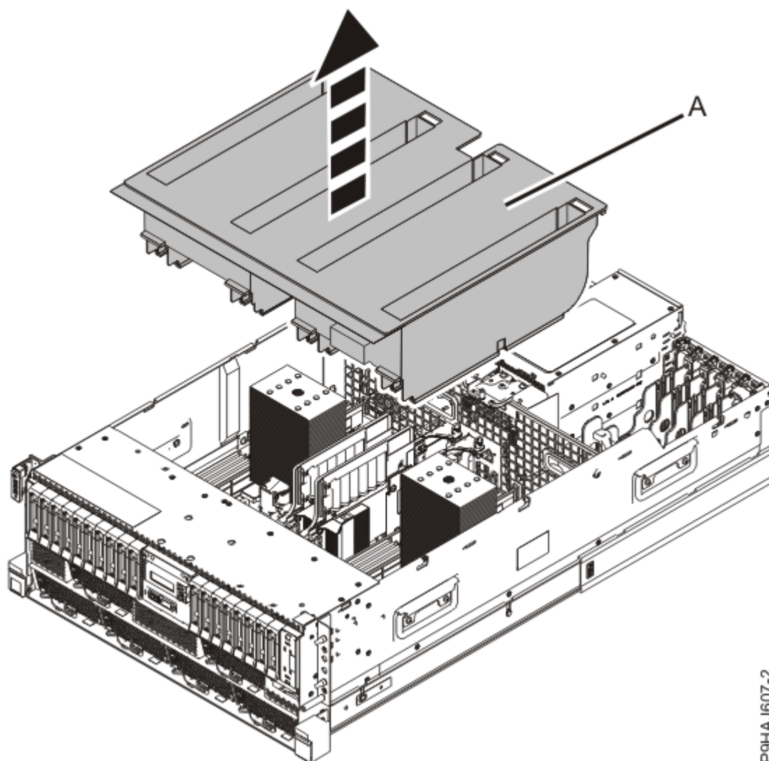
Figure 92. Retrait de la grille d'aération d'un système monté en armoire
