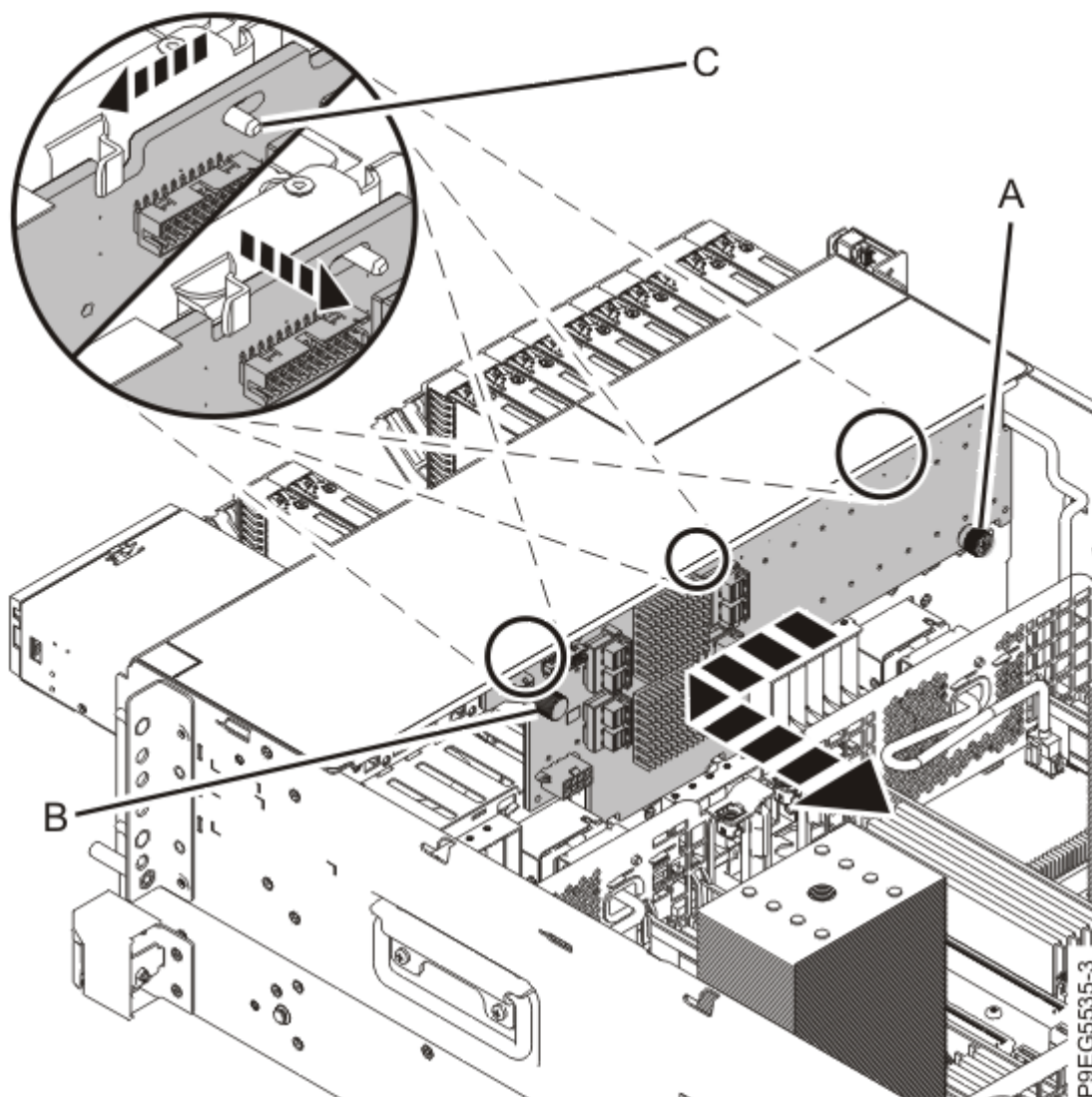
Figure 48. Retrait du fond de panier d'unité de disque
