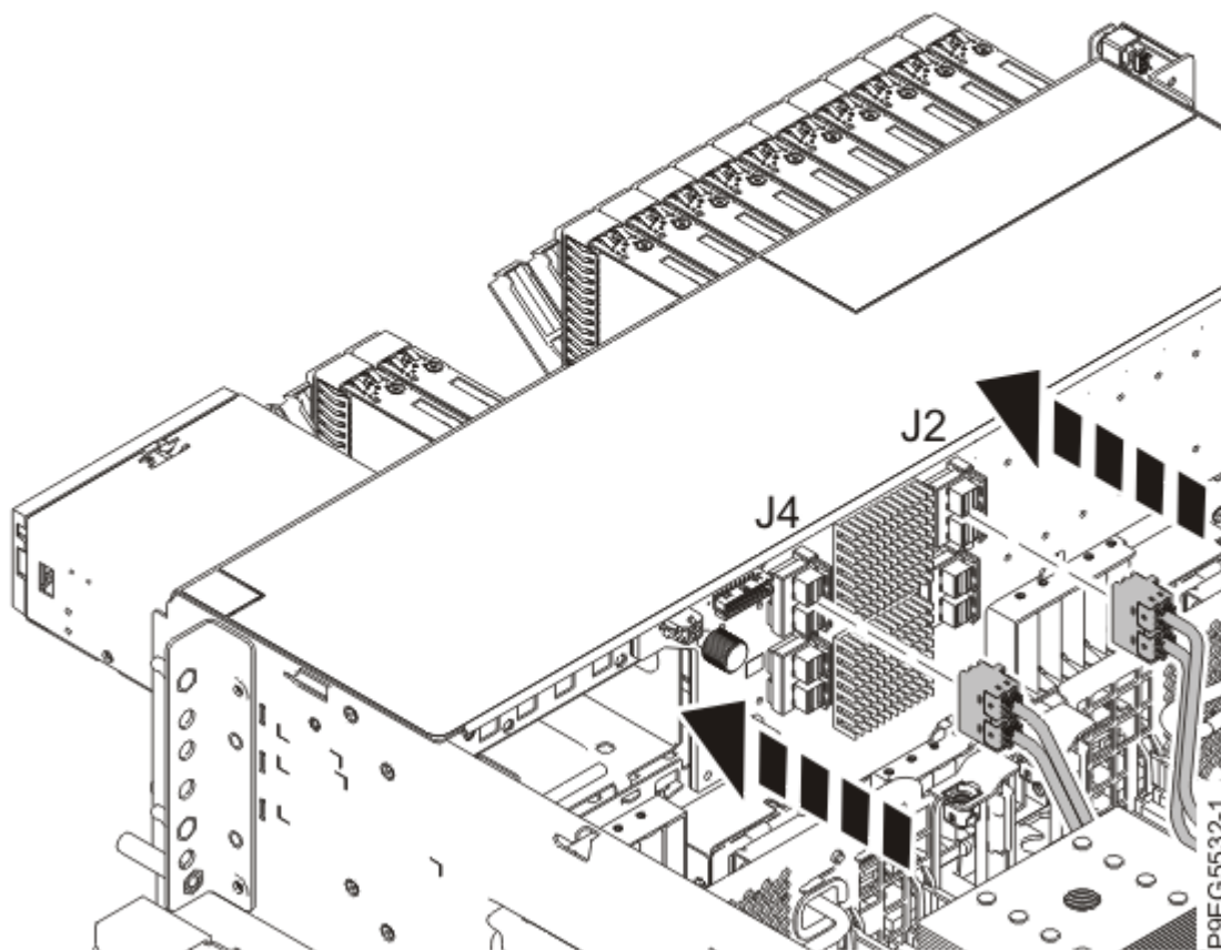
Figure 52. Reconnexion des câbles SAS avant
