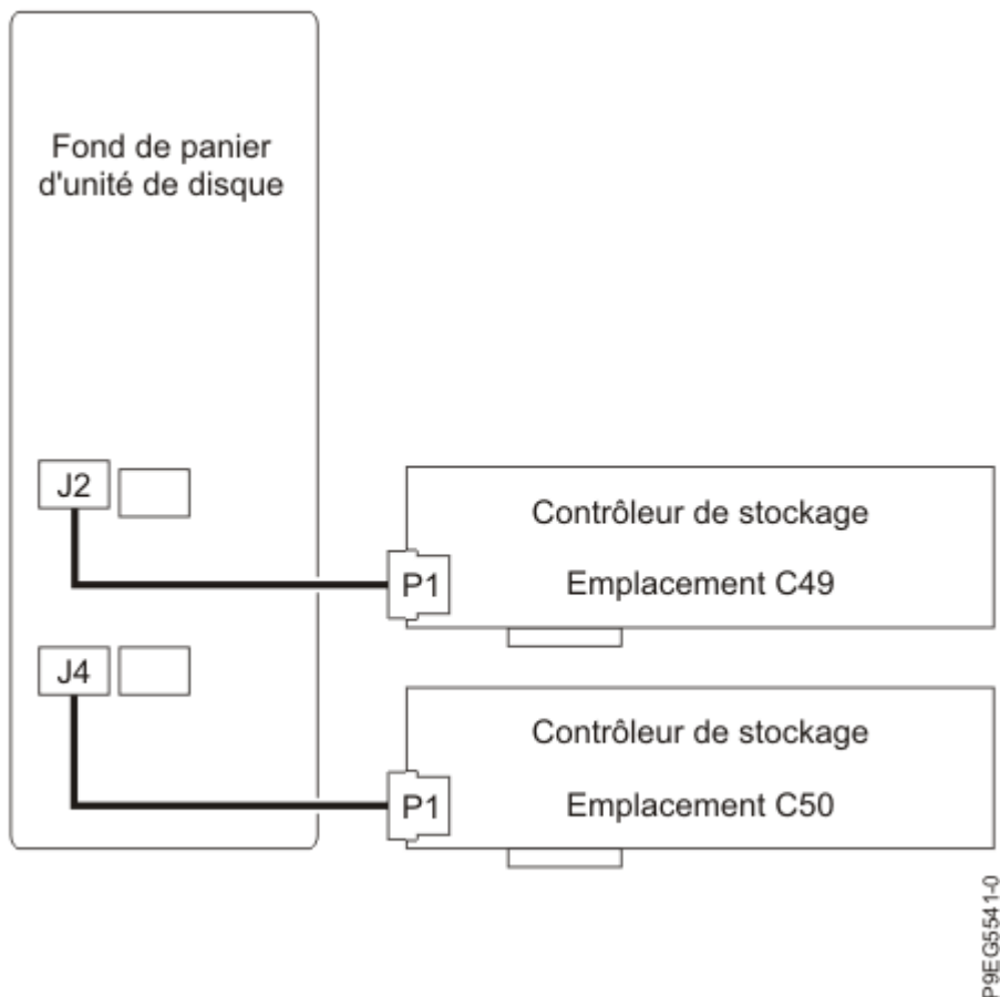
Figure 79. Reconnexion du câble SAS dans la configuration de fonction étendue 18 unités
