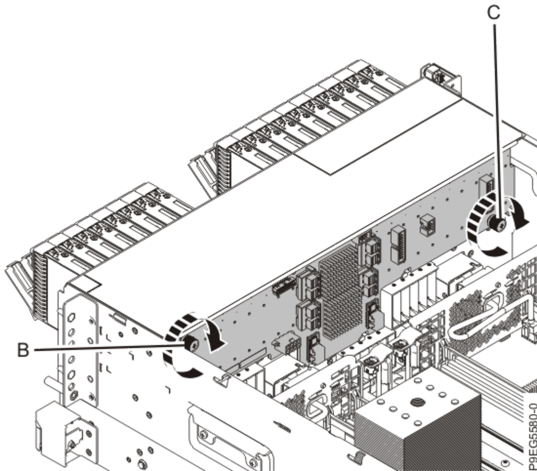
Figure 76. Remise en place du fond de panier d'unité de disque
