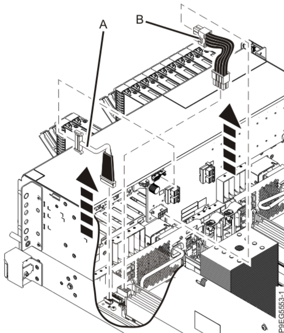
Figure 13. Déconnexion du cordon d'interface et du câble d'alimentation
