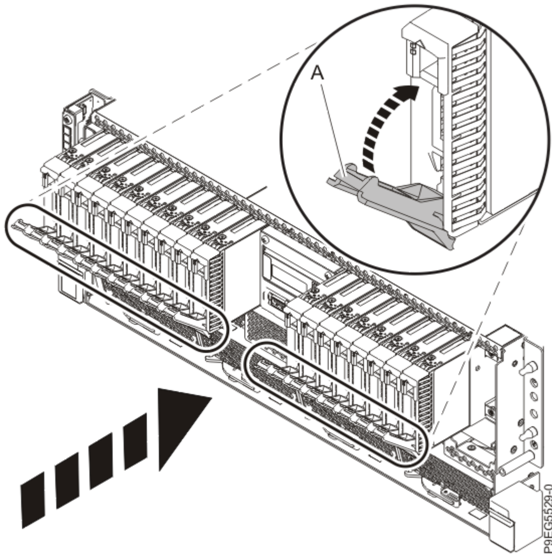
Figure 80. Remise en place des unités frontales
