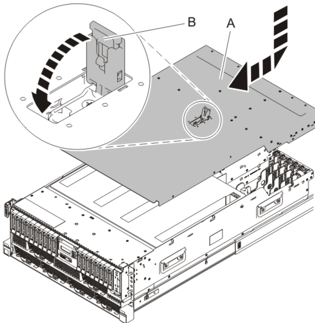
Figure 29. Installation du capot d'accès
