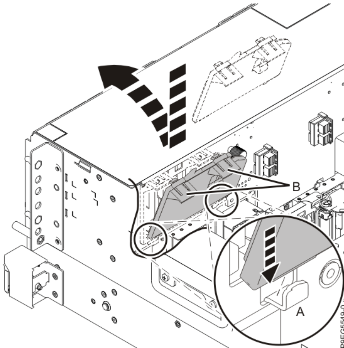
Figure 58. Remise en place de l'obturateur d'unité RDX
