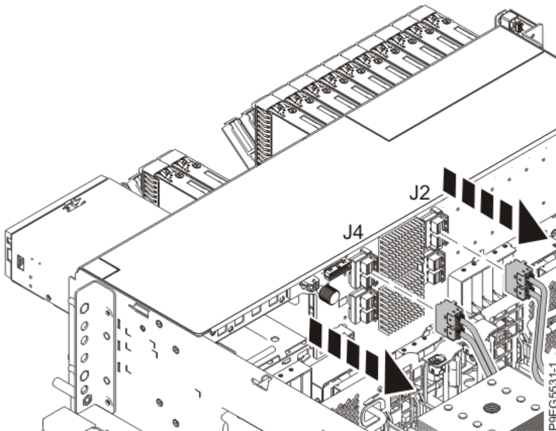
Figure 46. Déconnexion des câbles SAS avant
