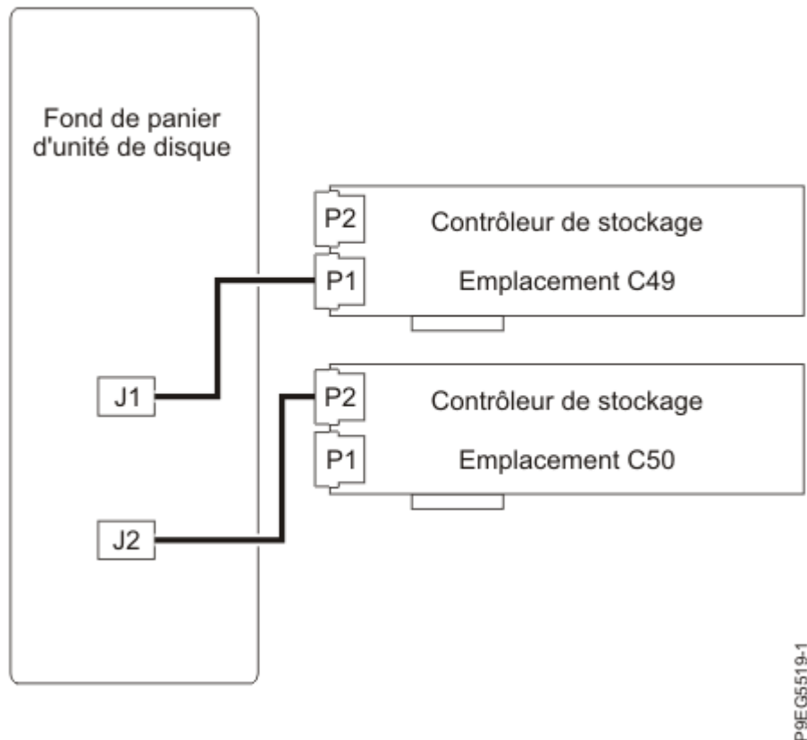
Figure 21. Reconnexion du câble SAS dans une configuration de disque partagé
