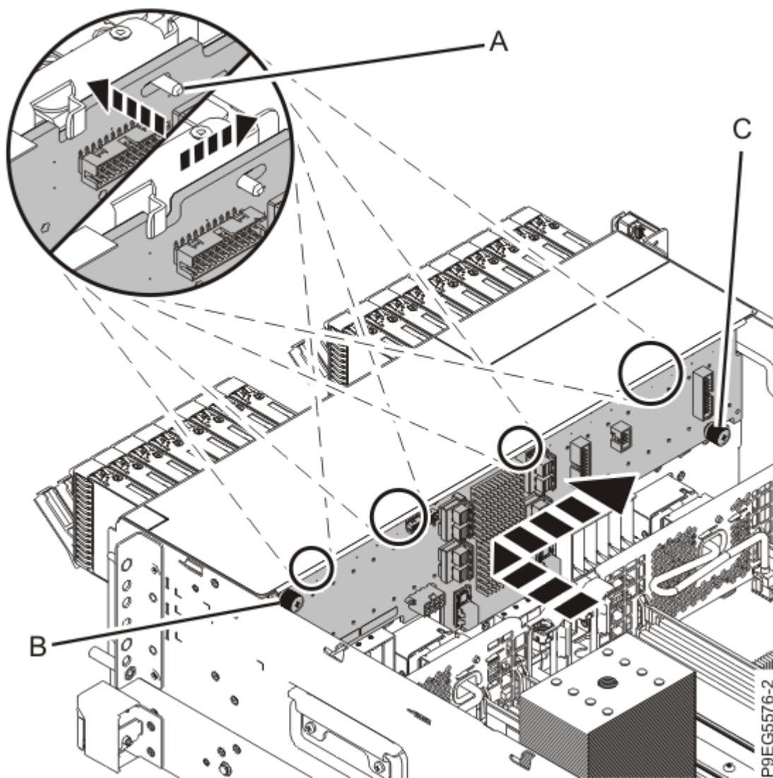
Figure 75. Remise en place du fond de panier d'unité de disque à l'aide des broches d'alignement
