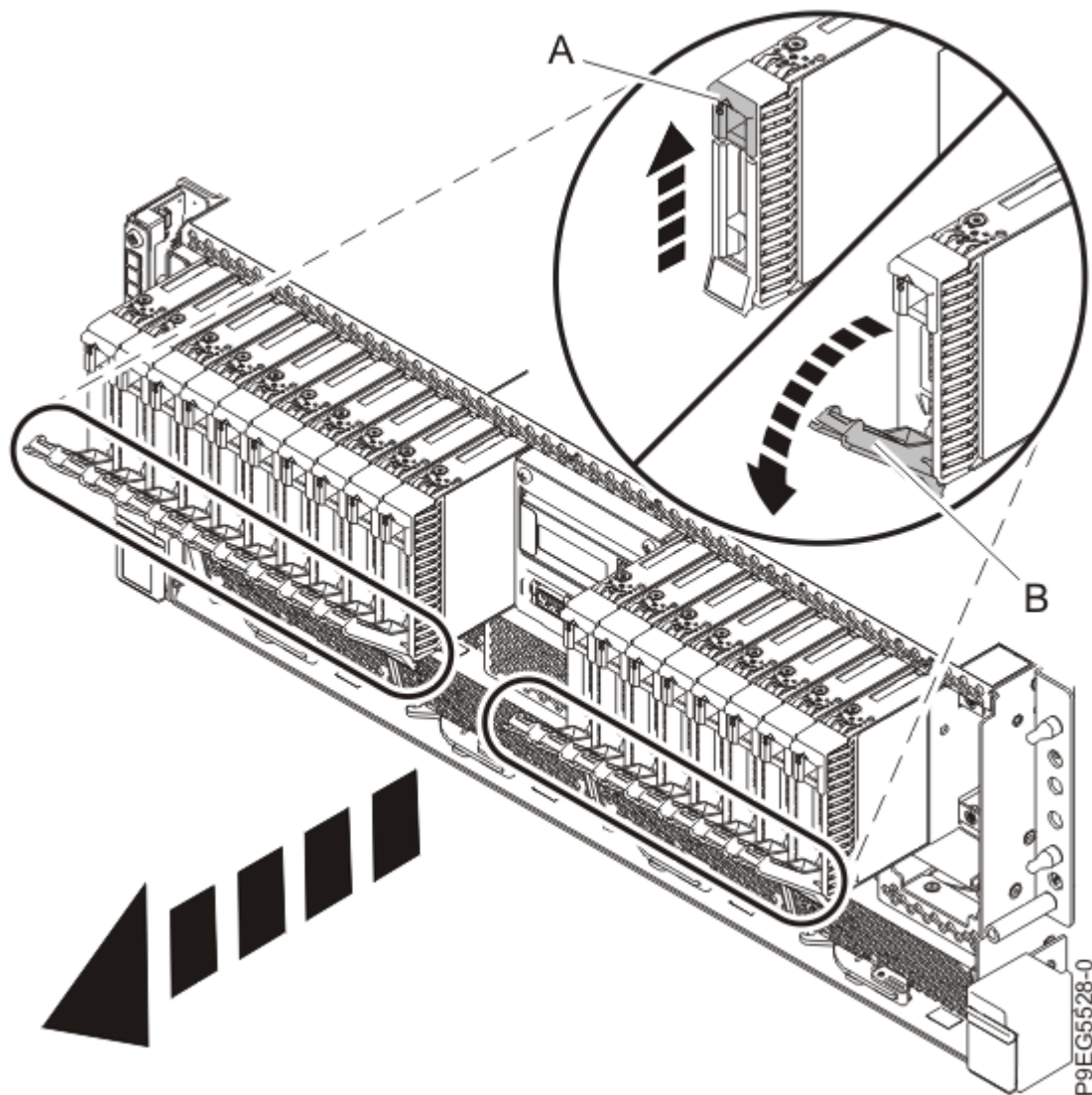
Figure 70. Retrait partiel des unités frontales
