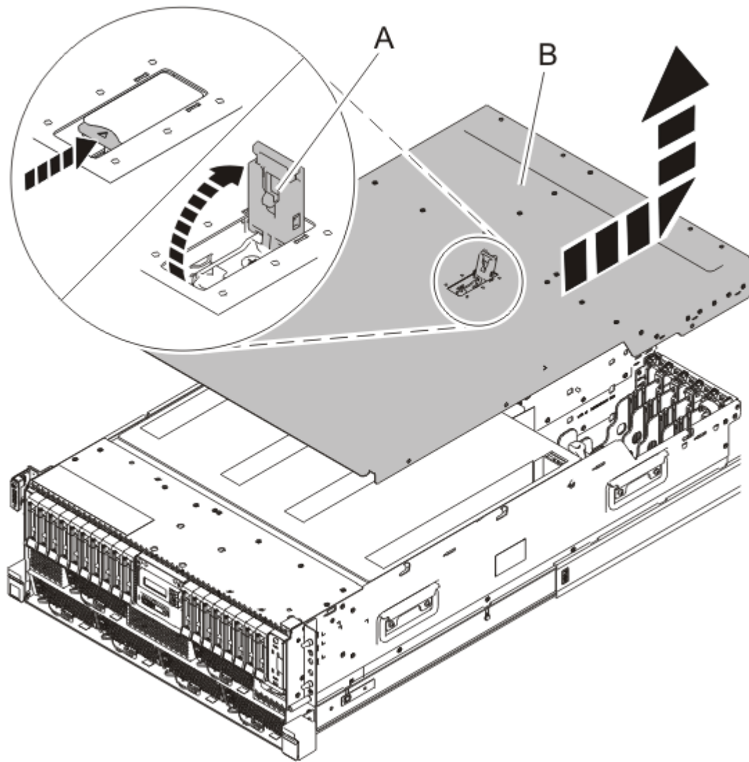
Figure 68. Retrait du capot d'accès d'un système monté en armoire
