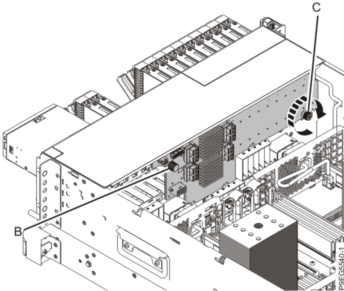
Figure 50. Remplacement du fond de panier d'unité de disque
