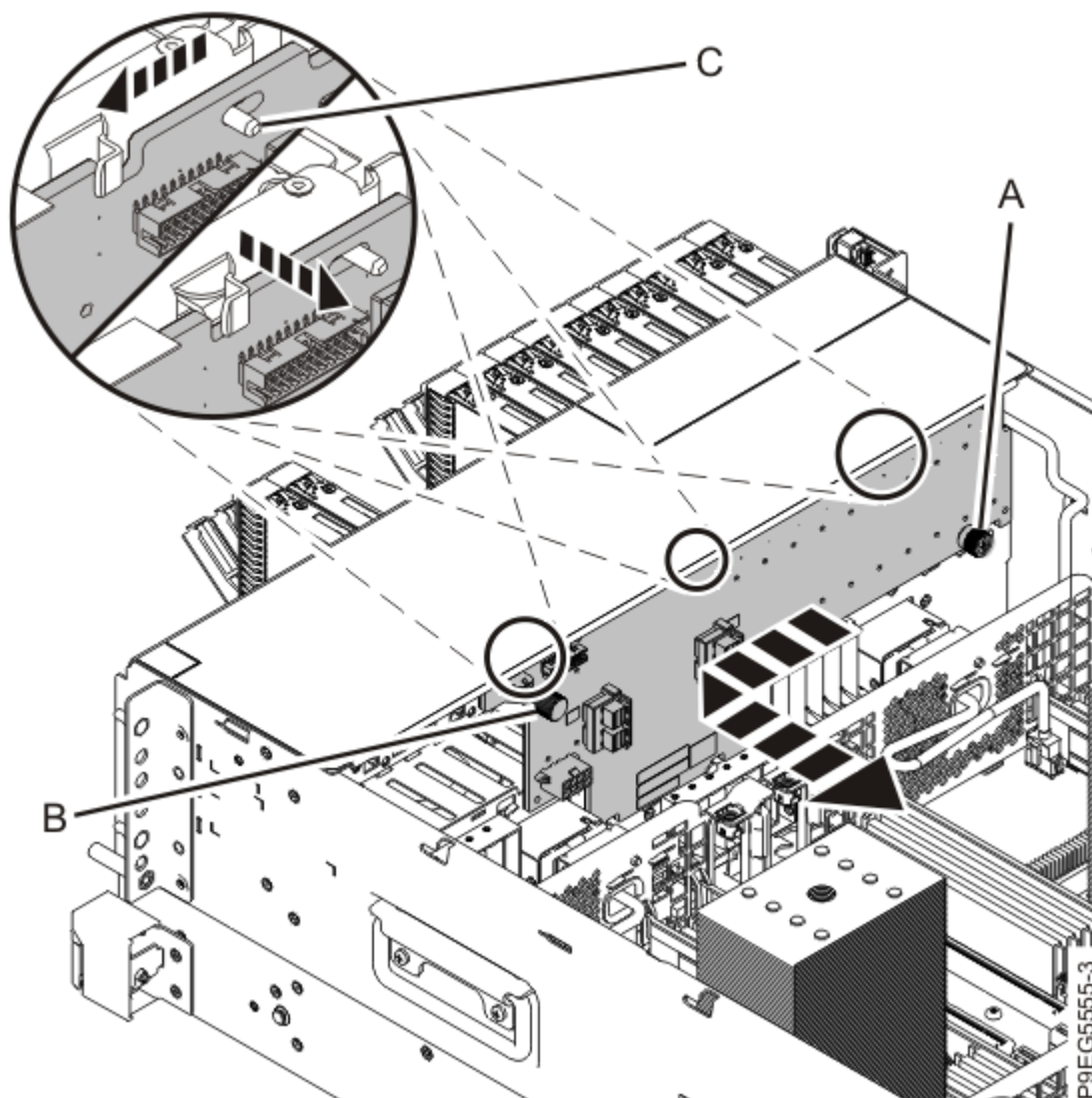
Figure 15. Retrait du fond de panier d'unité de disque
