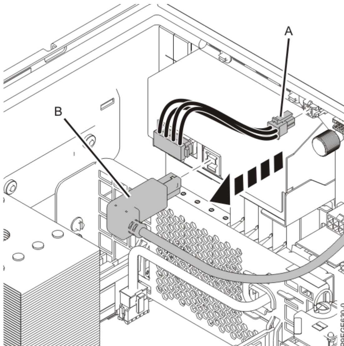
Figure 8. Déconnexion du câble d'alimentation RDX et du câble USB
