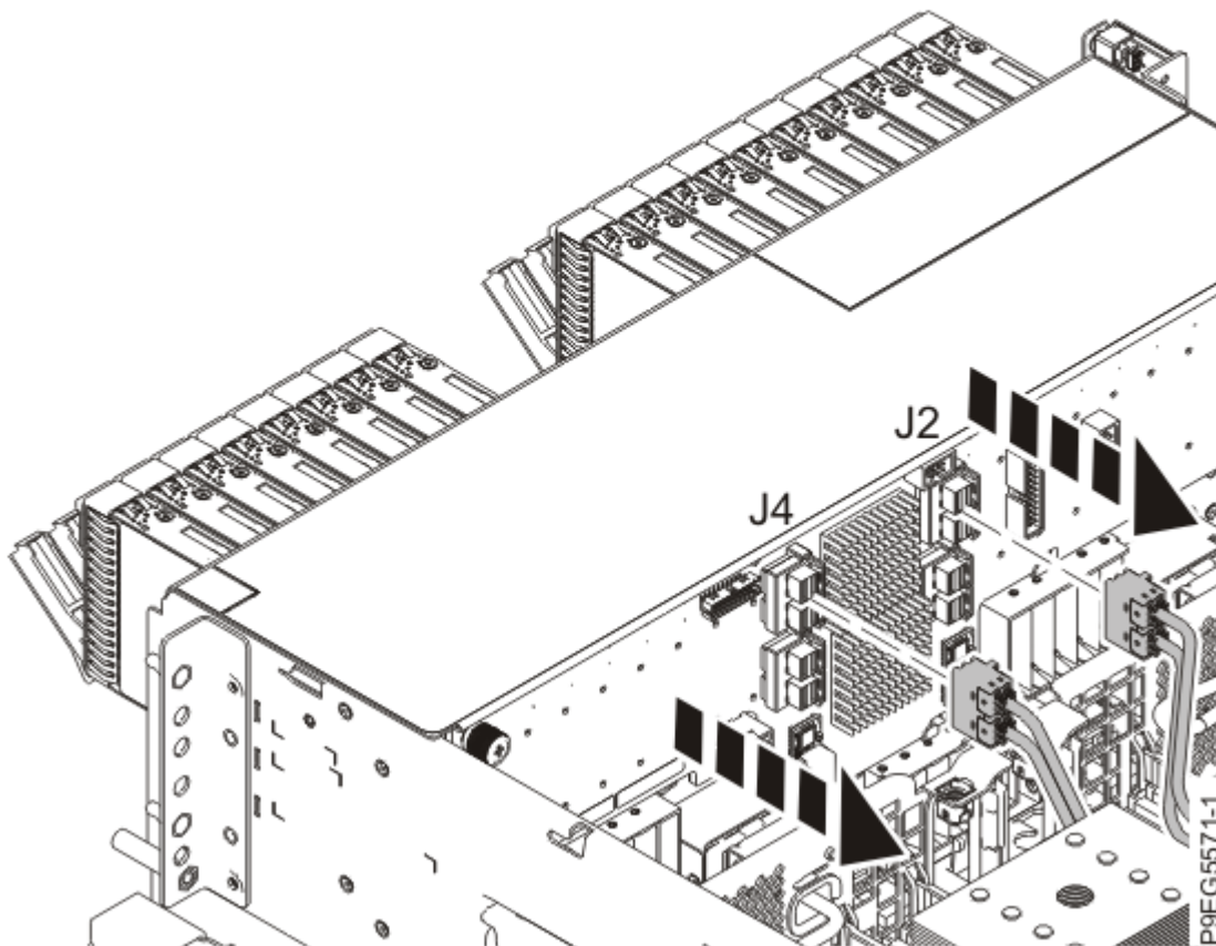
Figure 72. Déconnexion des câbles SAS frontaux
