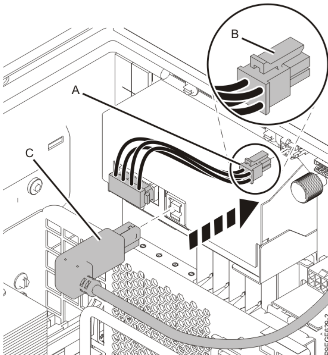
Figure 56. Reconnexion du câble d'alimentation RDX et du câble USB
