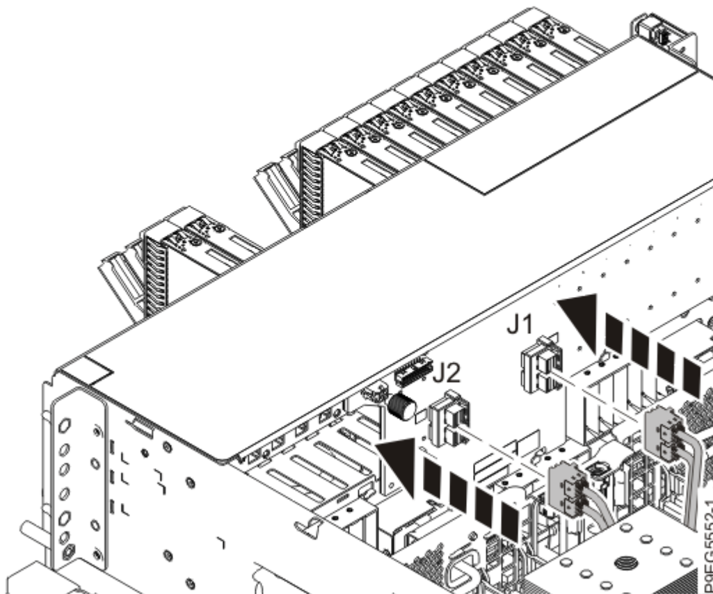
Figure 19. Reconnexion des câbles SAS avant
