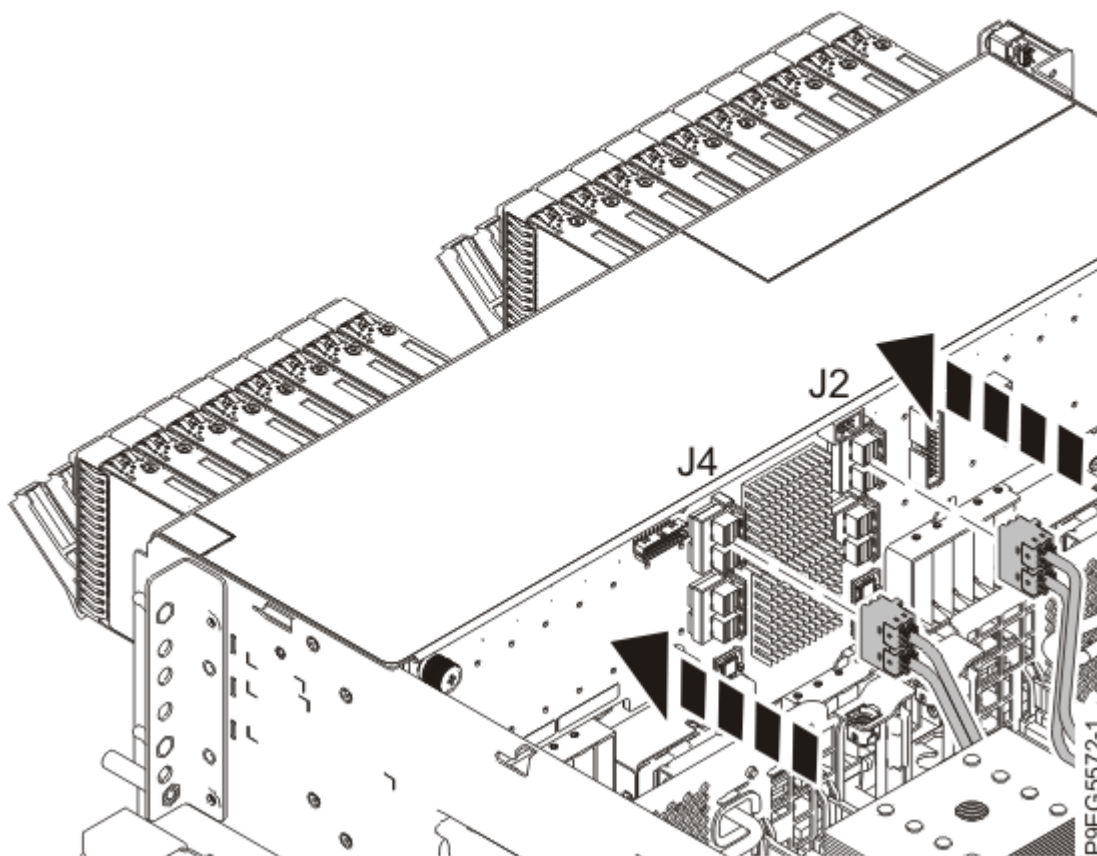
Figure 78. Reconnexion des câbles SAS avant
