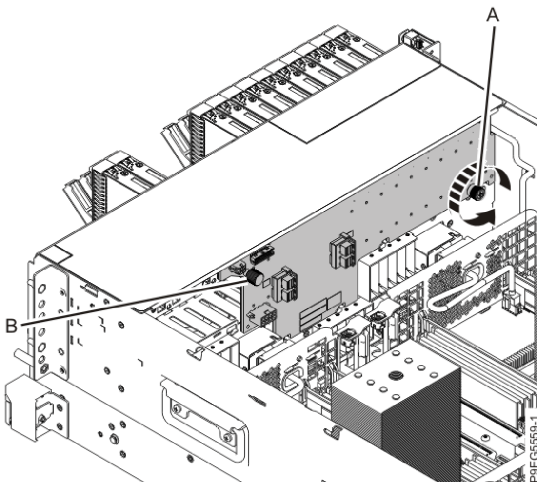
Figure 14. Desserrage de la vis du fond de panier de l'unité de disque
