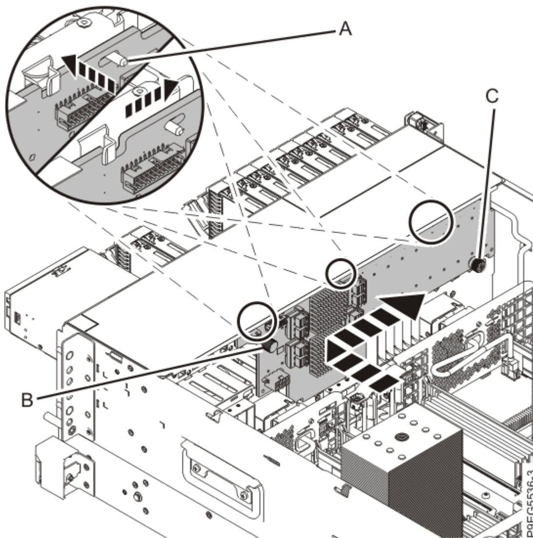
Figure 49. Remise en place du fond de panier d'unité de disque à l'aide des broches d'alignement
