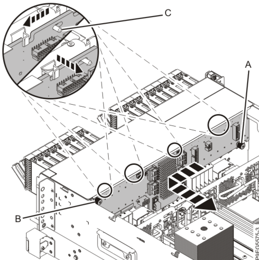
Figure 74. Retrait du fond de panier d'unité de disque
