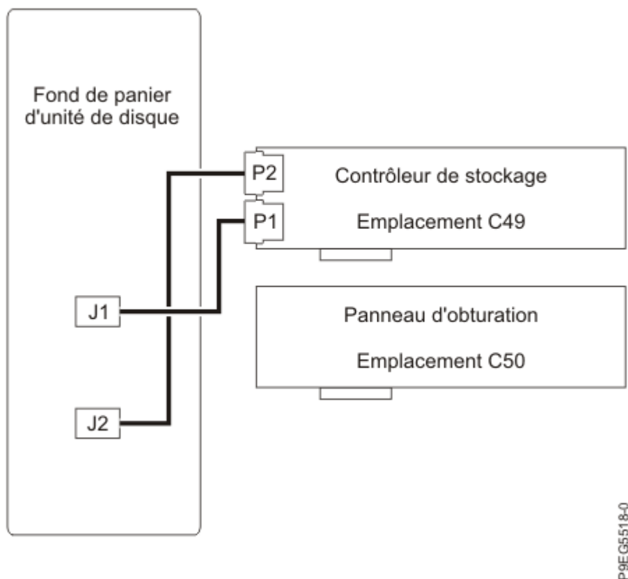
Figure 20. Reconnexion du câble SAS dans une configuration de stockage de base
