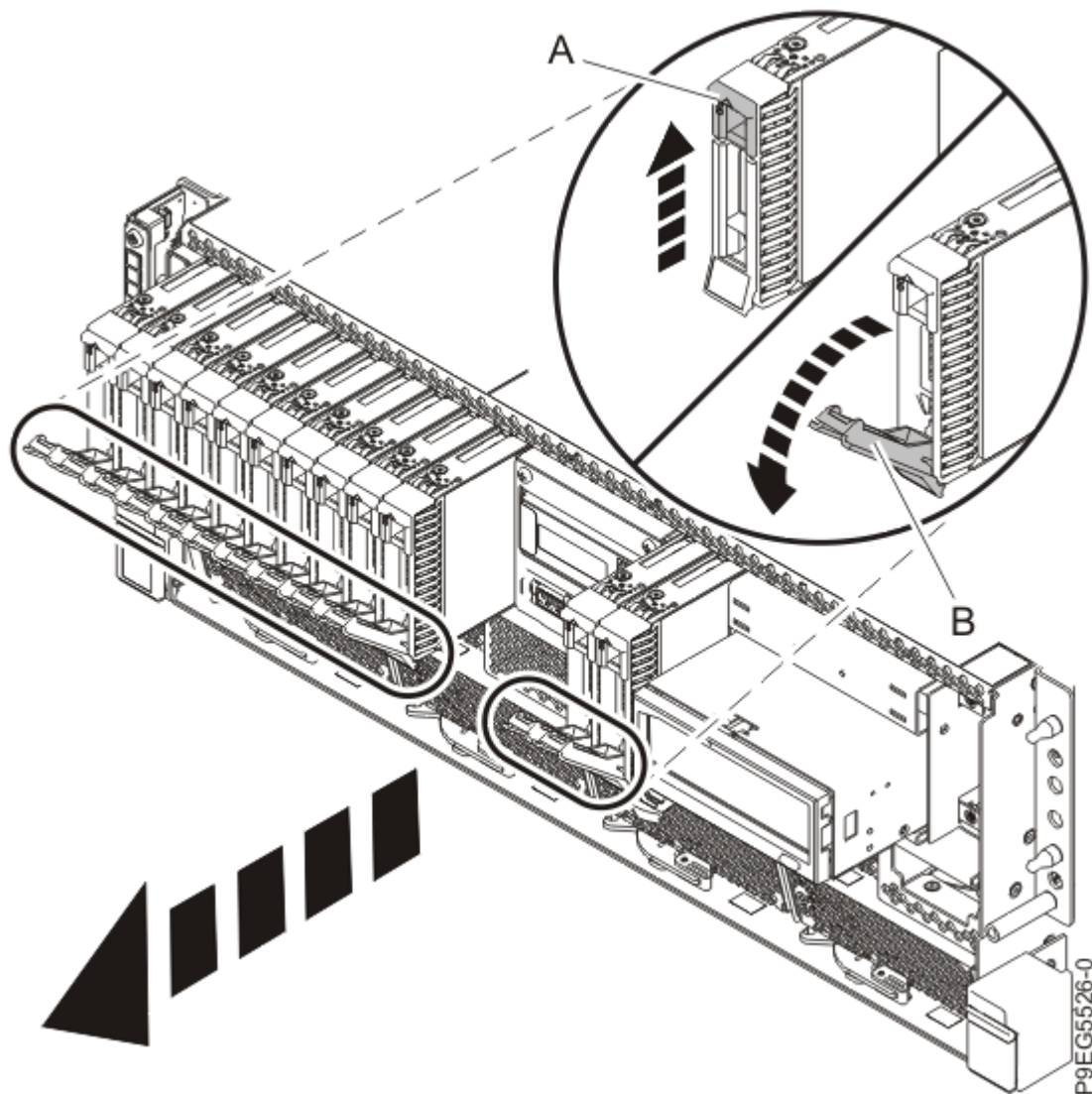
Figure 44. Retrait partiel des unités frontales
