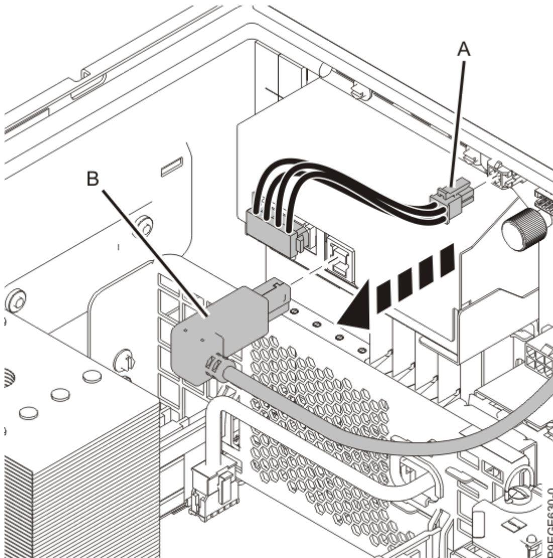
Figure 41. Déconnexion du câble d'alimentation RDX et du câble USB
