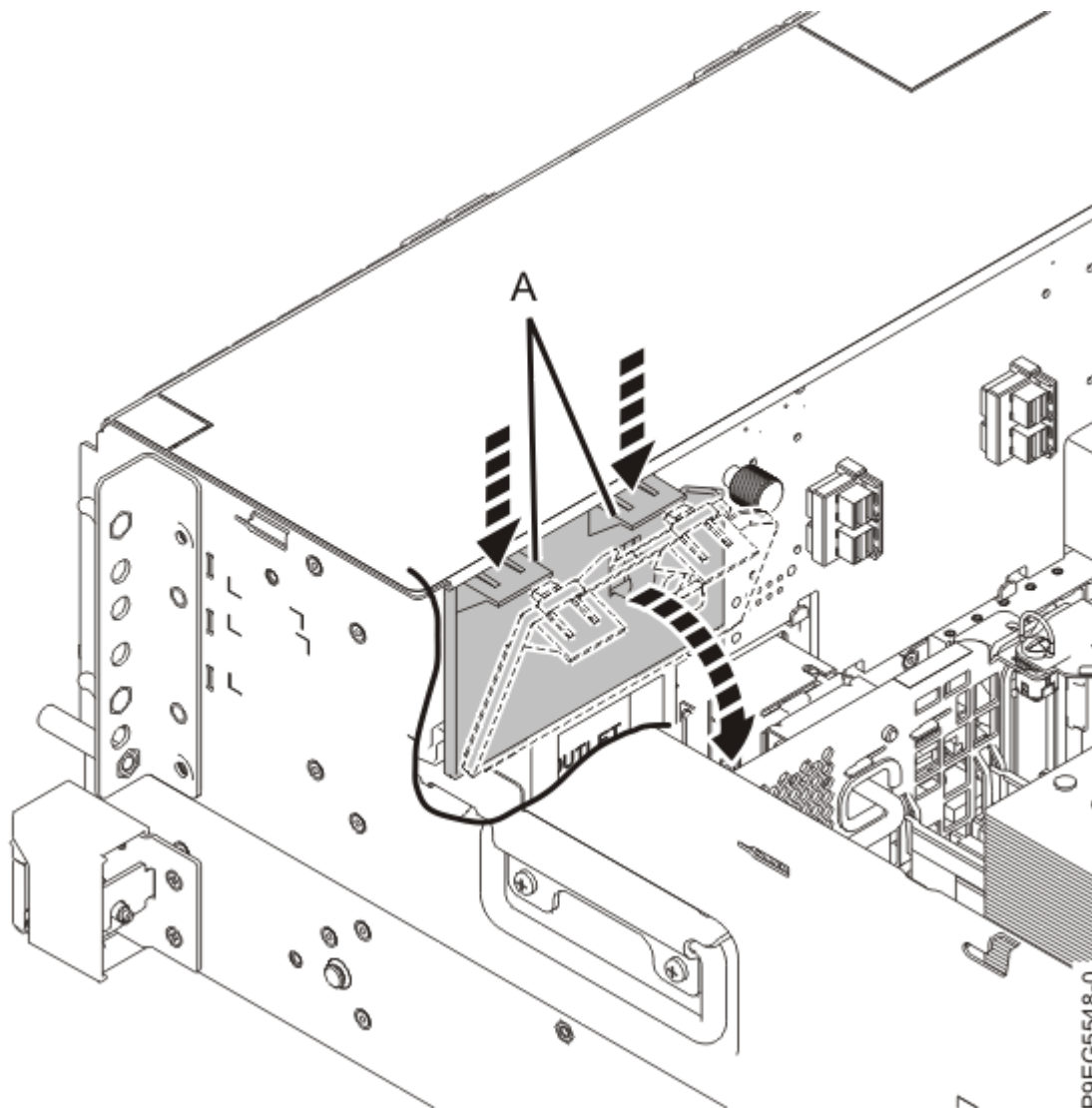
Figure 43. Retrait de l'obturateur d'unité RDX
