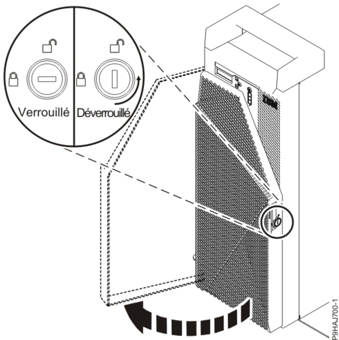
Figure 7. Déverrouillage du volet avant
