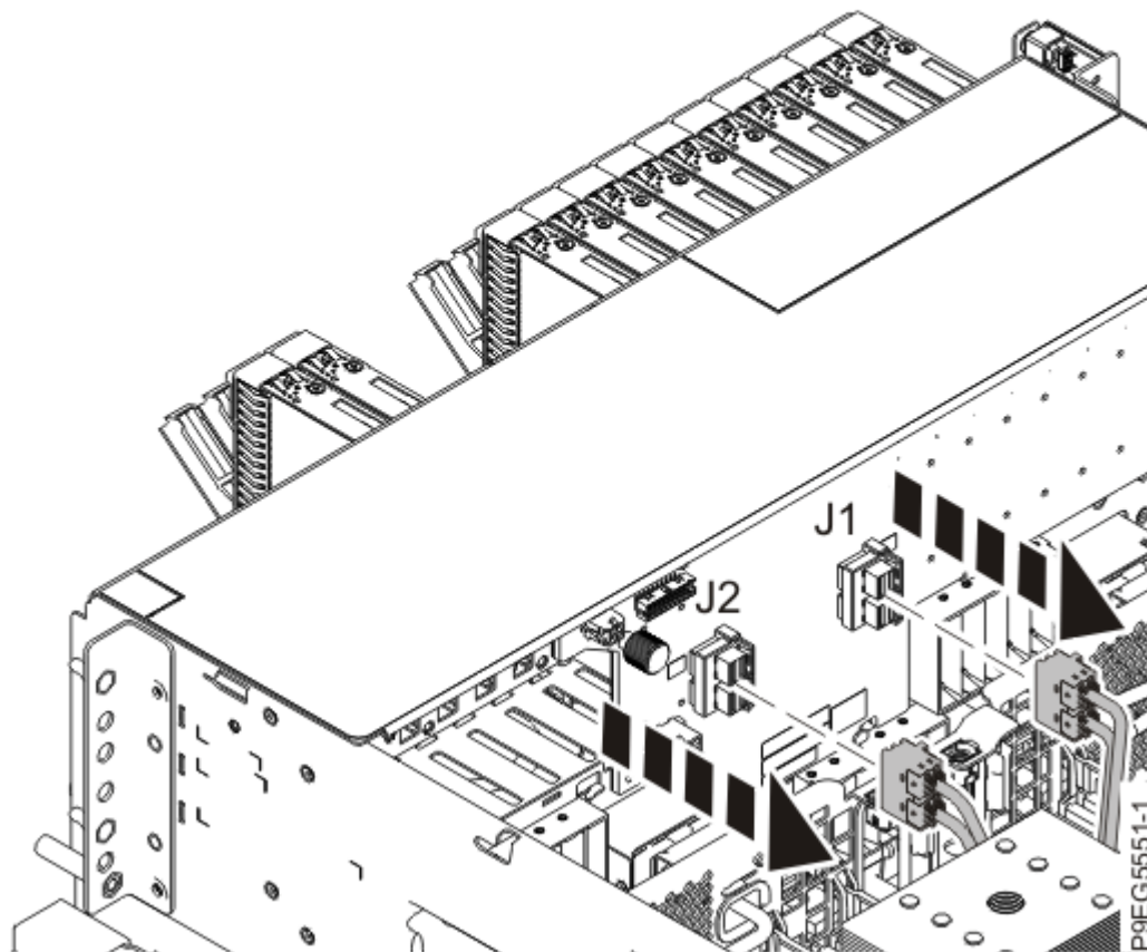
Figure 12. Déconnexion des câbles SAS frontaux
