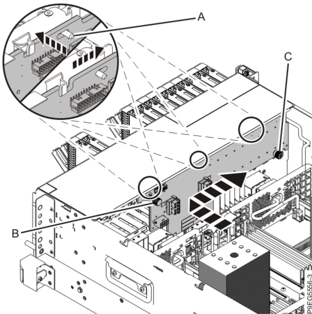
Figure 16. Remise en place du fond de panier d'unité de disque à l'aide des broches d'alignement
