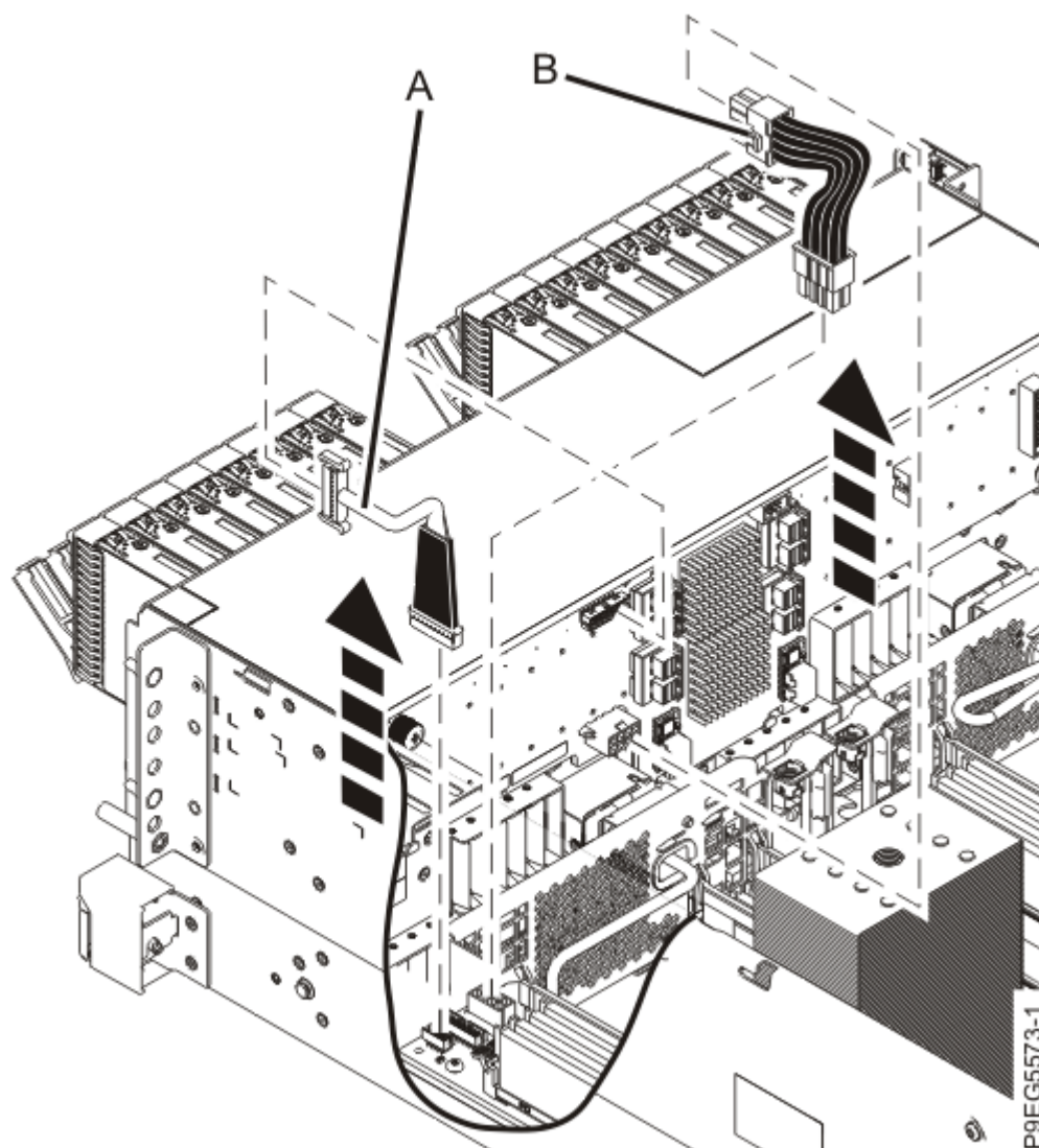
Figure 71. Déconnexion du cordon d'interface et du câble d'alimentation
