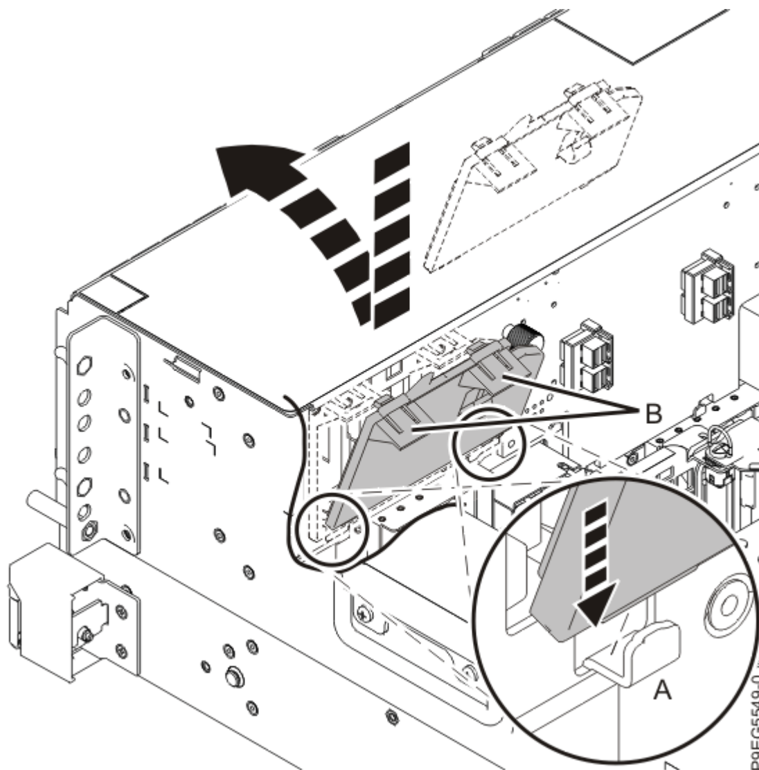
Figure 26. Remise en place de l'obturateur d'unité RDX
