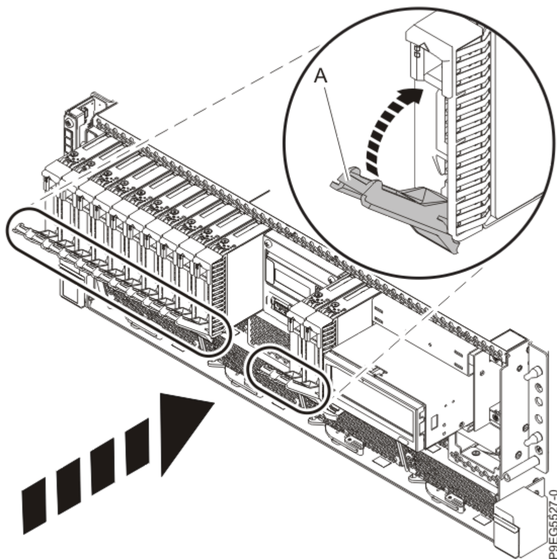
Figure 22. Remise en place des unités frontales
