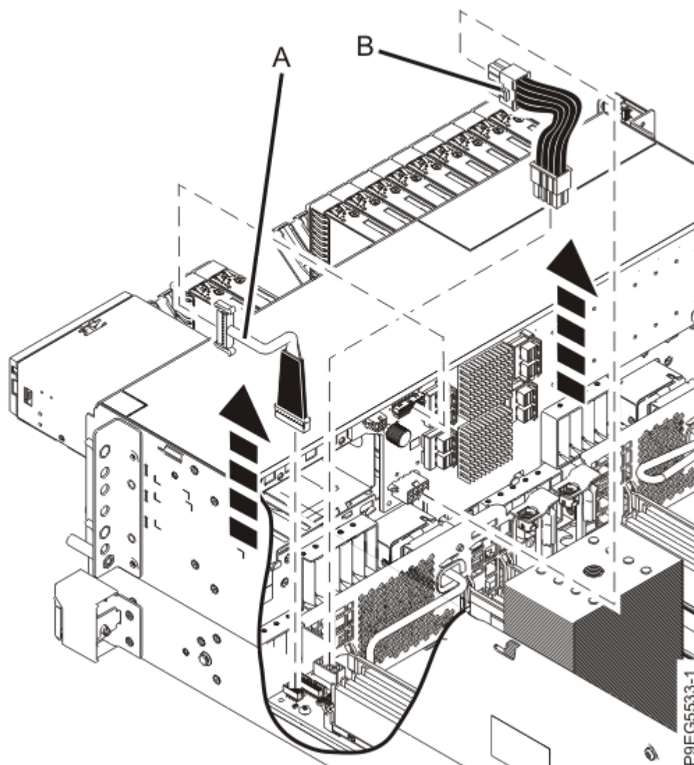
Figure 45. Déconnexion du cordon d'interface et du câble d'alimentation
