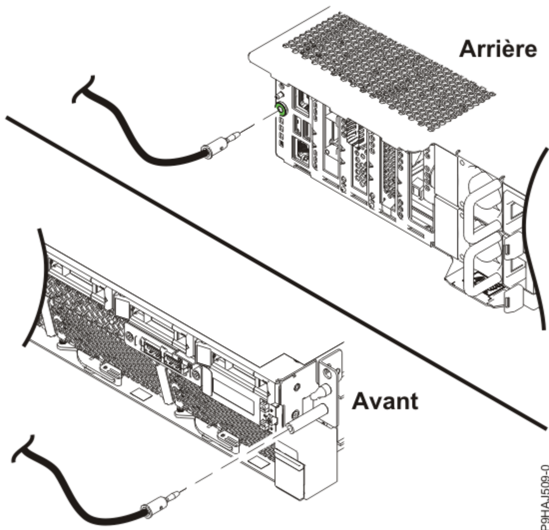
Figure 3. Emplacement des fiches de décharge électrostatique
