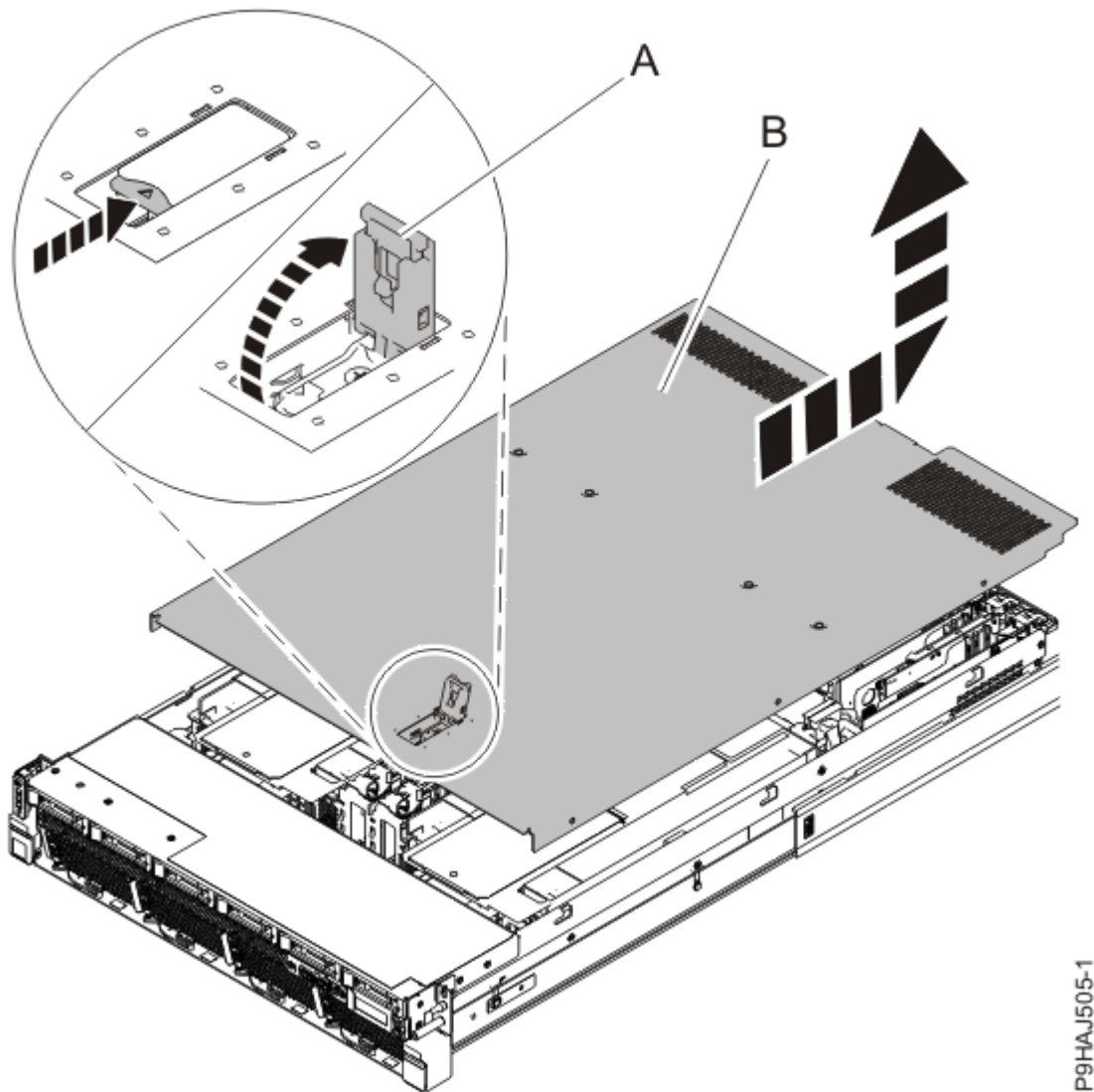
Figure 4. Retrait du capot d'accès
