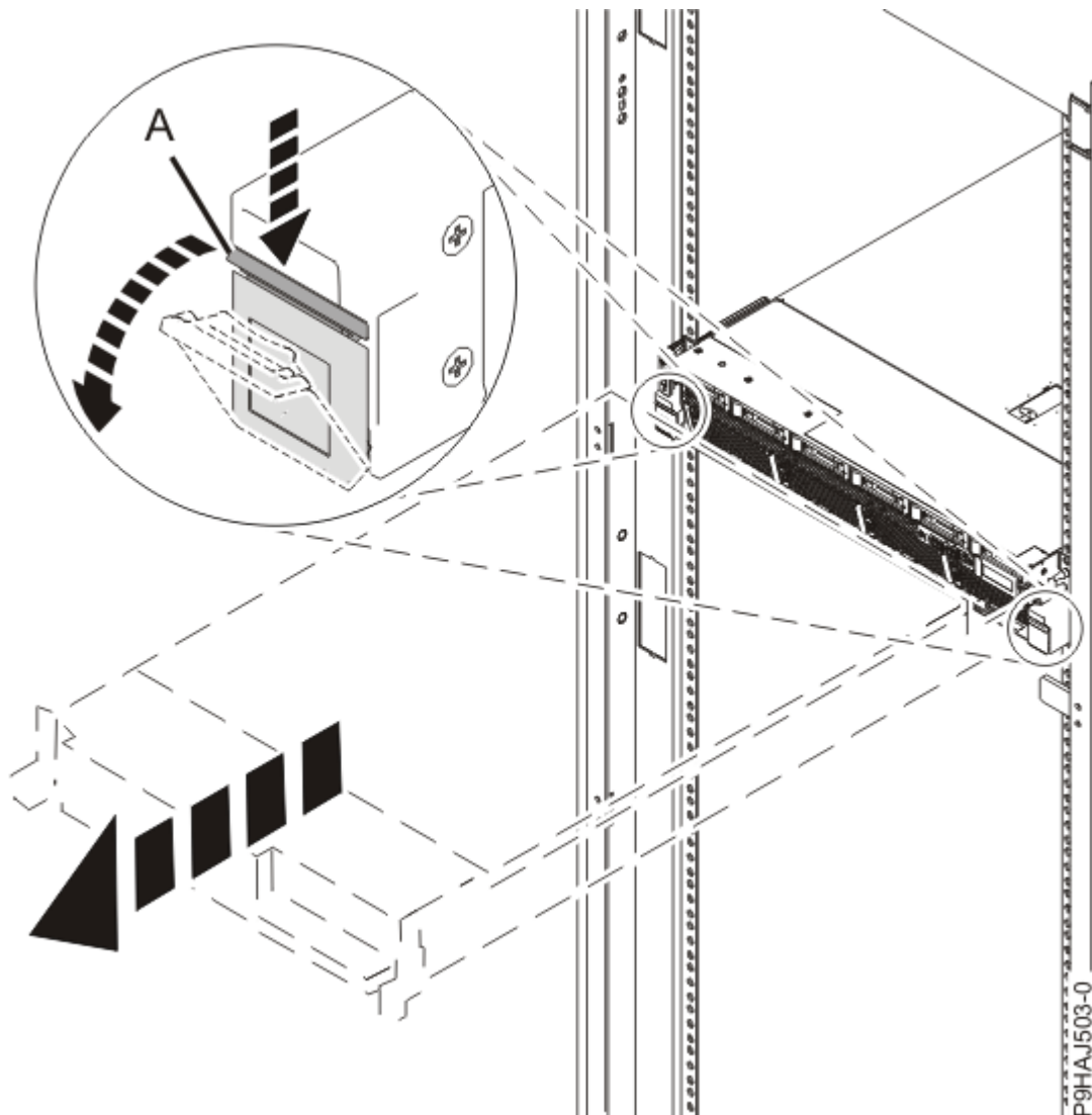
Figure 2. Déblocage des loquets latéraux
