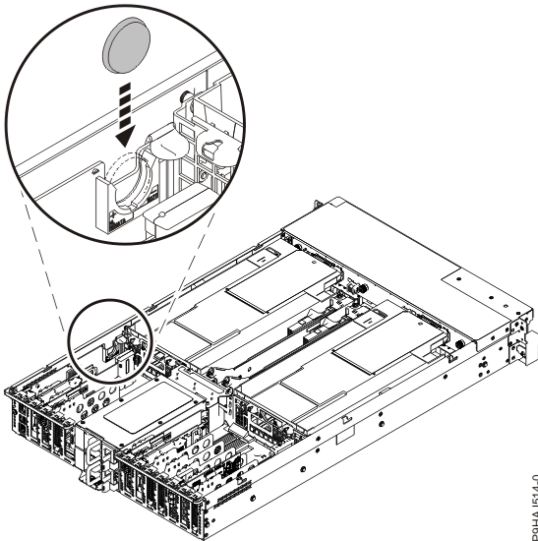
Figure 6. Insertion de la batterie de l'horloge
