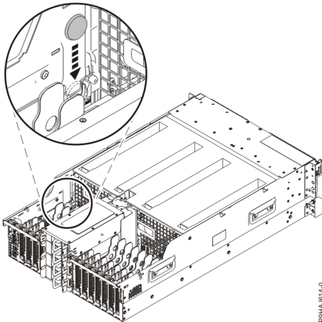
Figure 9. Insertion de la batterie de l'horloge dans un système monté en armoire
