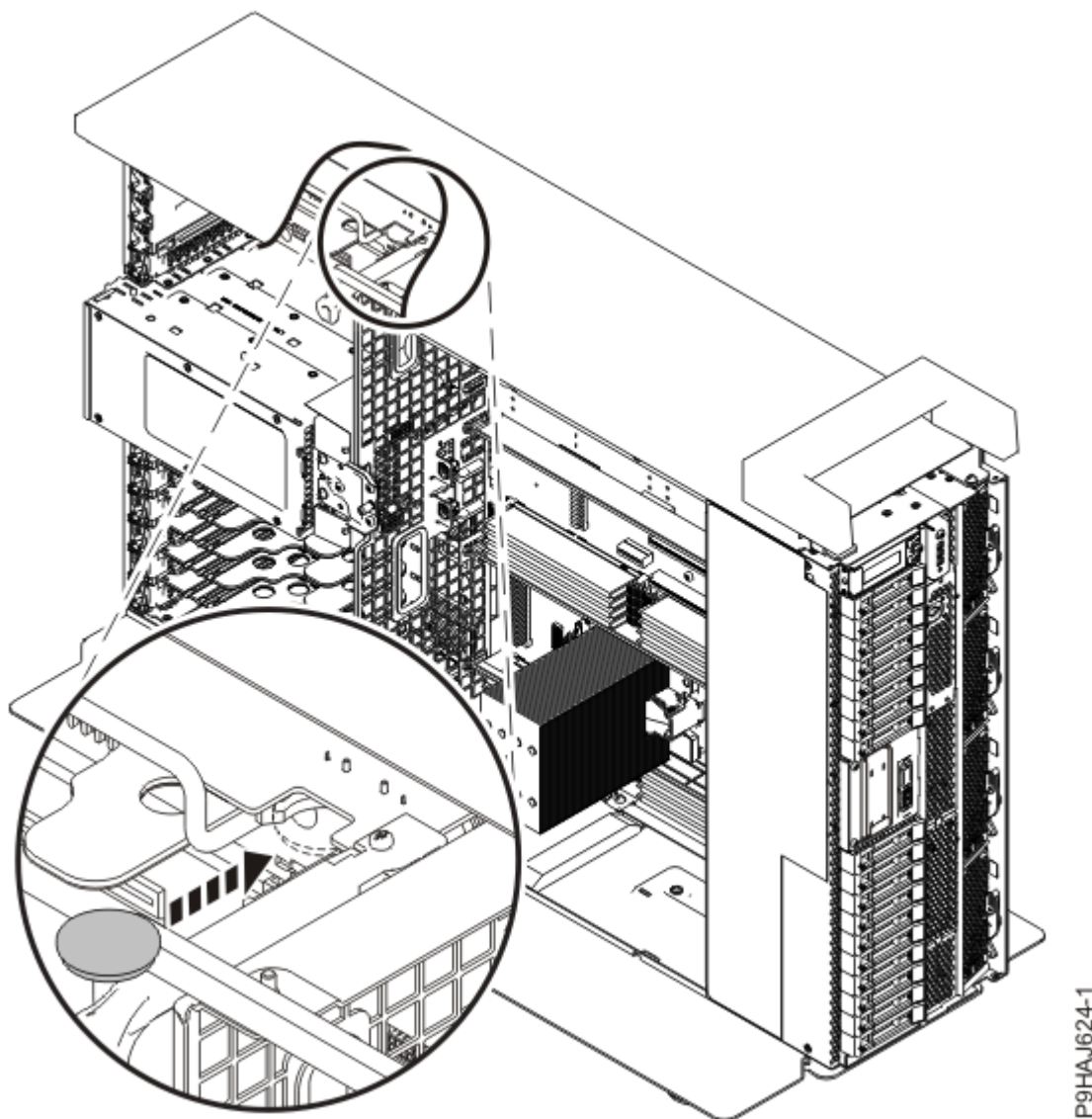
Figure 10. Insertion de la batterie de l'horloge dans un système autonome
