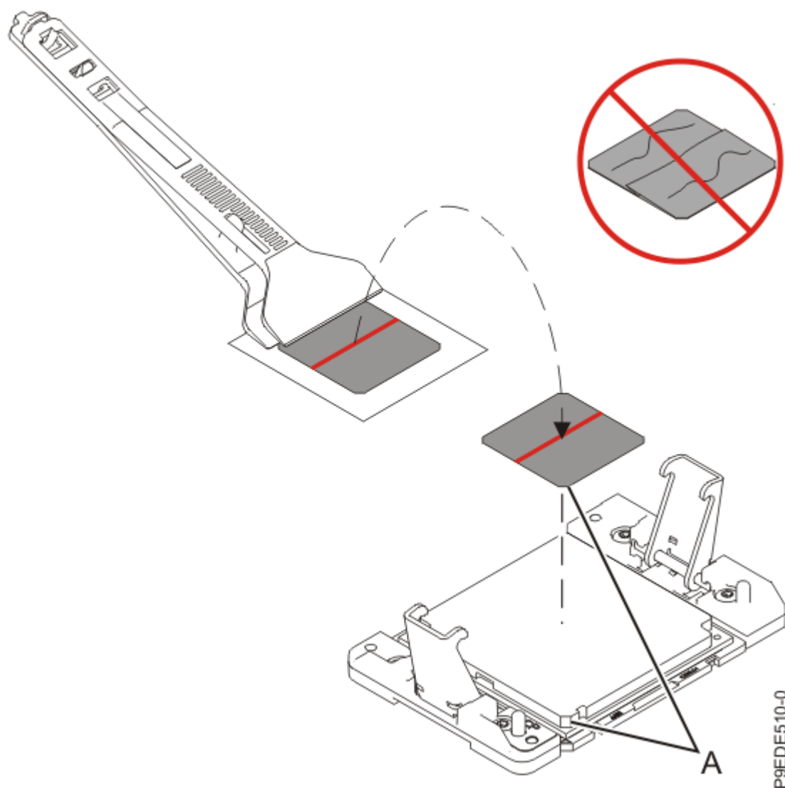
Figure 19. Installation du matériau d'interface thermique argenté sur le module processeur système
