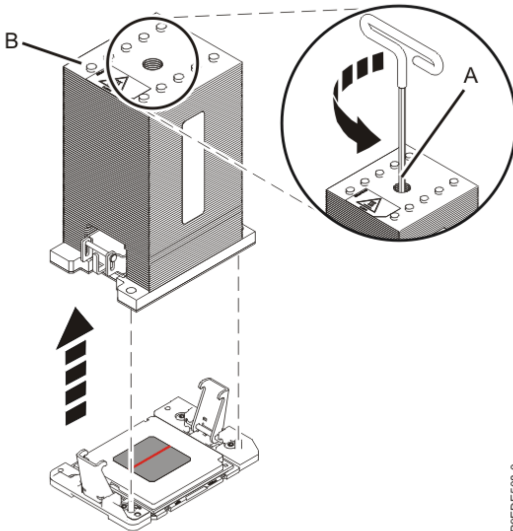
Figure 7. Retrait du dissipateur thermique
