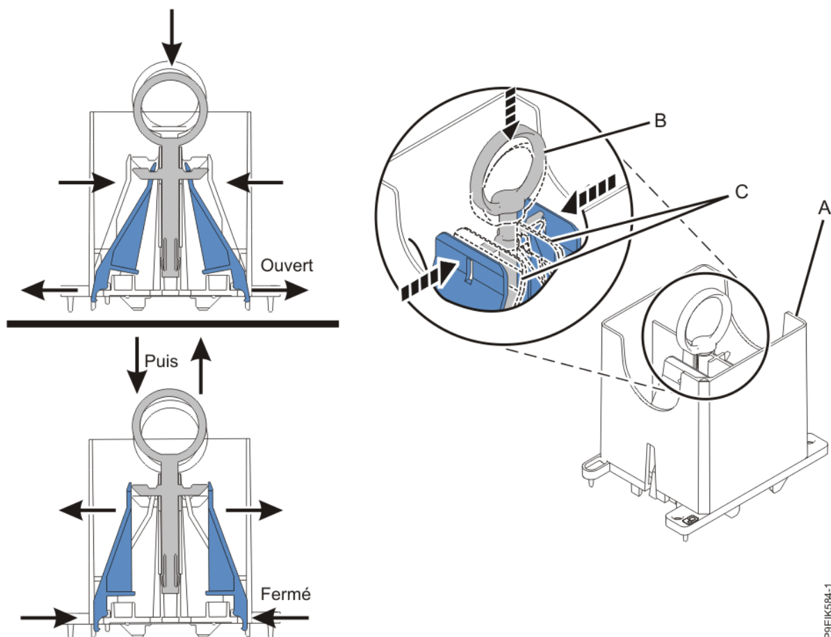
Figure 13. S'assurer que l'outil de retrait soit en position ouverte.
