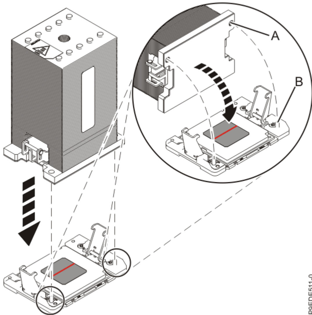
Figure 20. Installation du dissipateur thermique sur le matériau d'interface thermique argenté
