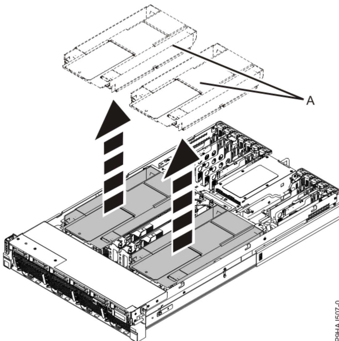
Figure 4. Retrait de la grille d'aération
