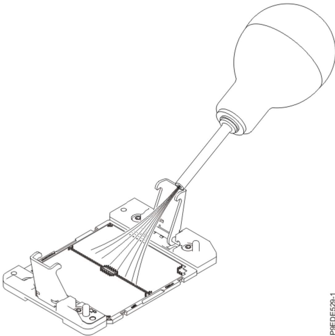
Figure 17. Retrait de la poussière et des particules du support du processeur système
