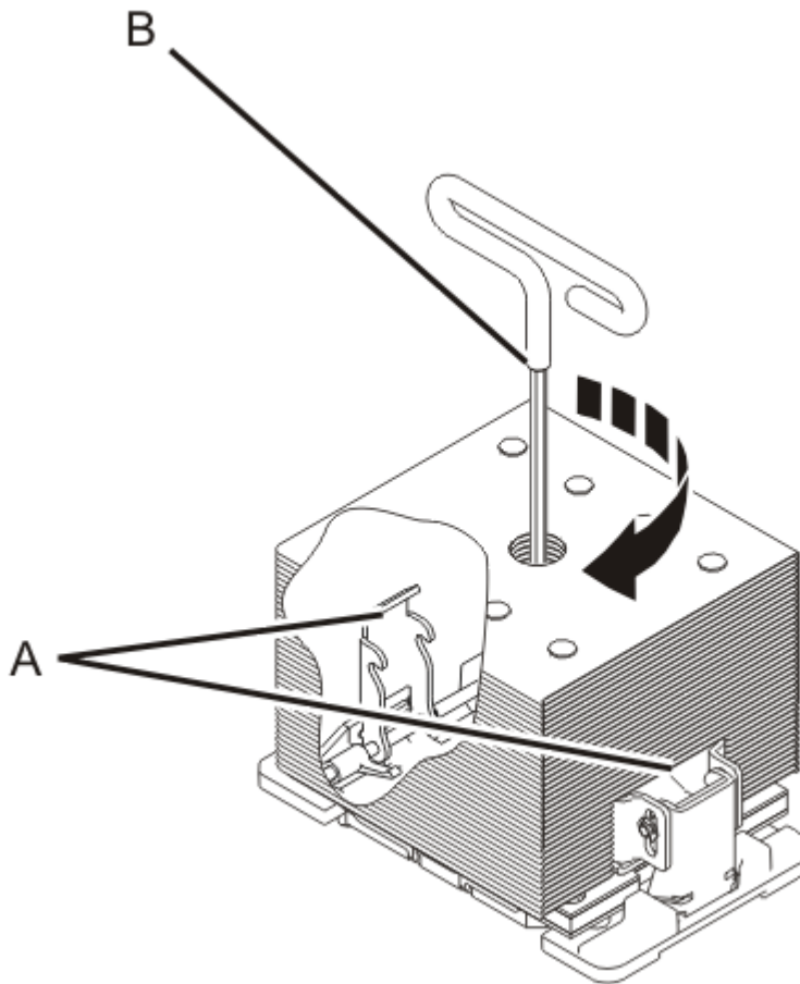
Figure 25. Serrage de la vis de pression centrale sur le dissipateur thermique
