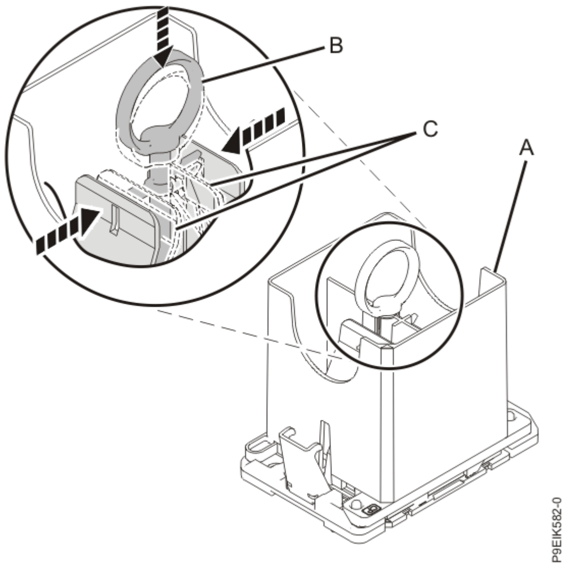
Figure 19. Retrait de l'outil du module de processeur système
