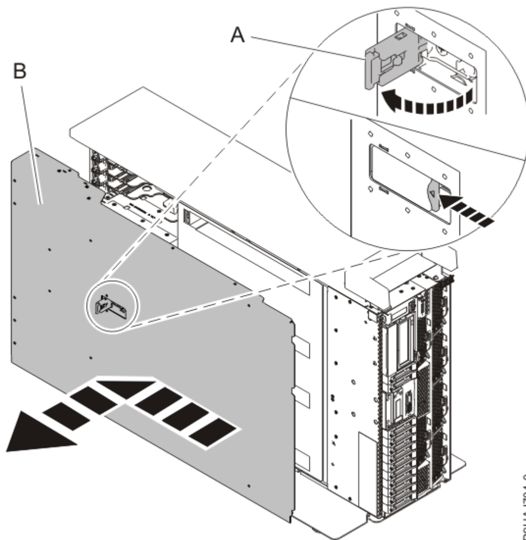
Figura 5. Extracción de la cubierta de acceso de servicio
