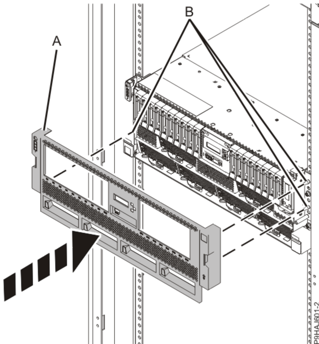
Figura 17. Instalación de la cubierta frontal
