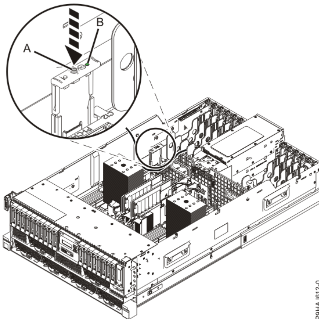
Figura 6. Activación del LED de identificación para un sistema montado en bastidor
