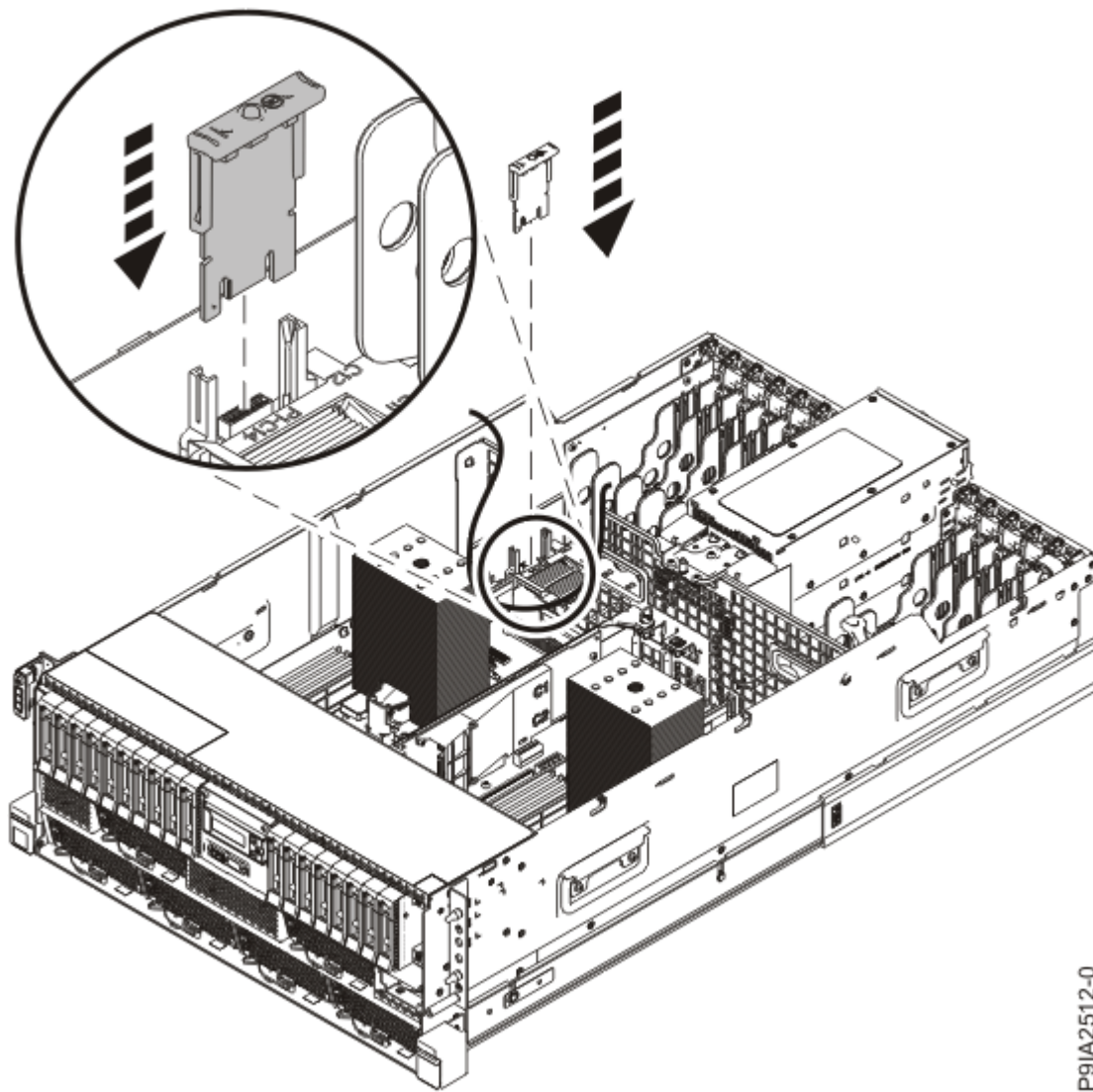
Figura 12. Sustitución de la tarjeta TPM en un sistema montado en bastidor
