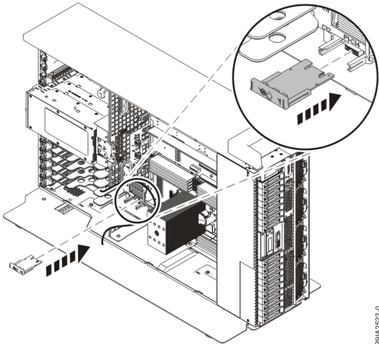
Figura 13. Sustitución de la tarjeta TPM en un sistema autónomo
