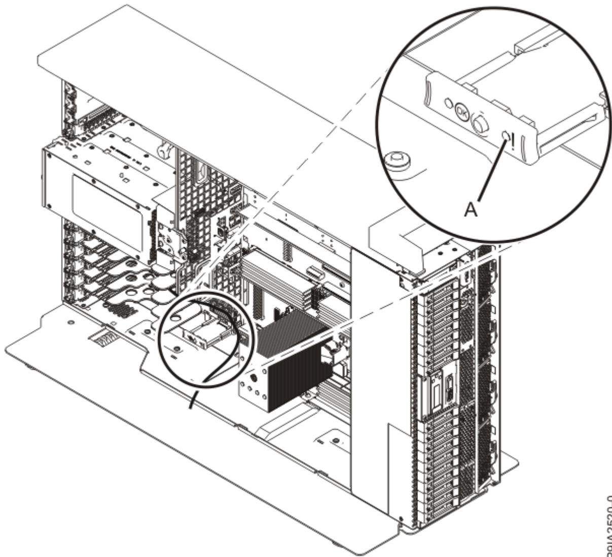
Figura 9. Ubicación del LED del indicador de servicio de la tarjeta de módulo de plataforma fiable en un servidor autónomo
