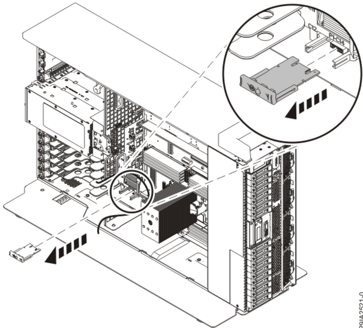
Figura 11. Extracción de la tarjeta TPM de un sistema autónomo
