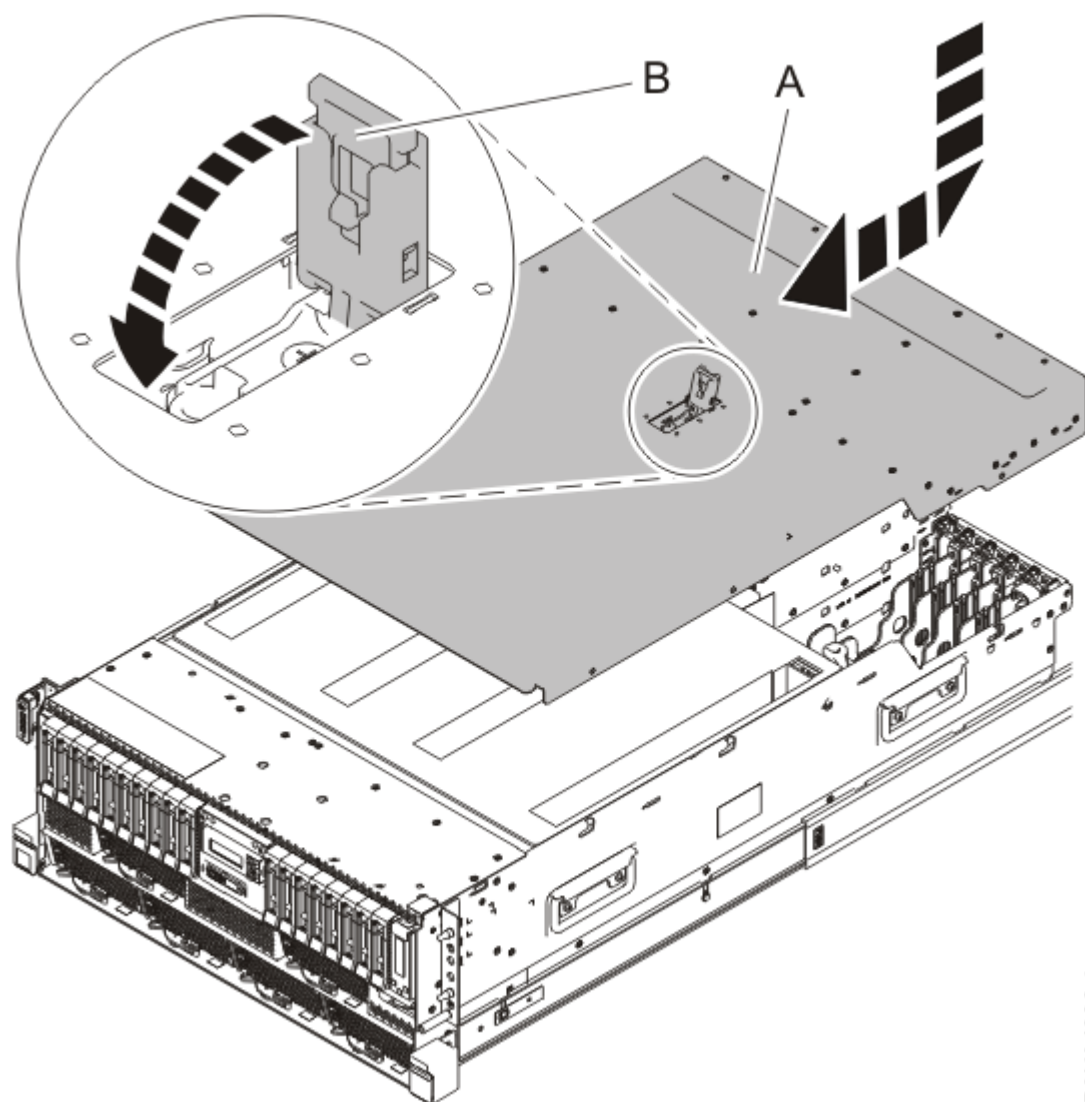
Figura 14. Instalación de la cubierta de acceso de servicio
