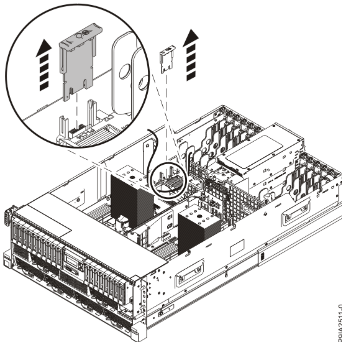
Figura 10. Extracción de la tarjeta TPM de un sistema montado en bastidor
