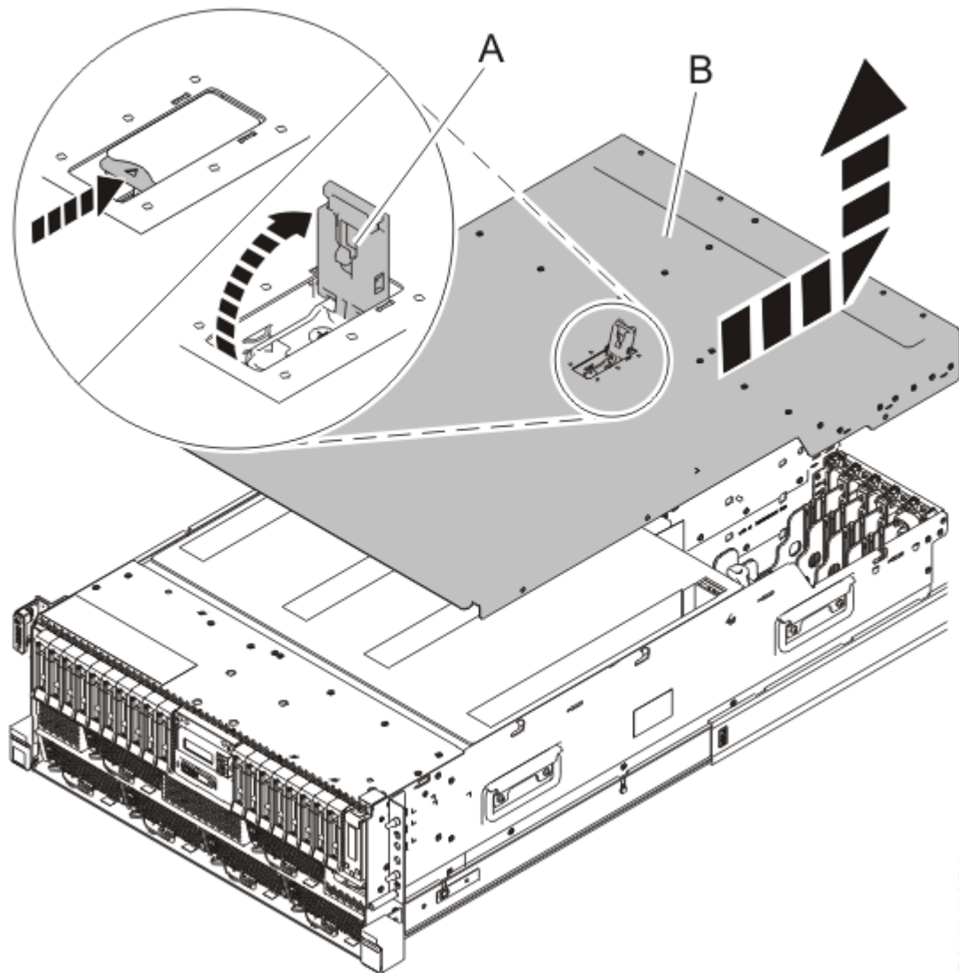
Figura 4. Extracción de la cubierta de acceso de servicio de un sistema montado en bastidor
