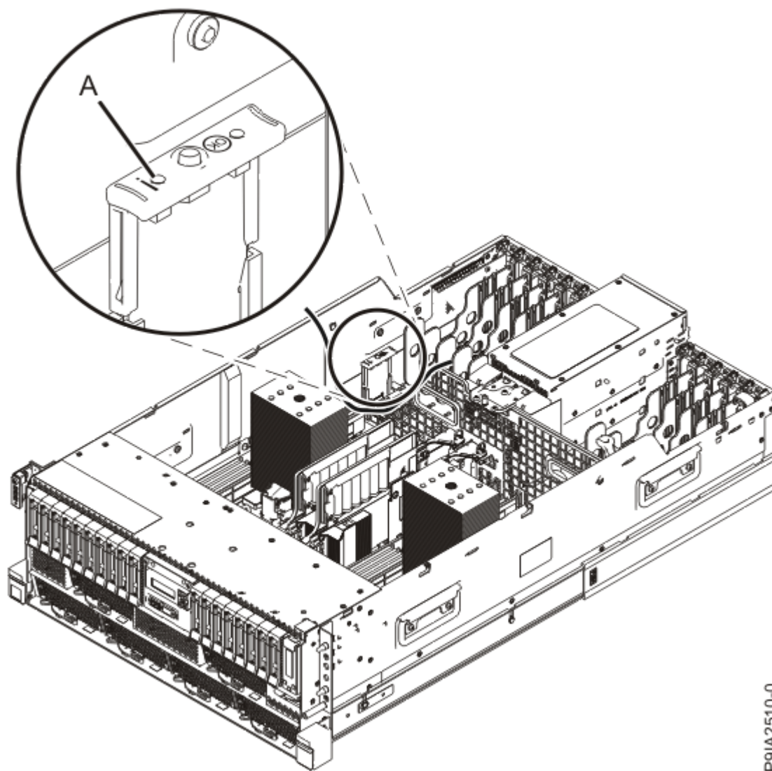
Figura 8. Ubicación del LED del indicador de servicio de la tarjeta de módulo de plataforma fiable en un servidor montado en bastidor
