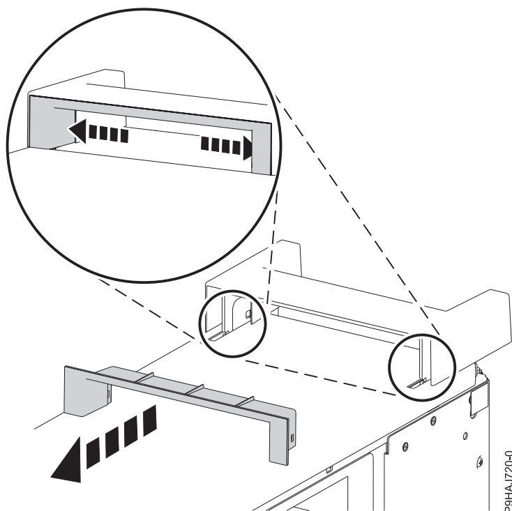
Figura 12. Extracción de la pieza de plástico de la tapa de asa
