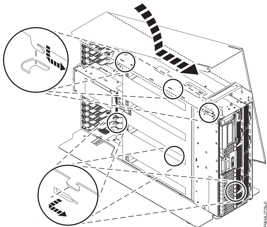
Figura 21. Instalación de la cubierta lateral
