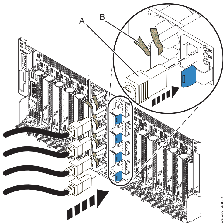
Figura 46. Conexión de los cables de alimentación
