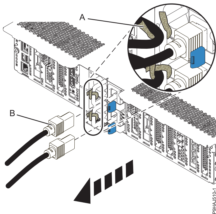
Figura 39. Extracción de los cables de alimentación
