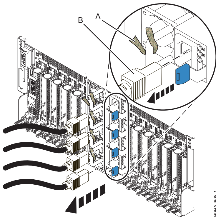
Figura 42. Extracción de los cables de alimentación
