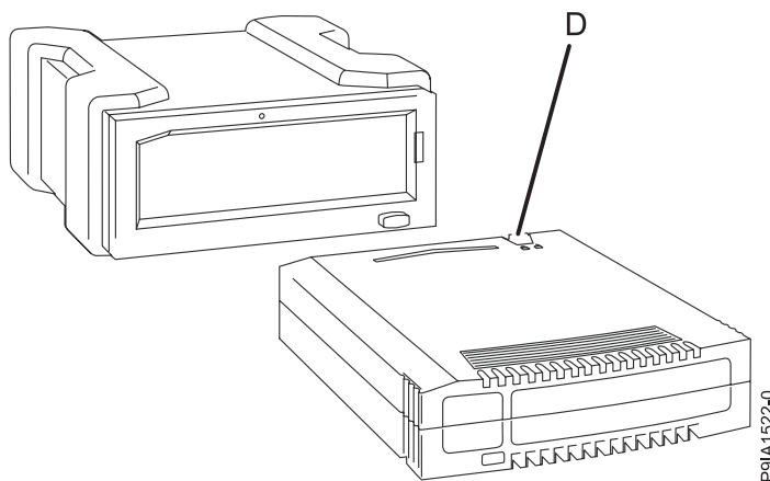
Figura 2. Vista frontal de una estación de acoplamiento USB externa y del cartucho de la unidad de disco extraíble
