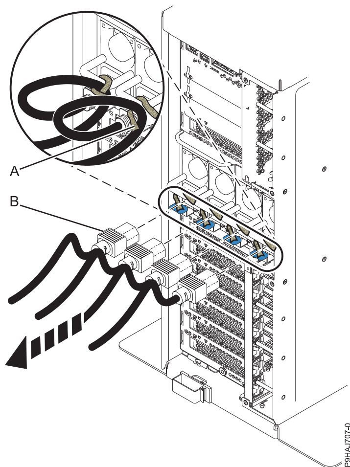
Figura 41. Extracción de los cables de alimentación de un servidor autónomo
