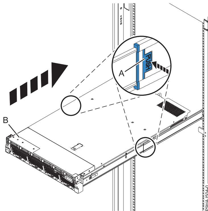
Figura 38. Colocación del sistema en la posición operativa
