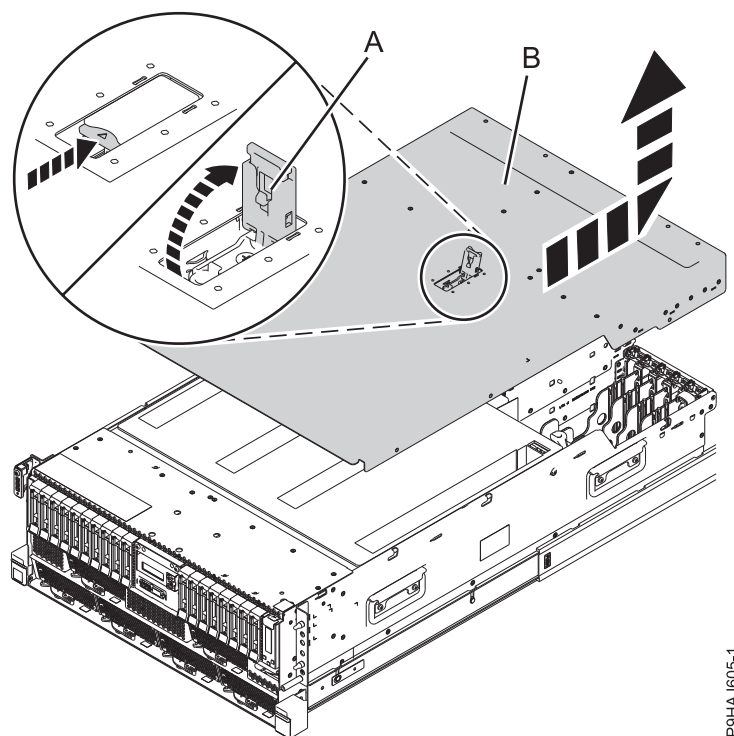
Figura 26. Extracción de la cubierta de acceso de servicio de un sistema montado en bastidor
