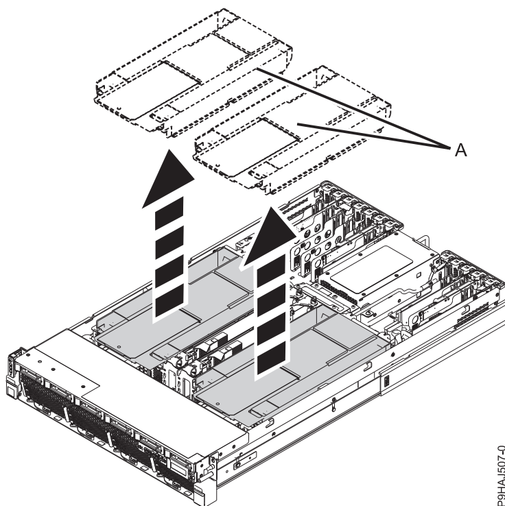
Figura 31. Extracción del deflector de aire
