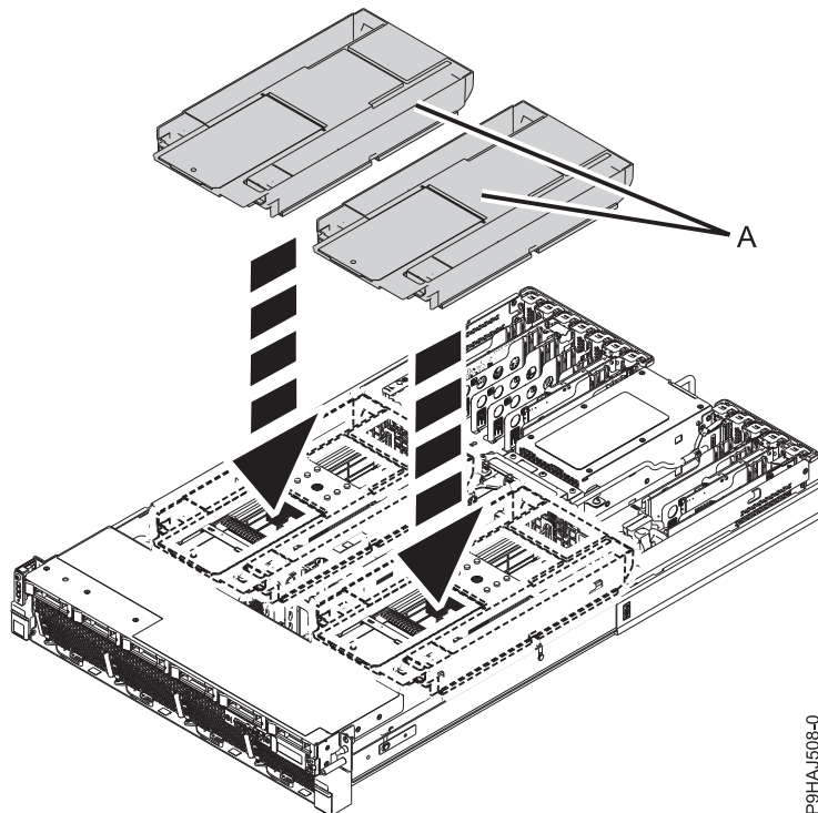
Figura 32. Sustitución del deflector de aire
